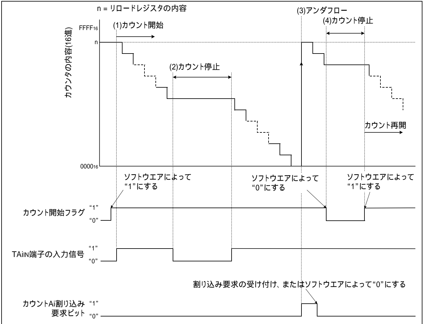
図 1 タイマモード、ゲート機能選択時の動作タイミング
