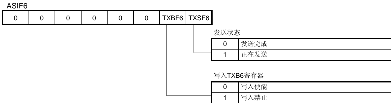
图 4-7. 异步串行接口发送状态寄存器 6 (ASIF6)的格式
