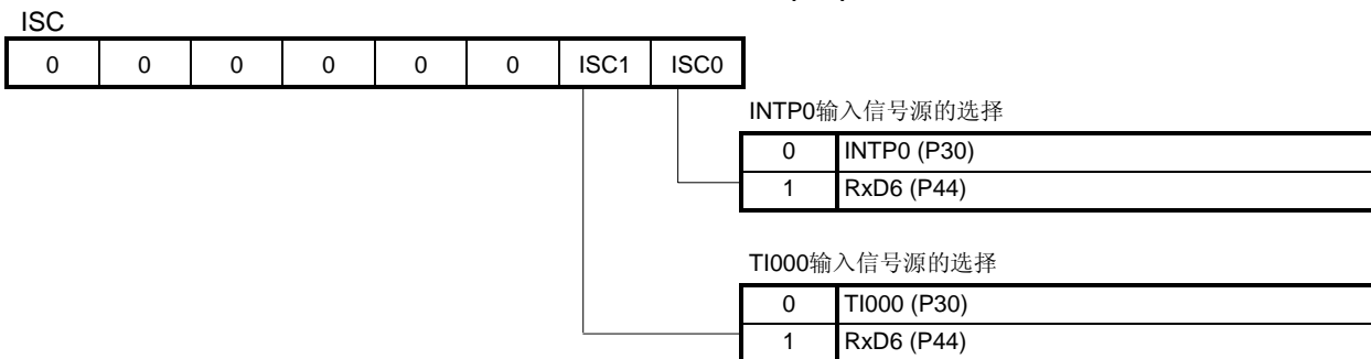
图 4-9. 输入开关控制寄存器(ISC)的格式
