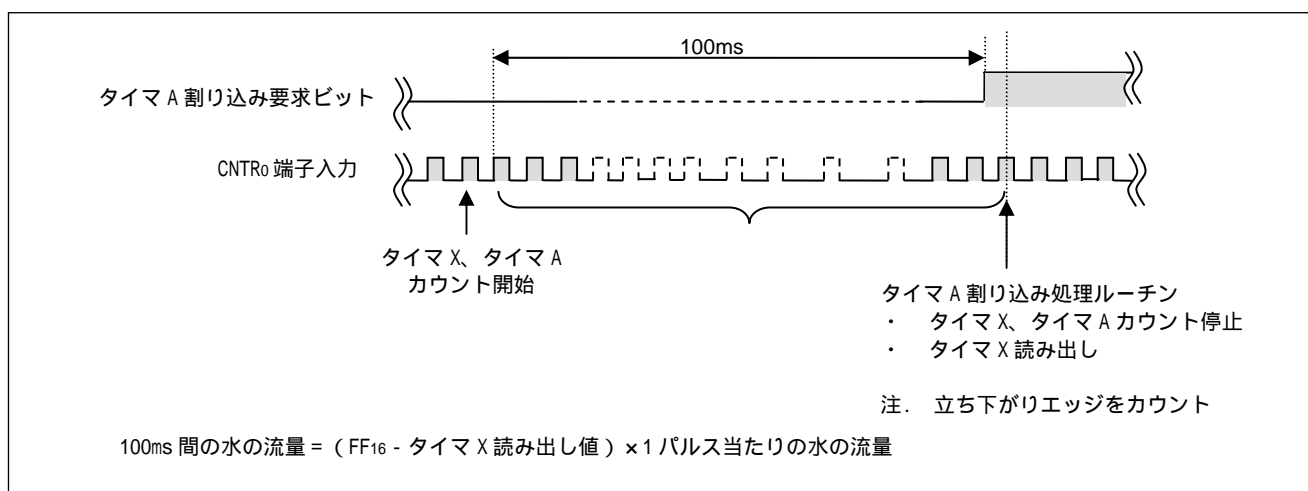
図 4. 水の流量の測定方法
