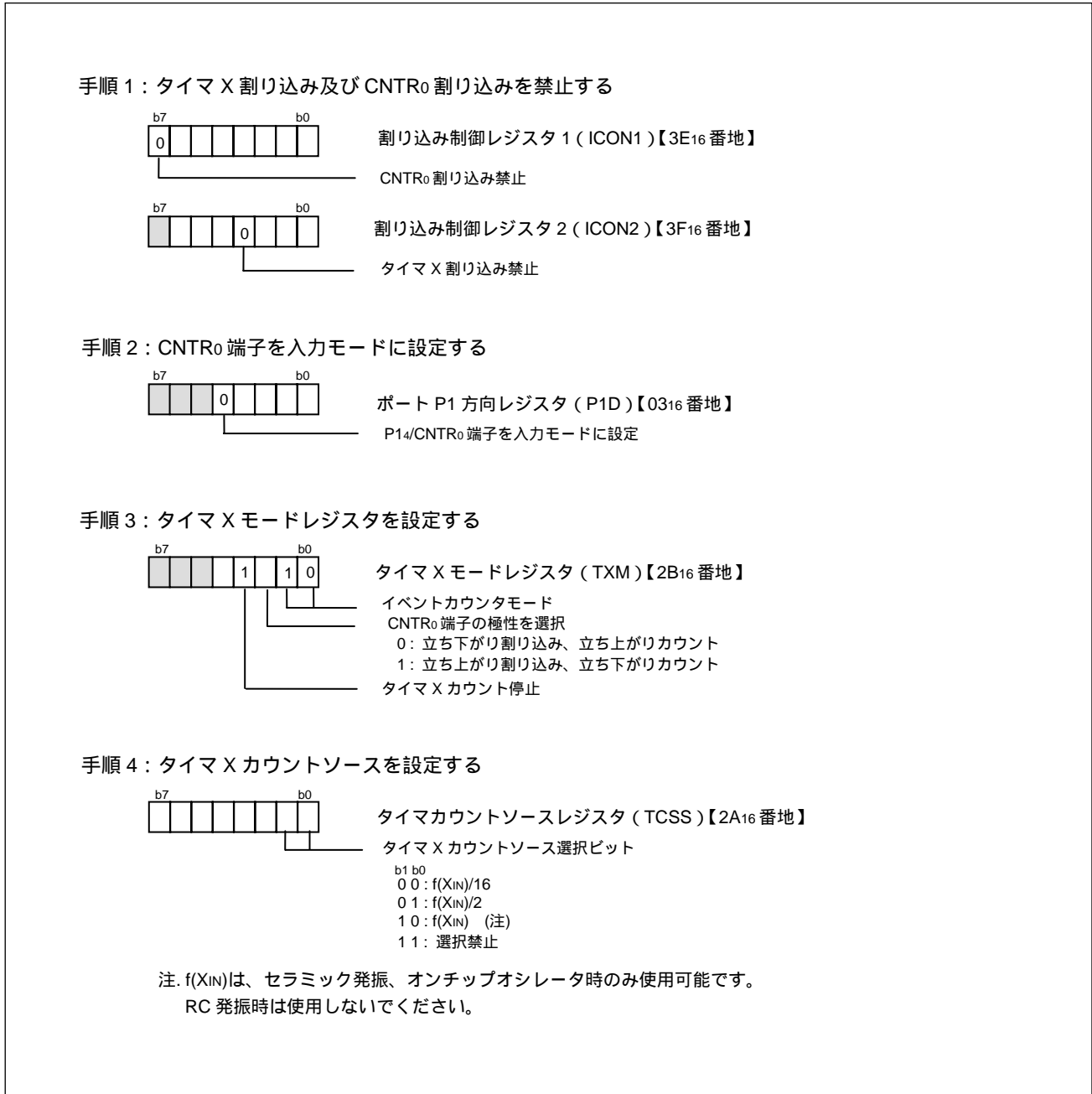
図 1. タイマ X イベントカウンタモードの設定方法(1)
