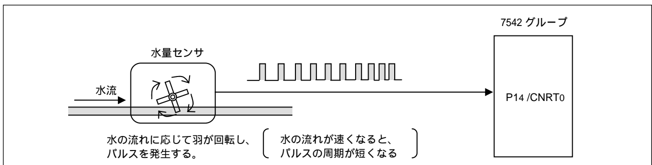
図 3. 周辺回路例
