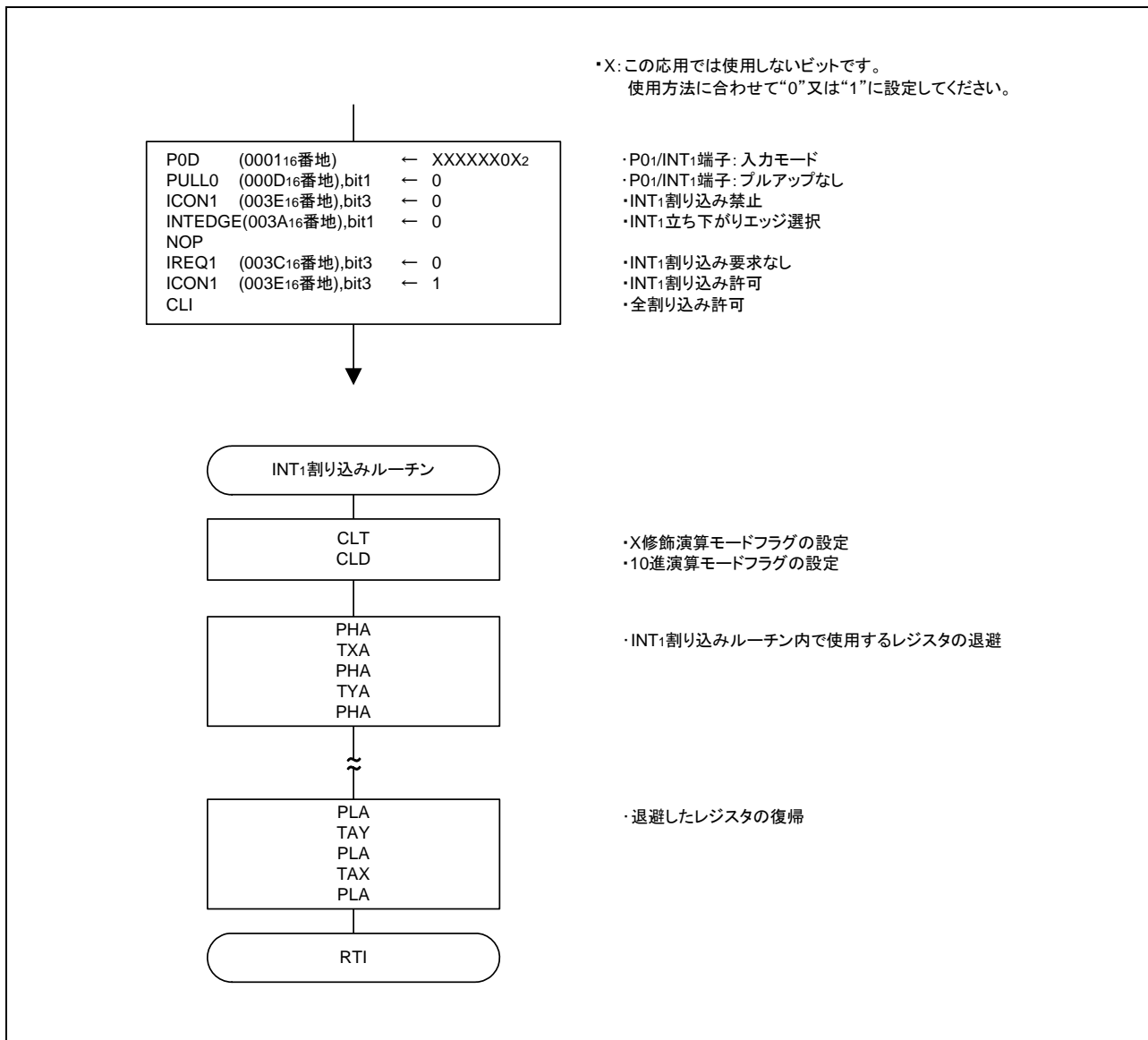
図 3.3 制御手順
