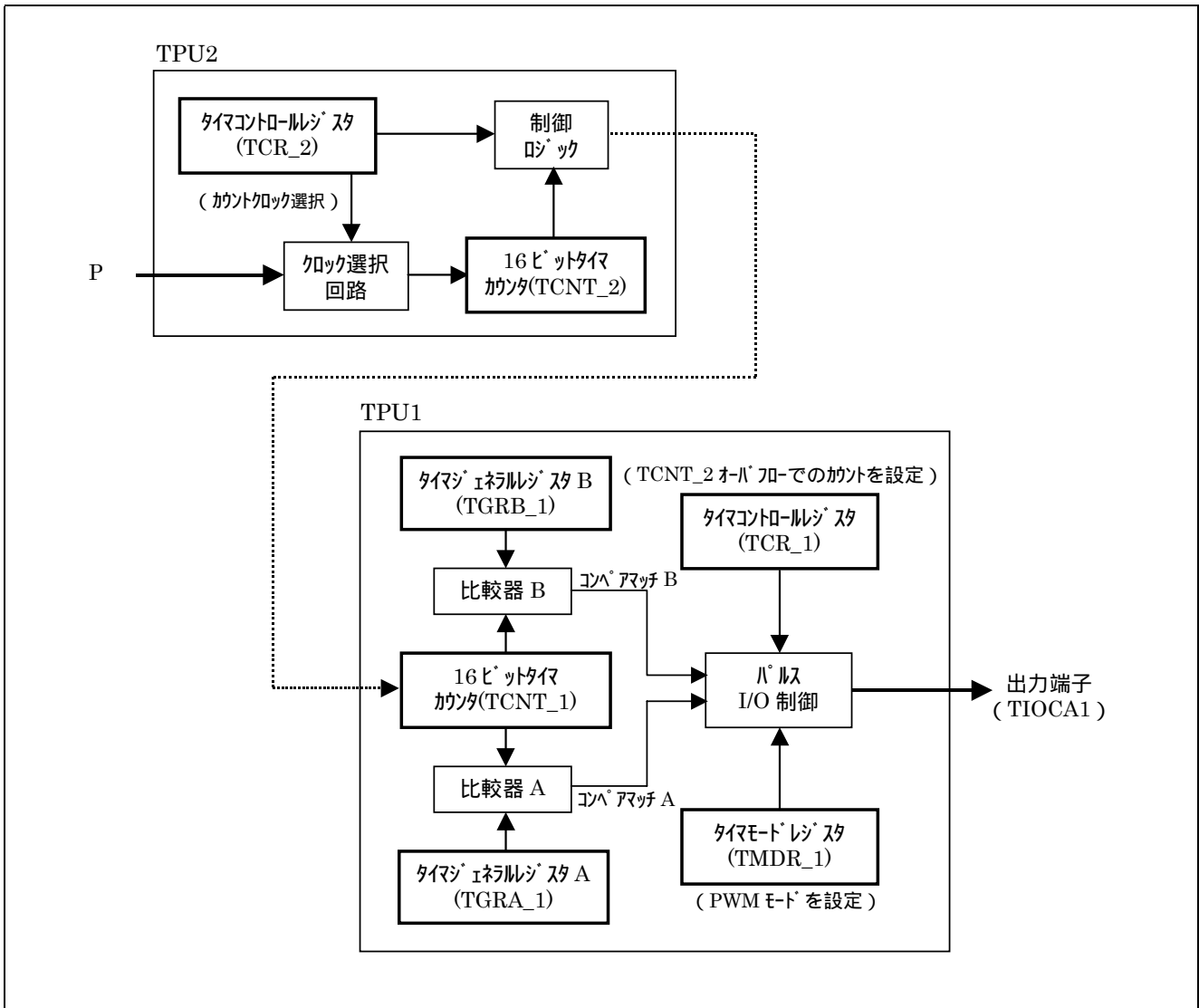
図 1 長周期パルス出力ブロック図
