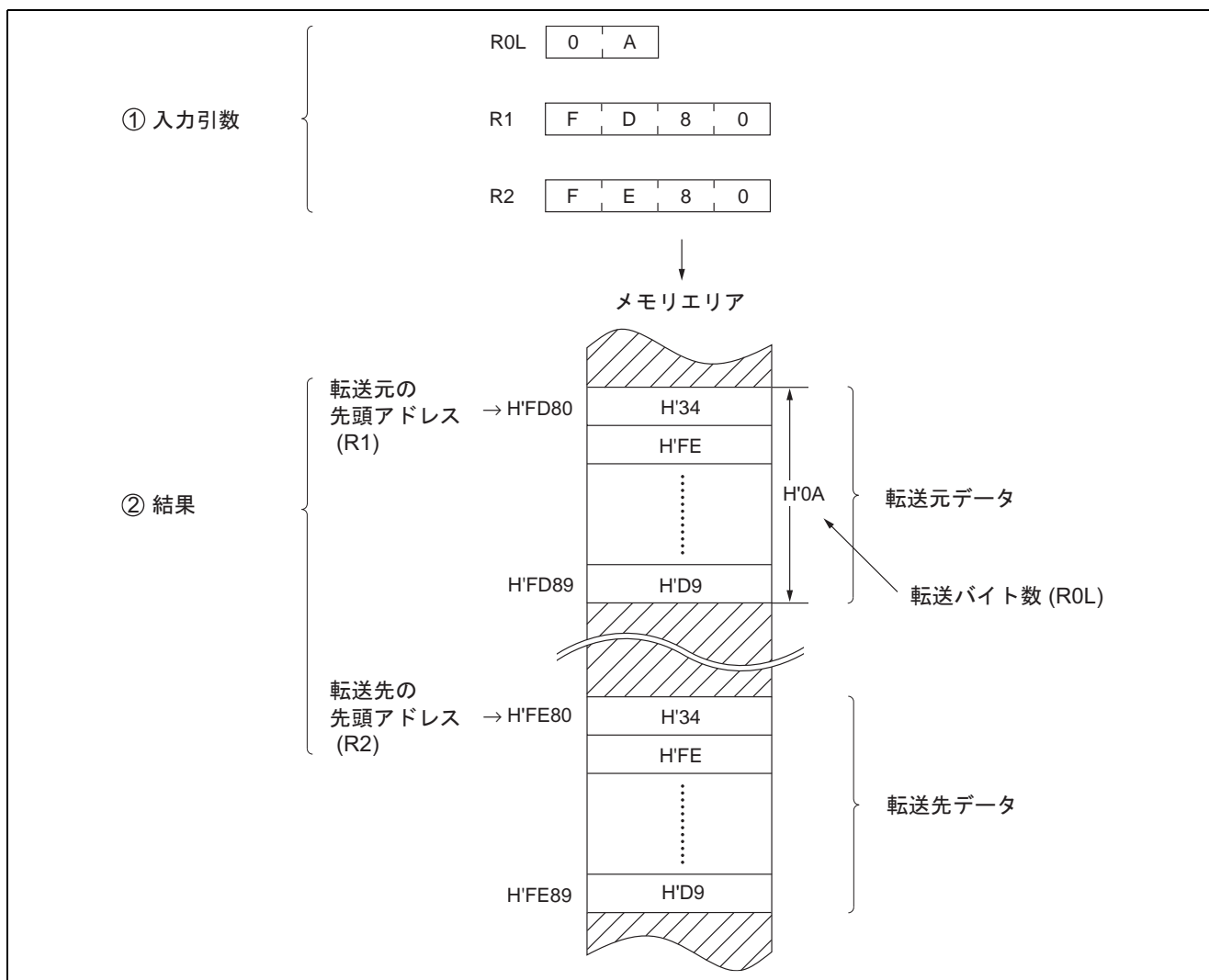
図 2-1 ソフトウェア MOVE1 の実行例
