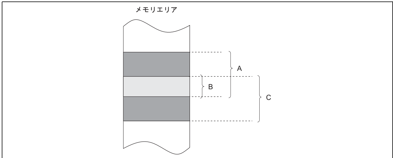
図 2-2 データメモリエリアが重なる場合のブロック転送
