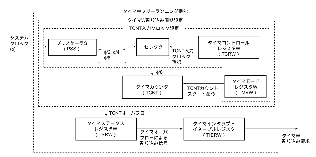
図 2.1 フリーランニング機能ブロック図
