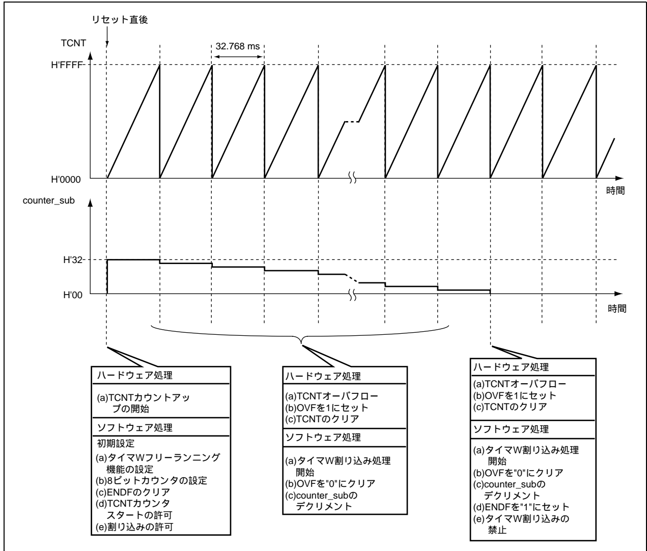
図 3.1 タイマ W16 ビットフリーランニング機能による割り込み回数のカウント動作原理
