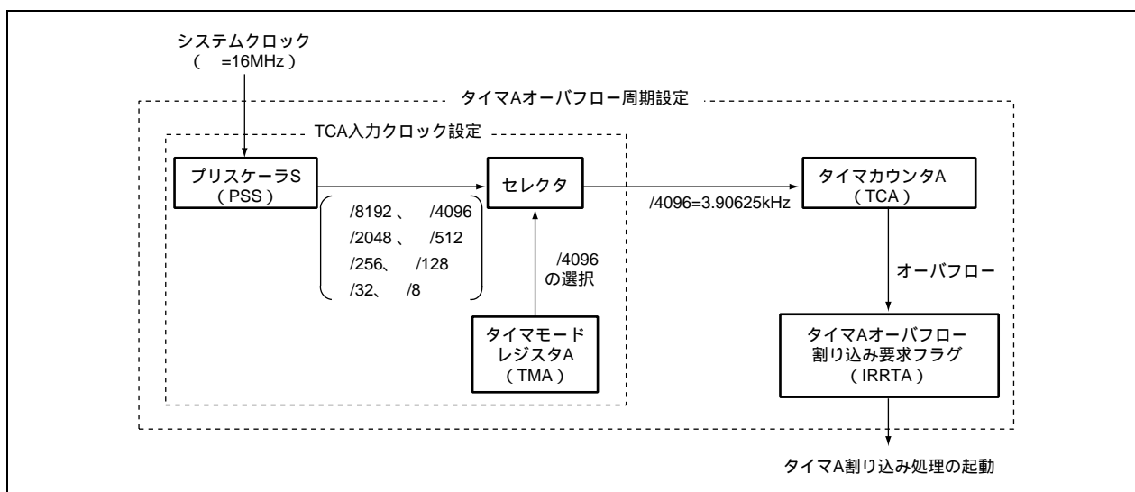
図 2.1 タイマ A インターバル機能ブロック図
