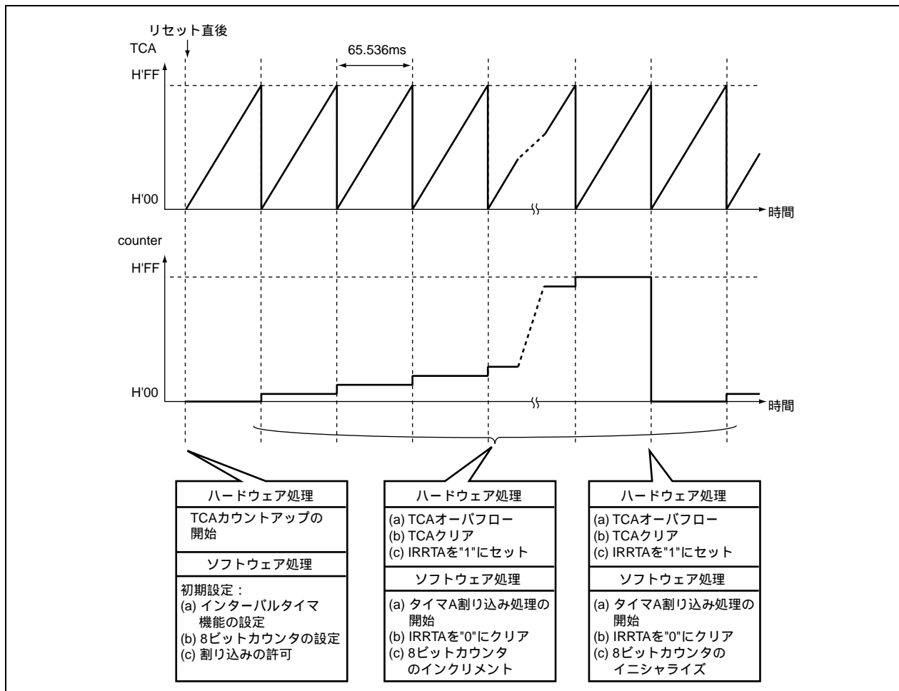
図 3.1 タイマ A インターバル機能による 8 ビットカウンタのカウントアップ動作の動作原理
