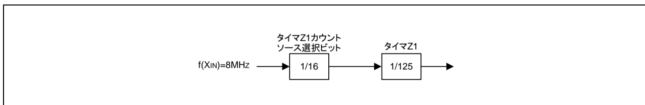
図 3.2 タイマの接続と分周比
