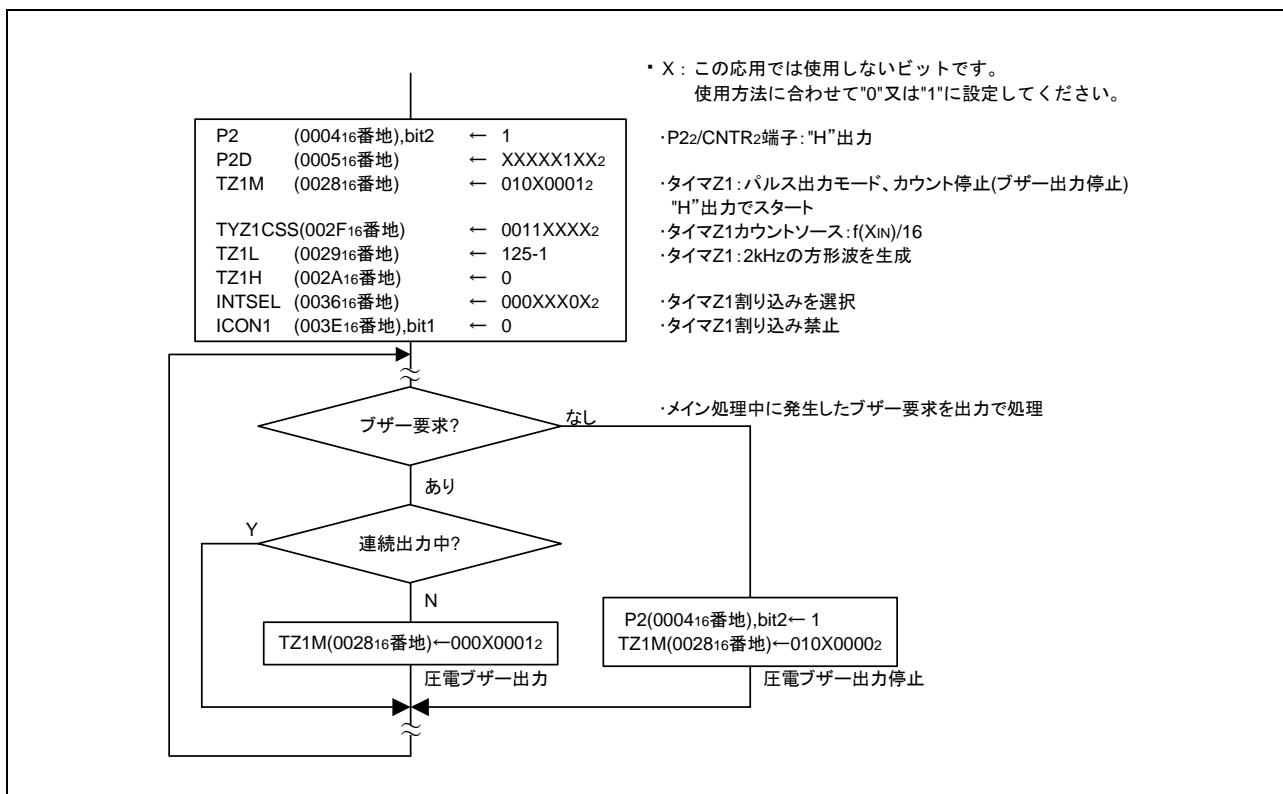
図 3.4 制御手順
