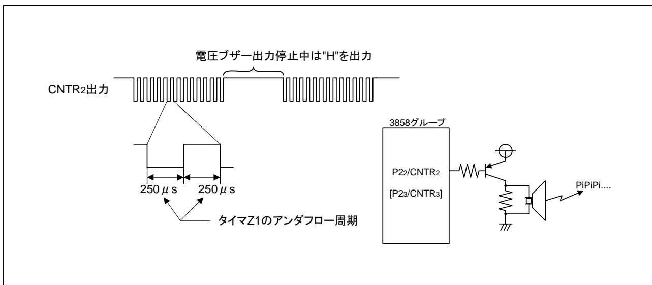
図 3.1 出力波形図及び周辺回路例
