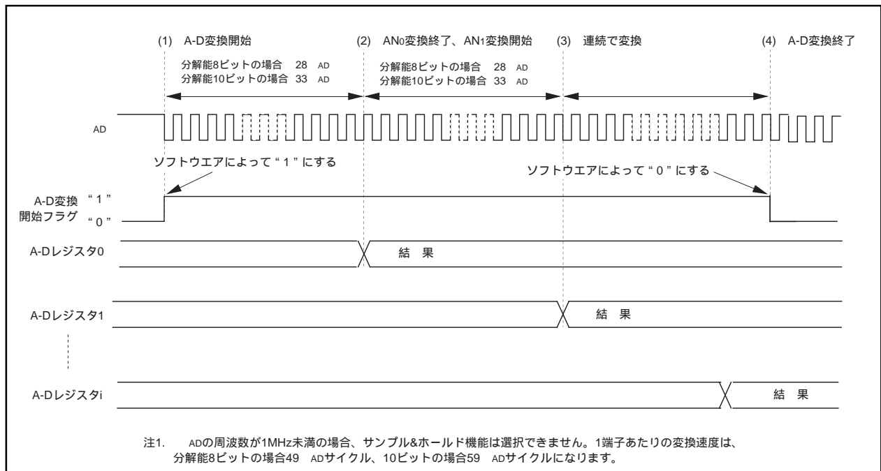
図1 繰り返し掃引モード0動作タイミング
