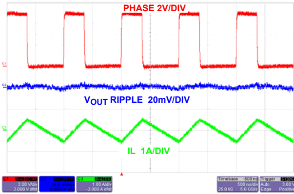
図 17. 無負荷での安定状態動作 (PWM)
