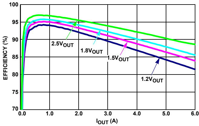
図 5. 効率 vs 負荷電流 (1 MHz、3.3 V_{IN} 、PWM)
