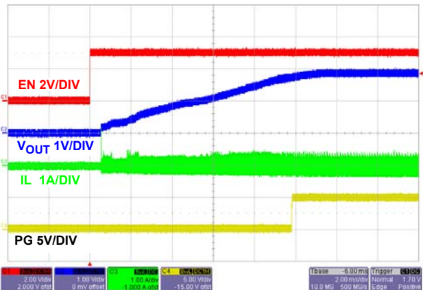
図 22. 無負荷時のソフトスタート (PWM)
