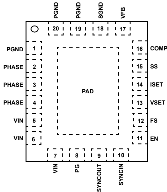
ISL8016 (20 LD QFN) 上面図
