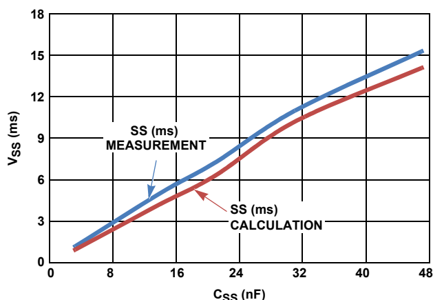
図 38. ソフトスタート時間 vs C_{SS}
