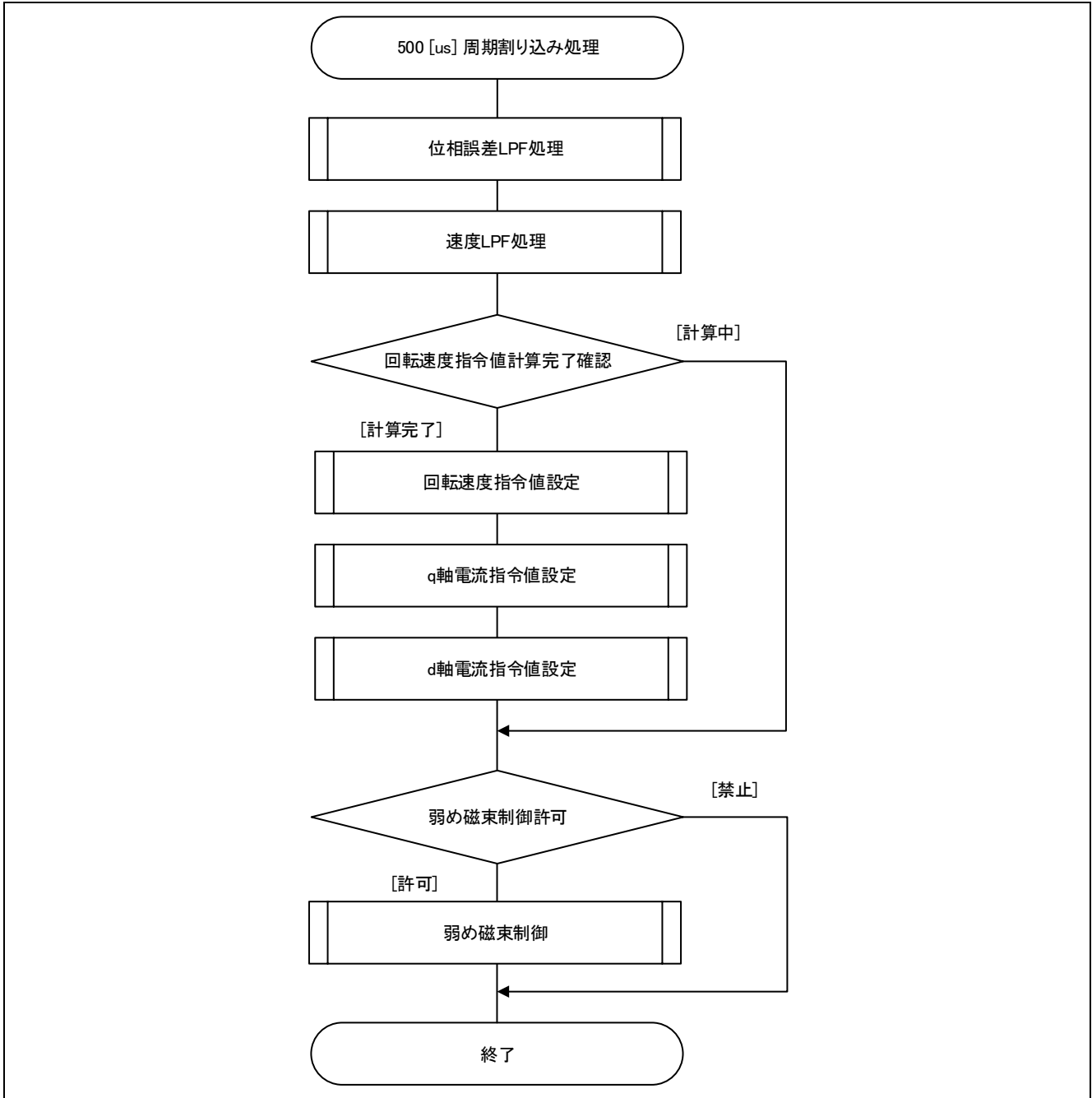
図 3-15 500 [μs]周期割り込み処理フローチャート
