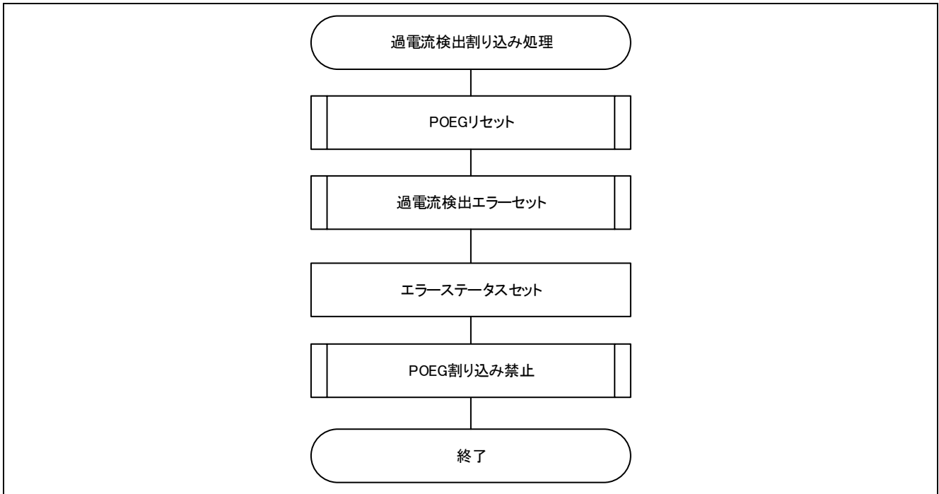
図 3-16 過電流検出割り込み処理フローチャート
