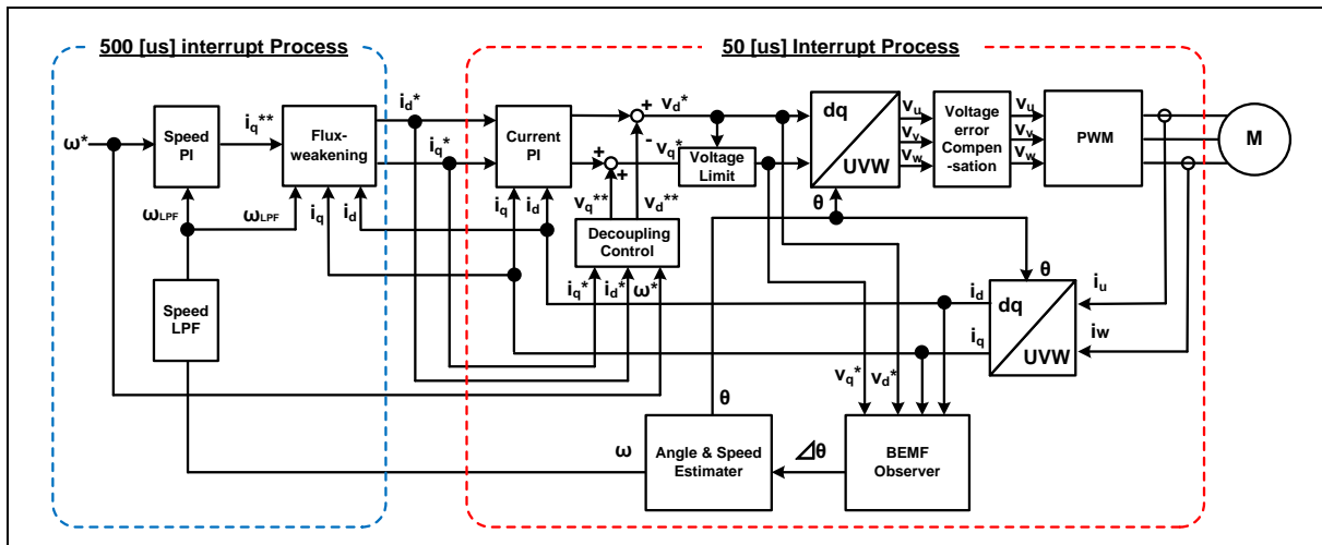
図 3-7 センサレスベクトル制御概略ブロック図(センサレス制御時)
