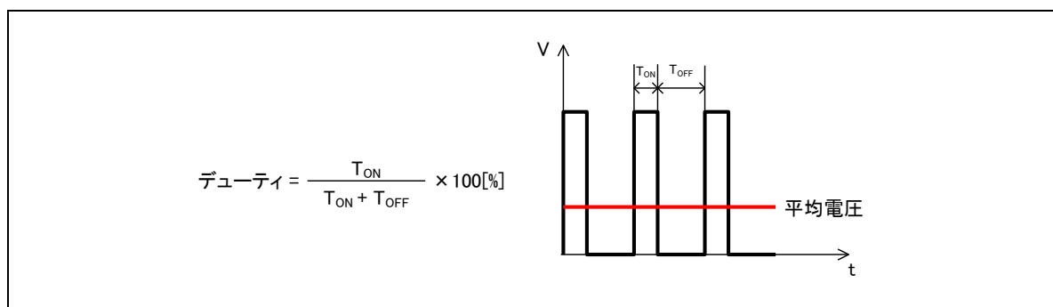
図 3-2 デューティの定義
