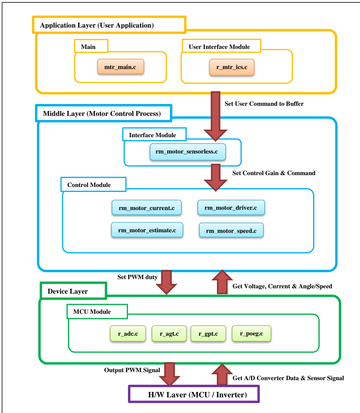
図 2-7 モジュール構成
