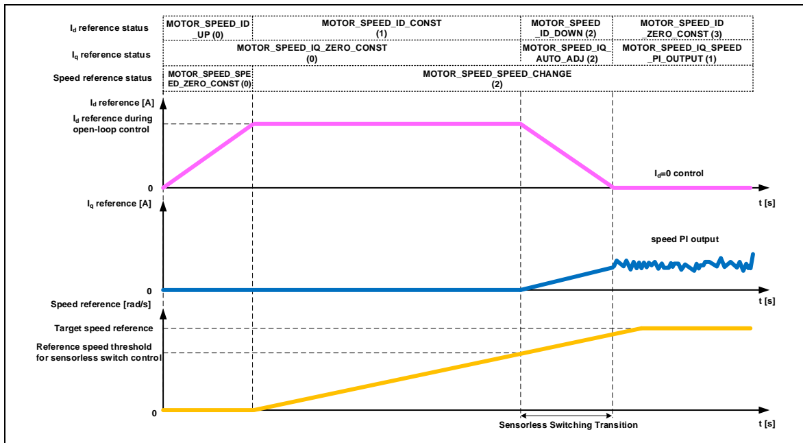
図 3-4 センサレスベクトル制御ソフトウェアの始動制御内容
