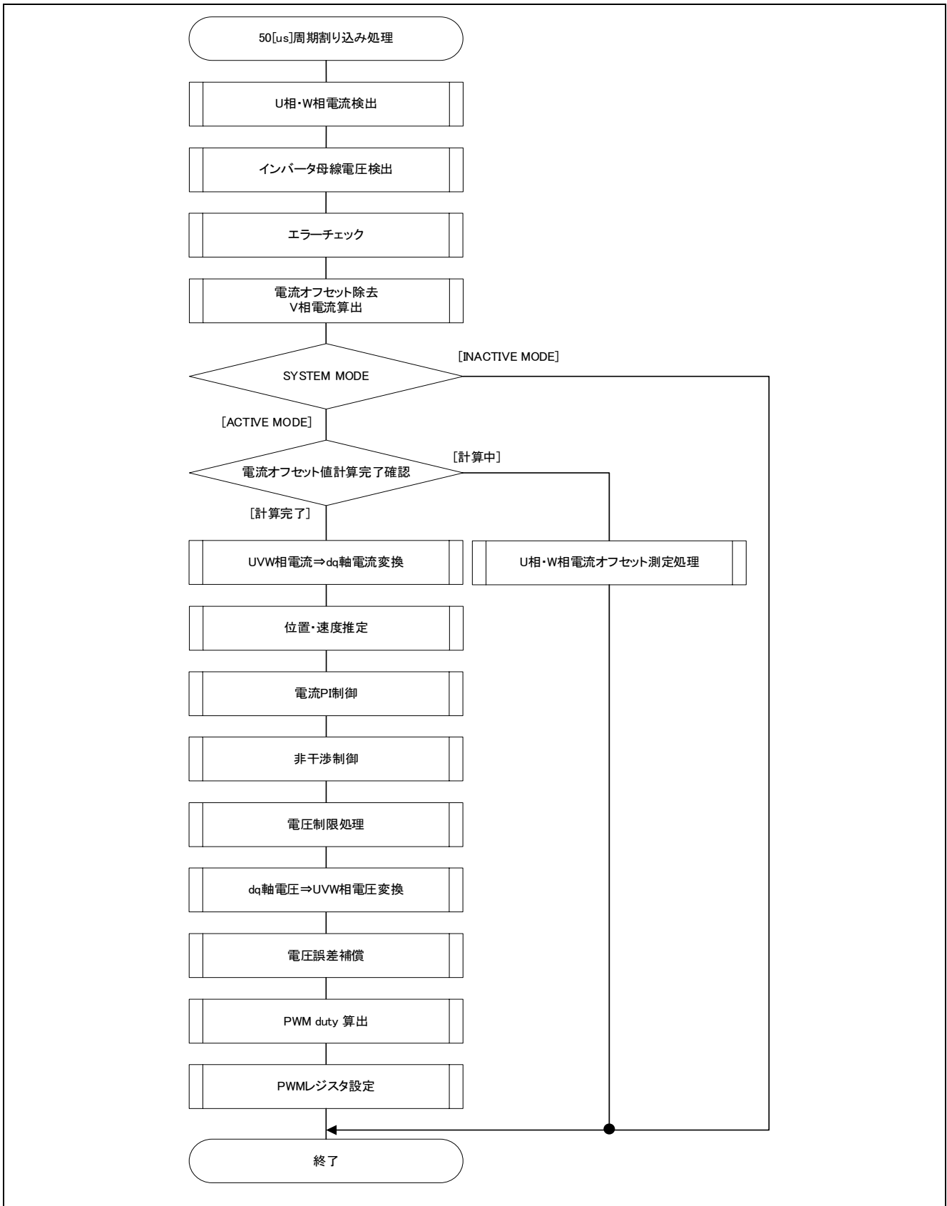
図 3-14 50[μs]周期割り込み処理フローチャート
