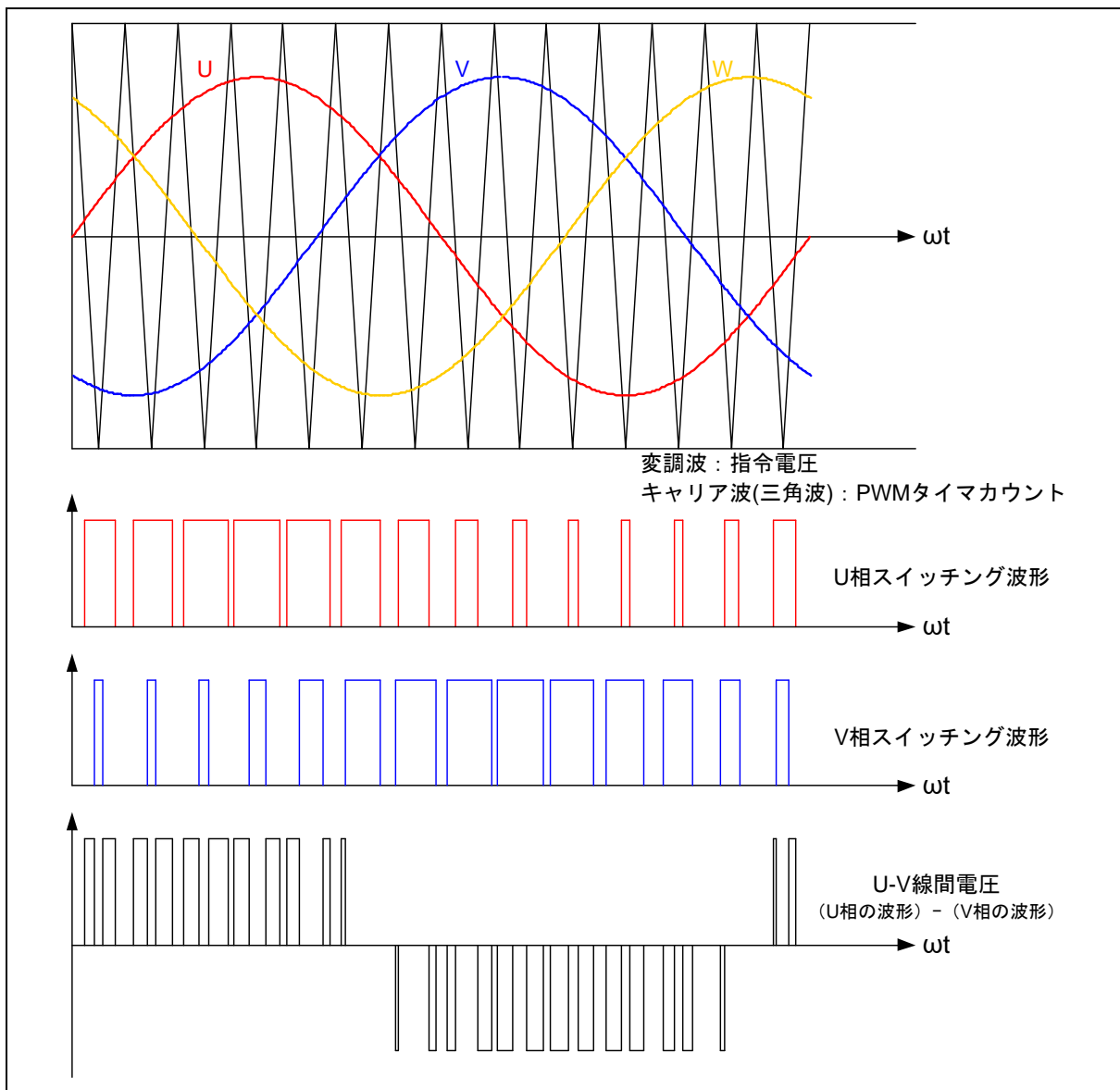
図 3-1 三角波比較法の概念図
