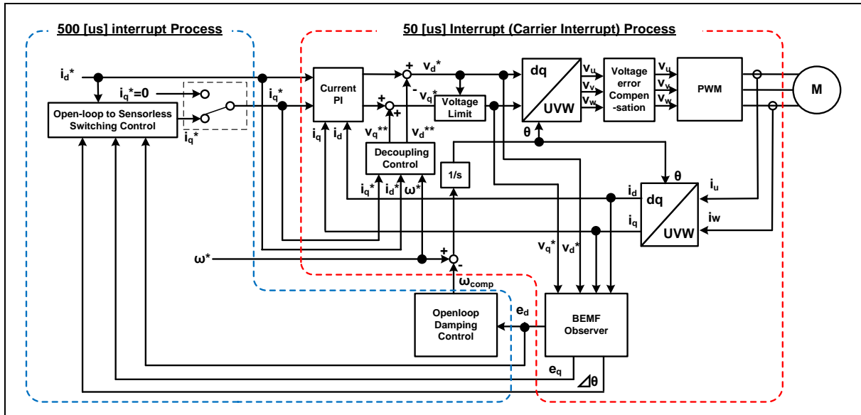
図 3-6 センサレスベクトル制御概略ブロック図(オープンループ制御時)
