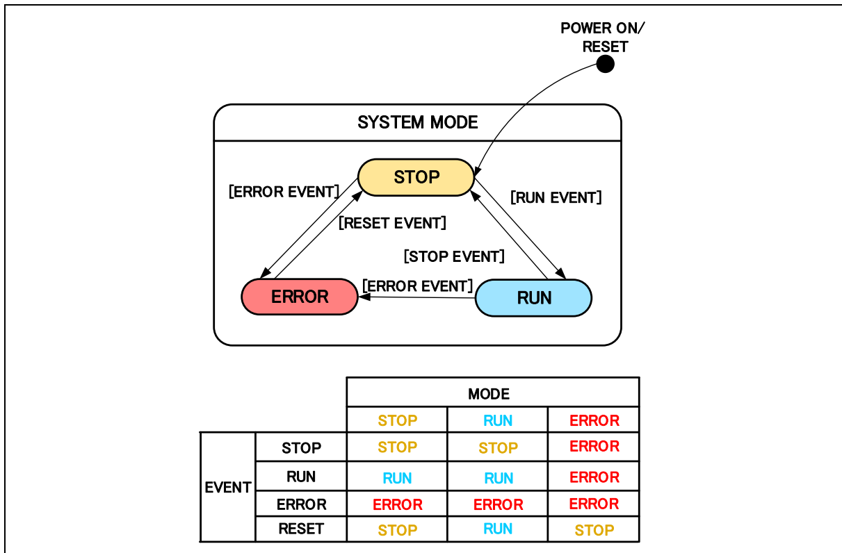
図 3-3 センサレスベクトル制御ソフトウェアの状態遷移図
