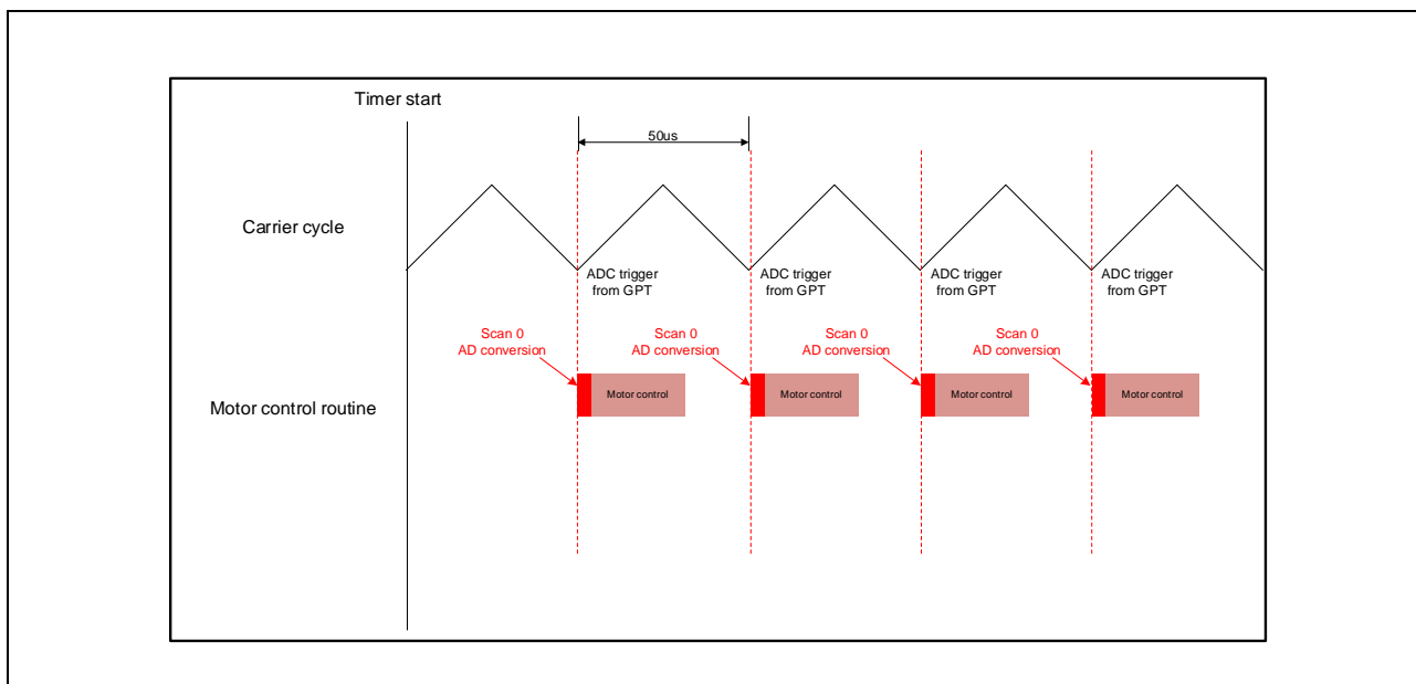
図 3-5 AD トリガタイミング
