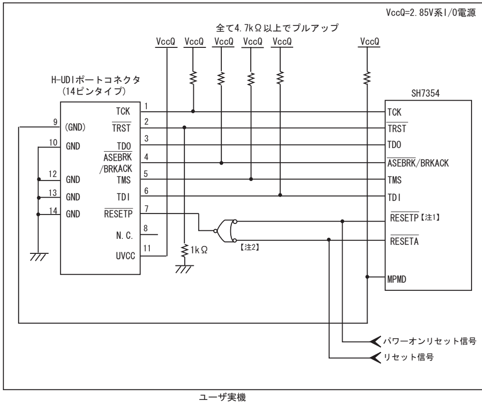
図 1.4 E10A-USB 使用時の H-UDI ポートコネクタ - チップ間の推奨接続例(14 ピンタイプ)
