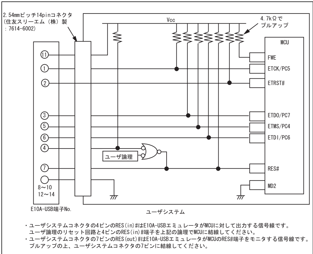
図 1.3 E10A-USB との接続例
