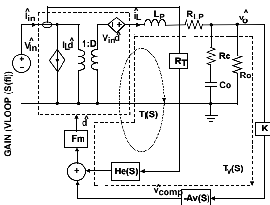
図 60. 同期整流型降圧レギュレータの小信号モデル
