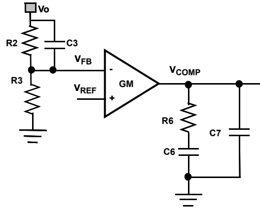
図 61. タイプ II 補償回路
