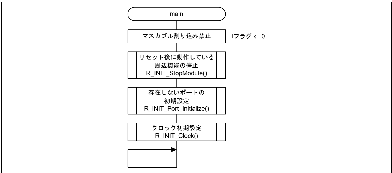
図 3.1 メイン処理
