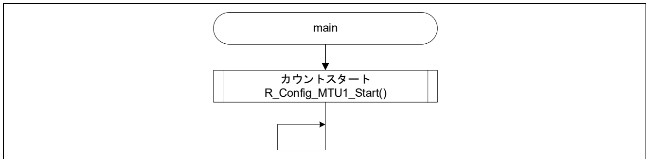
図 3-8 main 関数
