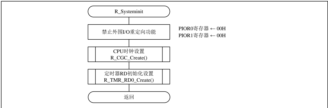
图 4.4 系统函数
