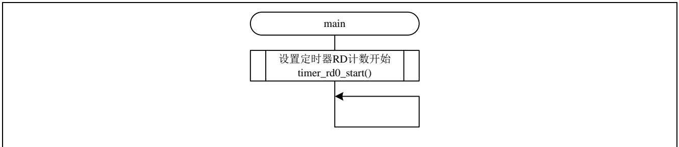
图 4.8 主函数处理
