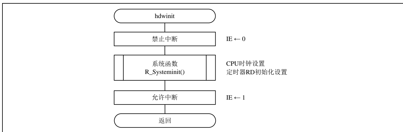
图 4.3 初始化函数
