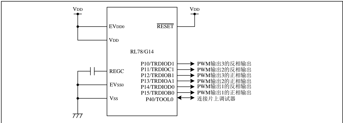
图 3.1 硬件配置
