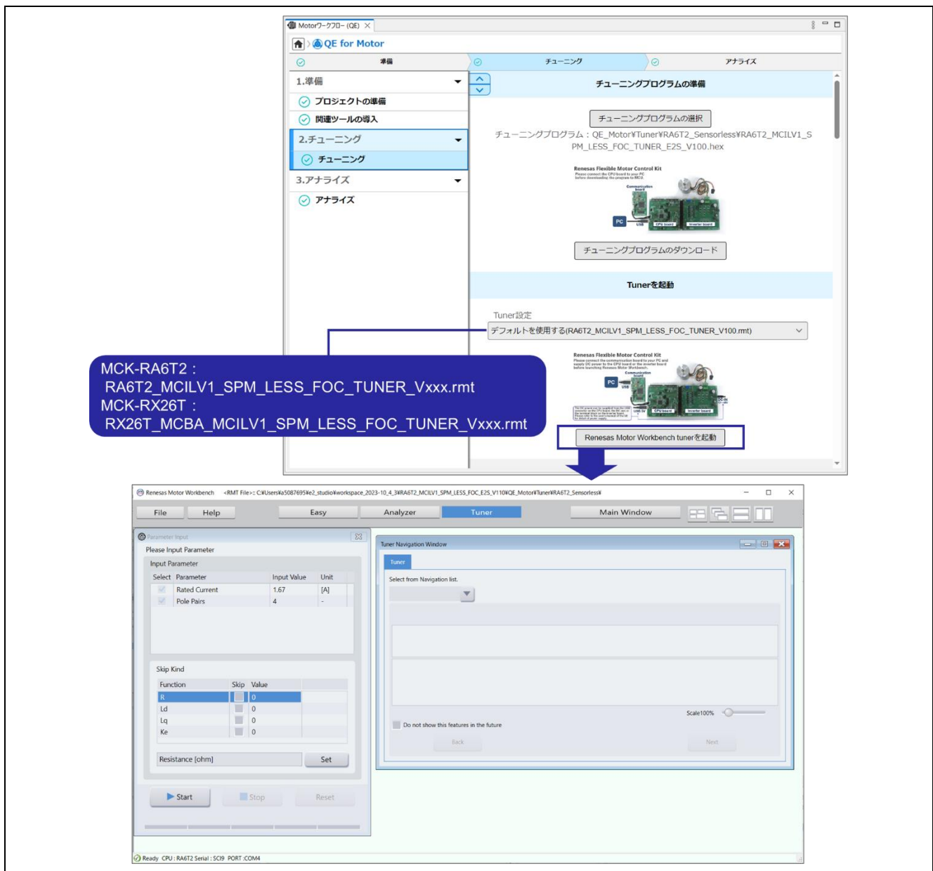
図 4-22 Tuner の起動
