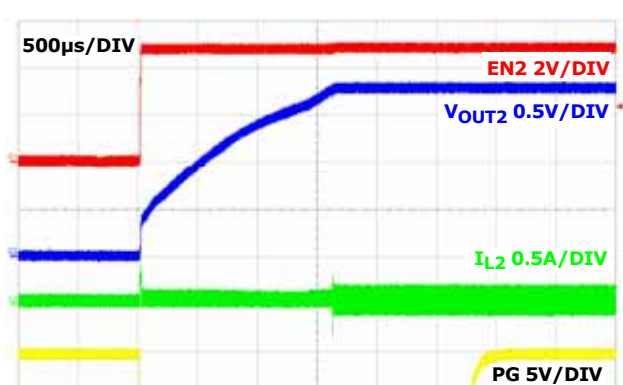
図 25. 無負荷時のソフトスタート、チャンネル 2 (PWM)
