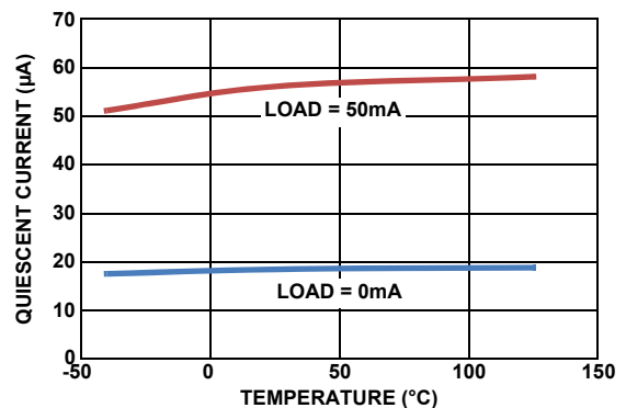
図 2. 自己消費電流 vs 負荷電流 (ユニティゲイン)、 V_{IN} = 14V
