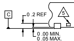
"X"の詳細
