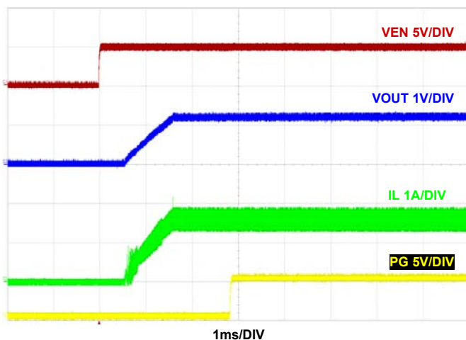
図 31. 1.5A 負荷時のスタートアップ F_{SW} = 2\text{MHz} , V_{IN} = 5\text{V} , MODE = PFM, T_A = +25^\circ\text{C}
