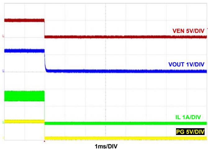
図 32. 1.5A 負荷時のシャットダウン F_{SW} = 2\text{MHz} , V_{IN} = 5\text{V} , MODE = PFM, T_A = +25^\circ\text{C}
