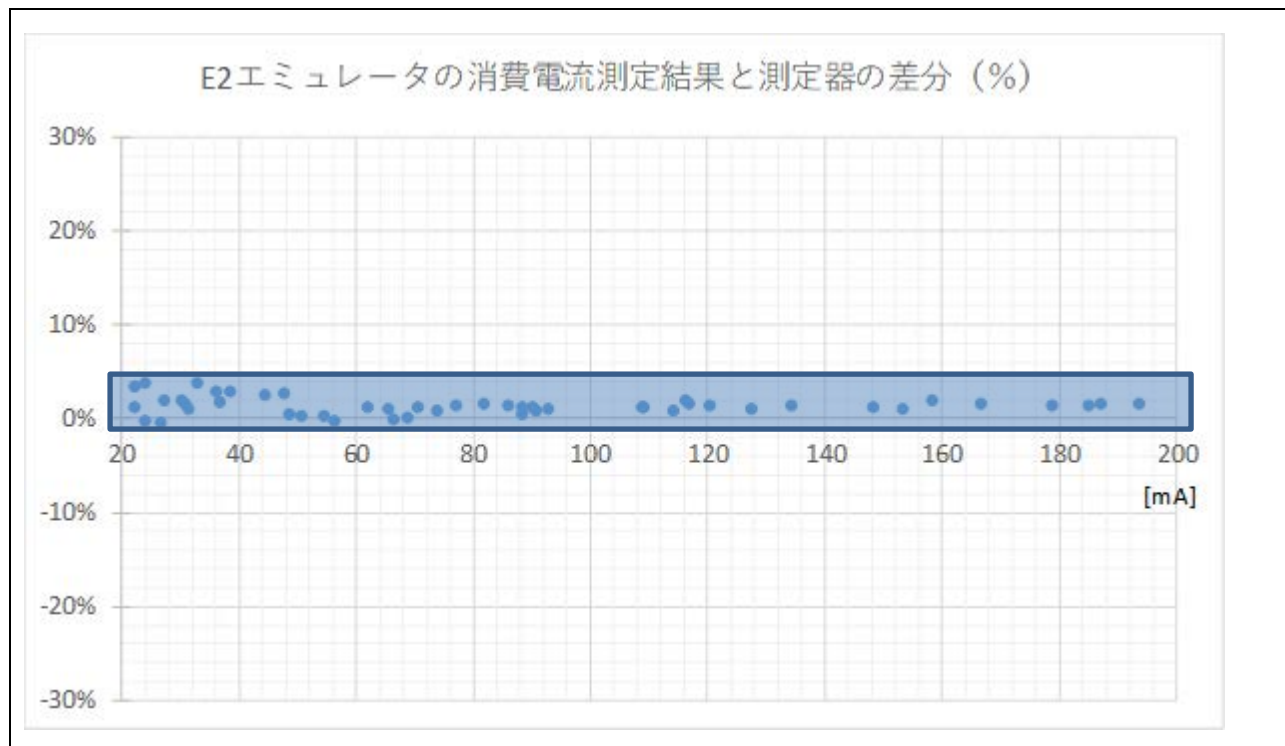
図 5-3 消費電流測定結果と測定器の差分 1
