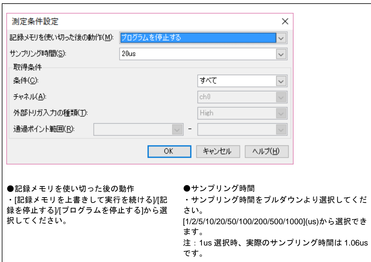
図 4-6 消費電流測定設定 1
