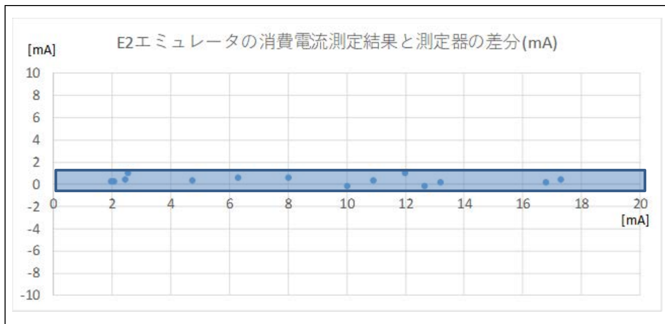
図 5-4 消費電流測定結果と測定器の差分 2
