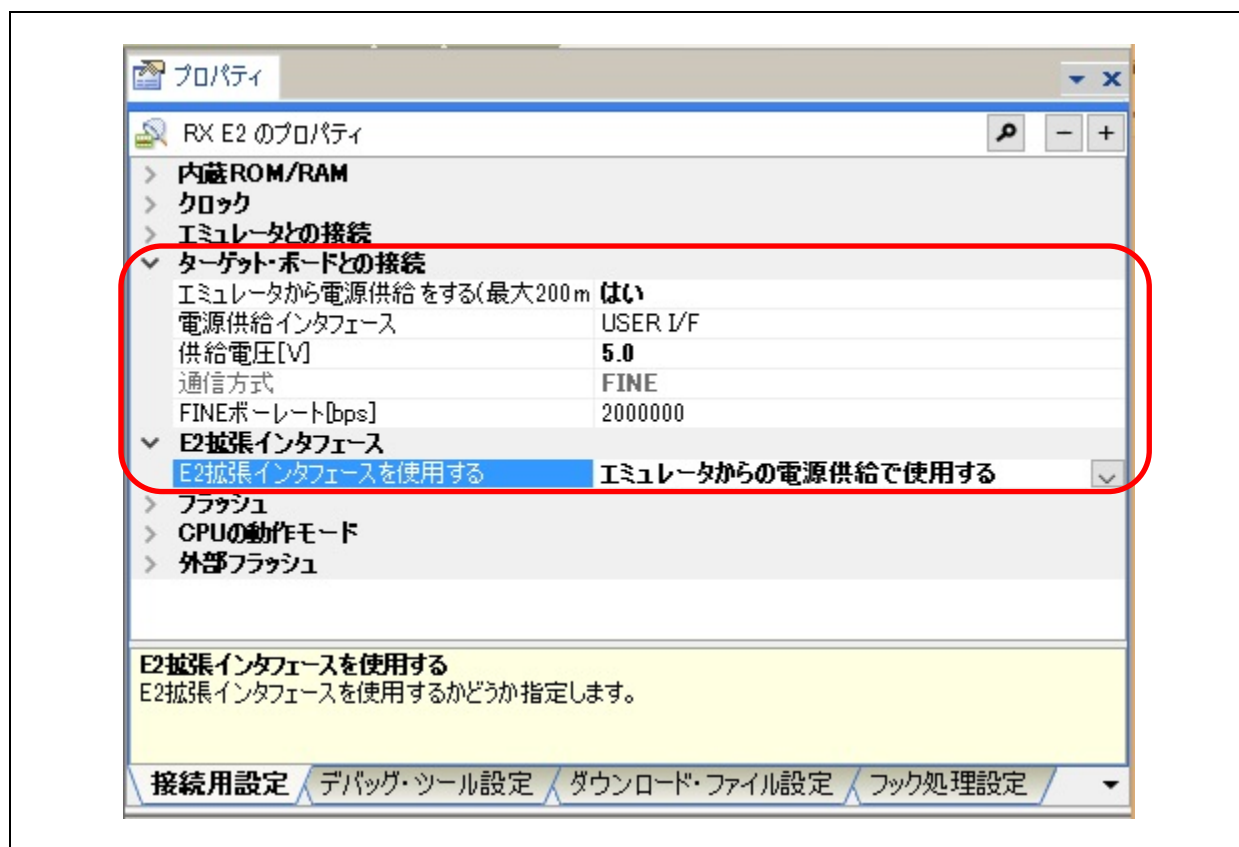
図 4-1 E2 エミュレータデバッガの接続設定
