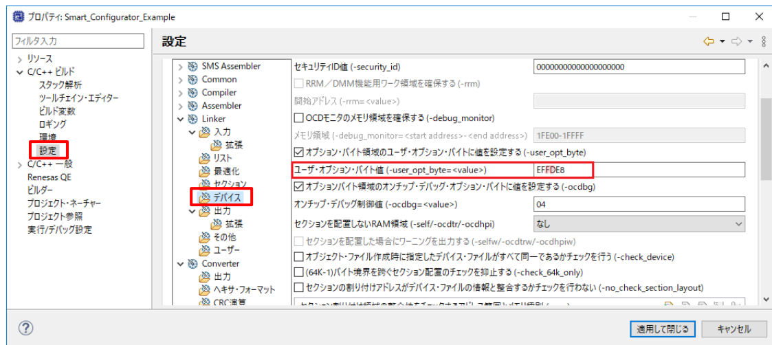
図 3-5 e 2 studio のオプションバイト値 (C1H)
