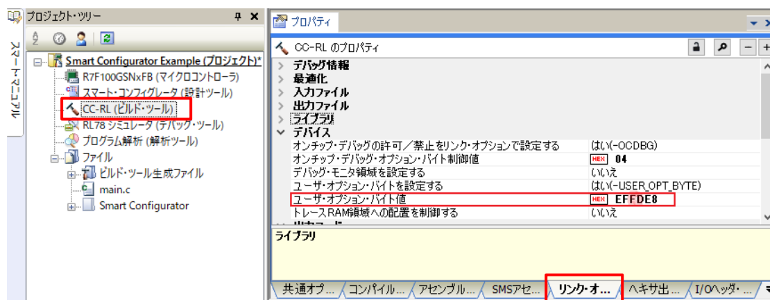
図 3-3 CS+のオプションバイト値 (C1H)
