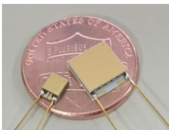
Micro TEG module
