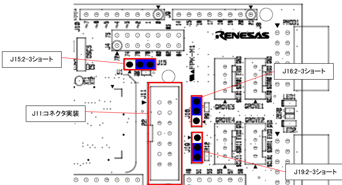
図 5-13 : エミュレータコネクタ使用時設定(部品面)
