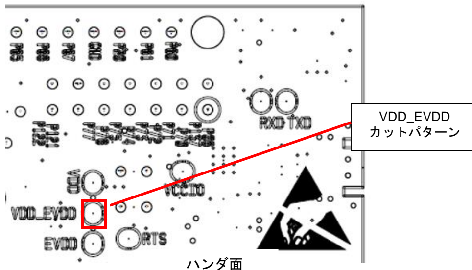
図 5-11 : VDD_EVDD カットパターン位置
