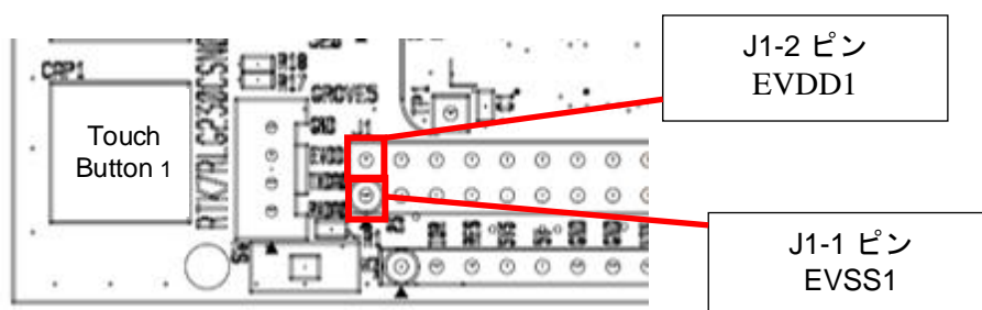
図 5-8: 外部電源供給接続先位置(部品面)
