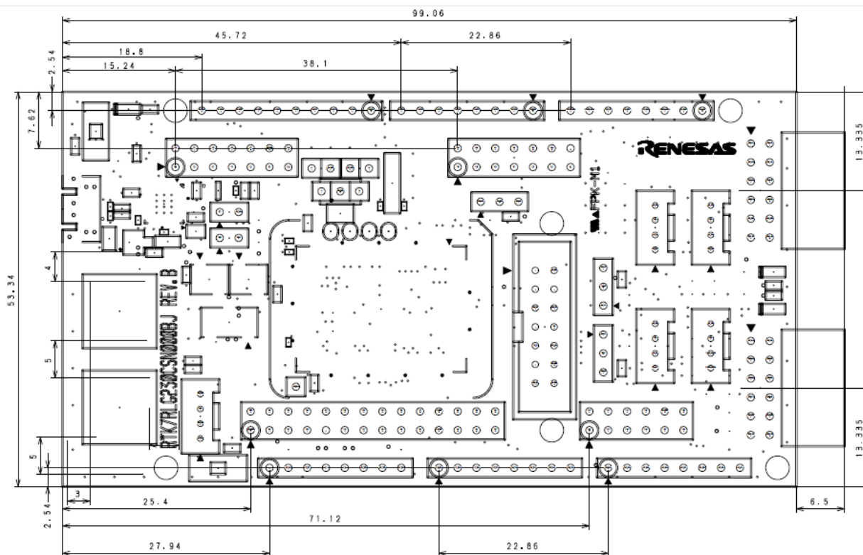
図 3-2: 寸法図
