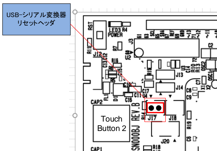
図 5-4: USB-シリアル変換器リセットヘッダ位置(部品面)
