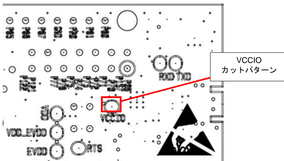
図 5-12 : VCCIO カットパターン位置
