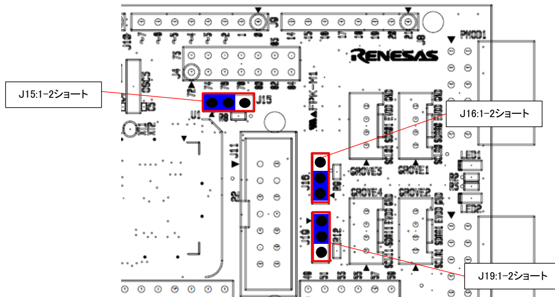
図 5-15 : COM port デバッグ使用時設定(部品面)
