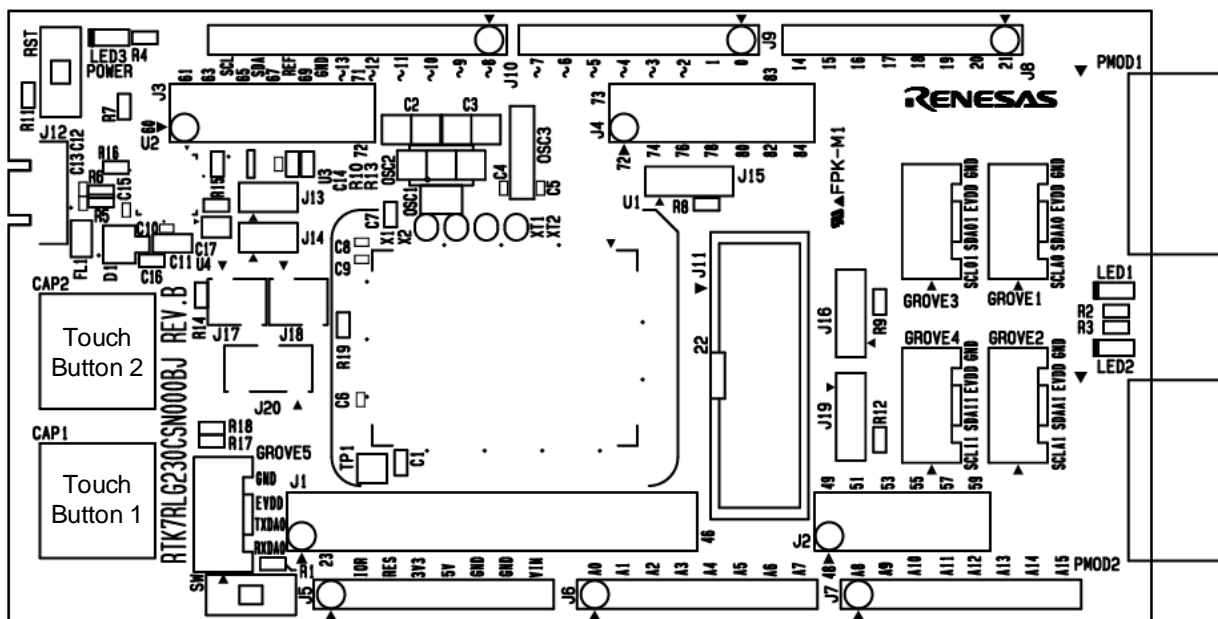
図 3-1: 部品配置図
