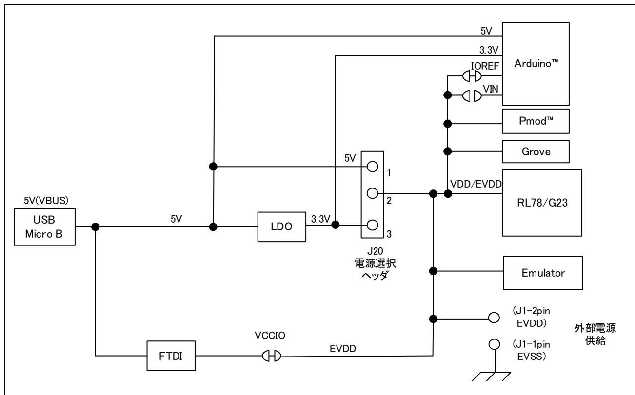
図 6-1 電源回路ブロック図
