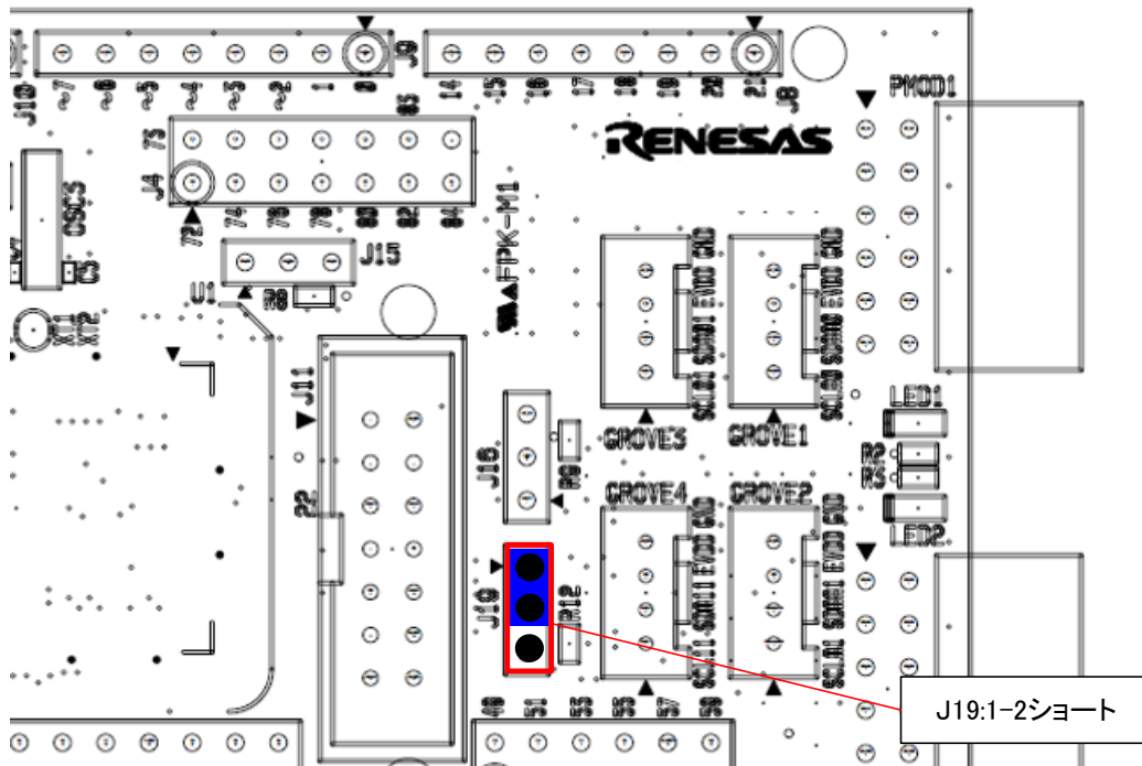
図 6-4 : COM port デバッグ使用時設定(部品面)
