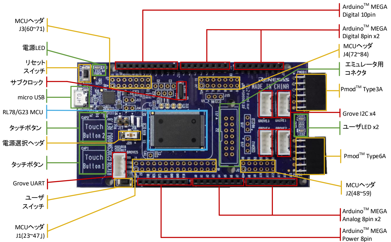
図 2-1: 部品面外観図
