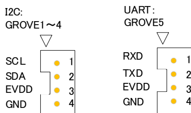
図 5-3 Grove コネクタピン配置
