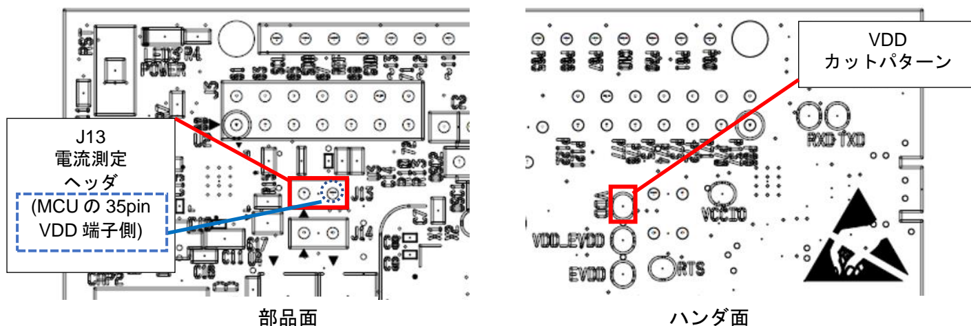
図 5-9 : J13 電流測定ヘッダ及び VDD カットパターン位置
