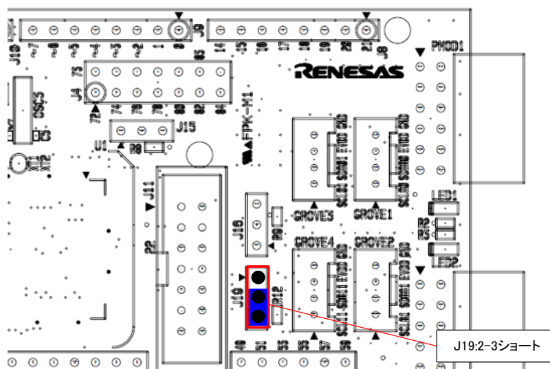
図 6-3 : QE のシリアル接続機能を実行する場合の設定(部品面)
