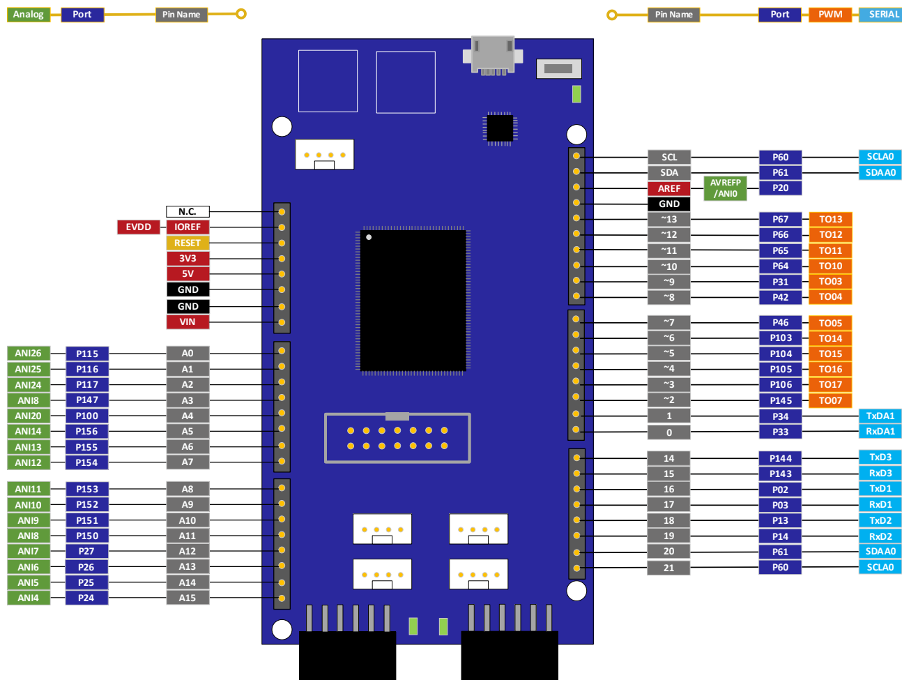
図 5-1: Arduino™ コネクタピン配置
