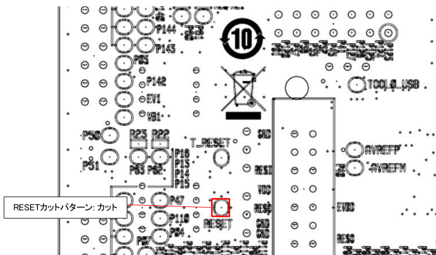
図 6-2 : QE のシリアル接続機能を実行する場合の設定(ハンダ面)
