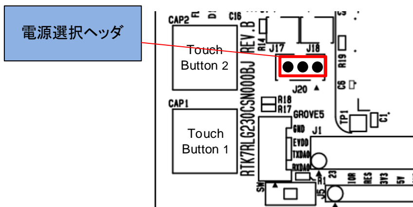
図 5-7: エミュレータ/外部電源使用時のヘッド設定(部品面)
