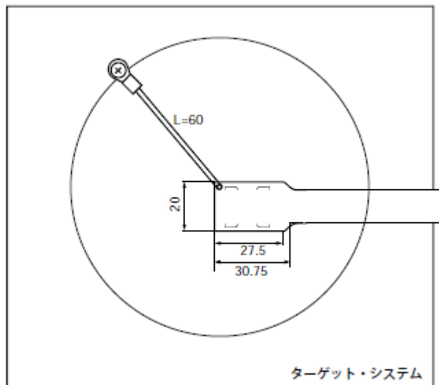
図2-6 GND線接続可能箇所
