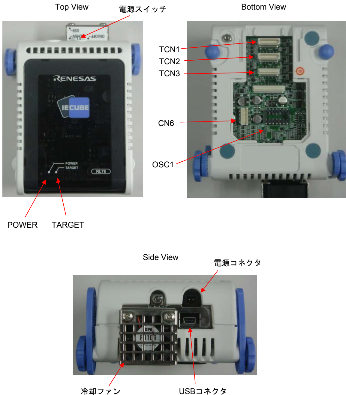
図1-1 QB-RL78F12の各部の名称
