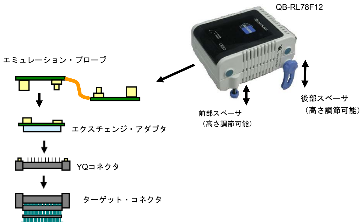
図2-7 エミュレーション・プローブを使用する場合の接続
