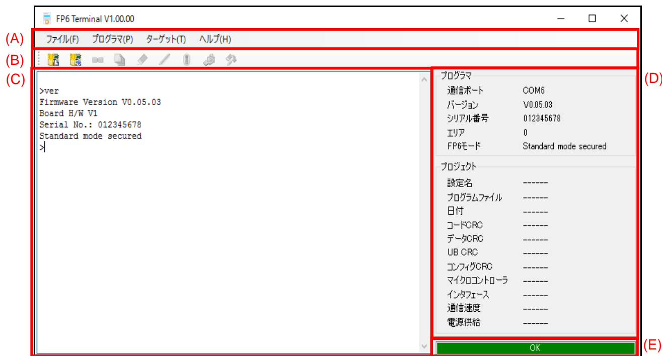
図 4.1 メインウィンドウ
