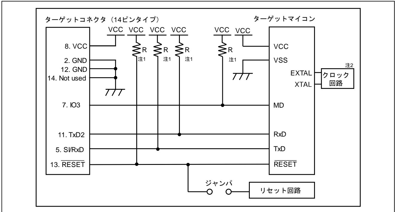
図 9.17 UART の回路例 (S7G2 の回路例)
