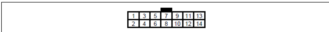
図 8.12 ターゲットケーブル（14ピンタイプ）14ピン2.54mmピッチ汎用コネクタ（メス）概要（ソケット側から見た図）
