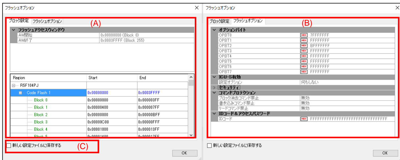
図 4.17 [フラッシュオプション]ダイアログボックス
