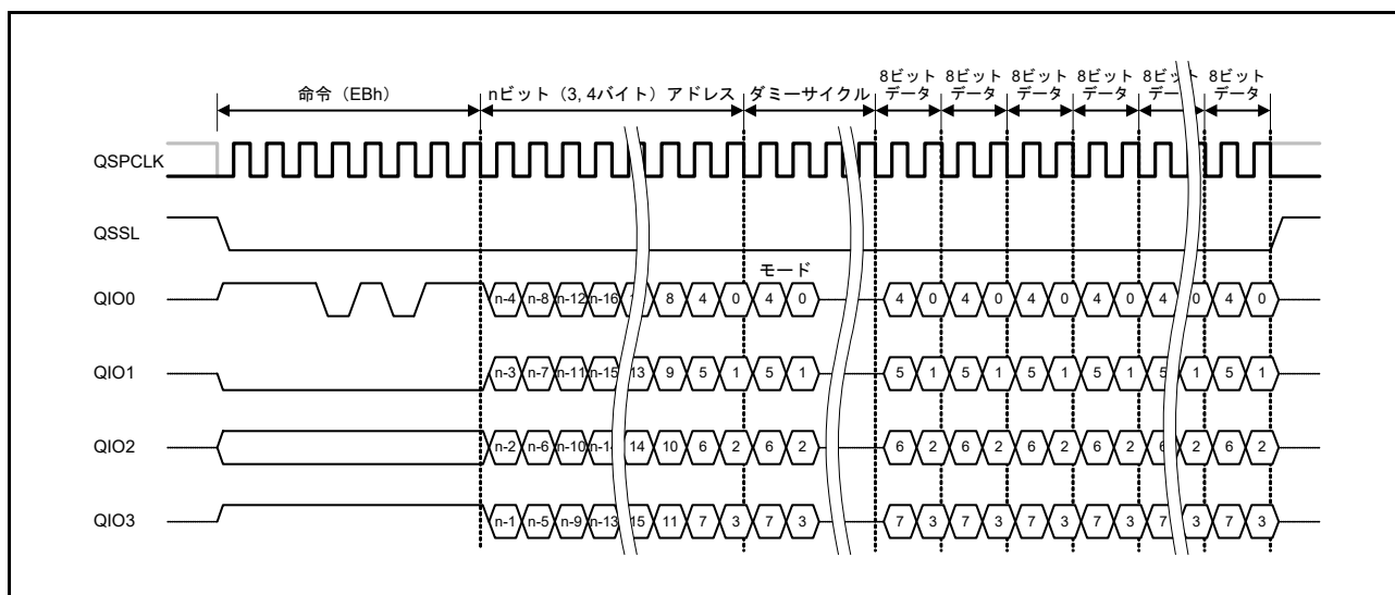
図 35.24 ファストリード Quad I/O バスサイクル
