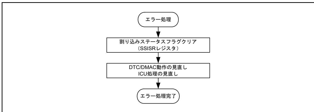
図 37.56 エラー処理手順
