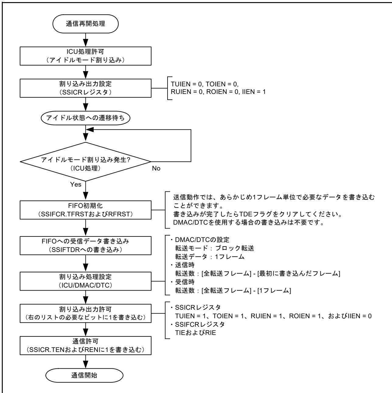
図 37.57 通信再開手順 (CPU 動作手順)
