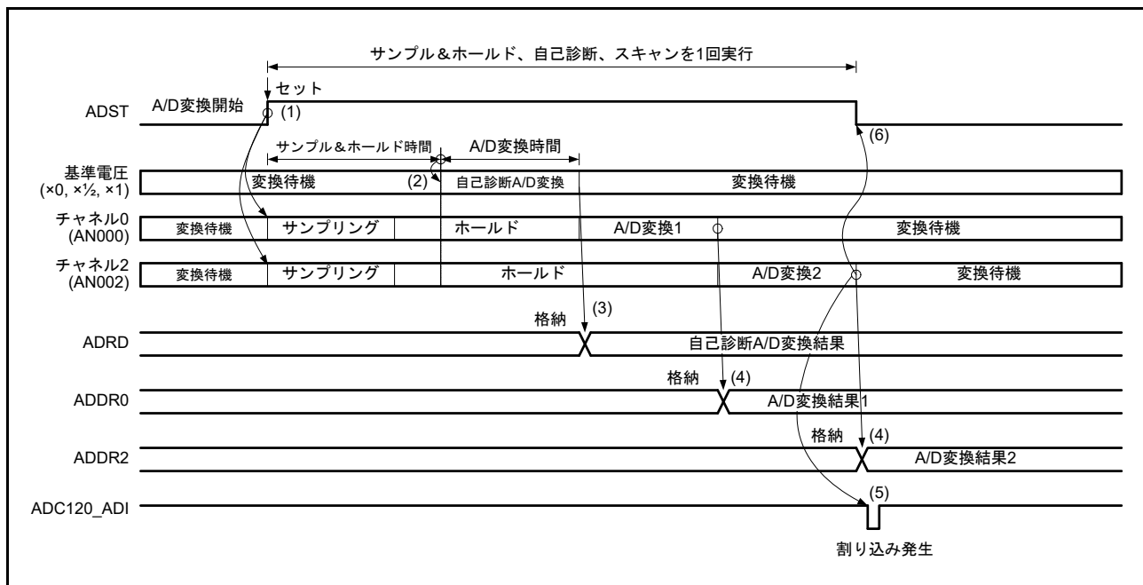
図 42.11 シングルスキャンモードの動作例 (チャンネル専用サンプル&ホールド回路使用、AN000 および AN002 選択 + 自己診断、常時サンプリング無効)
