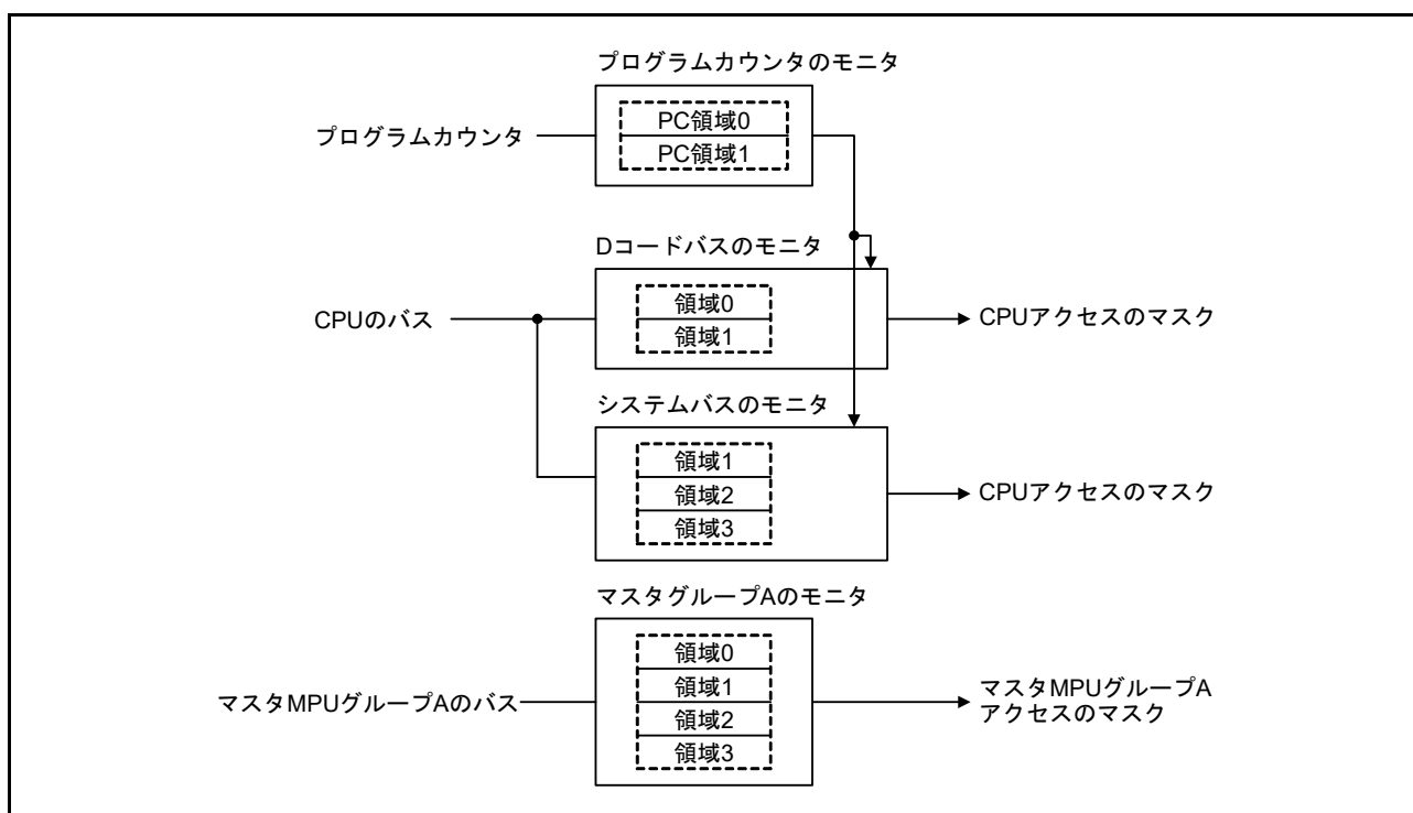
図 16.10 セキュリティ MPU のブロック図
