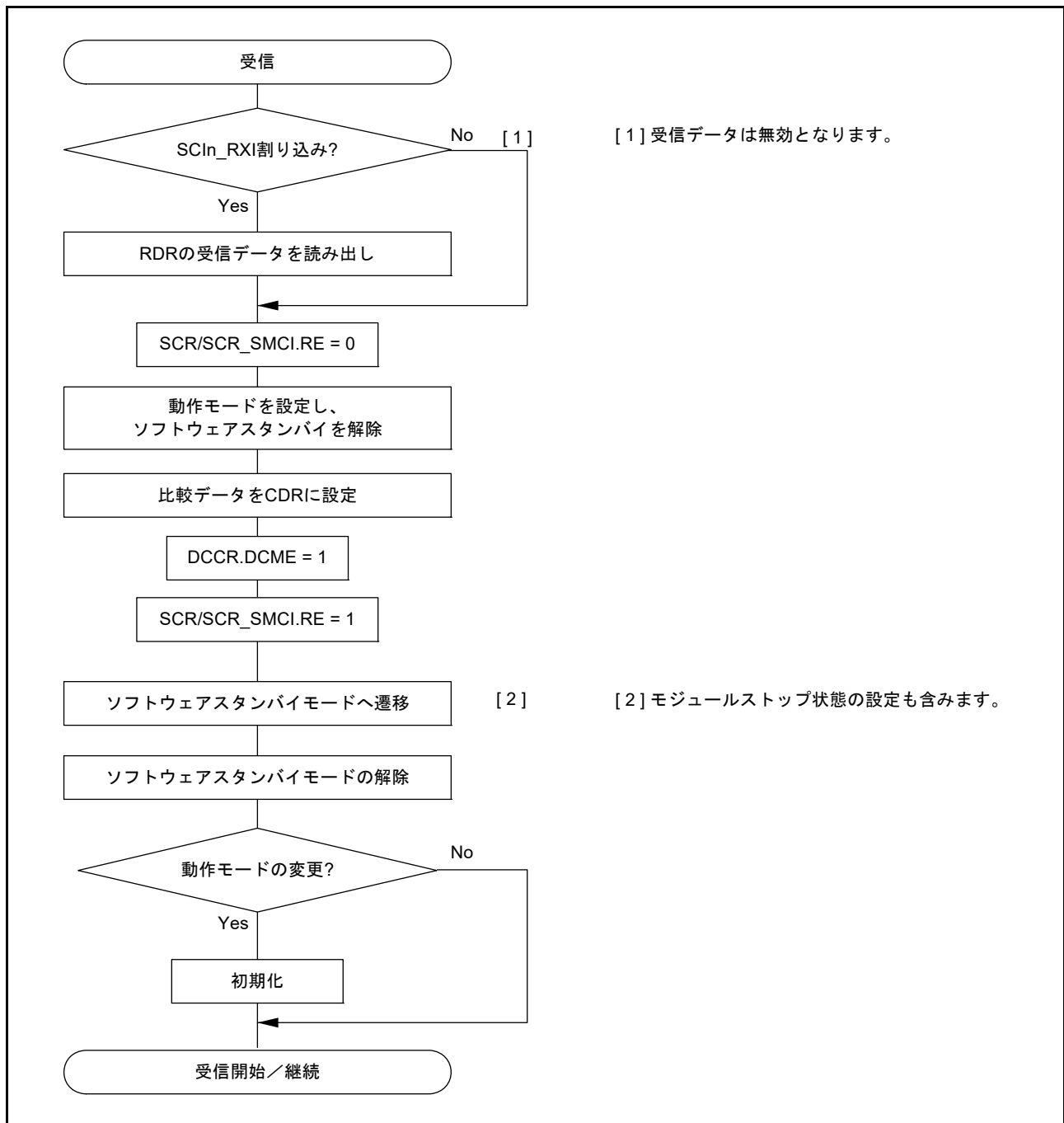
図 30.77 アドレス一致を用いて受信中にソフトウェアスタンバイモードへ遷移する場合のフローチャート例
