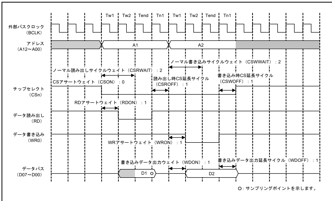
図 15.7 ノーマルアクセスの動作例（読み出し／書き込み）（ n = 0, 1, 4 \sim 7 ）
