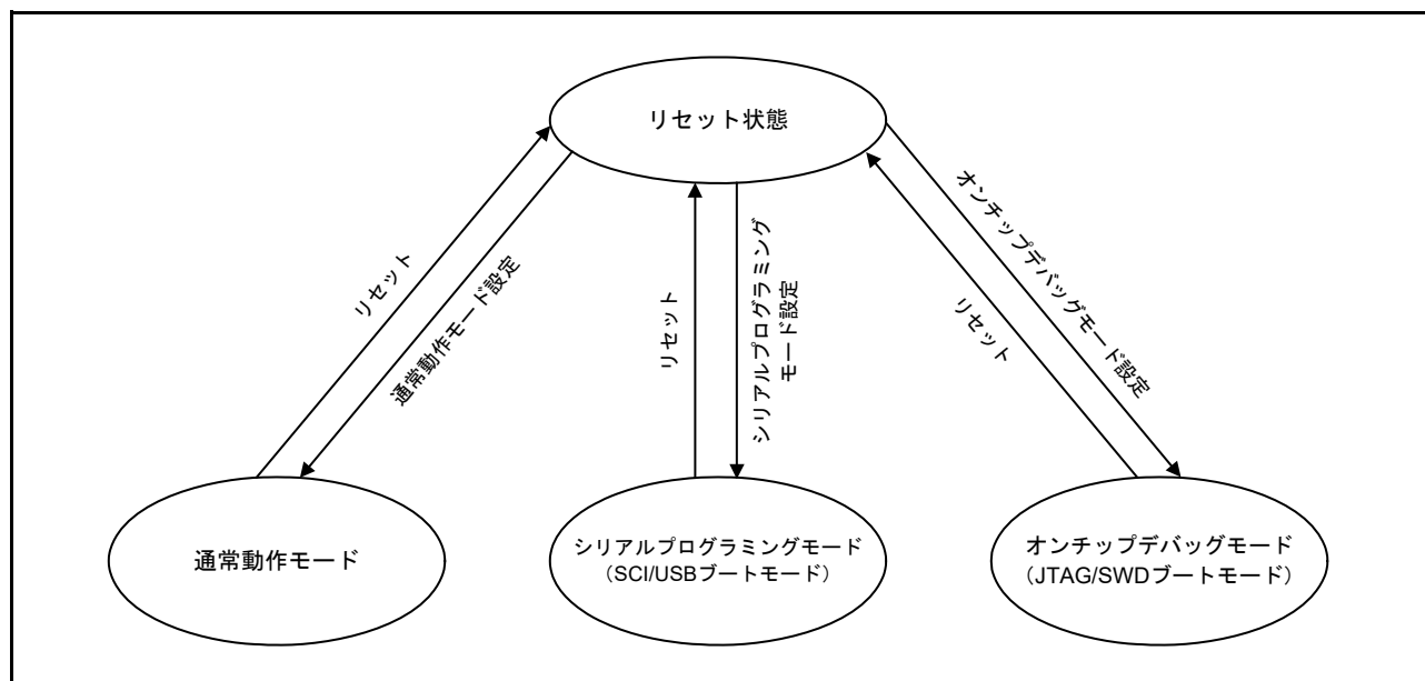
図 50.5 フラッシュメモリに関するモード遷移図
