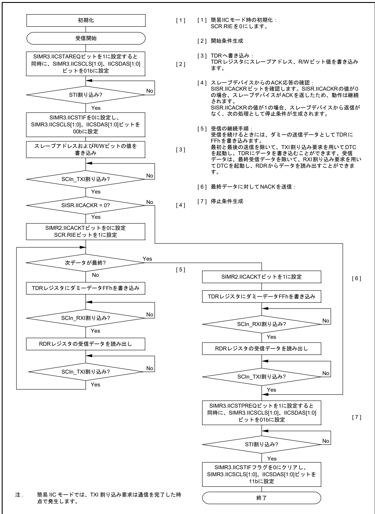
図 30.68 簡易 IIC モードにおけるマスタ受信のフローチャート例 (送信割り込み、受信割り込み使用時)
