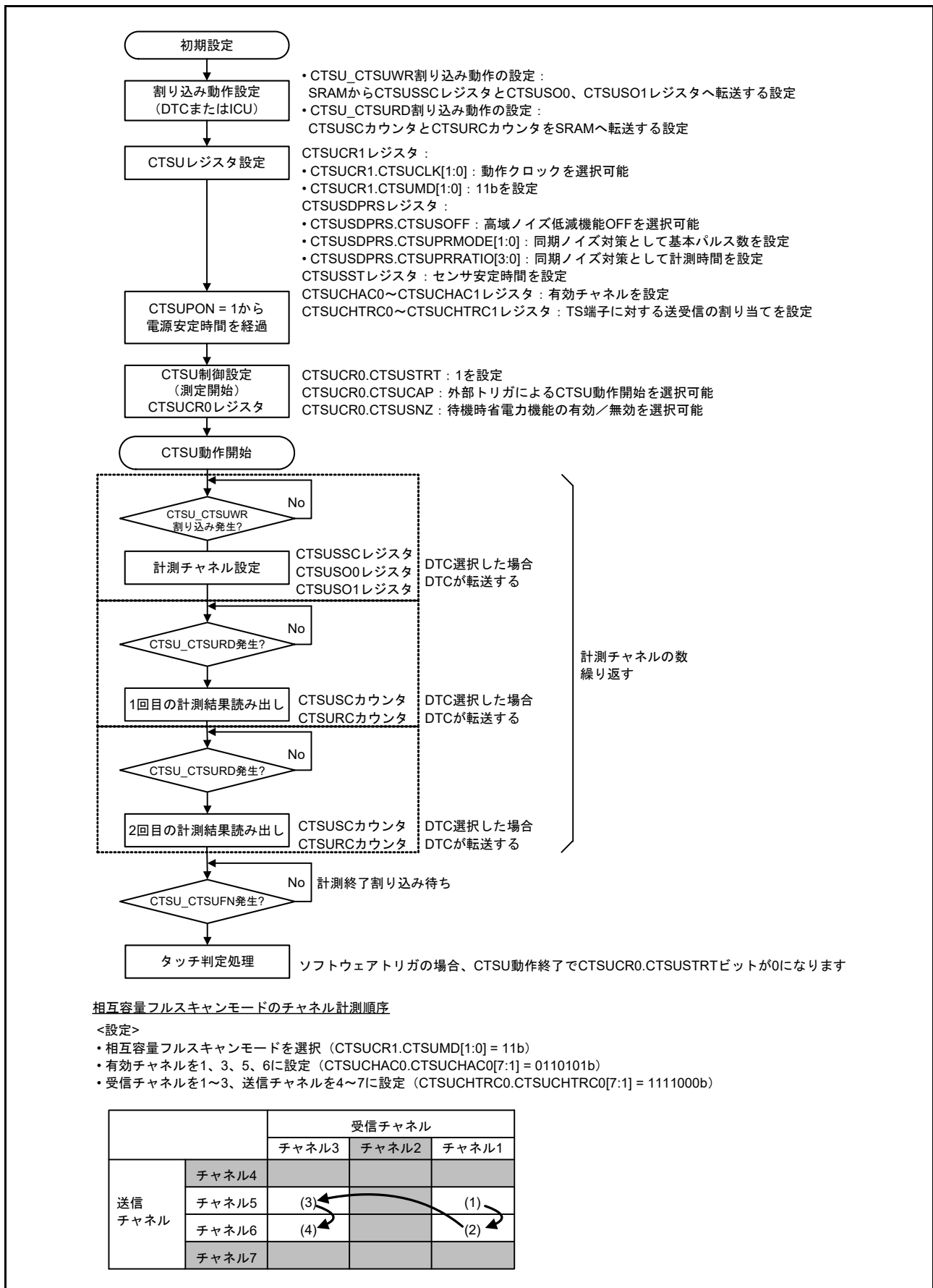
図 46.16 相互容量フルスキャンモードのソフトウェアフローと動作例
