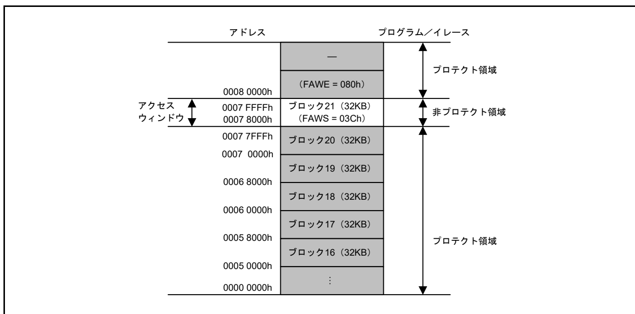
図 50.11 アクセスウィンドウに最終ブロックのみ含まれる場合のアクセスウィンドウの開始ブロックアドレス (FAWS) と終了ブロックアドレス (FAWE)
