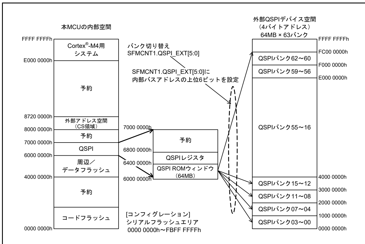
図 35.2 デフォルト領域設定および AHB 空間メモリマップ
