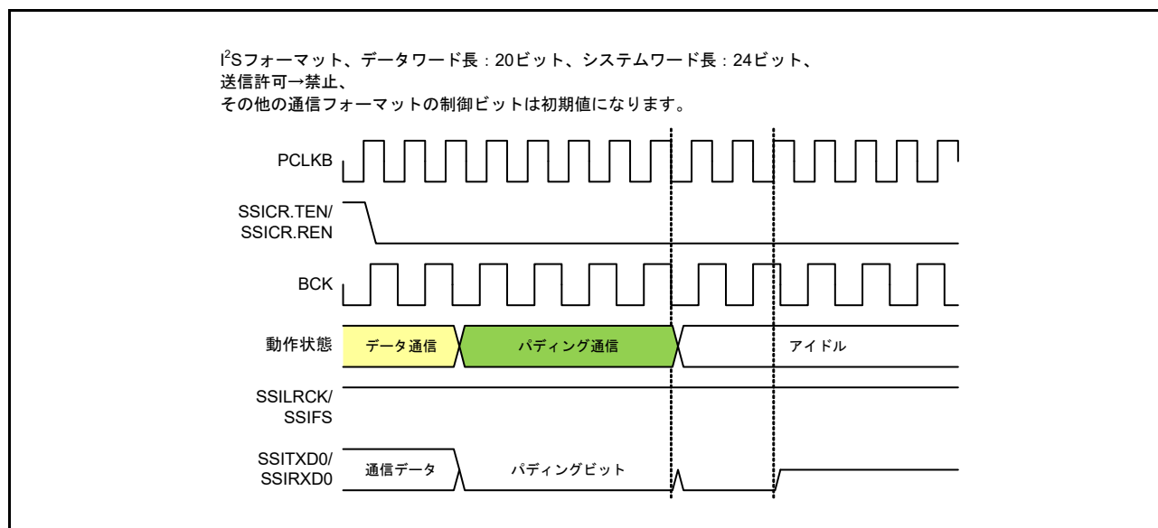
図 37.50 パディング通信からの停止
