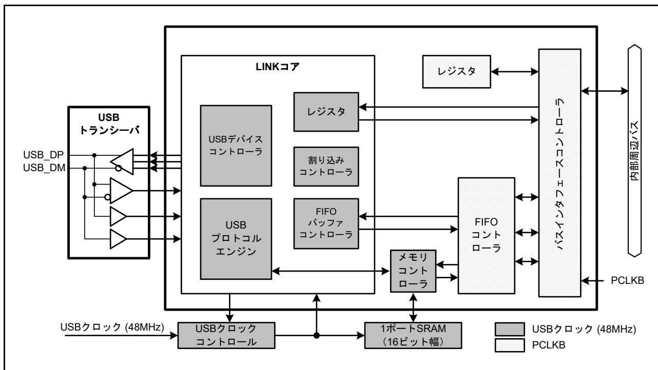
図 29.1 USBFS のブロック図
