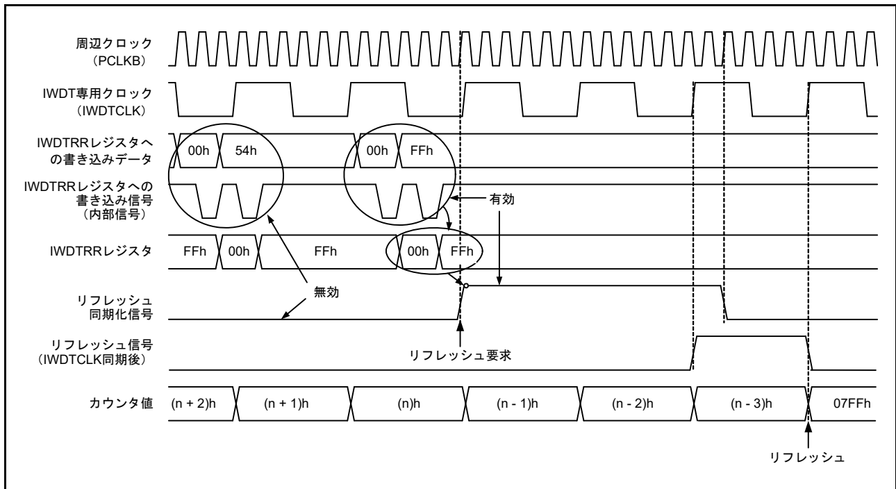
図 28.4 IWDT リフレッシュ動作波形 (OFS0.IWDTCK[3:0] = 0000b、OFS0.IWDTTOPS[1:0] = 11b の場合)
