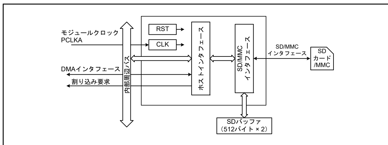
図 39.1 SD/MMC ホストインタフェースのブロック図
