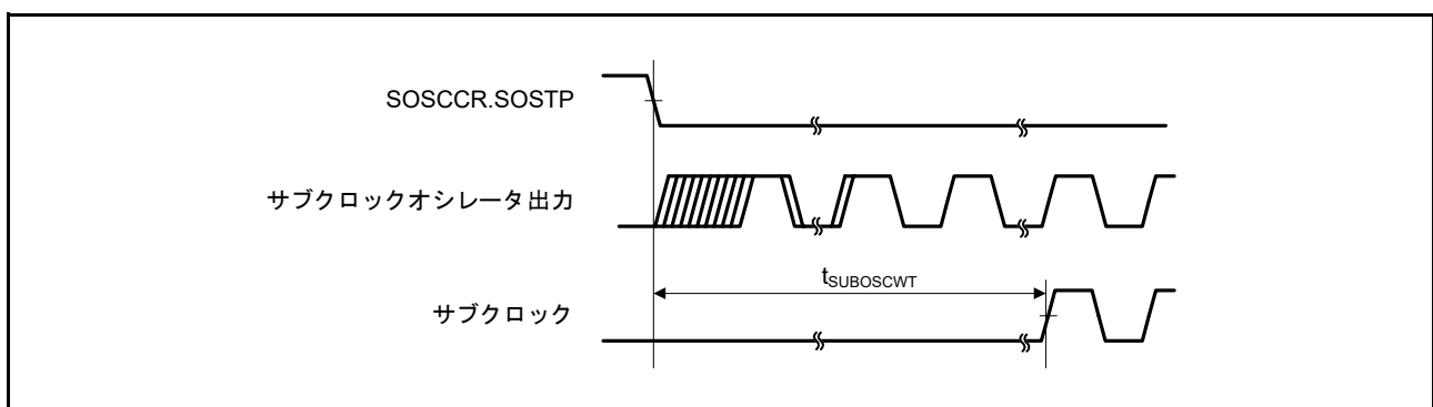
図 52.12 サブクロック発振開始タイミング
