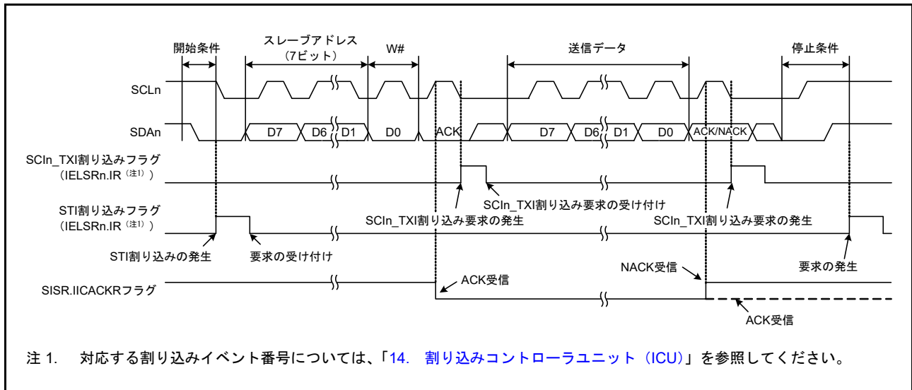
図 30.64 簡易 IIC モードにおけるマスタ送信の動作例 1 (7 ビットスレーブアドレス、送信割り込み、受信割り込み使用時)
