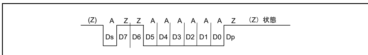
図 30.48 インバースコンベンション (SCMR.SDIR ビット = 1、SCMR.SINV ビット = 1、SMR_SMCI.PM ビット = 1)
