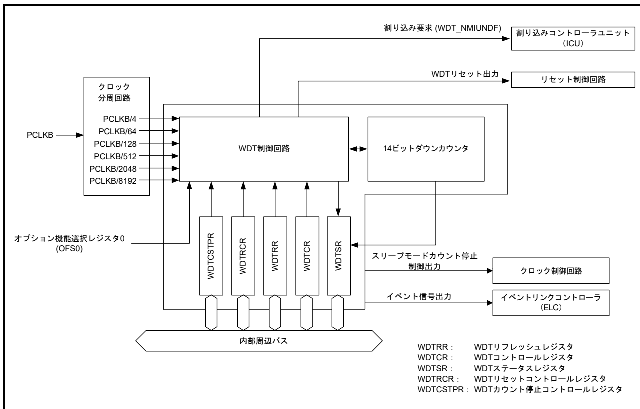
図 27.1 WDT のブロック図
