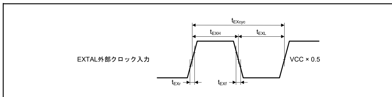
図 52.8 EXTAL 外部クロック入カタイミング
