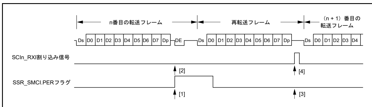
図 30.55 SCI 受信モードでの再転送動作
