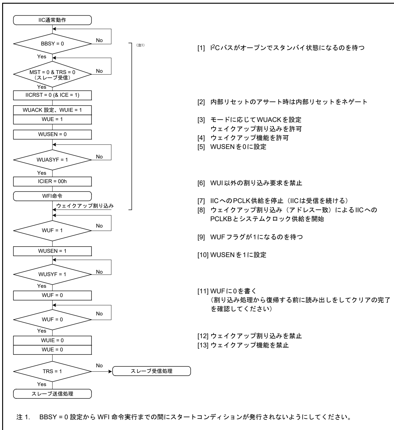
図 32.30 ノーマルウェイクアップモード1の動作例 (スレープアドレス一致時のウェイクアップ割り込みによるウェイクアップの場合)
