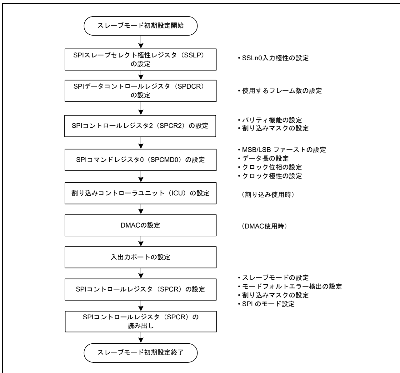
図 34.40 スレーブモード時の SPI 動作の初期化フロー例
