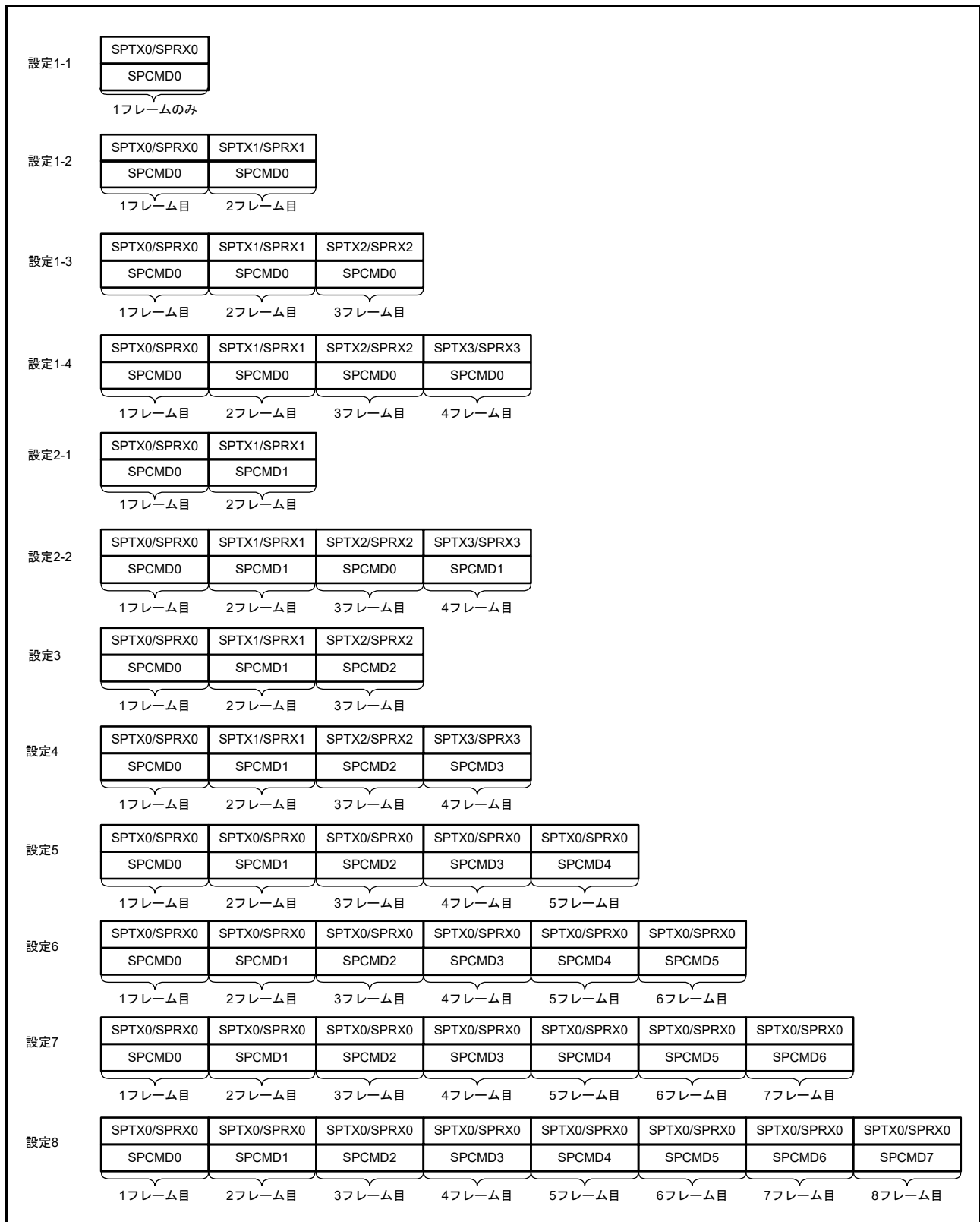
図 34.34 シーケンス動作時の SPI コマンドレジスタと送受信バッファの対応関係
