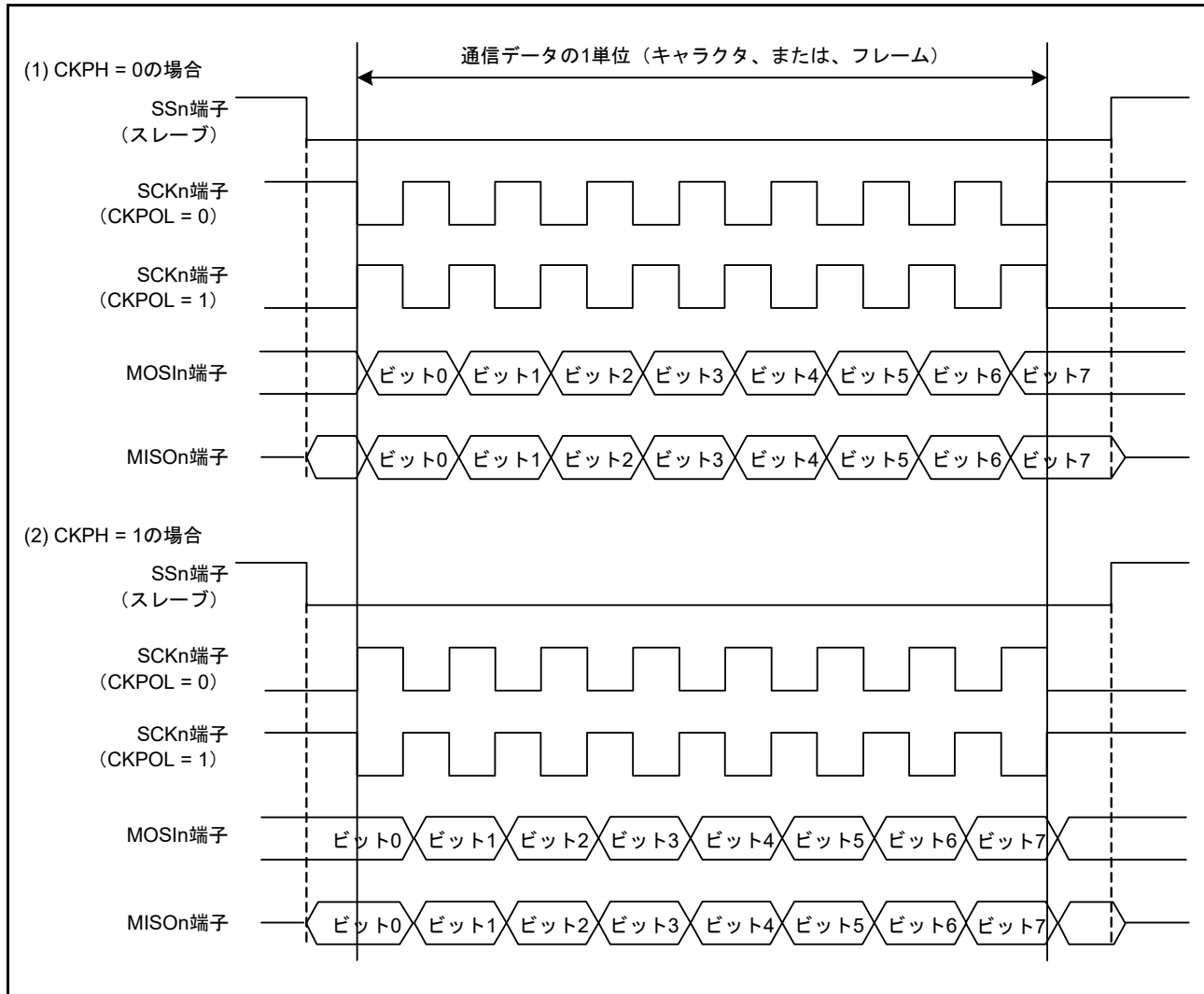
図 30.70 簡易 SPI モードにおけるクロックと送受信データの関係
