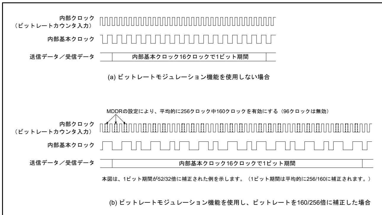
図 30.71 ビットレートモジュレーション機能使用時の内部基本クロックの例
