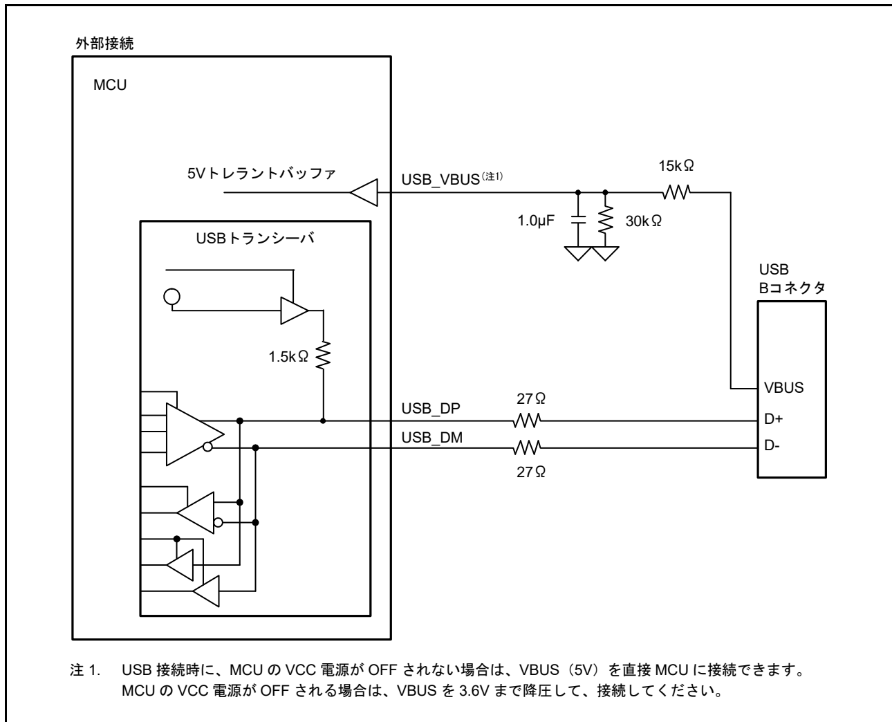
図 29.3 セルフパワー状態でのデバイス接続例
