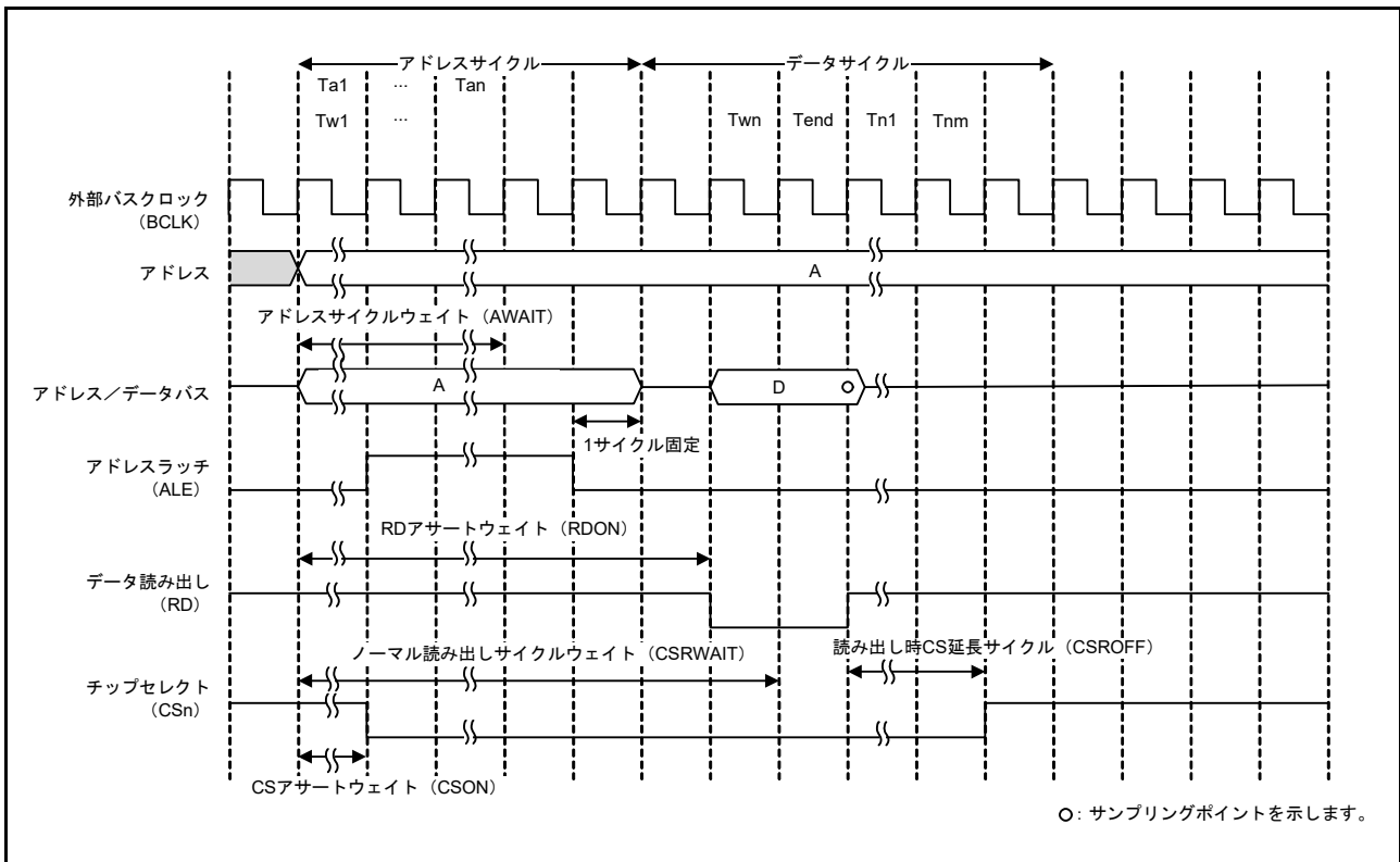
図 15.21 アドレス/データマルチプレクス I/O インタフェース時のリードアクセスの動作例 (n = 0, 1, 4 ~ 7)
