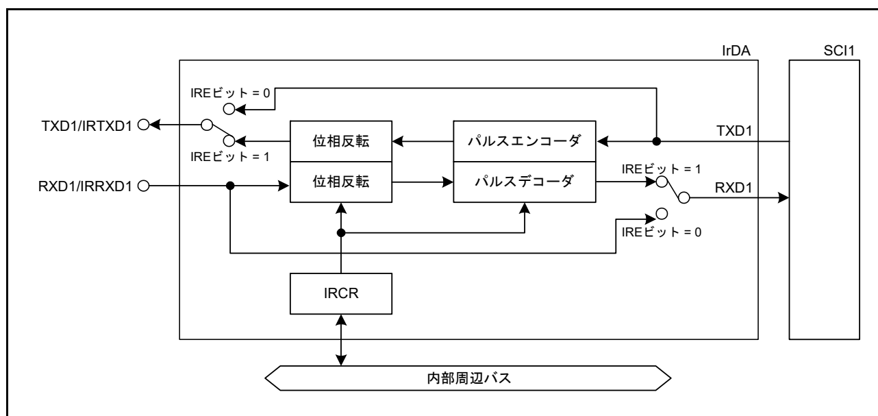
図 31.1 IrDA インタフェースと SCI1 の連携
