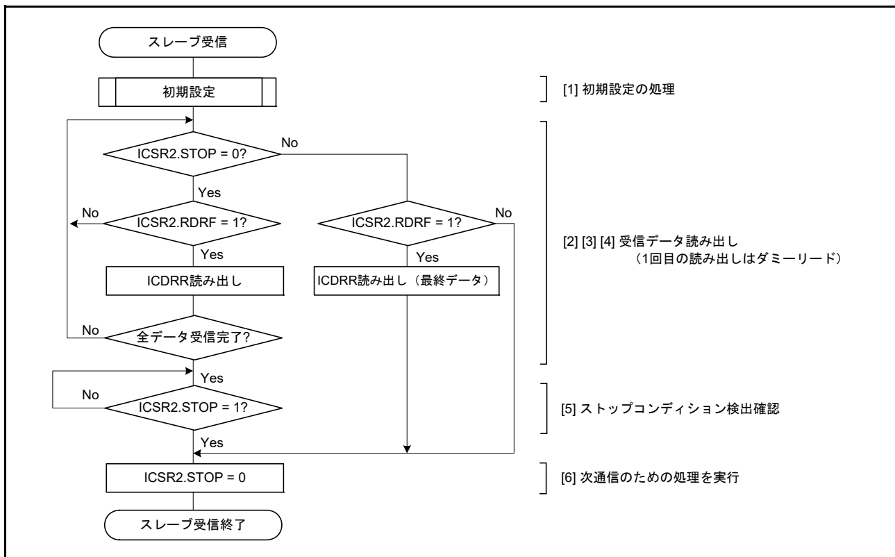
図 32.18 スレーブ受信のフロー例
