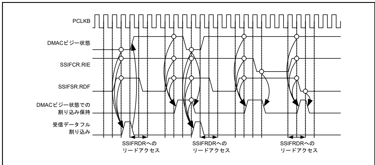
図 37.21 受信データフル割り込みのタイミング
