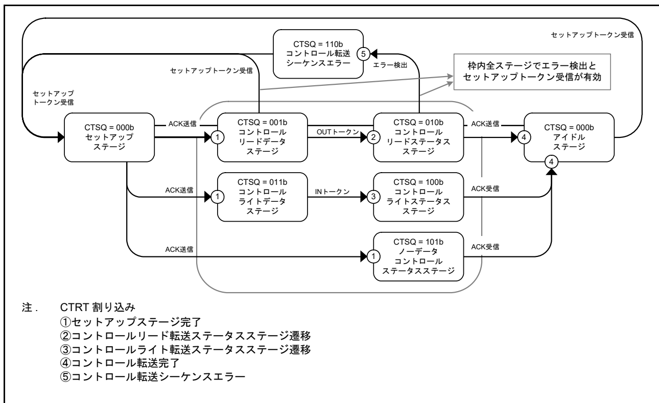
図 29.15 コントロール転送ステージの遷移
