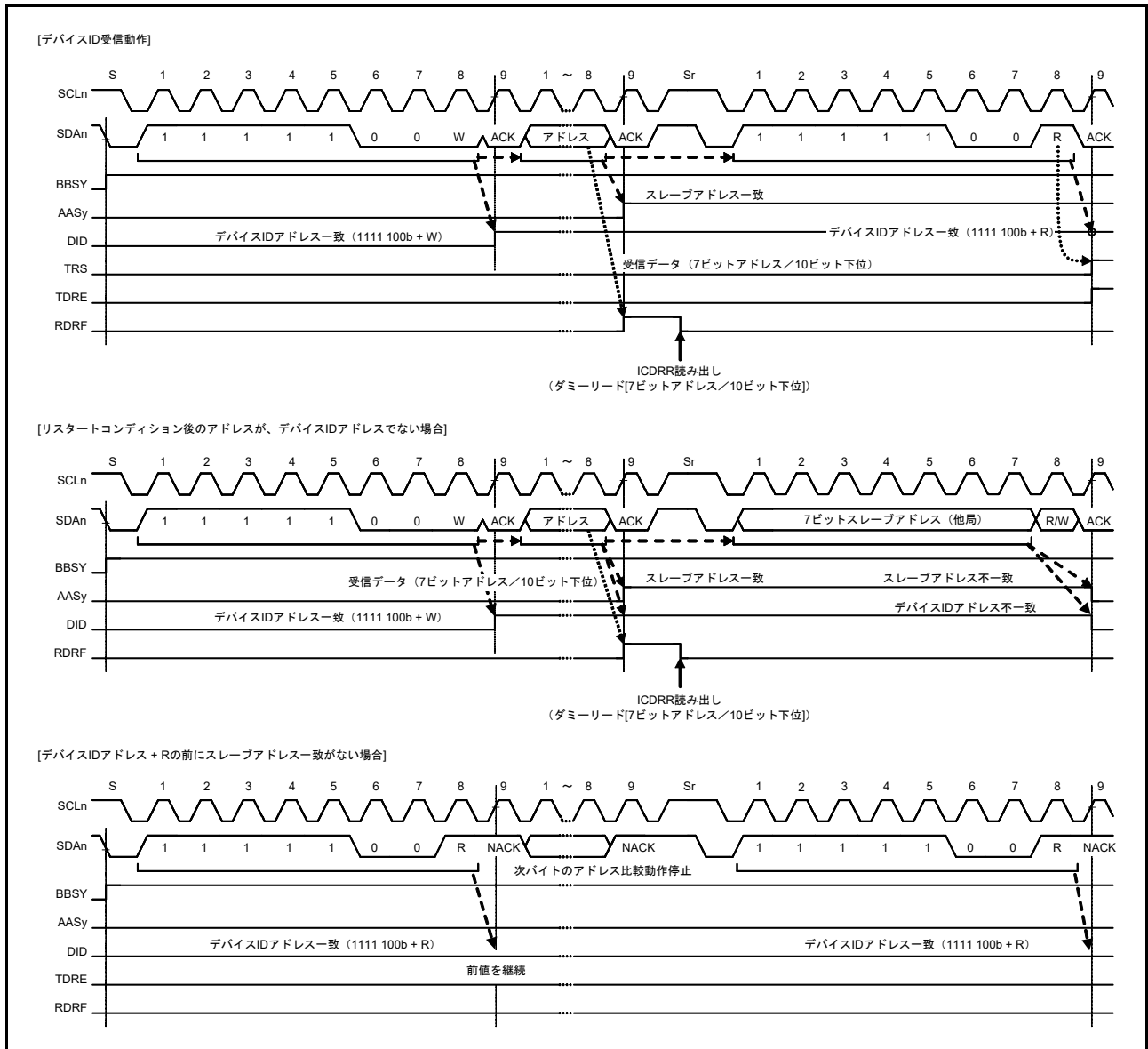
図 32.28 デバイス ID 受信時の AASy および DID フラグのセット/クリアタイミング
