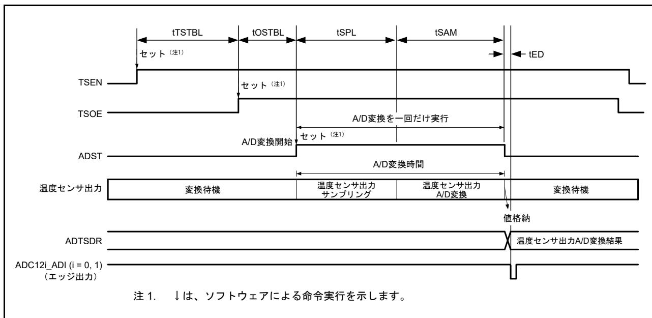
図 44.3 温度センサの動作開始から A/D 変換完了までのタイミング
