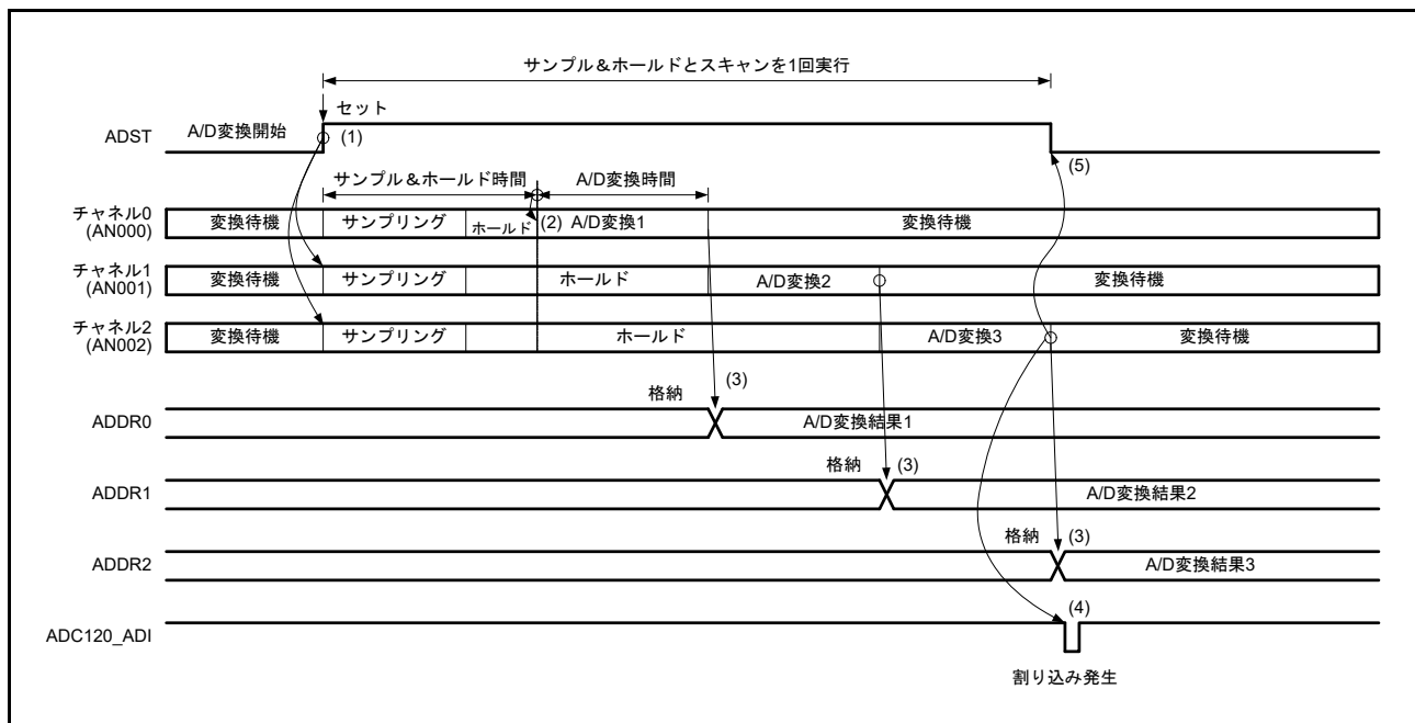
図 42.8 シングルスキャンモードの動作例 (チャンネル専用サンプル&ホールド回路使用、AN000 ~ AN002 選択)
