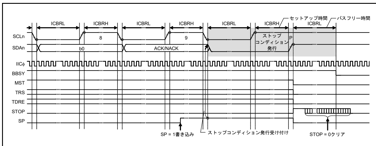
図 32.47 ストップコンディション発行動作タイミング (SP ビットの使用)
