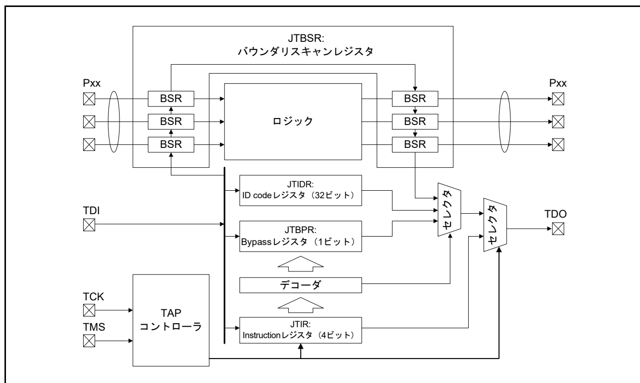
図 40.1 バウンダリスキャン機能のブロック図
