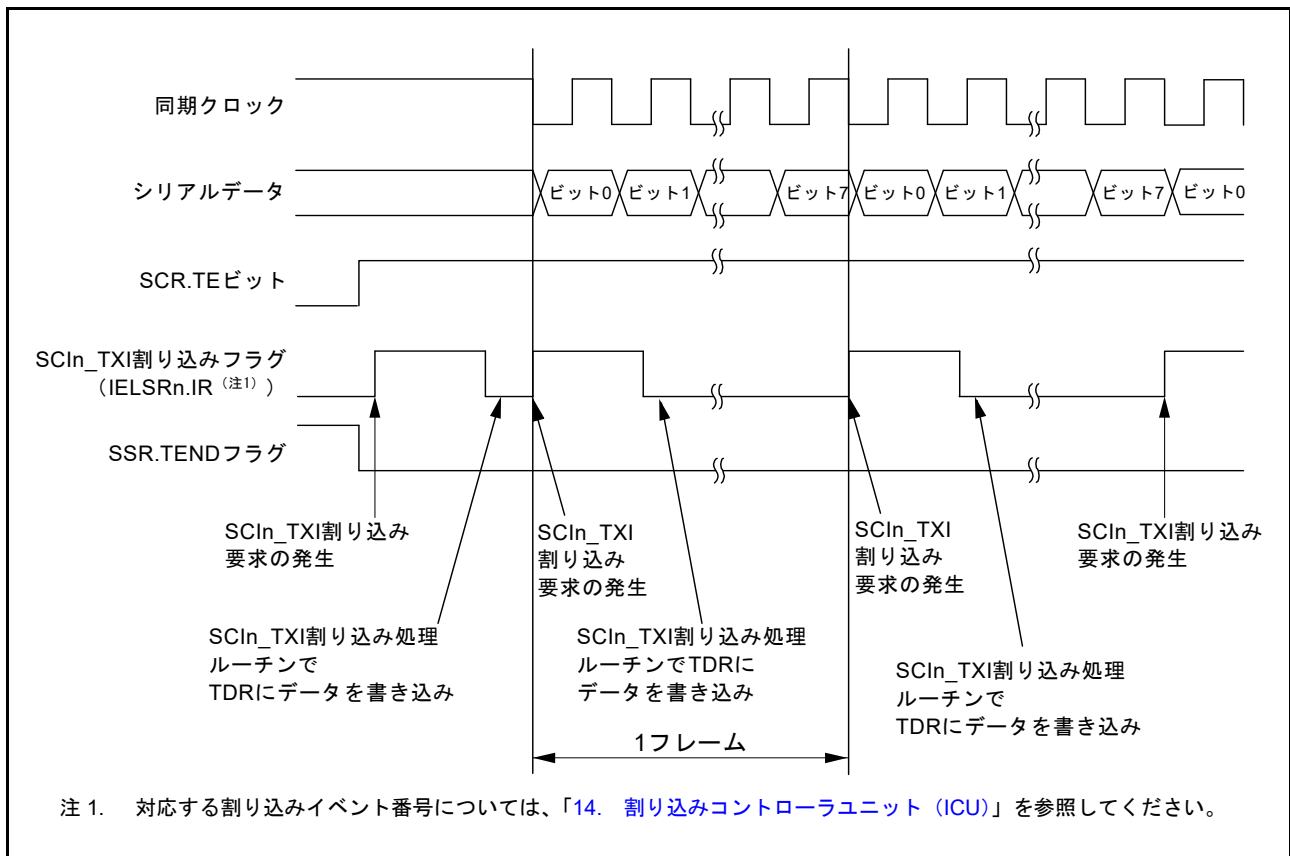
図 30.34 クロック同期式モードにおけるシリアル送信の動作例 (送信開始時に CTS 機能を使用しない場合)
