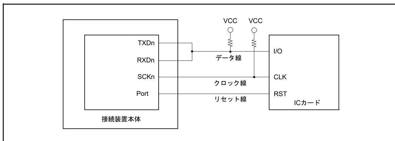
図 30.45 スマートカード (IC カード) との接続例
