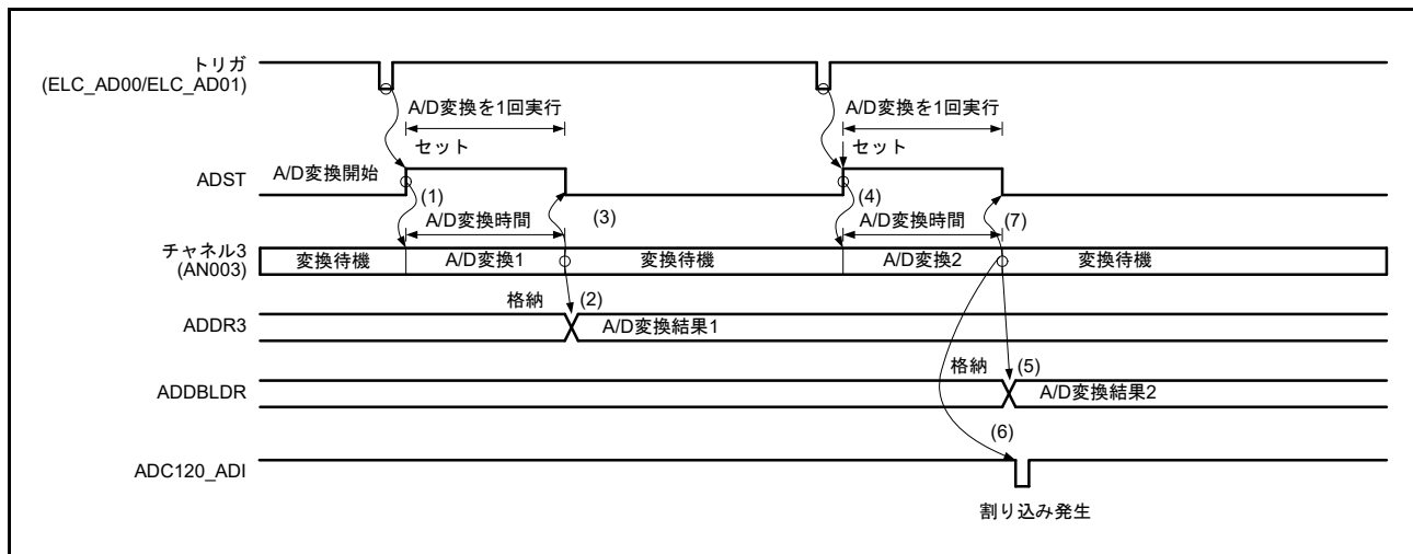
図 42.14 シングルスキャンモードの動作例 (ダブルトリガモード選択、AN003 を 2 重化)
