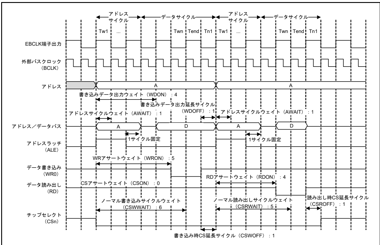
図 15.23 アドレス/データマルチプレクス I/O インタフェース時のバスタイミング例 (n = 0, 1, 4 ~ 7)
