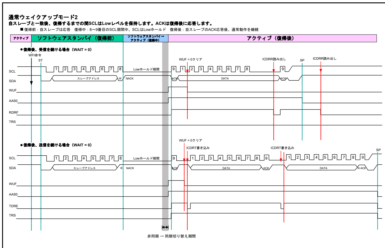
図 32.34 ノーマルウェイクアップモード2のタイミング
