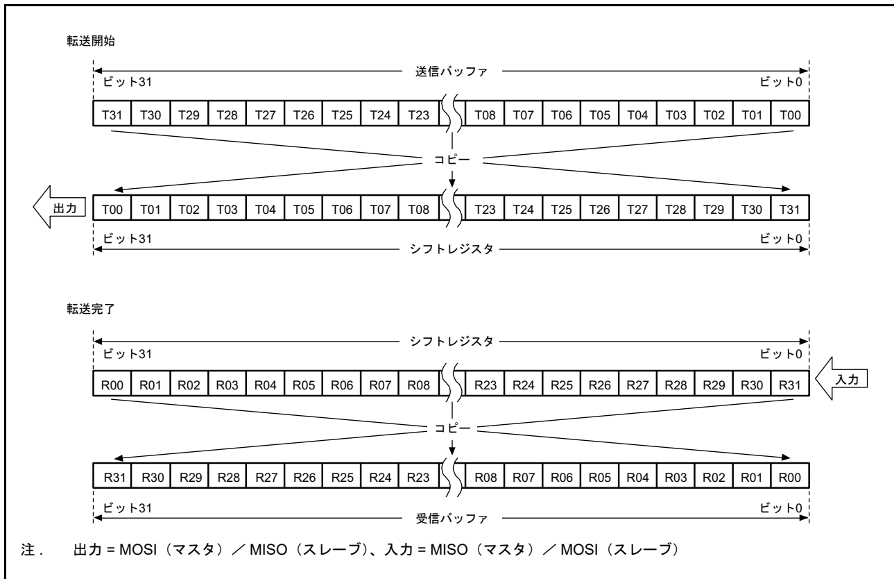
図 34.16 LSB ファースト転送 (32 ビットデータ/パリティ機能無効)
