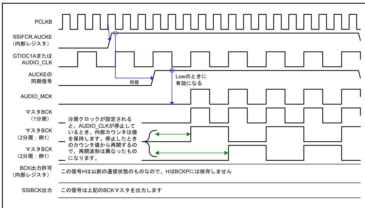
図 37.26 通信停止からマスタモード通信開始までの動作のタイミング図
