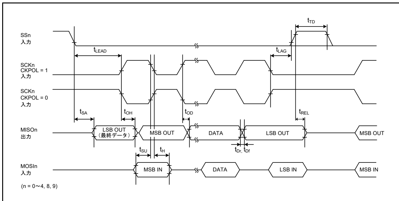
図 52.42 CKPH = 0 の場合におけるスレーブの SCI 簡易 SPI モードタイミング
