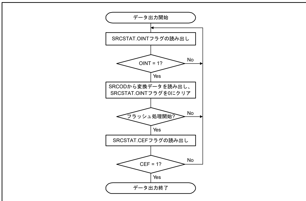
図 38.4 データ出力フロー
