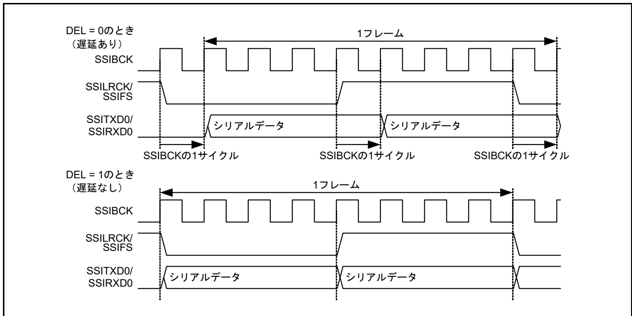
図 37.6 シリアルデータディレイの設定
