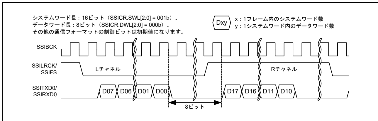
図 37.35 パディングビットの転送例 (I 2 S フォーマット、システムワード長>データワード長)
