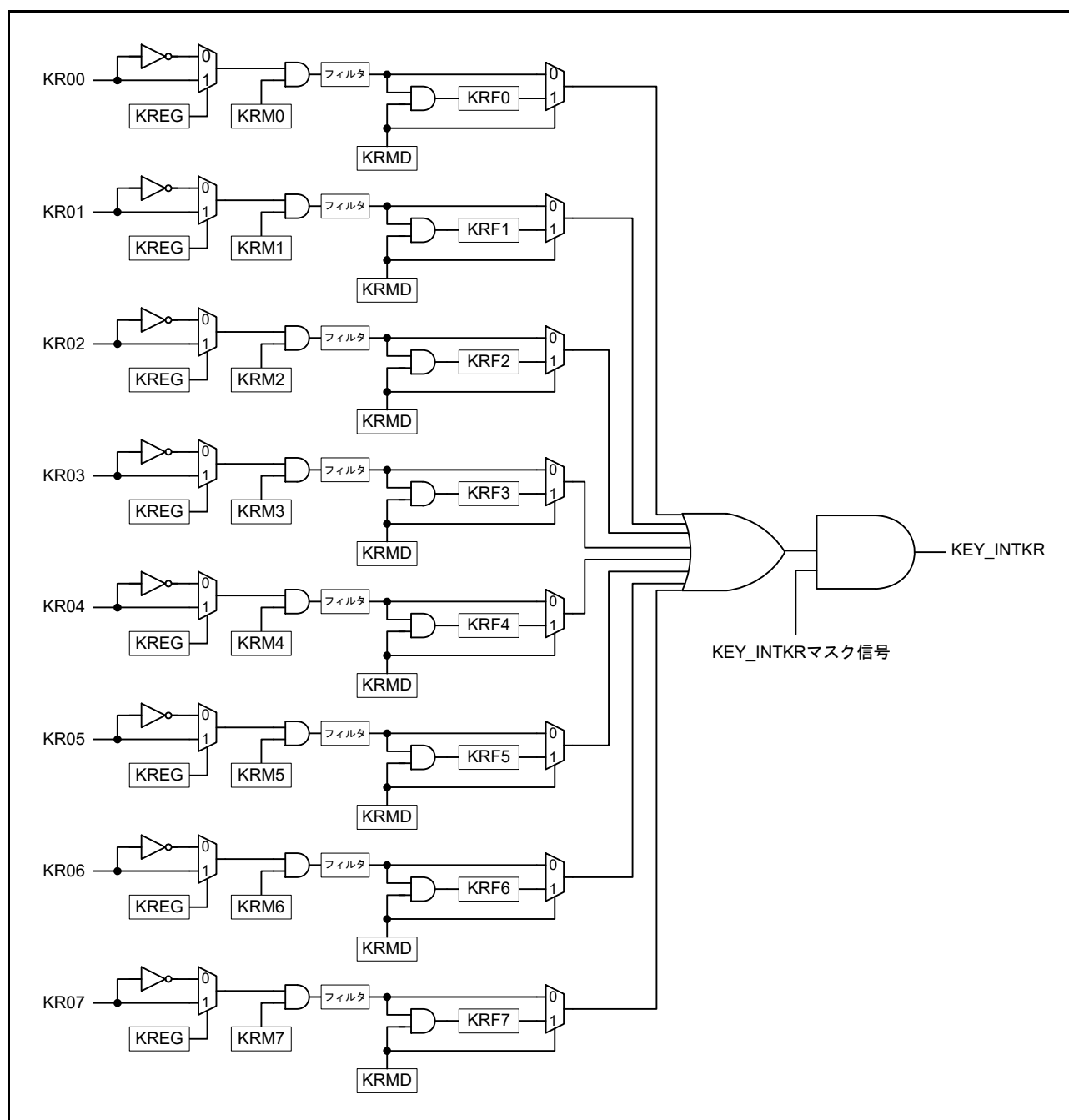
図 21.1 キー割り込み機能のブロック図
