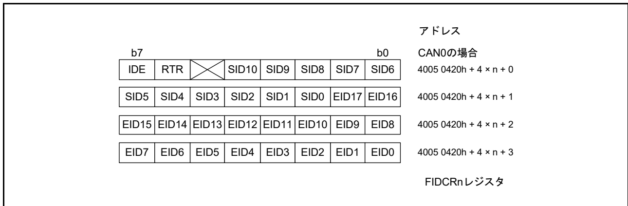
図 33.15 FIDCRn レジスタの構成 (n = 0, 1)
