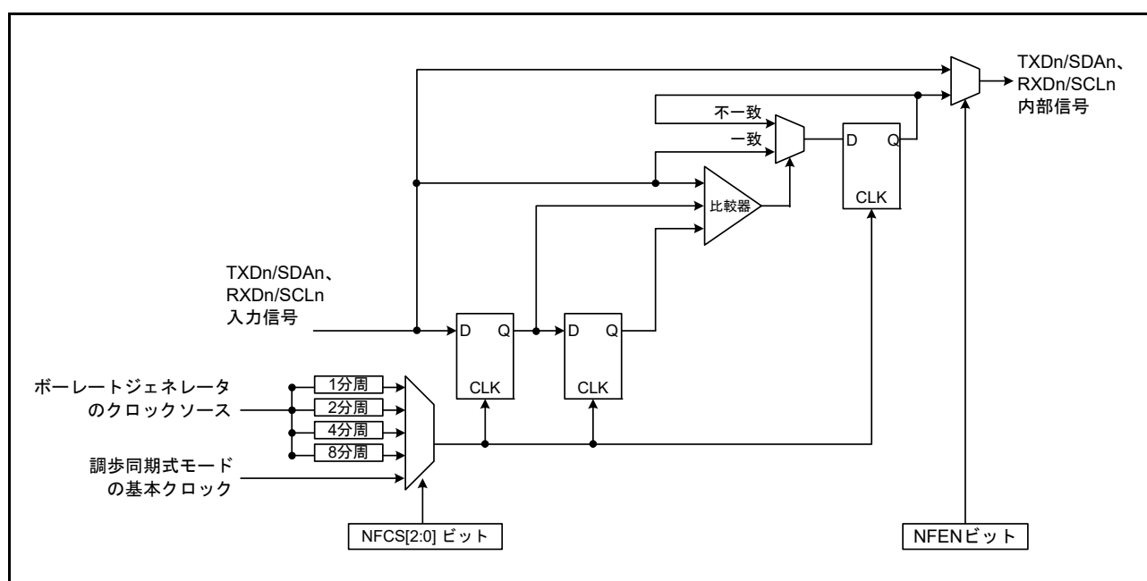
図 30.72 デジタルノイズフィルタ回路のブロック図
