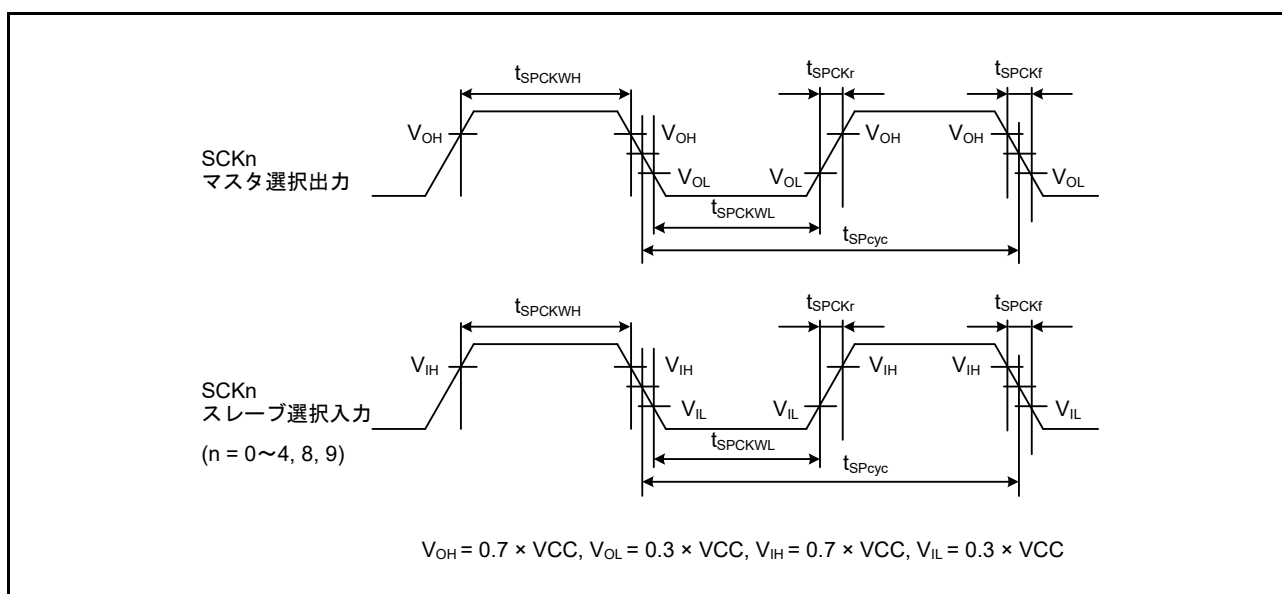
図 52.38 SCI 簡易 SPI モードクロックタイミング
