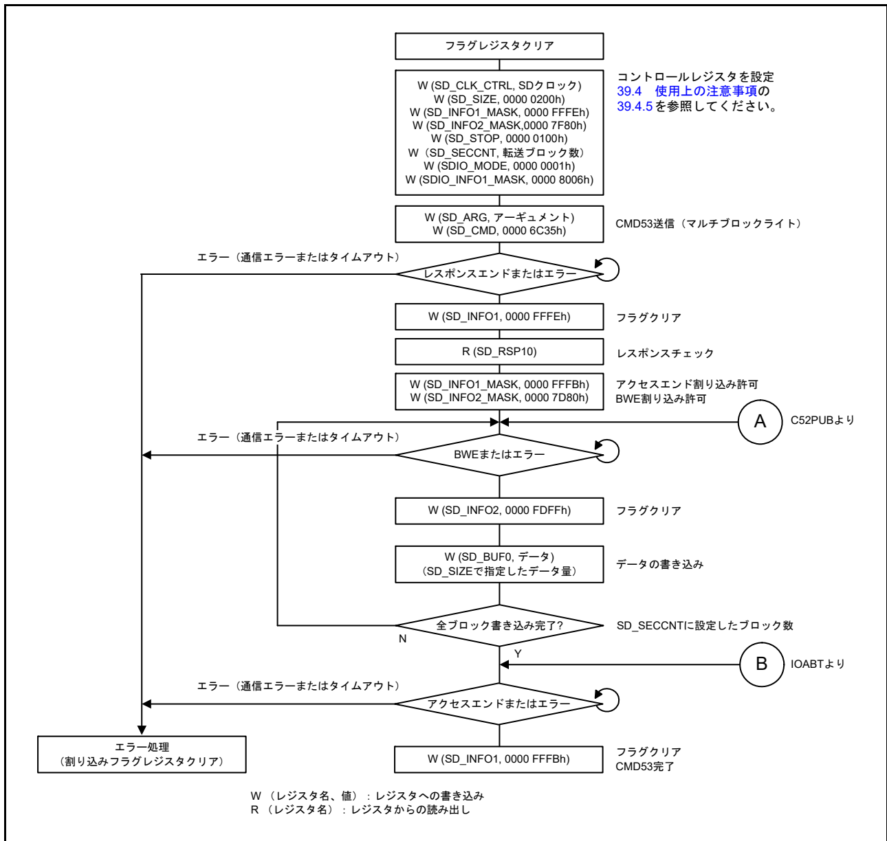
図 39.19 CMD53 マルチブロックライト動作時の IO_RW_EXTENDED コマンドの例
