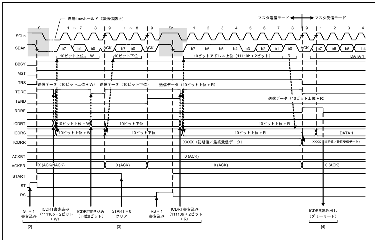
図 32.13 マスタ受信の動作タイミング (2) (10 ビットアドレスフォーマットで RDRFS = 0 の場合)
