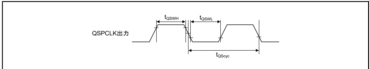
図 52.51 QSPI クロックタイミング
