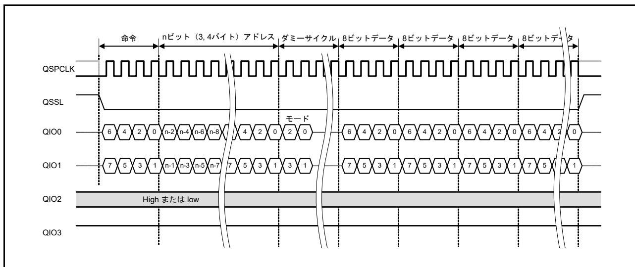
図 35.6 Dual-SPI プロトコル例 (ファストリード Dual I/O)
