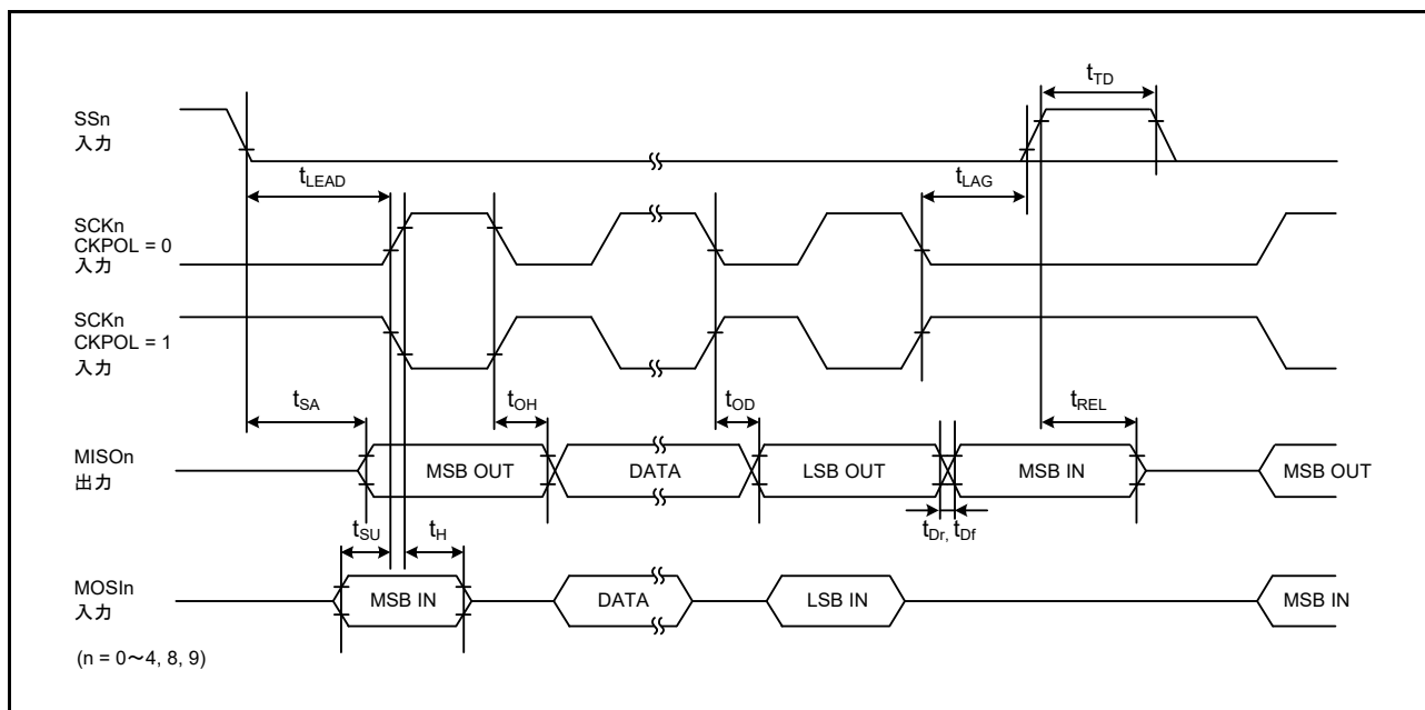
図 52.41 CKPH = 1 の場合におけるスレーブの SCI 簡易 SPI モードタイミング
