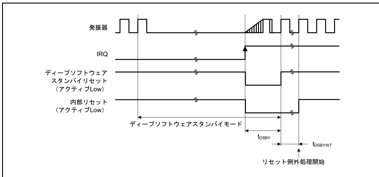
図 52.16 ディープソフトウェアスタンバイモード解除タイミング
