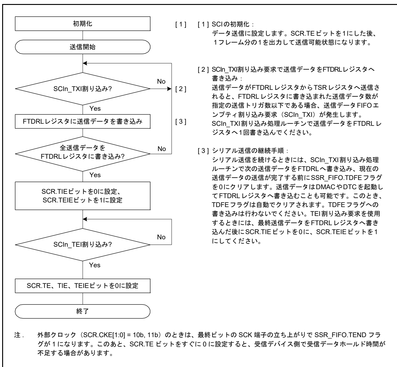
図 30.38 クロック同期式モードにおけるシリアル送信のフローチャート例 (FIFO 選択時)
