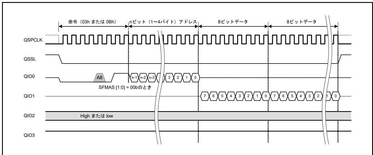
図 35.15 標準リードバスサイクル
