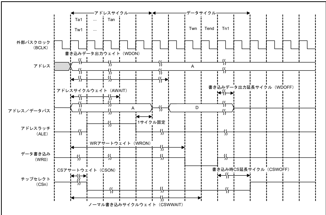
図 15.22 アドレス/データマルチプレクス I/O インタフェース時のライトアクセスの動作例 (n = 0, 1, 4 ~ 7)
