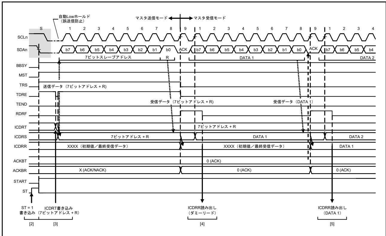
図 32.12 マスタ受信の動作タイミング (1) (7 ビットアドレスフォーマットで RDRFS = 0 の場合)
