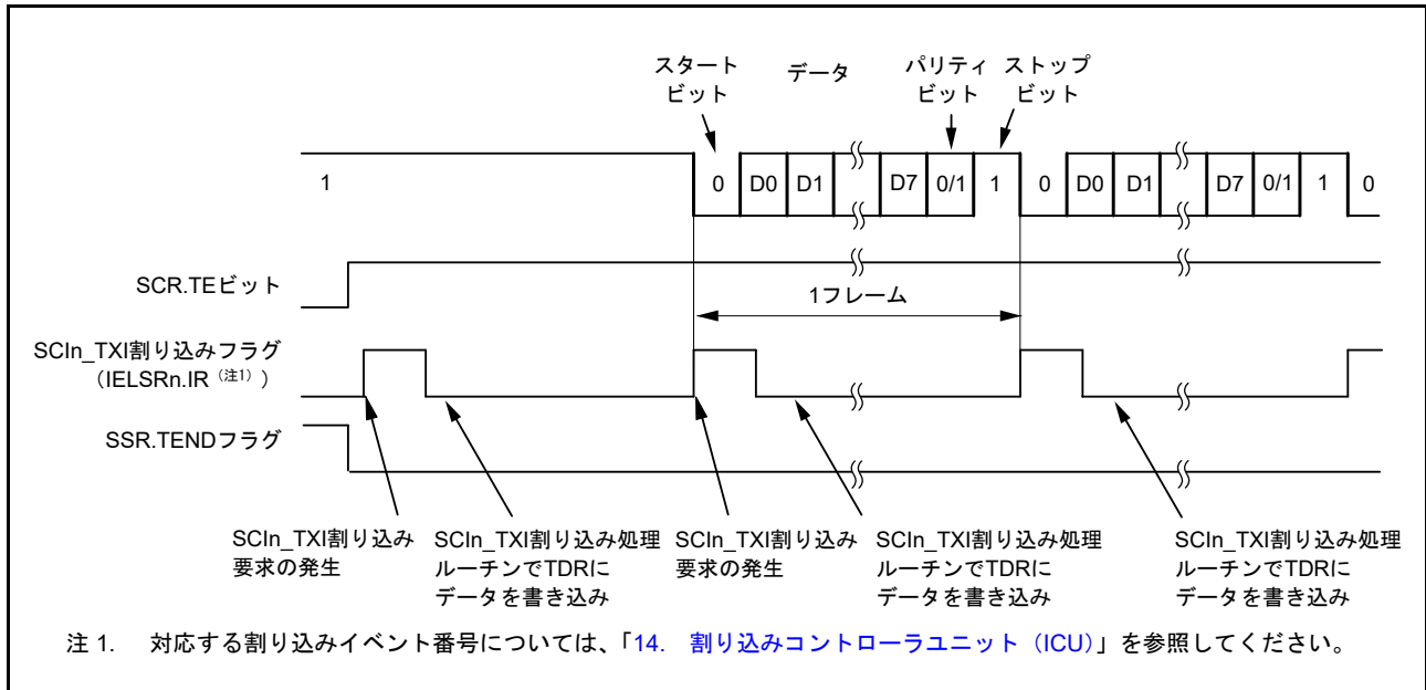
図 30.9 調歩同期式モードにおけるシリアル送信の動作例 (1) (8 ビットデータ/パリティあり/1ストップビット/CTS 機能不使用/送信開始時)
