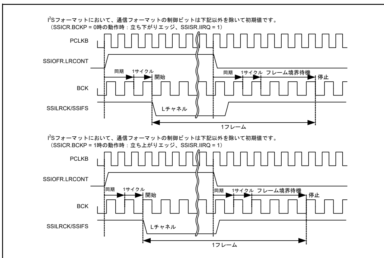
図 37.43 SSIOFR.LRCONT ビットによる LR クロック/フレーム同期継続の禁止例
