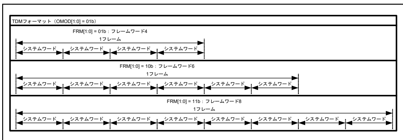
図 37.12 フレームワード数
