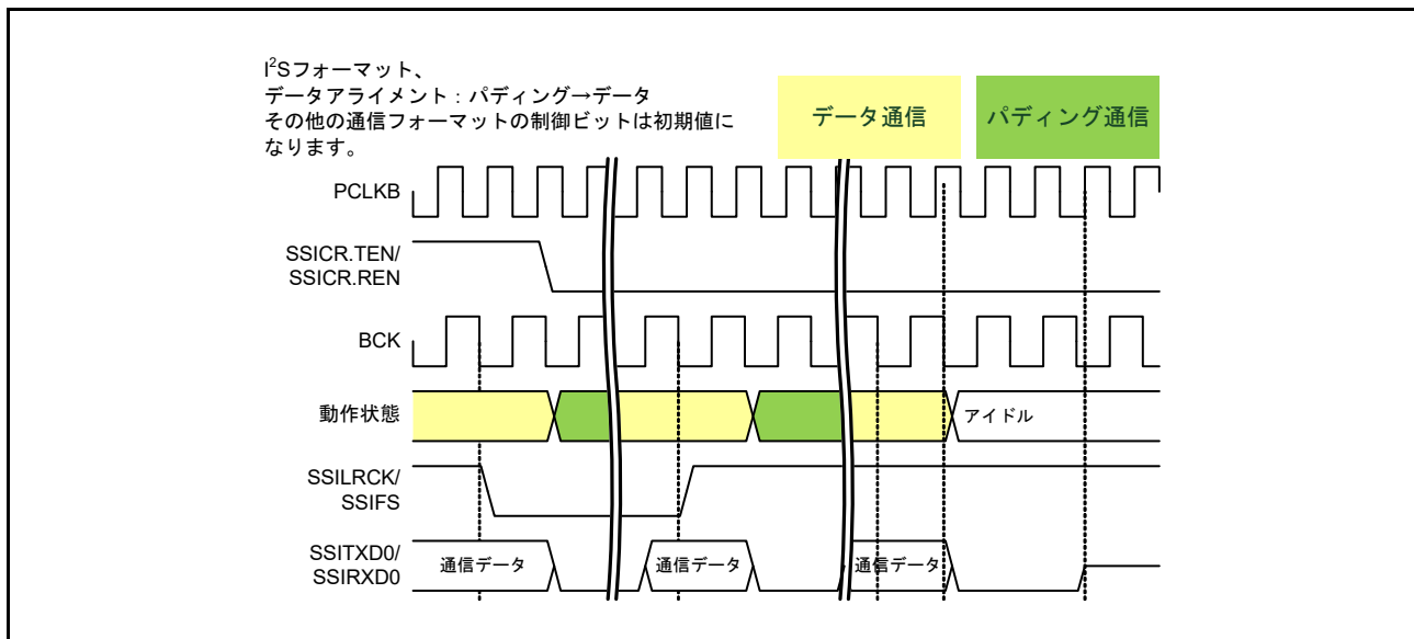
図 37.49 データ通信からの停止 (パディングビットあり)
