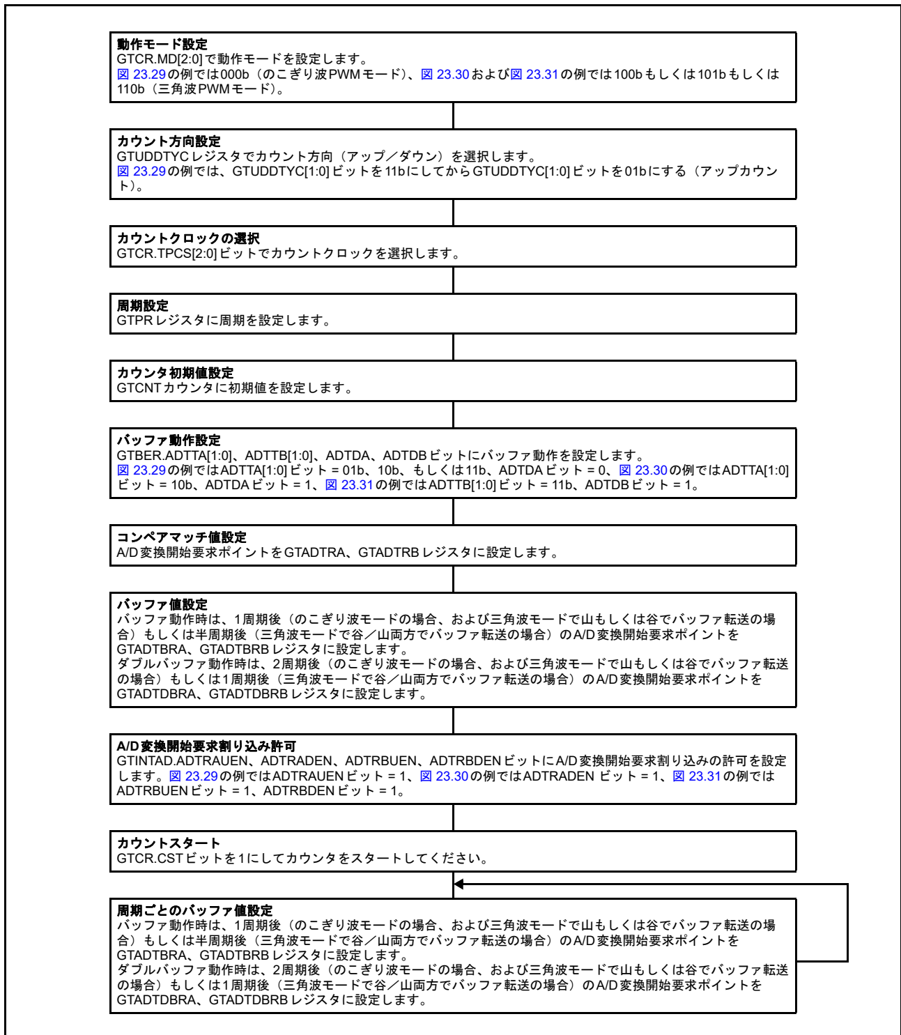
図 23.32 GTADTRA、GTADTRB レジスタのバッファ動作設定例
