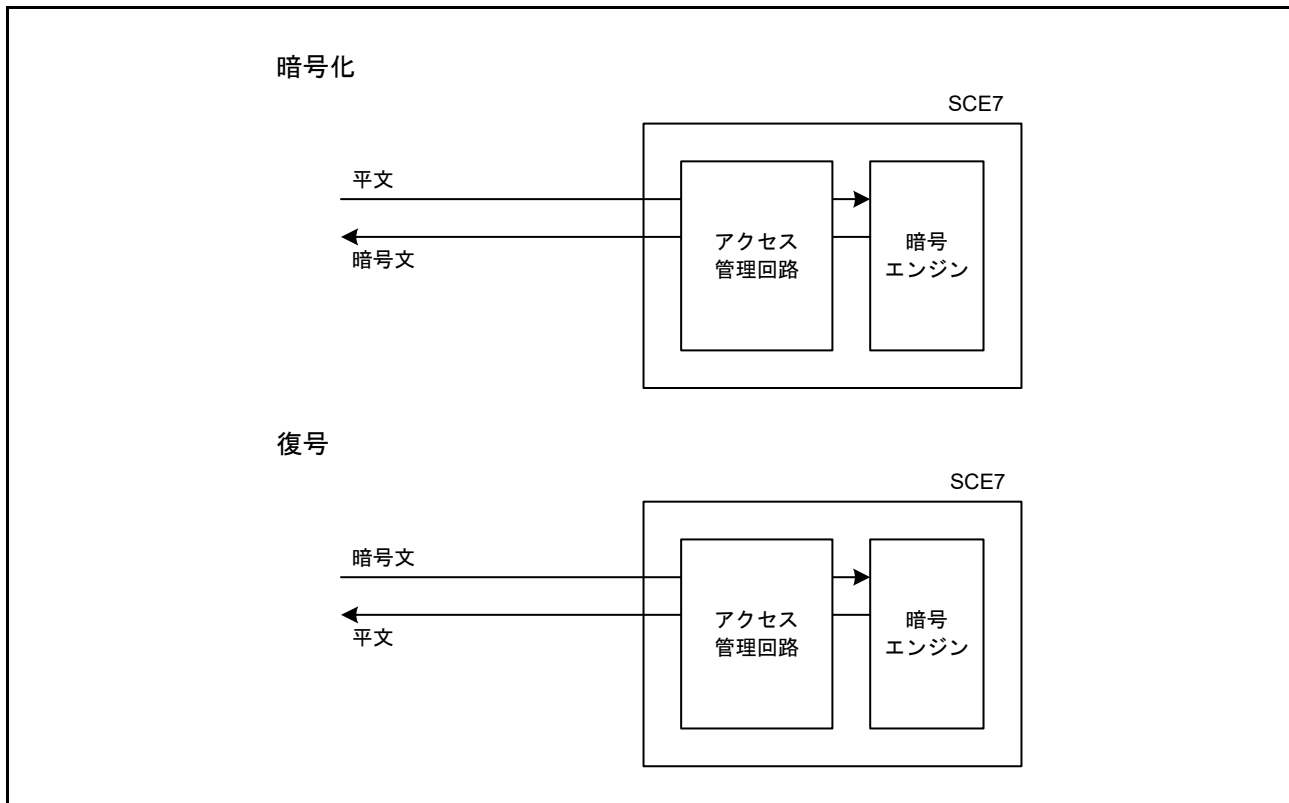
図 41.2 暗号エンジンによる暗号化と復号
