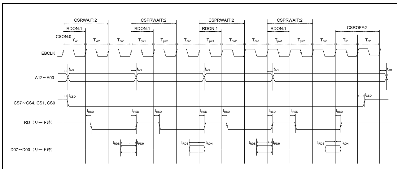
図 52.24 バスクロック同期を使用したページリードサイクルの外部バスタイミング
