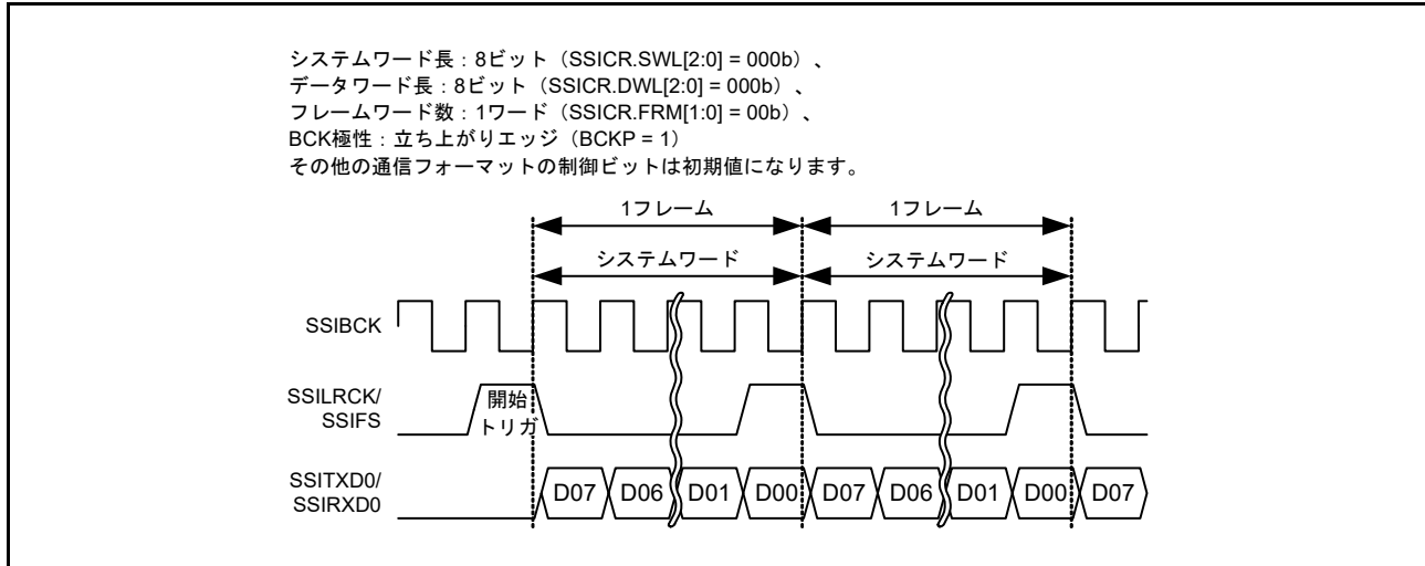
図 37.37 モノラルフォーマットでのショートフレーム (パディングなし、システムワード長 = データワード長)
