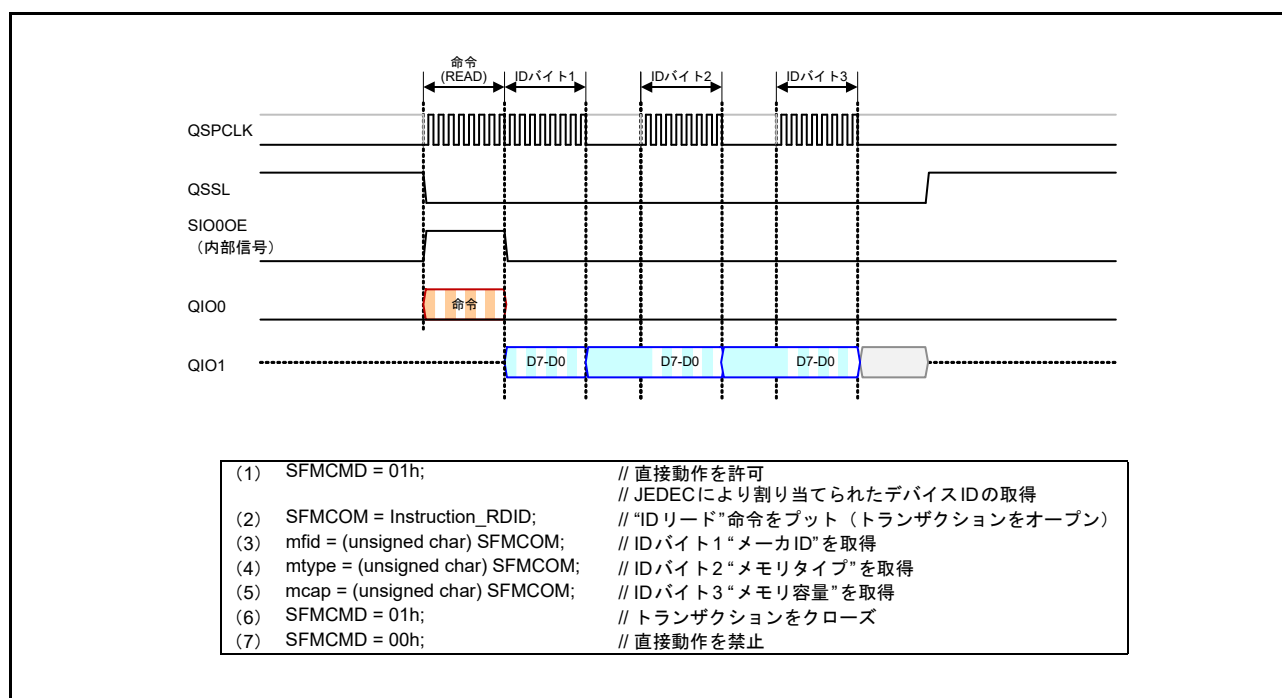
図 35.33 ID リードの直接通信タイミング例
