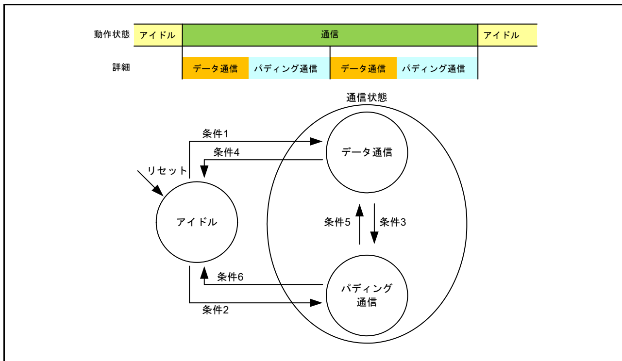
図 37.45 通信の状態遷移
