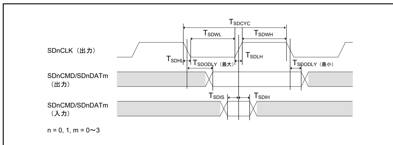
図 52.59 SD/MMC ホストインタフェース信号タイミング
