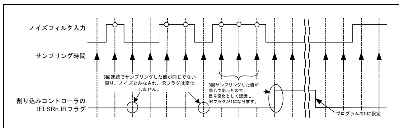
図 45.4 ノイズフィルタおよび割り込み動作例
