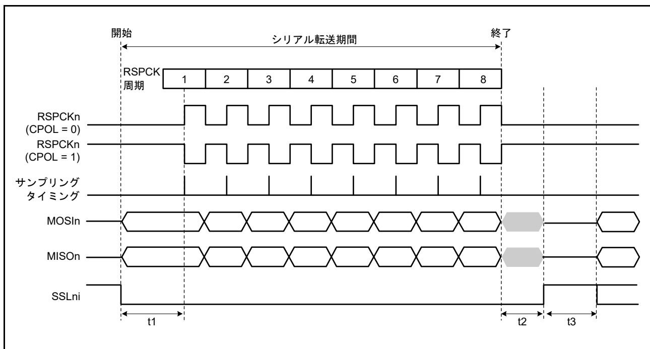
図 34.22 SPI 転送フォーマット (CPHA ビット = 0)
