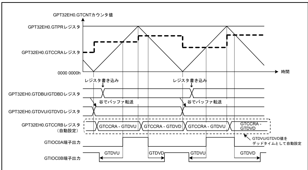
図 23.46 デッドタイム付きコンペアマッチ値の自動設定機能の動作例 (三角波 PWM モード 2 または 3、GTDVU/GTDGD レジスタはバッファ動作、アクティブ High の場合)
