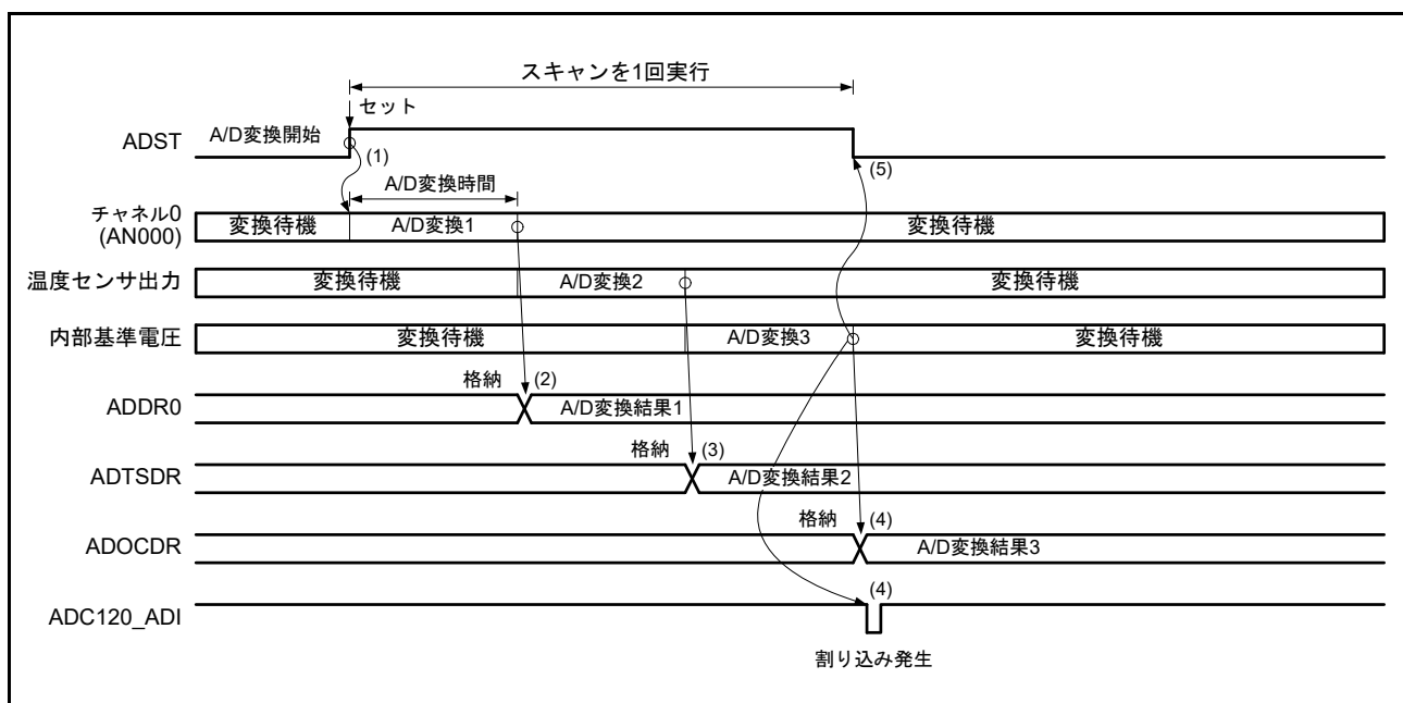
図 42.13 シングルスキャンモードの基本動作例 (AN000、温度センサ出力または内部基準電圧選択)
