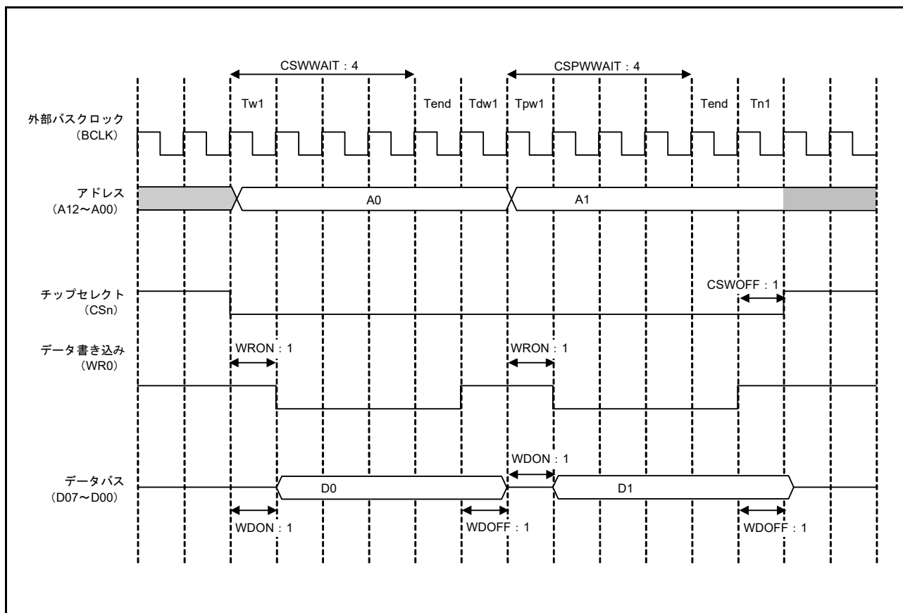
図 15.18 ページライトアクセスの動作例 (8 ビットバス空間に対する 16 ビットアクセスの場合、1 ライトストローブモード時) (n = 0, 1, 4 ~ 7)
