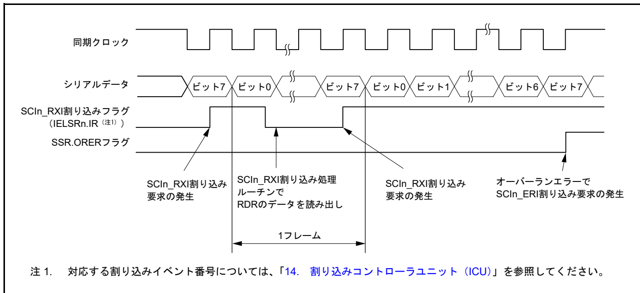
図 30.39 クロック同期式モードにおけるシリアル受信の動作例 (1) (RTS 機能を使用しない場合)
