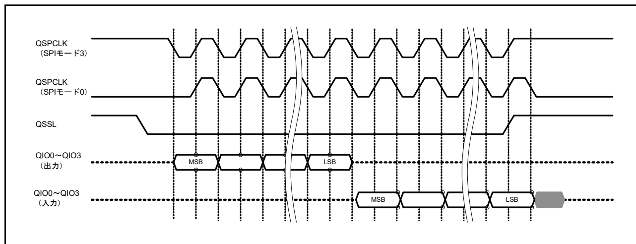
図 35.8 シリアルインタフェースの基本タイミング
