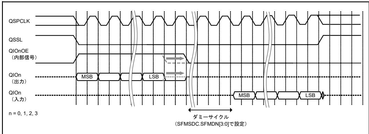
図 35.12 SFMOEX ビットを使用した出力許可ホールド時間調整
