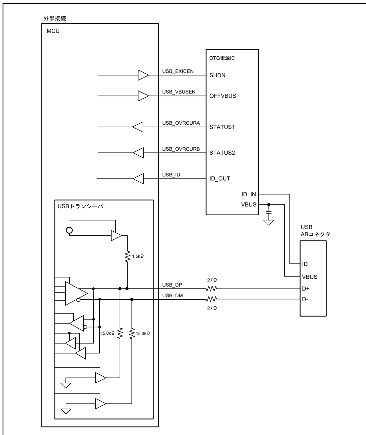
図 29.2 セルフパワー状態での OTG 接続例
