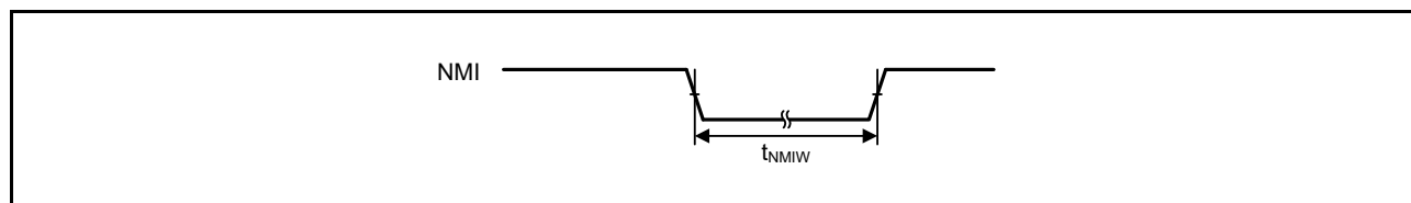
図 52.18 NMI 割り込み入力タイミング
