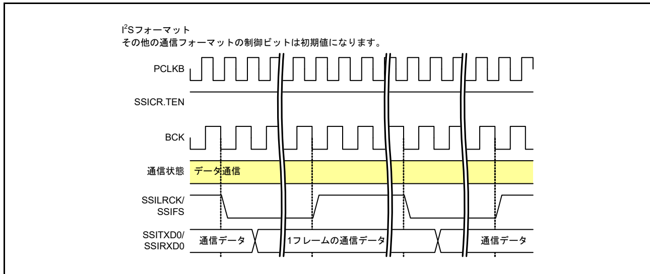
図 37.46 データ通信の継続
