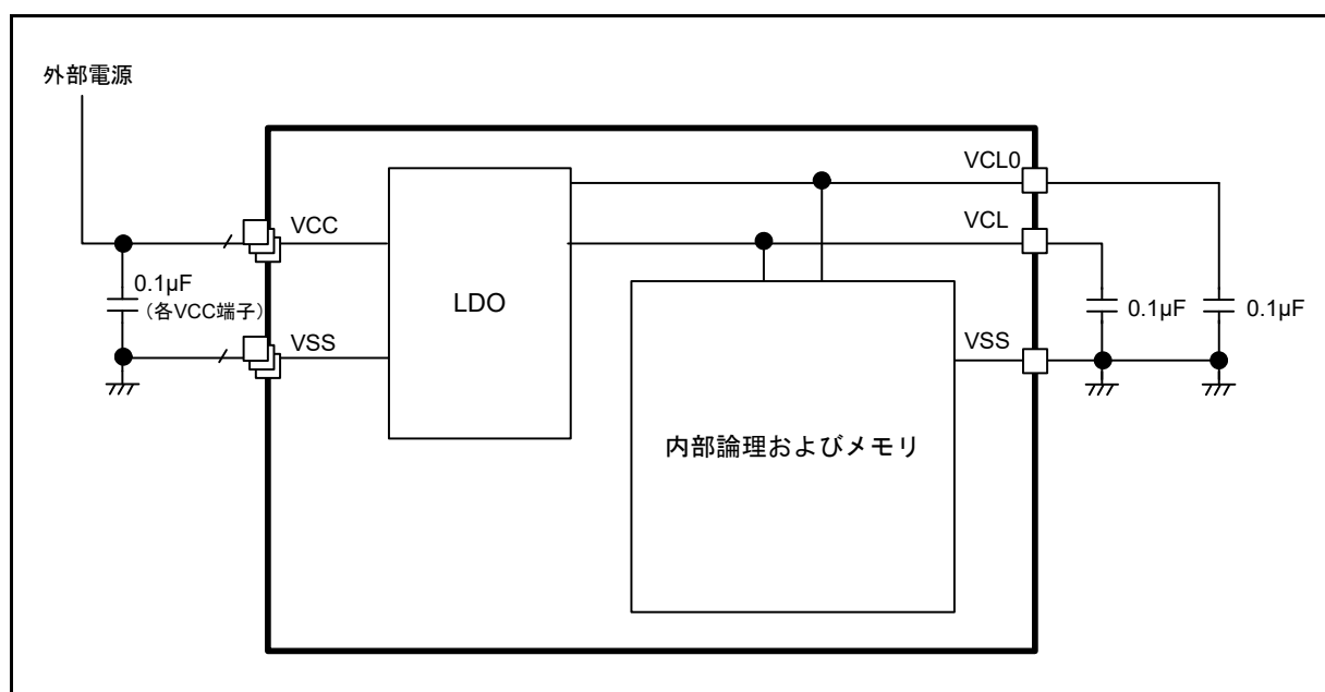
図 51.1 LDOモード設定
