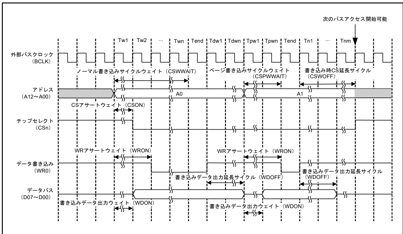
図 15.16 ページライトアクセスのタイミング (n = 0, 1, 4 ~ 7)
