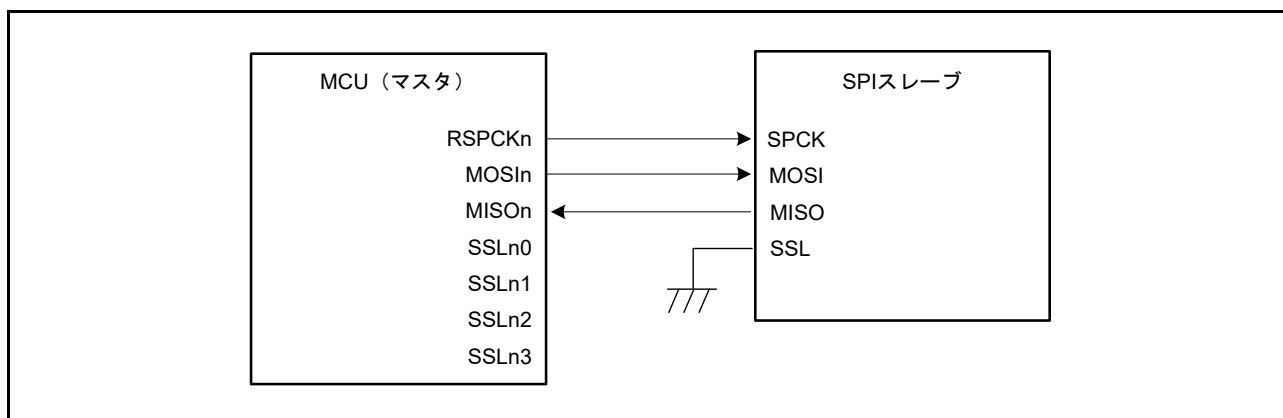
図 34.5 シングルマスタ/シングルスレーブの構成例 (MCU はマスタ)
