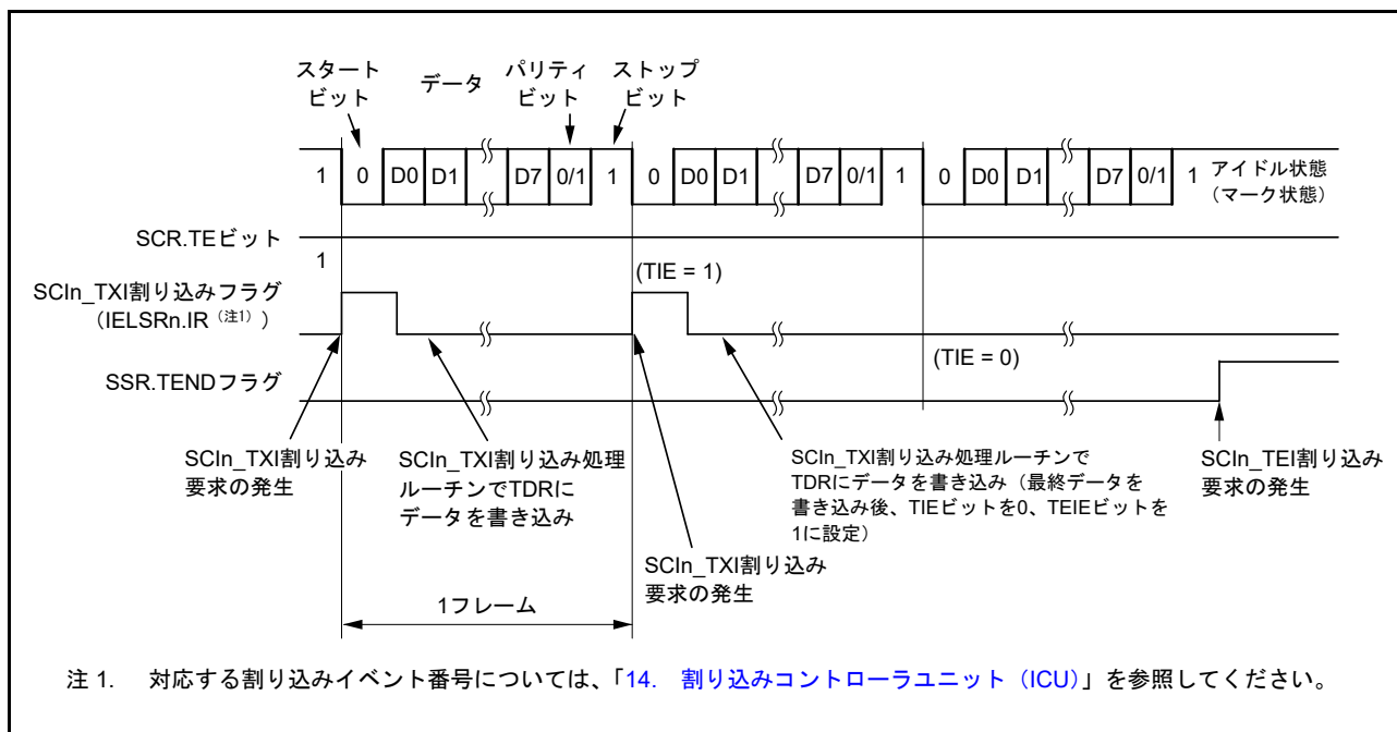
図 30.11 調歩同期式モードにおけるシリアル送信の動作例 (3) (8 ビットデータ/パリティあり/1 ストップビット/CTS 機能不使用/送信中~送信終了時)
