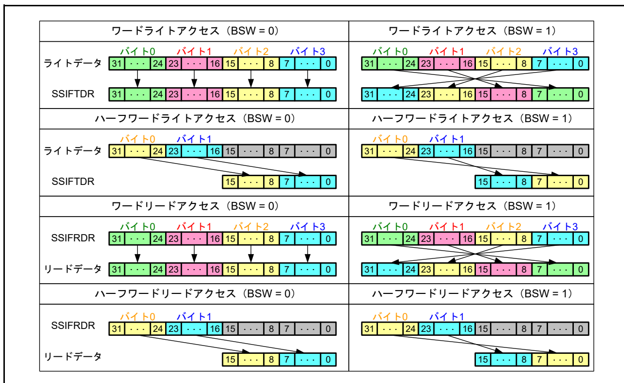
図 37.23 バイトスワップの動作例
