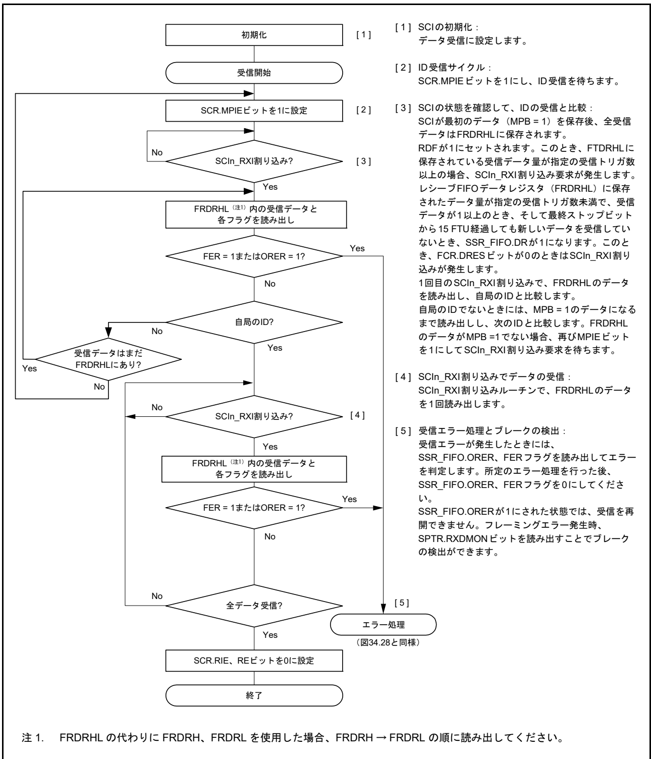
図 30.30 マルチプロセッサモードにおけるシリアル受信のフローチャート例 (FIFO 選択時)
