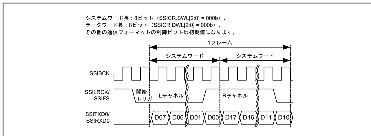
図 37.36 I 2 S フォーマット (パディングなし、システムワード長 = データワード長)
