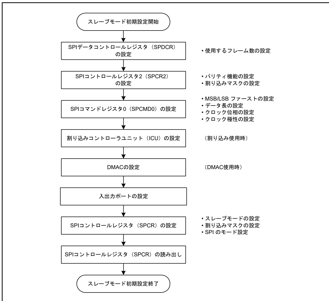
図 34.48 スレーブモード時のクロック同期式動作の初期化フロー例
