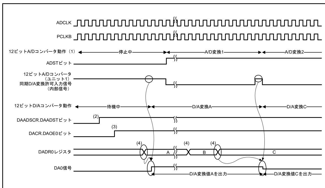
図 43.3 DAC12をADC12に同期して変換する例
