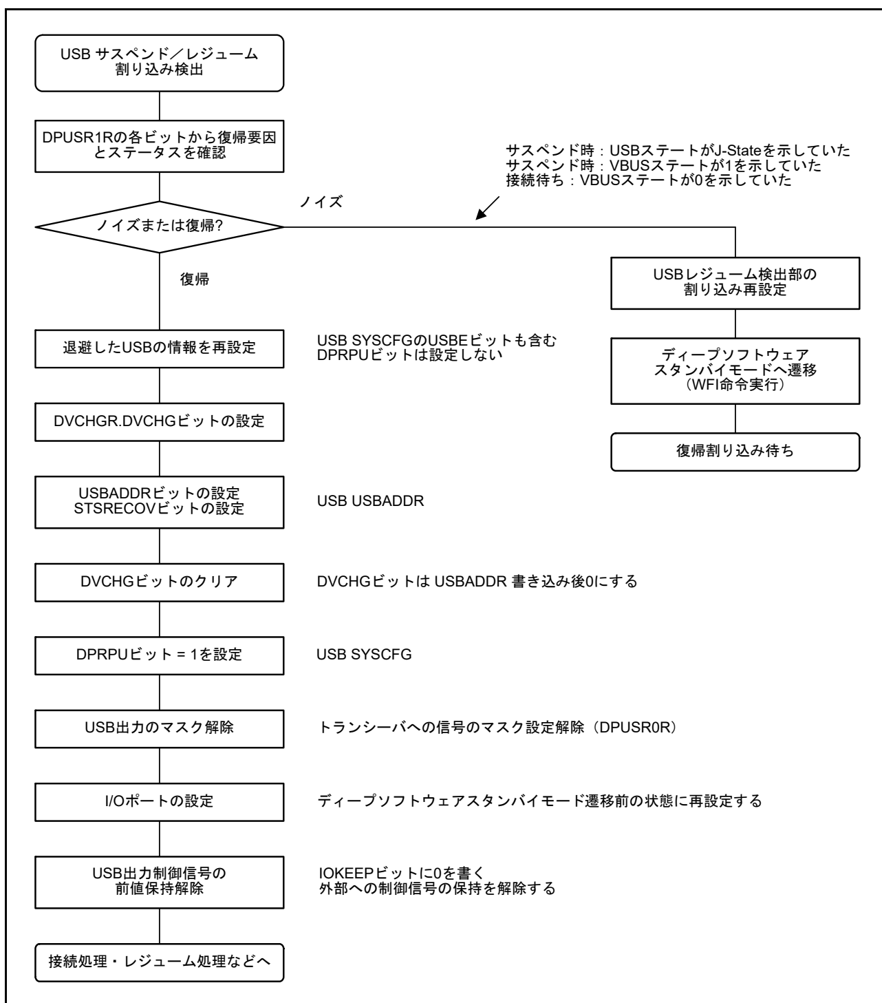
図 29.9 デバイスコントローラ機能選択時におけるディープソフトウェアスタンバイモード解除時の USBFS 設定フロー
