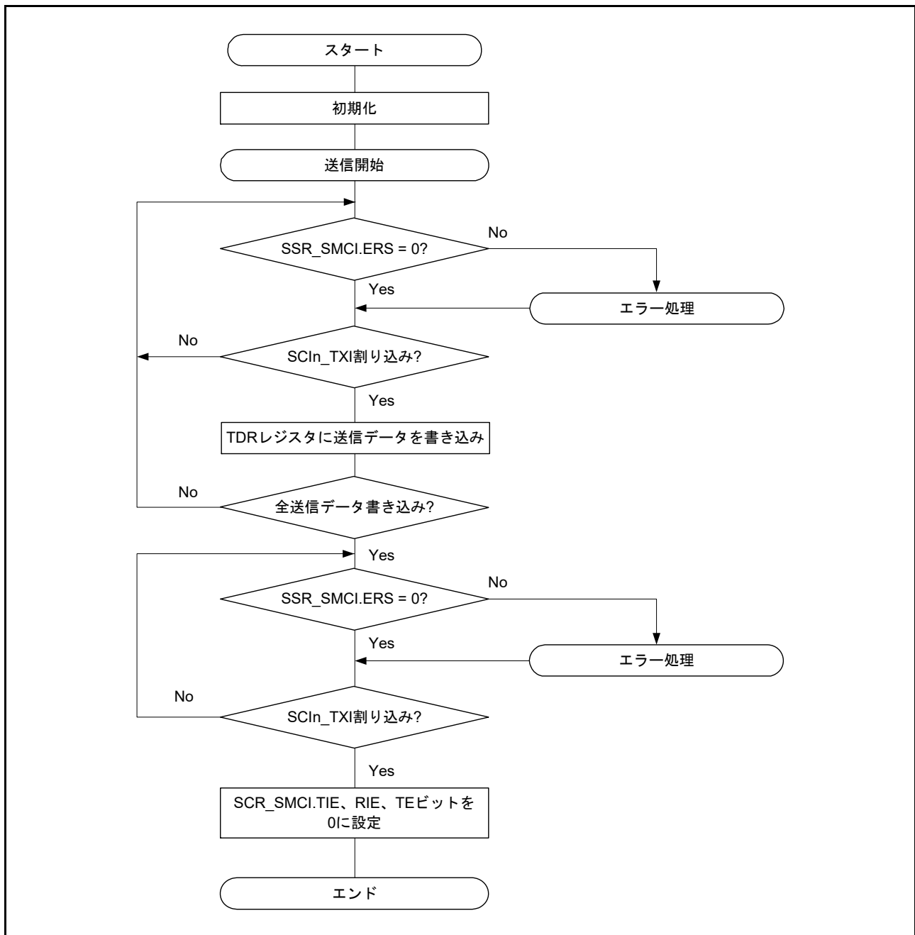
図 30.54 スマートカードインタフェース送信のフローチャート例
