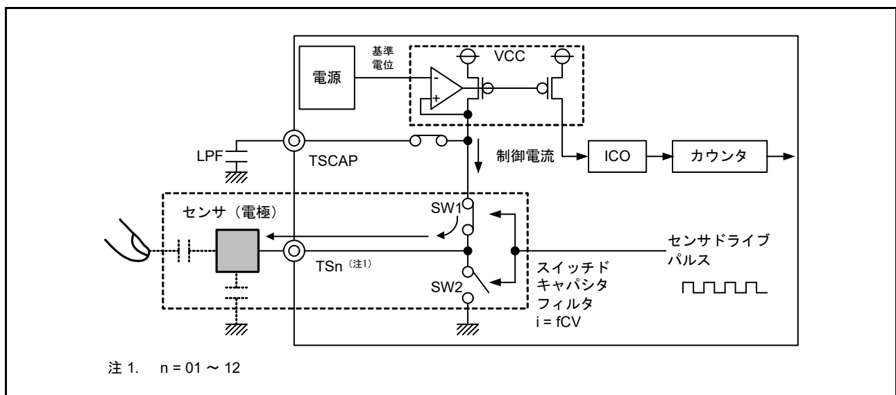
図 46.5 充電動作
