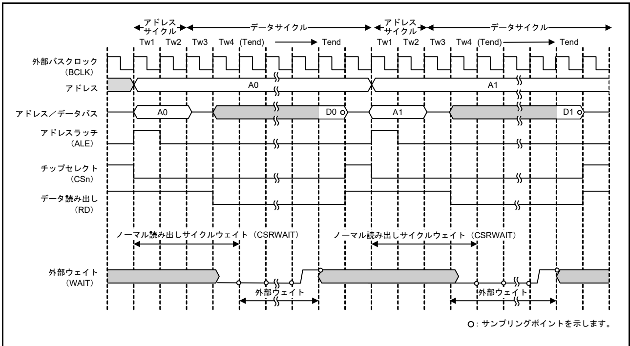
図 15.28 アドレス/データマルチプレクス I/O インタフェース時の外部ウェイト挿入のタイミング例 (n = 0, 1, 4 ~ 7)
