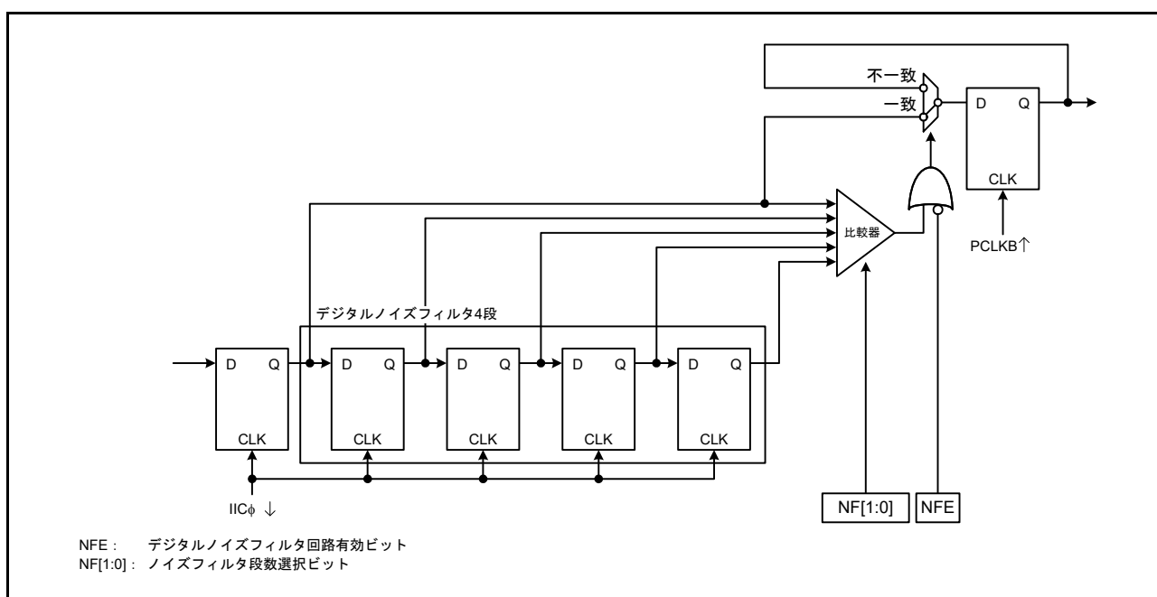
図 32.23 デジタルノイズフィルタ回路のブロック図
