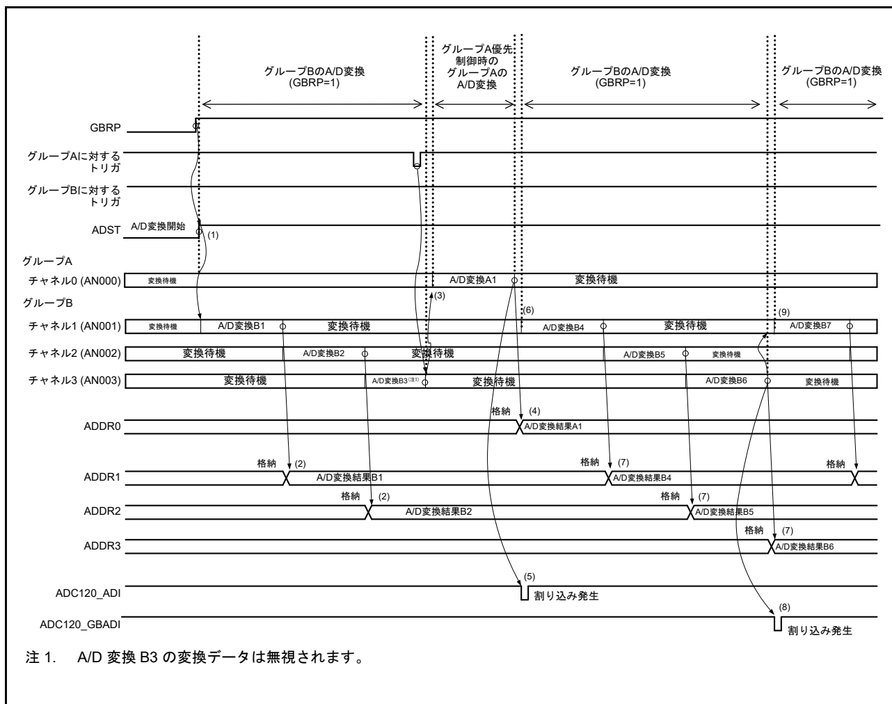
図 42.30 グループ A 優先制御の動作例 (5) (ADGSPCR.GBRP = 1 の場合)
