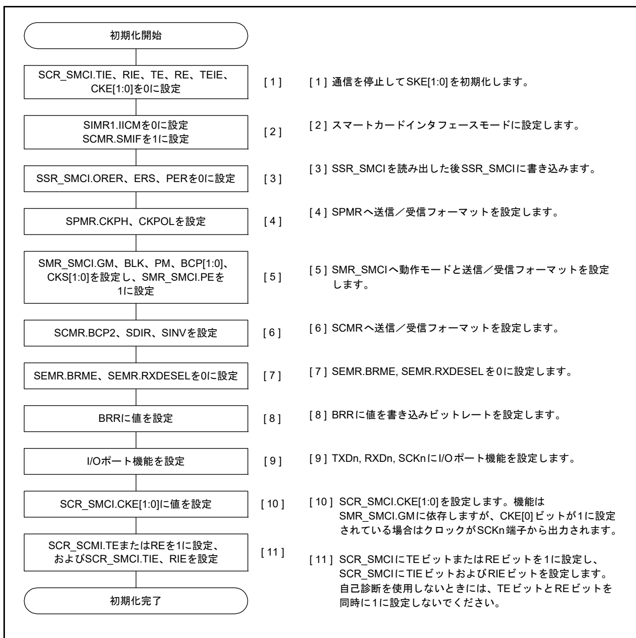
図 30.50 SCI の初期化フローチャート例（スマートカードインタフェースモード）
