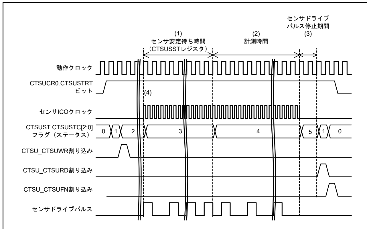
図 46.18 センサ安定待ちと計測のタイミング
