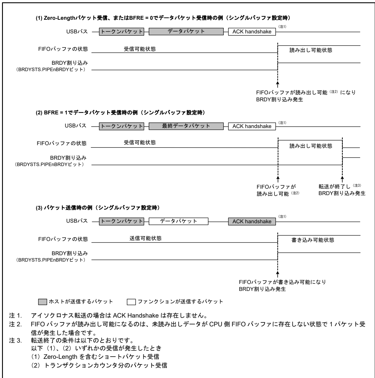
図 29.11 BRDY 割り込み発生タイミング
