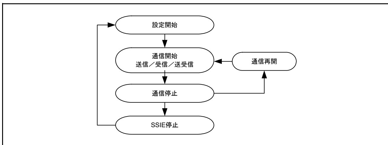
図 37.51 SSIE 通信動作
