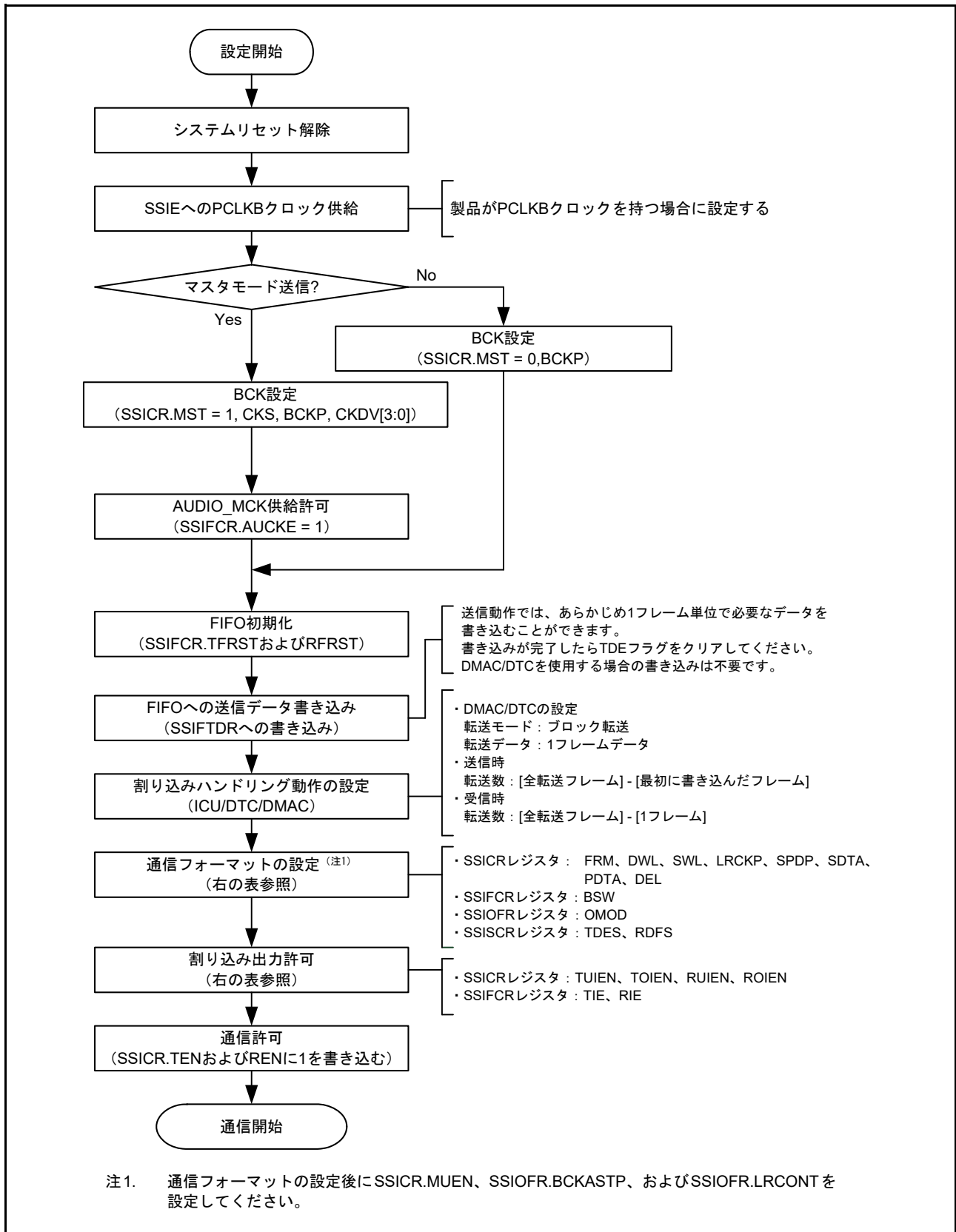
図 37.52 通信開始手順 (CPU 動作手順)
