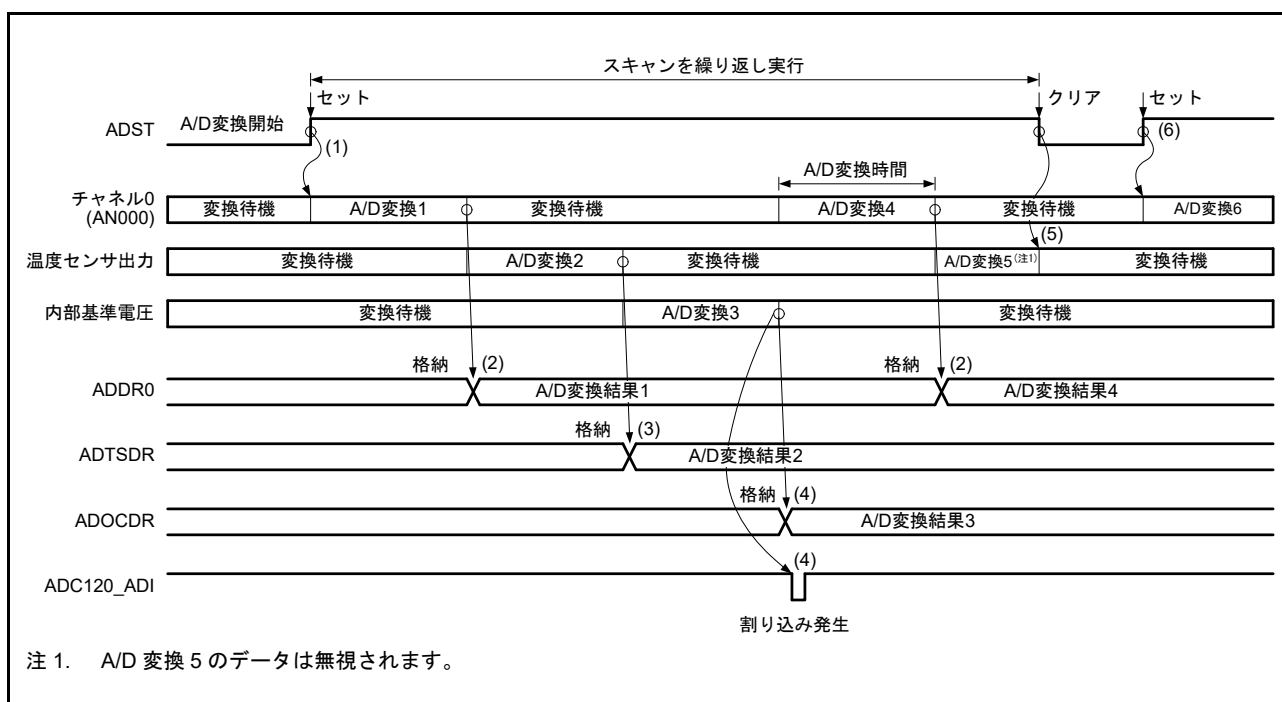
図 42.22 連続スキャンモードの基本動作例 (AN000、温度センサ出力または内部基準電圧選択)
