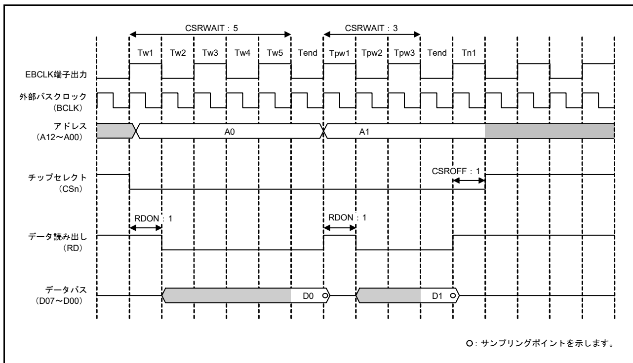
図 15.19 ページリードアクセスの動作例 (EBCLK 端子出力選択ビットで BCLK の 2 分周を設定した場合、および 1 転送要求に対して 2 回バスアクセスが発生する場合) ( n = 0, 1, 4 \sim 7 )
