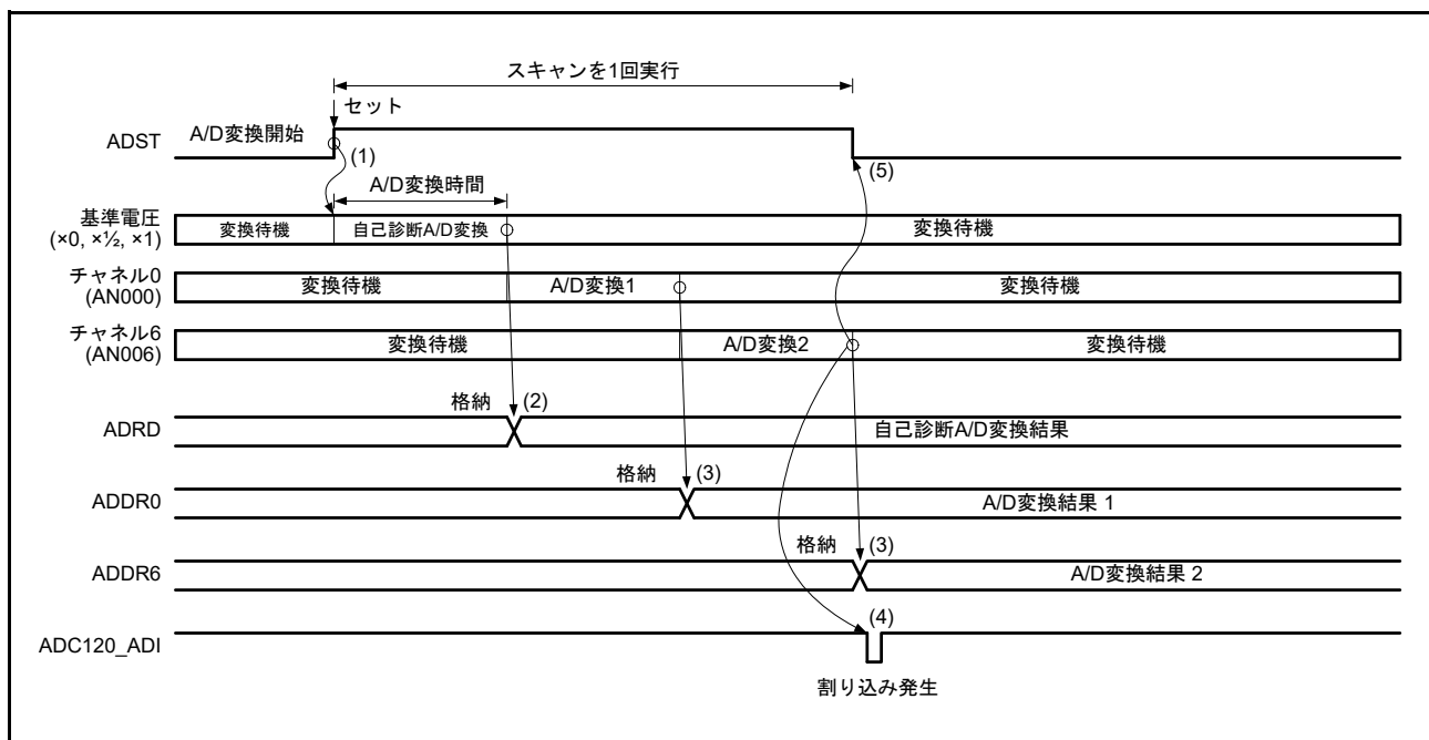
図 42.10 シングルスキャンモードの基本動作例 (AN000、AN006 選択 + 自己診断)
