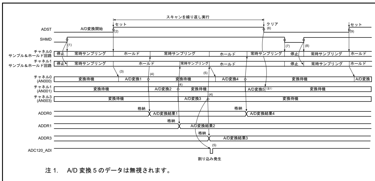
図 42.18 連続スキャンモードの動作例 (チャンネル専用サンプル&ホールド回路使用、AN000、AN001、および AN003 選択、常時サンプリング有効)
