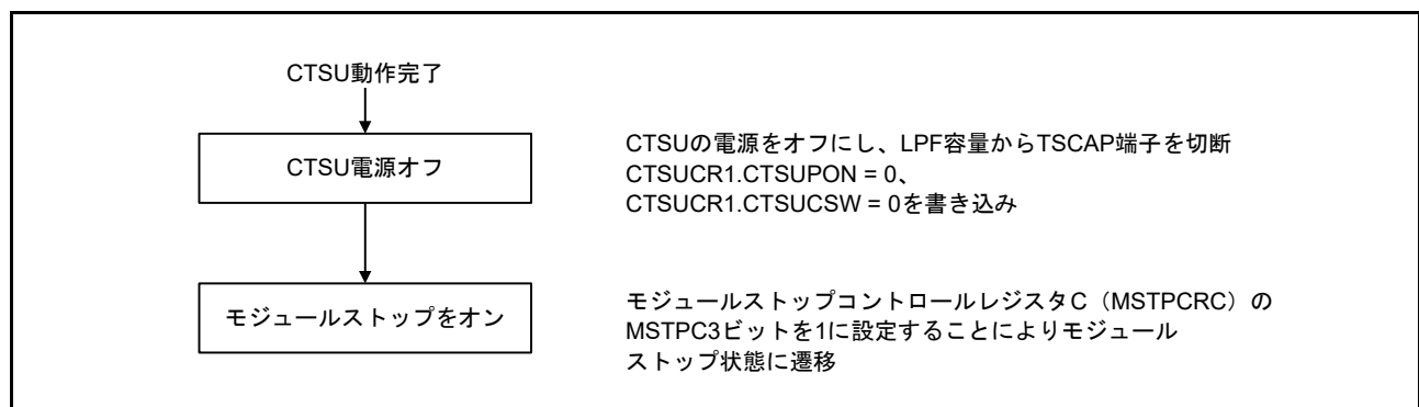
図 46.10 CTSU 停止フロー
