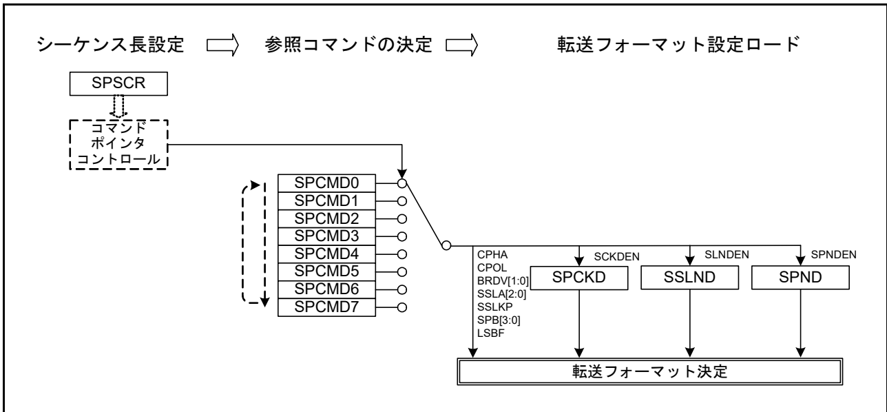
図 34.44 マスタモードでのシリアル転送方式の決定方法
