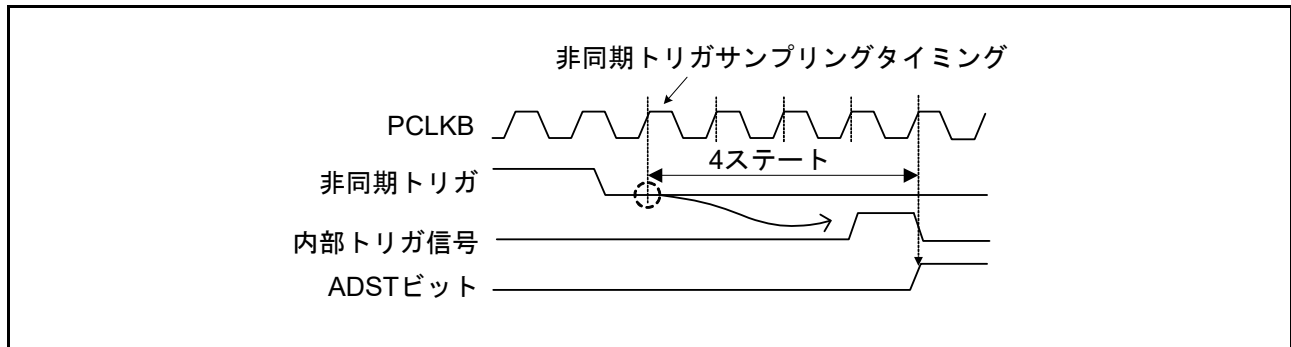
図 42.39 非同期トリガ入力タイミング
