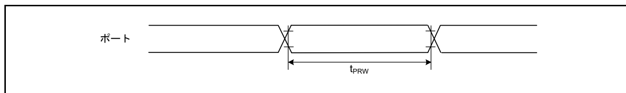
図 52.27 I/Oポート入力タイミング
