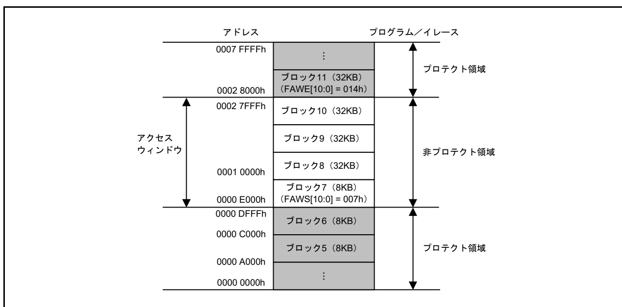
図 50.9 アクセスウィンドウに 8KB および 32KB のブロックが含まれる場合のアクセスウィンドウの開始ブロックアドレス (FAWS) と終了ブロックアドレス (FAWE)
