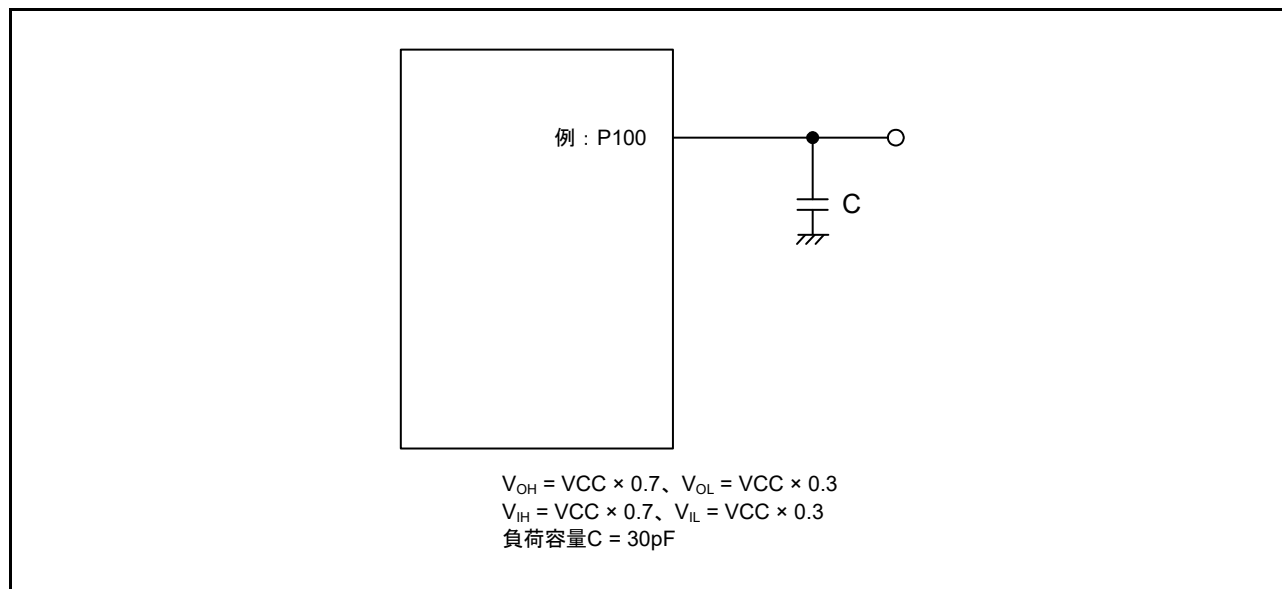
図 52.1 入出力タイミング計測条件
