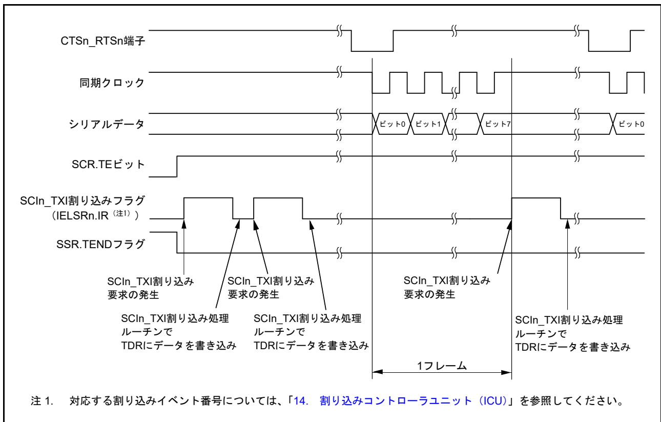
図 30.35 クロック同期式モードにおけるシリアル送信の動作例 (送信開始時に CTS 機能を使用する場合)
