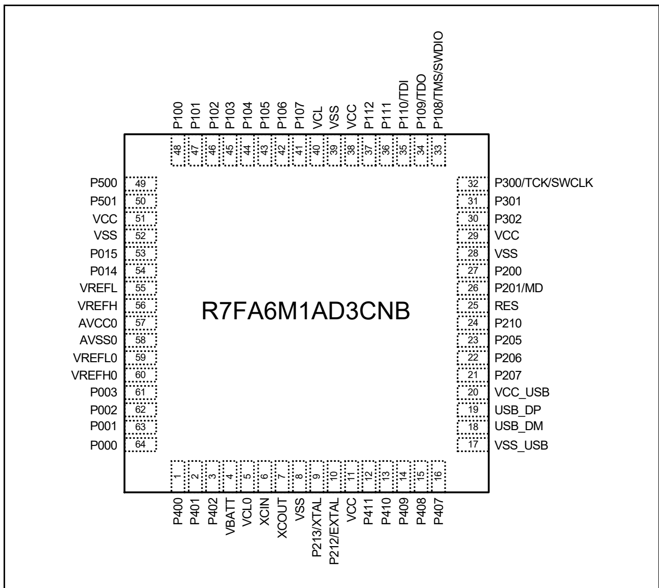
図 1.6 64-pin QFN のピン配置図 (上面図)
