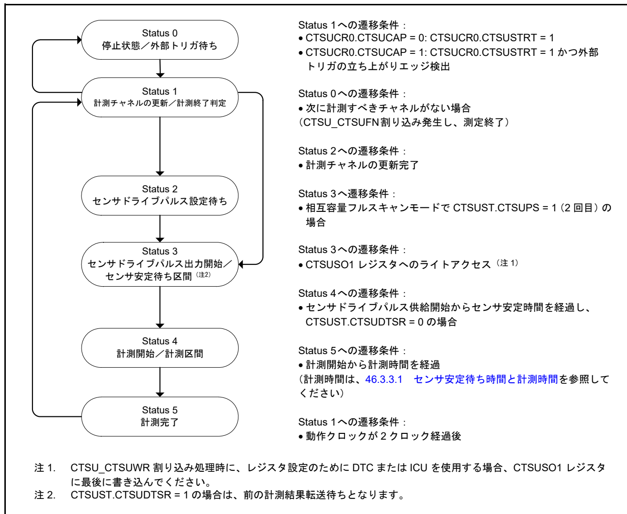
図 46.11 ステータス動作遷移図
