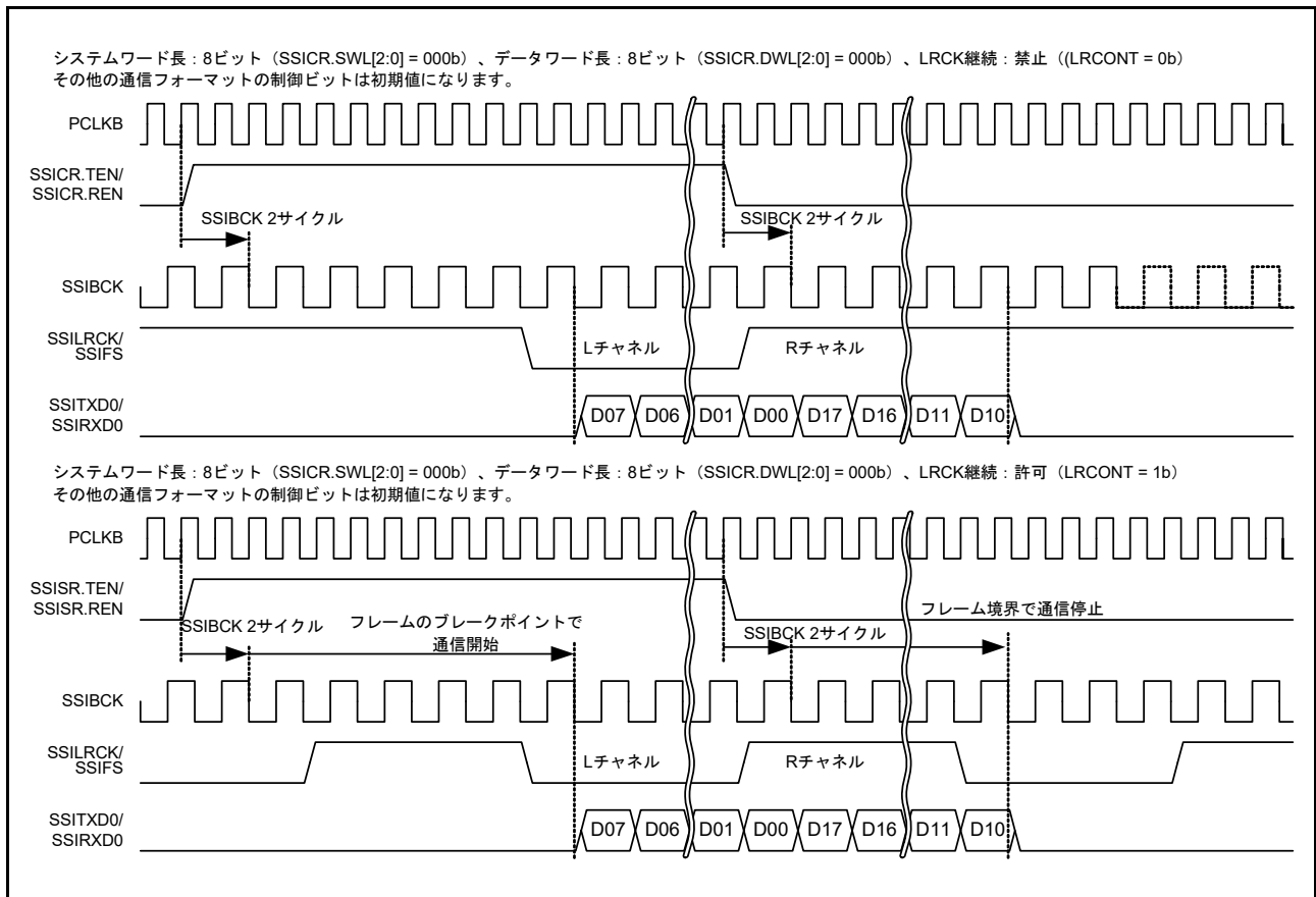
図 37.32 LR クロック/フレーム同期継続の動作例
