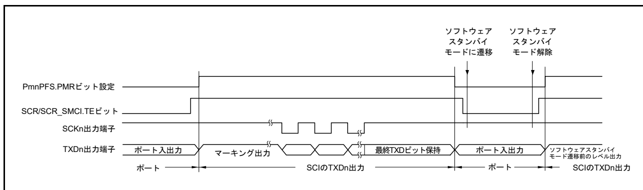
図 30.75 ソフトウェアスタンバイモード遷移中のポートの端子状態 (内部クロック、クロック同期送信)
