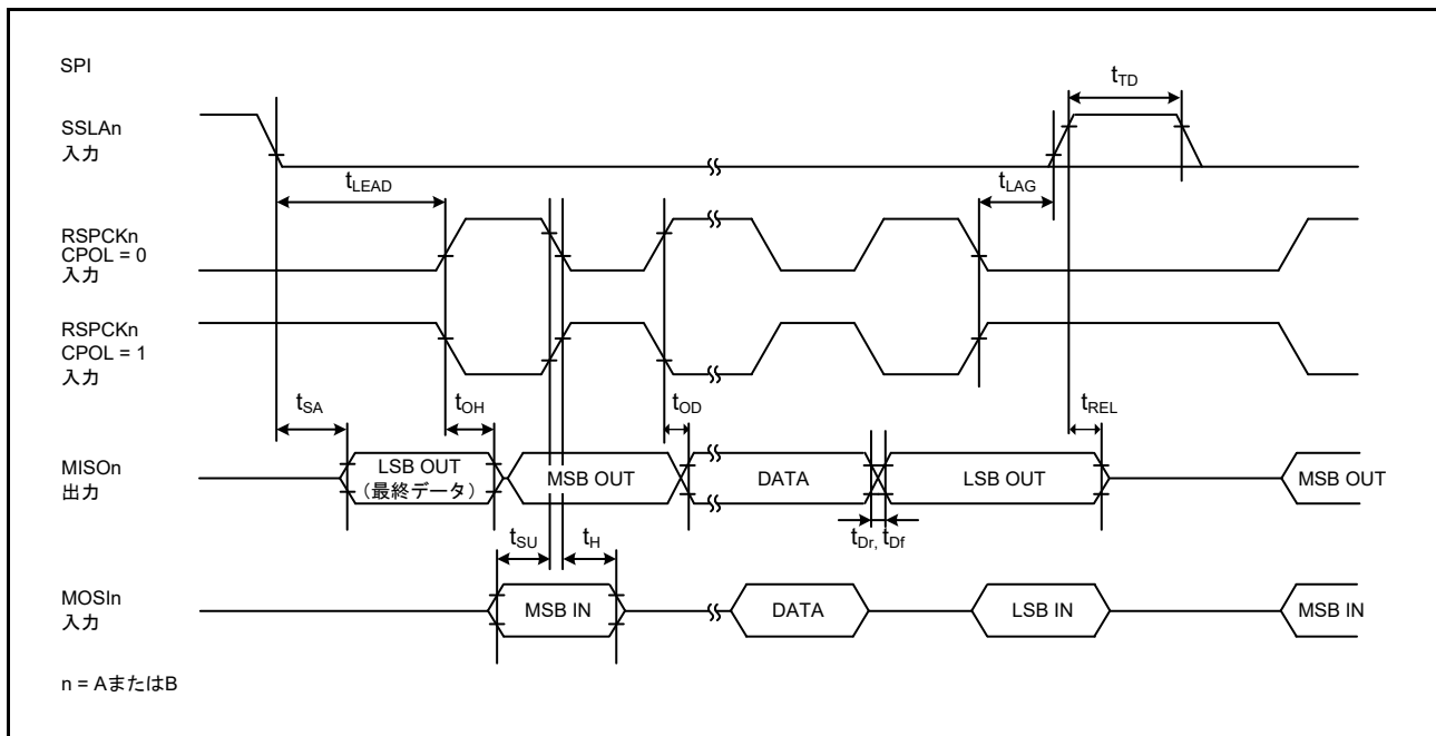
図 52.50 CPHA = 1 の場合におけるスレーブの SPI タイミング
