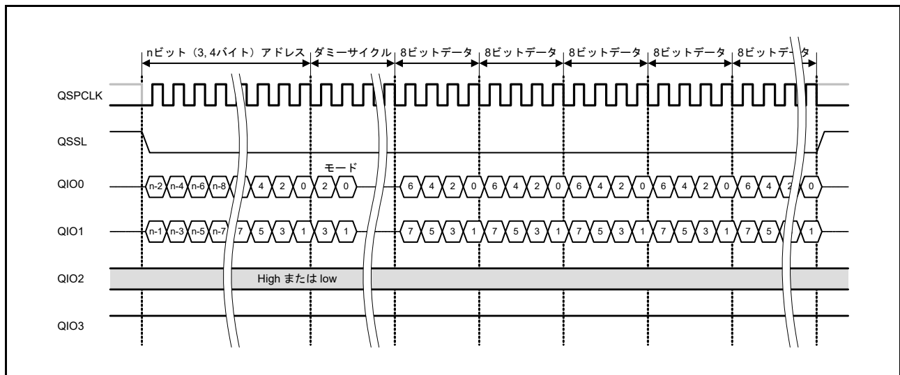
図 35.21 XIP モード時のファストリード Dual I/O バスサイクル
