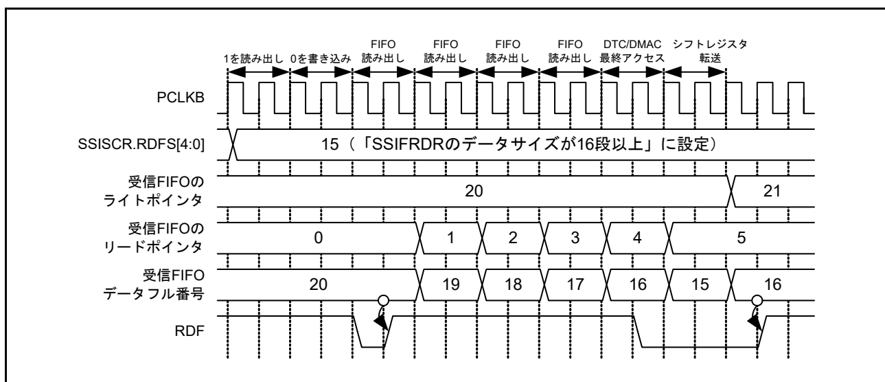
図 37.27 RDF の設定およびクリアのタイミング図
