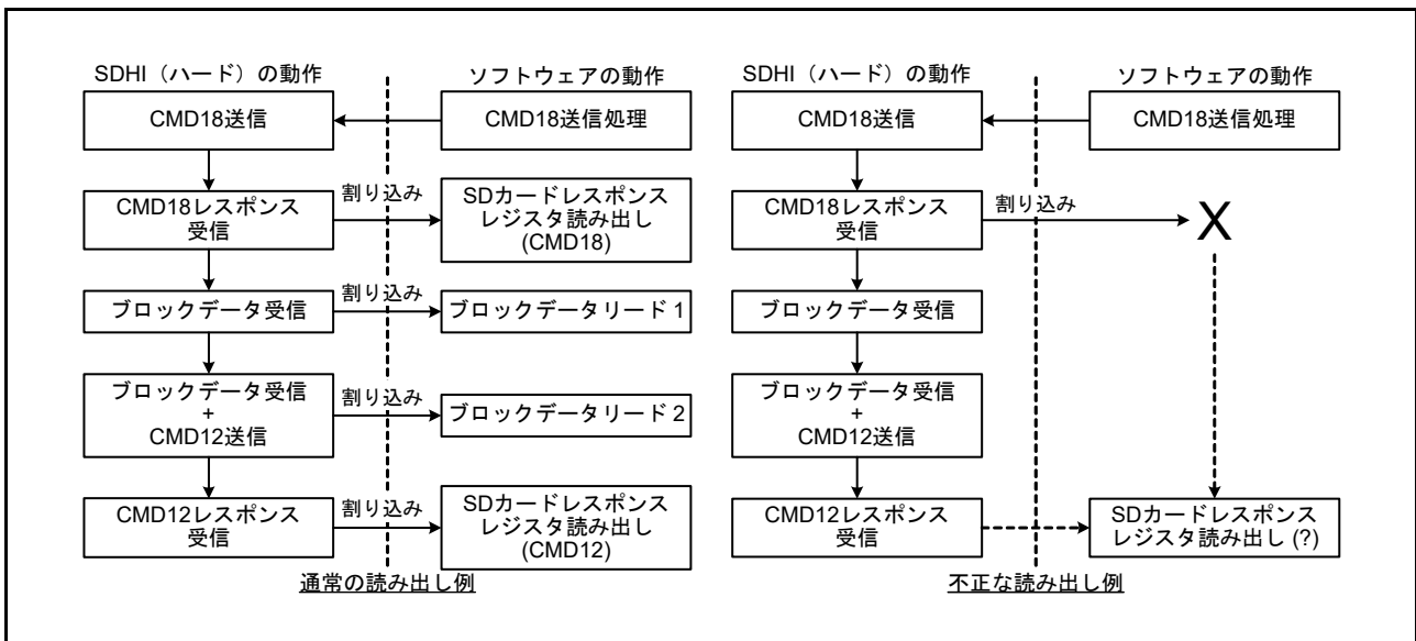
図 39.24 マルチブロックリード動作のフローチャート (2 ブロック)
