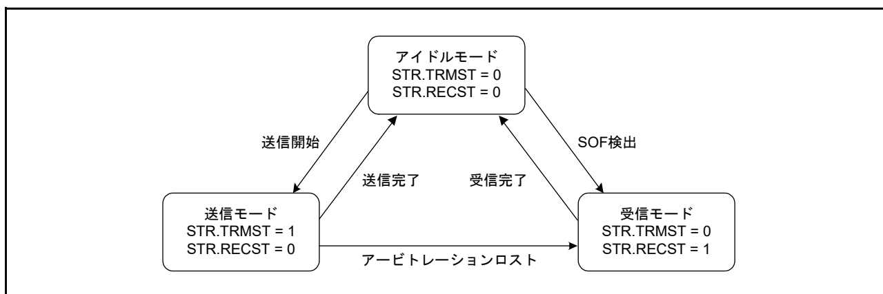
図 33.10 CAN オペレーションモードのサブモード
