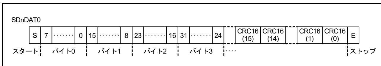
図 39.2 1 ビット幅モードの SDnDAT
