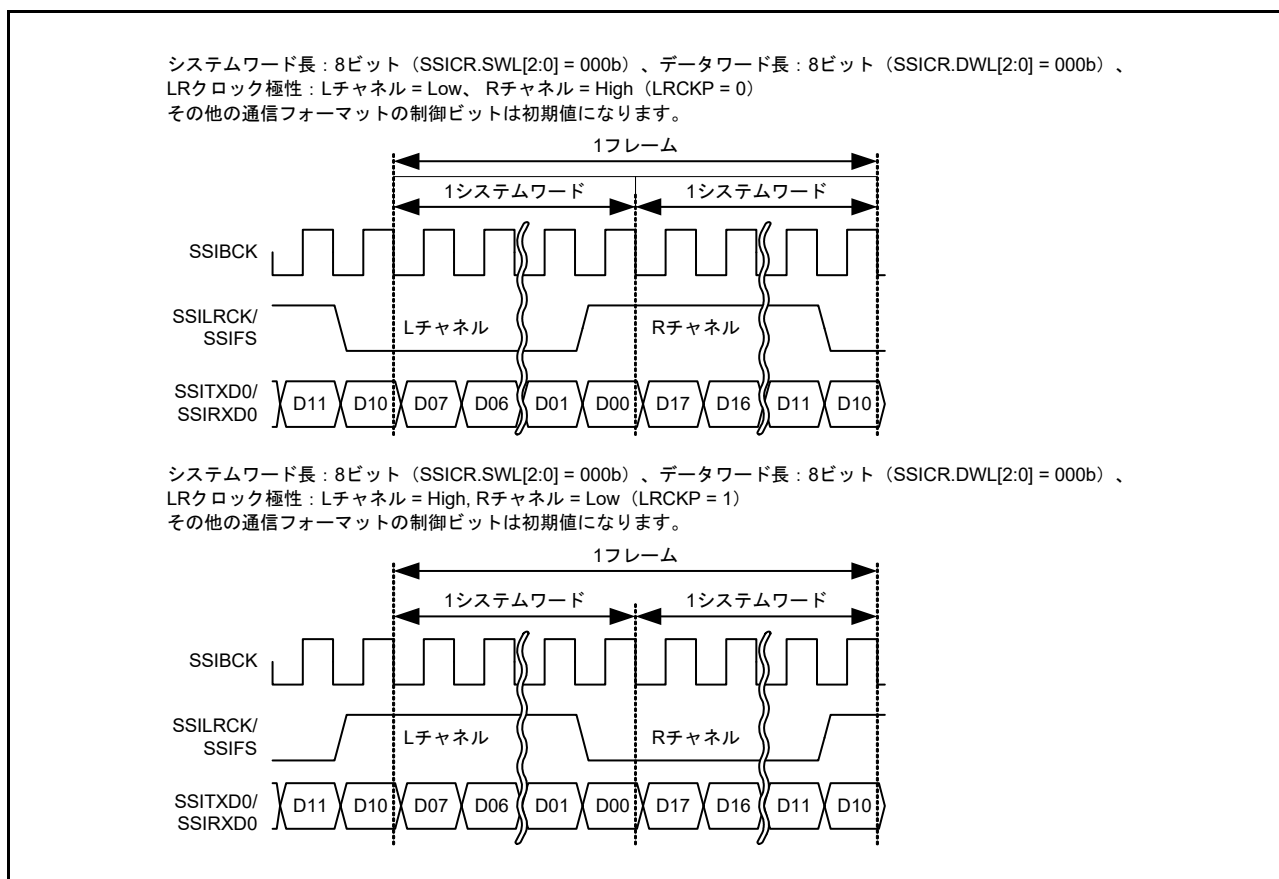
図 37.11 LR クロック/フレーム同期極性設定
