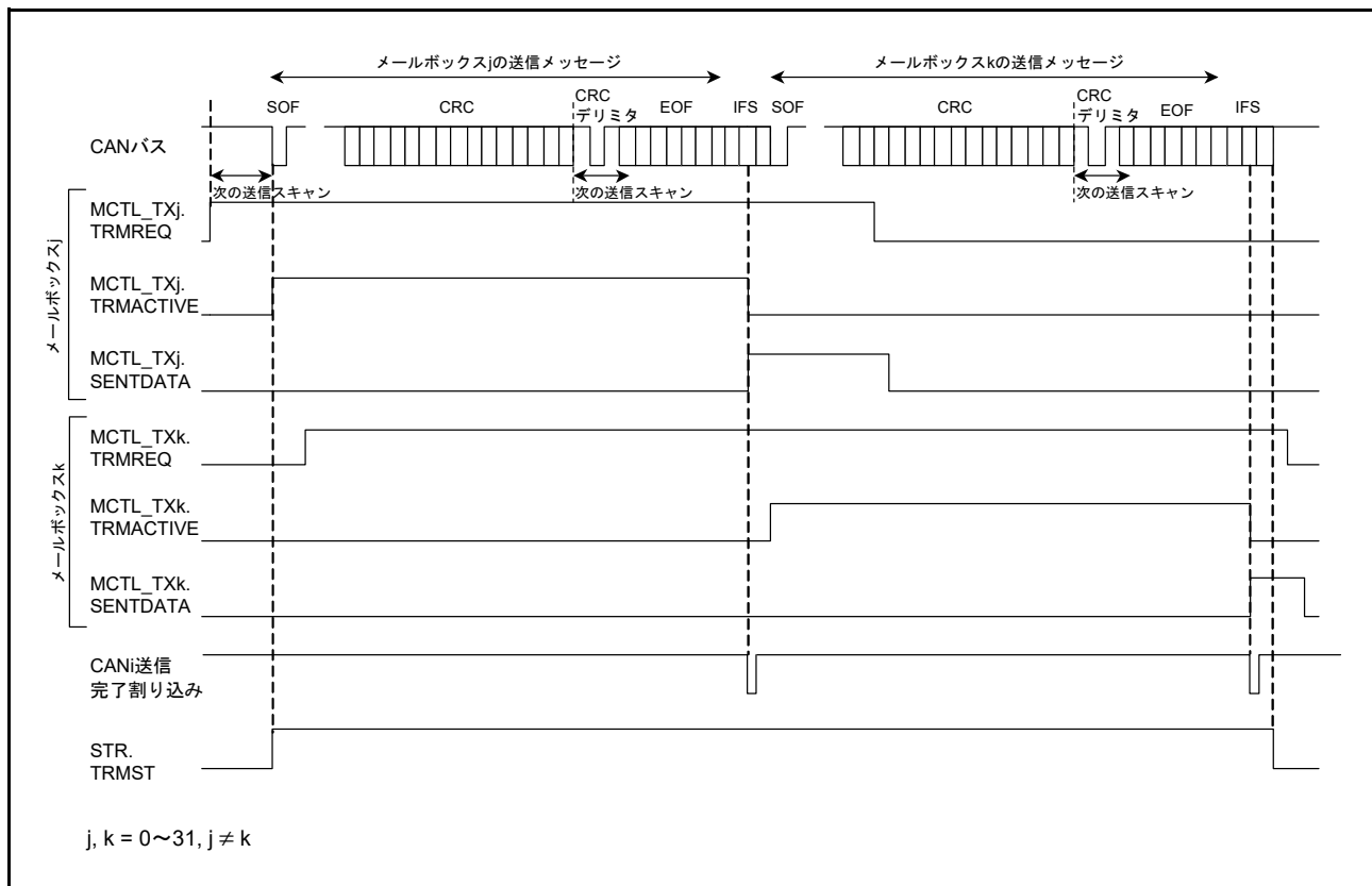
図 33.20 データフレーム送信時の動作例
