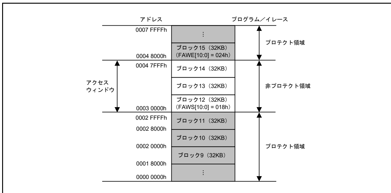
図 50.10 アクセスウィンドウに 32KB のブロックのみ含まれる場合のアクセスウィンドウの開始ブロックアドレス (FAWS) と終了ブロックアドレス (FAWE)
