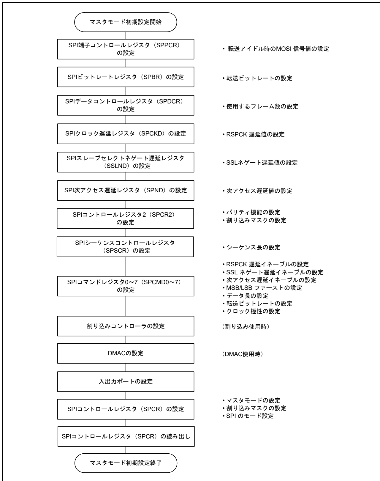
図 34.47 マスタモード時のクロック同期式動作の初期化フロー例
