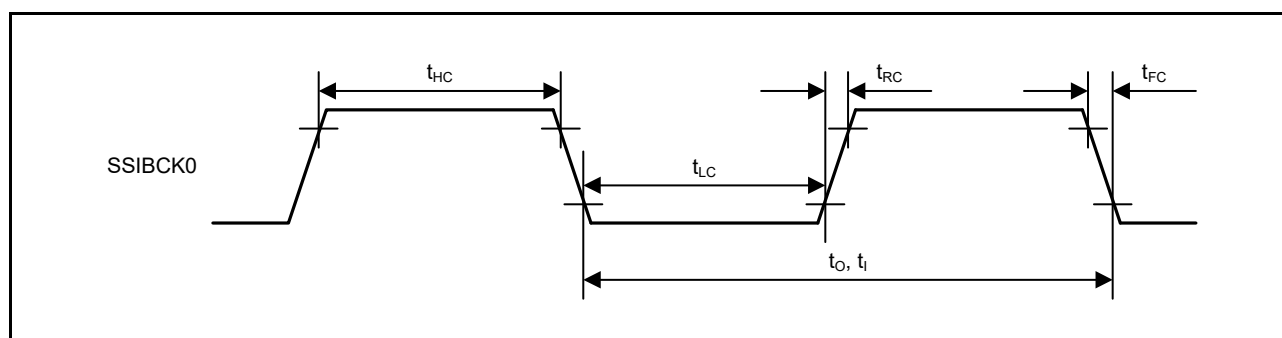
図 52.54 SSIE クロック入出力タイミング
