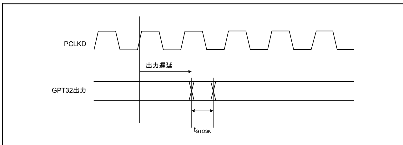
図 52.31 OPS の GPT32 出力遅延スキュー
