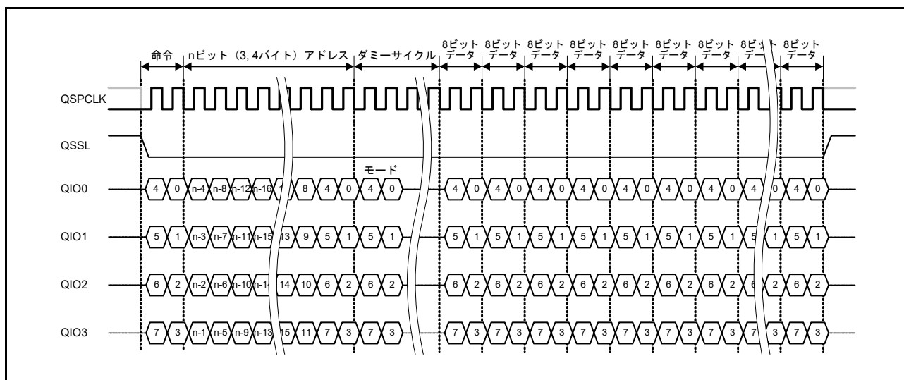
図 35.7 Quad-SPI プロトコル例 (ファストリード Quad I/O)
