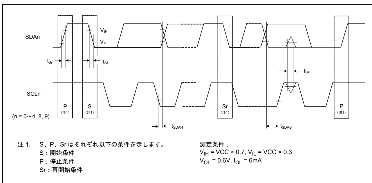
図 52.43 SCI 簡易 IIC モード タイミング
