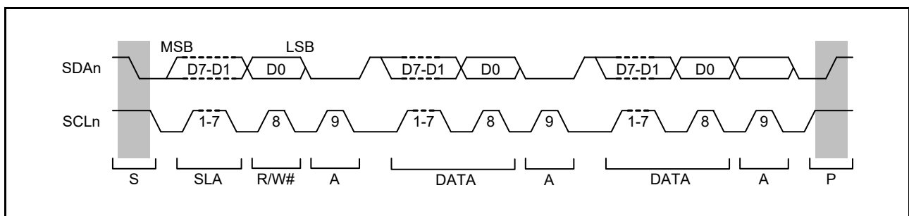
図 30.59 I 2 C バスタイミング (SLA = 7 ビットの場合)
