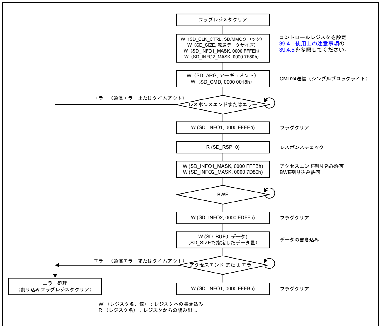
図 39.11 シングルブロックライト動作の例
