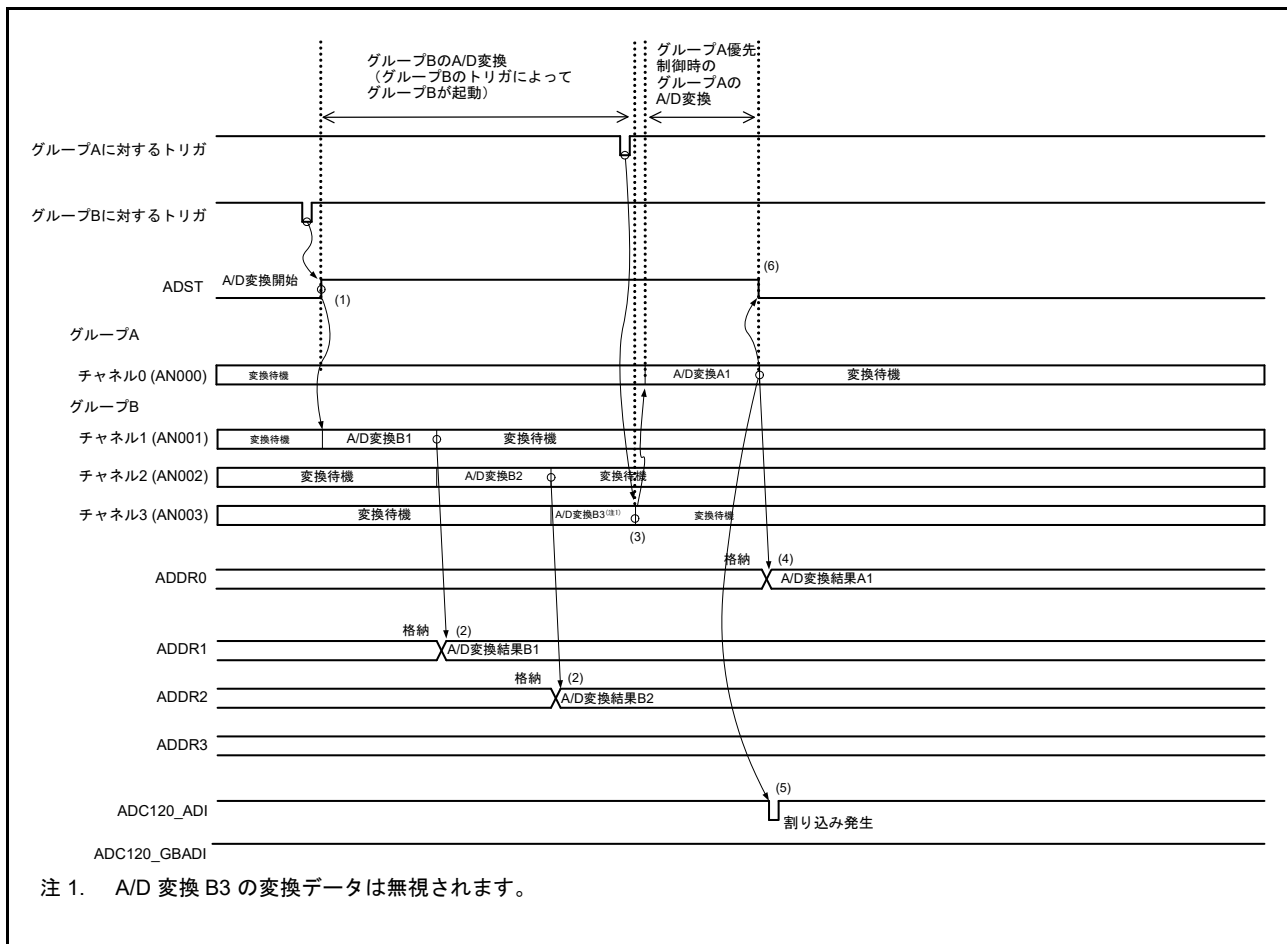
図 42.29 グループ A 優先制御の動作例 (4) (ADGSPCR.GBRSCN = 0、ADGSPCR.GBRP = 0 の場合)
