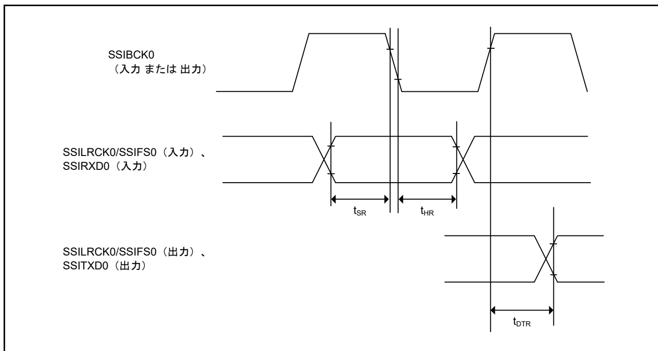
図 52.57 SSICR.BCKP = 1 の場合の SSIE データ送受信タイミング
