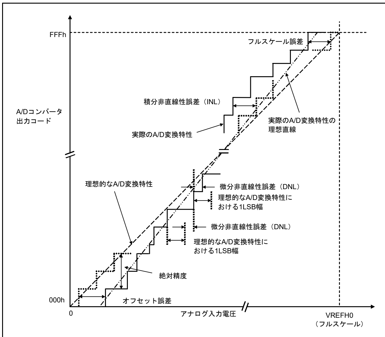
図 52.64 ADC12 特性用語の解説図
