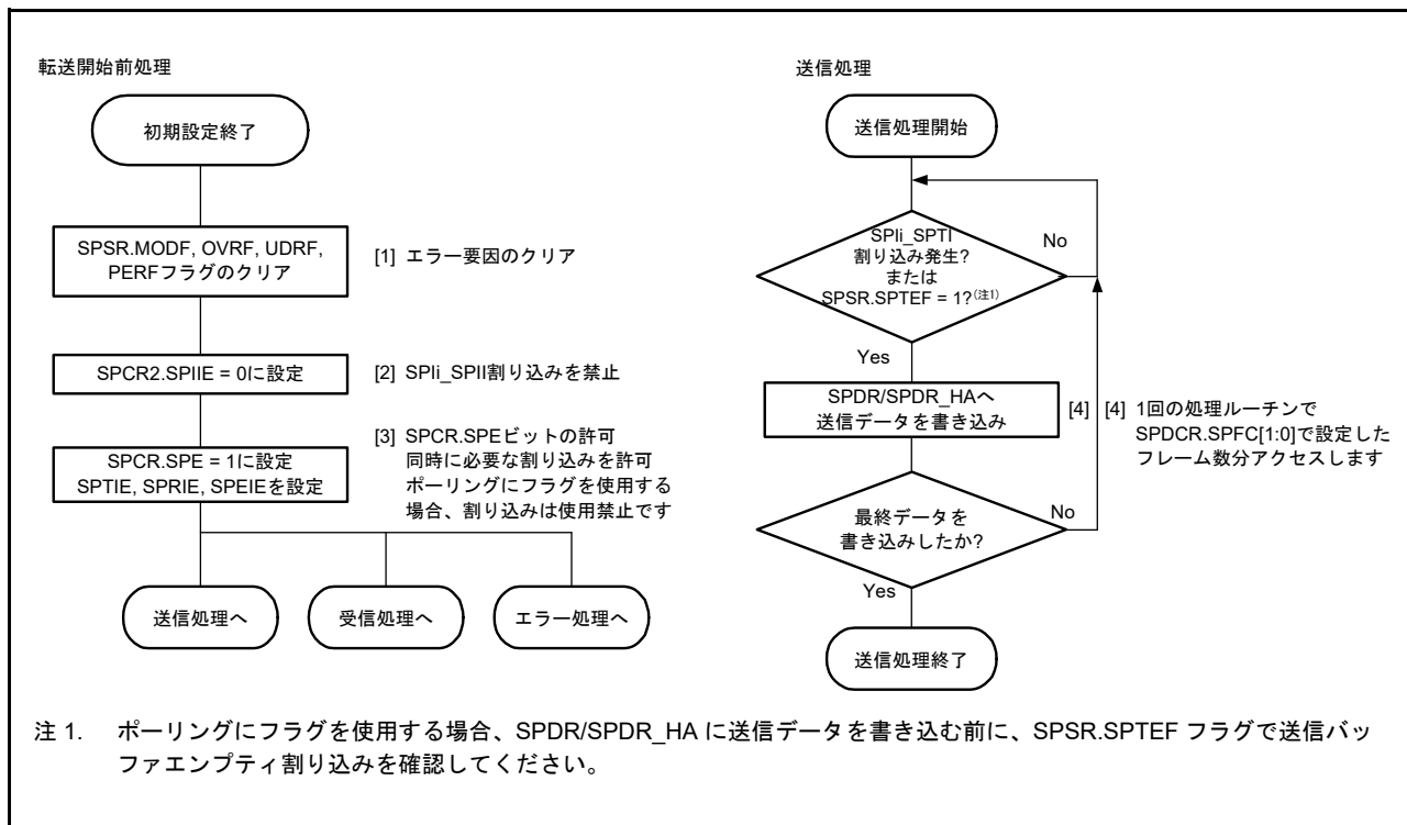
図 34.41 スレーブモードでの送信フロー
