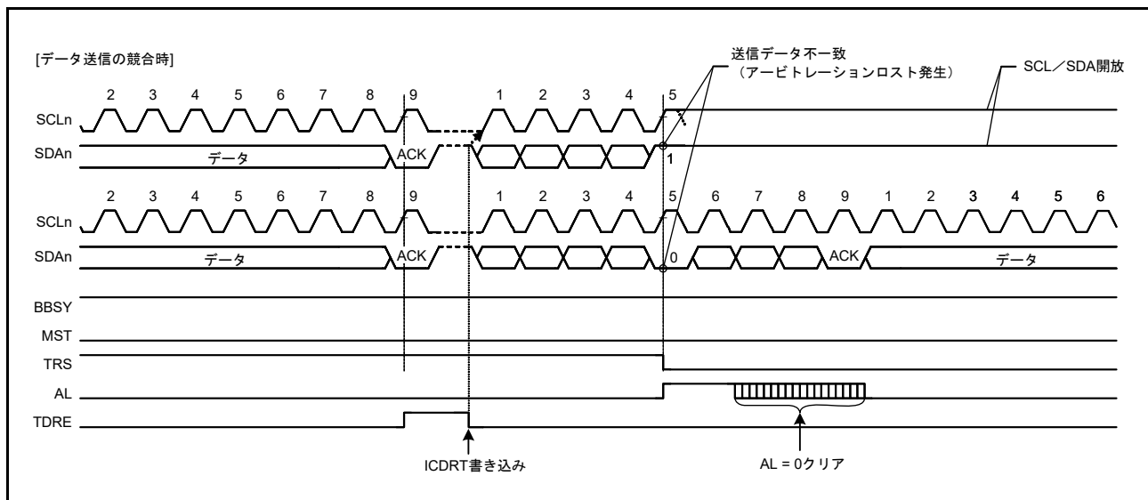
図 32.44 スレーブアービトレーションロスト検出の動作例 (SALE = 1 の場合)
