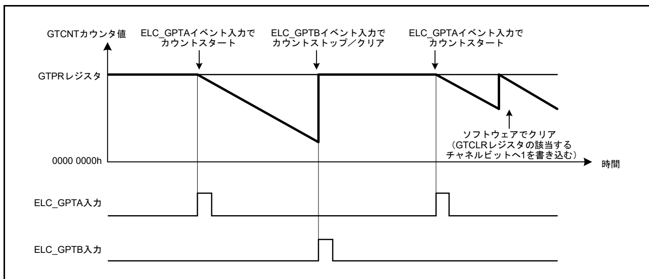
図 23.58 ハードウェア要因によるカウンタクリア動作例 (のこぎり波ダウンカウント、ELC_GPTA イベント入力でスタート、ELC_GPTB イベント入力でストップ/クリアの場合)
