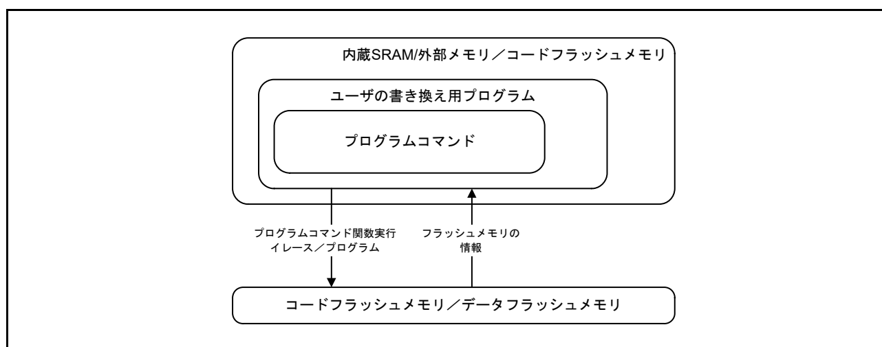
図 50.15 セルフプログラミングの概念
