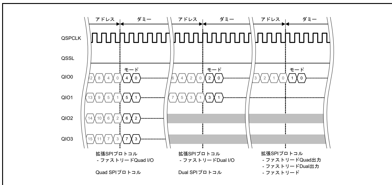
図 35.32 XIP モード制御データ
