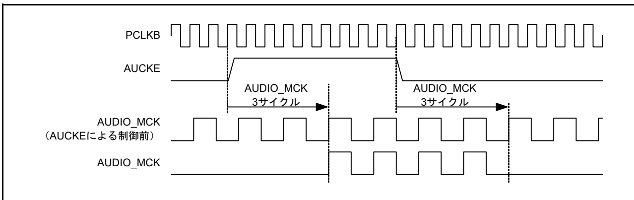
図 37.24 AUDIO_MCK の停止/再開
