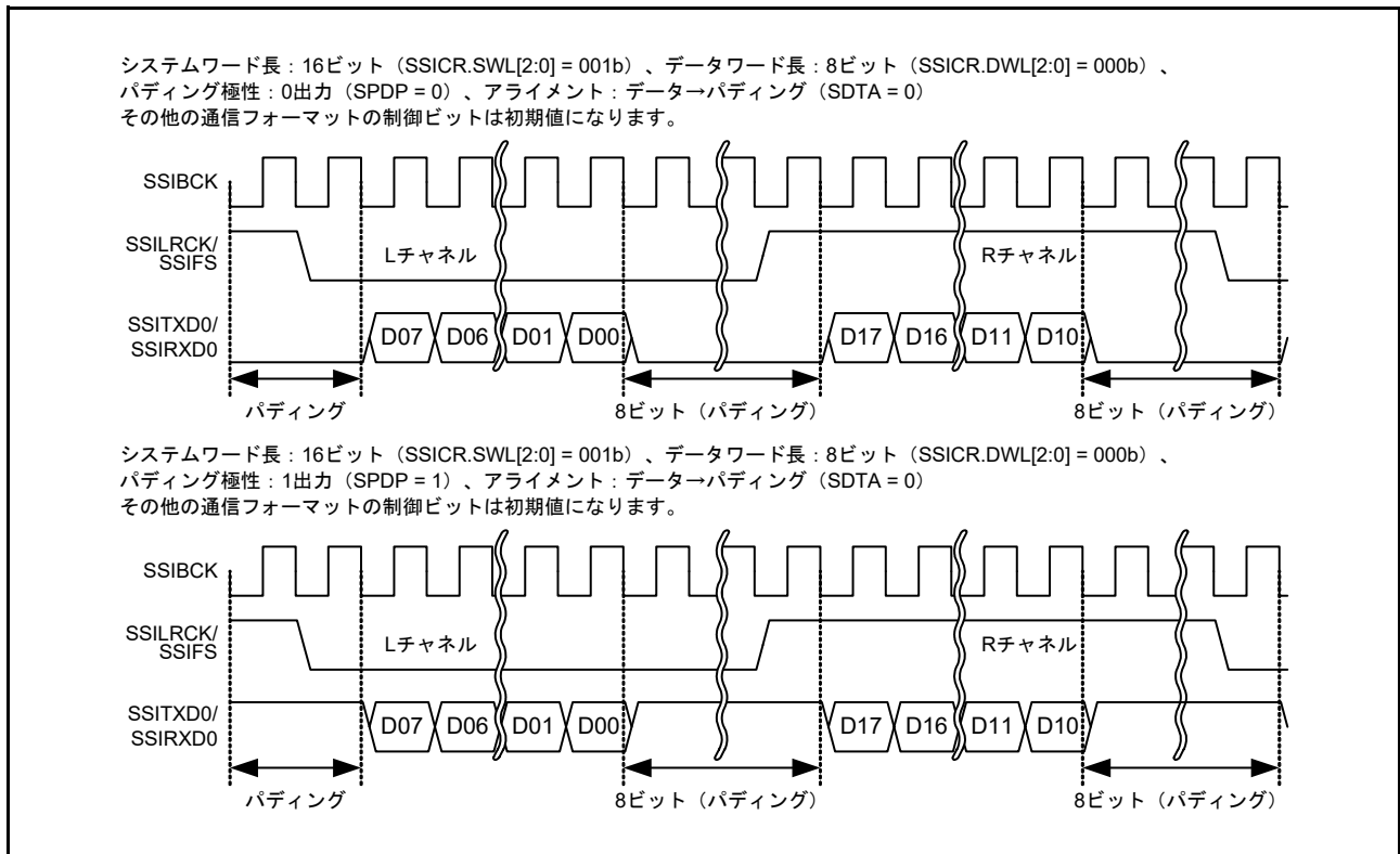
図 37.10 パディングビット極性
