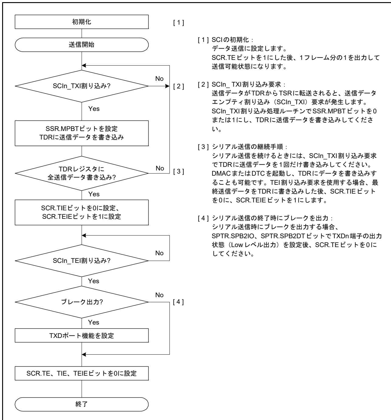
図 30.23 マルチプロセッサシリアル送信のフローチャート例 (非 FIFO 選択時)
