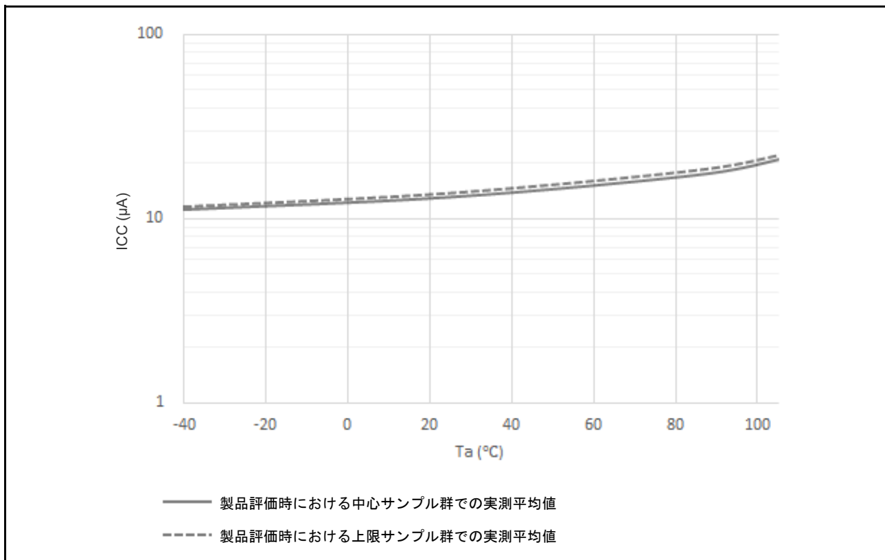
図 52.4 ディープソフトウェアスタンバイモード時の温度依存性：SRAM および USB レジューム検出部への電源供給なし、パワーオンリセット回路の低消費電力機能無効（参考データ）
