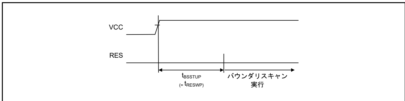
図 52.74 バウンダリスキャン回路起動タイミング
