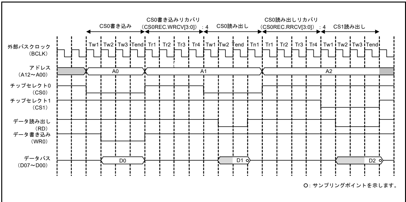
図 15.29 セパレートバスインタフェース時のリカバリサイクルの挿入例
