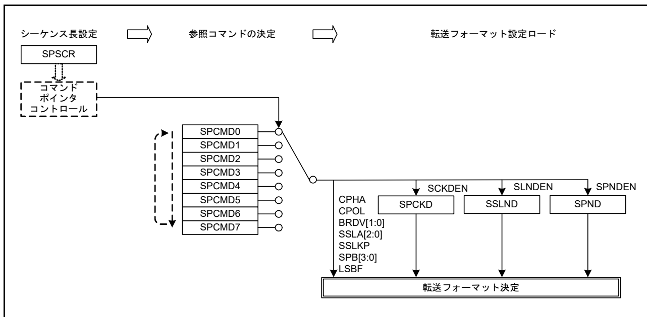
図 34.32 マスタモードでのシリアル転送方式の決定方法
