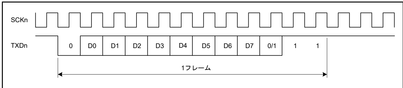
図 30.4 出力クロックと送信データの位相関係 (調歩同期式モード: SMR.CHR = 0、PE = 1、MP = 0、STOP = 1)
