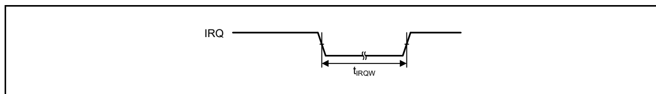
図 52.19 IRQ 割り込み入力タイミング
