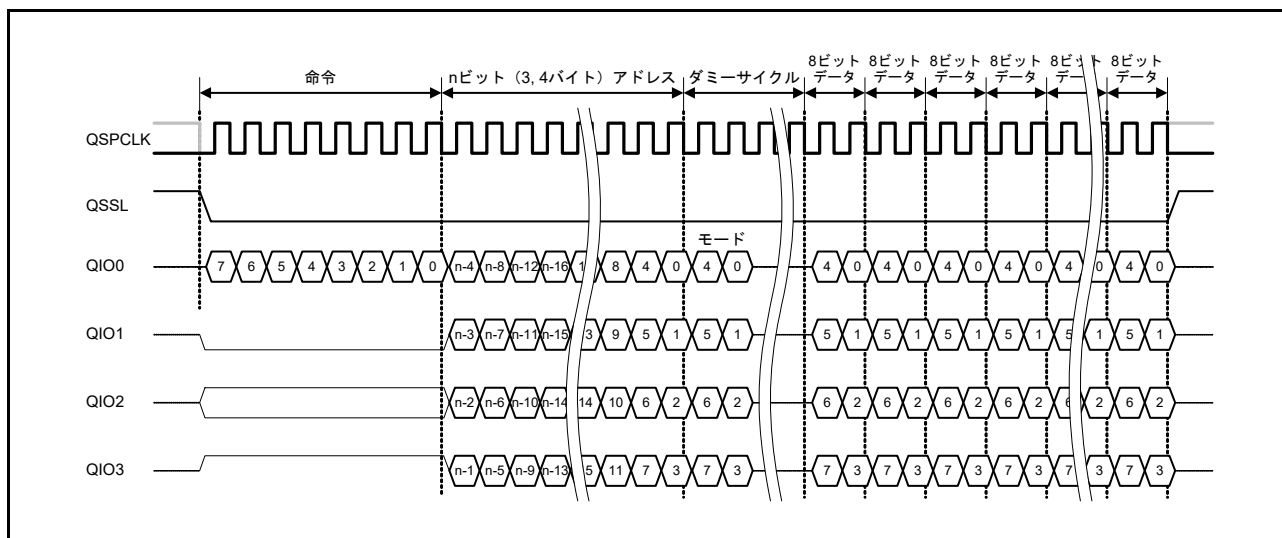
図 35.5 拡張 SPI プロトコル例 2 (ファストリード Quad I/O)
