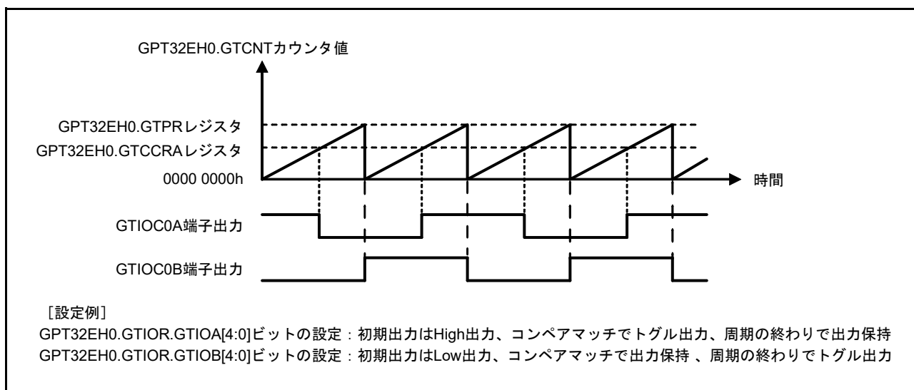
図 23.14 トグル出力動作例 (2)
