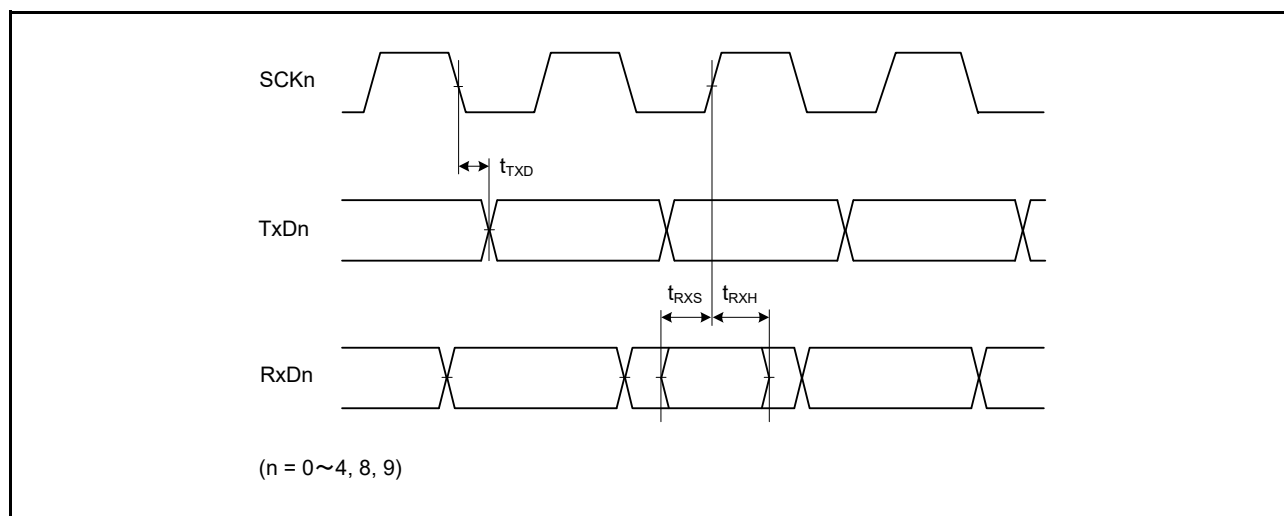
図 52.37 クロック同期式モードにおける SCI 入出力タイミング
