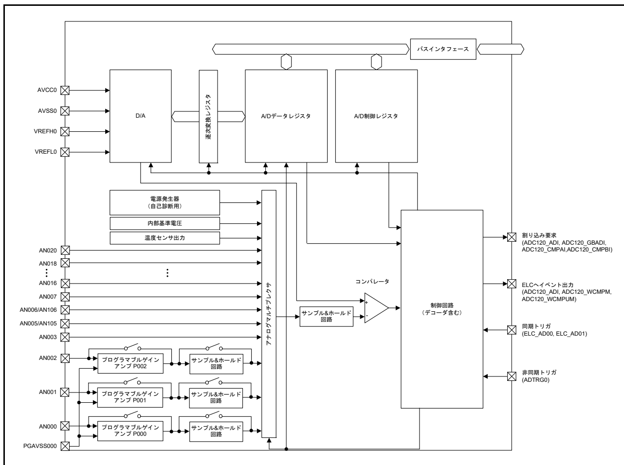
図 42.1 ADC12 (ユニット 0) のブロック図
