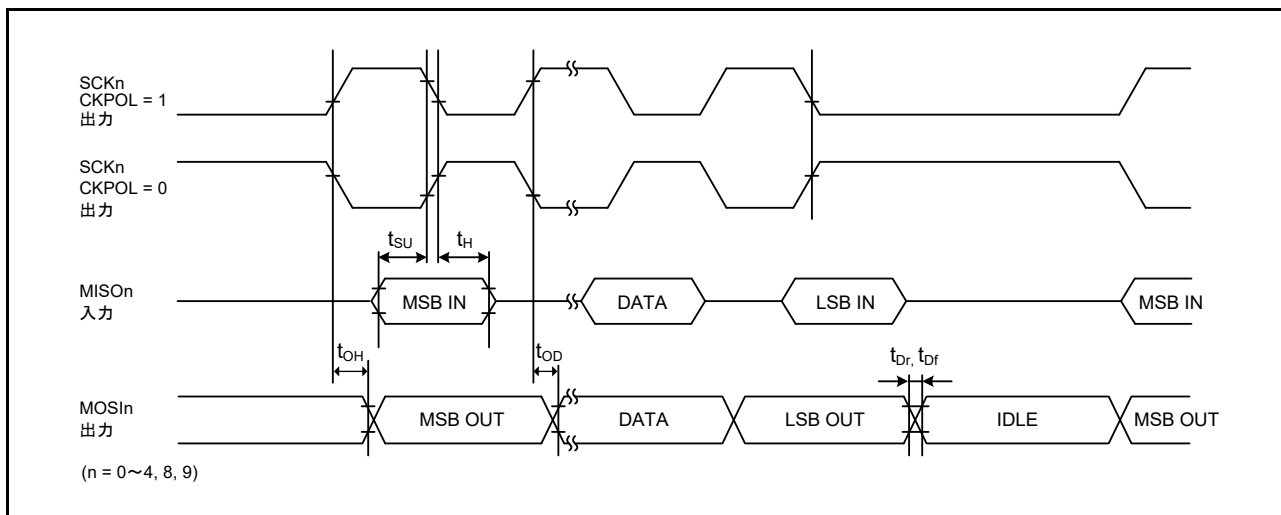
図 52.40 CKPH = 0 の場合におけるマスタの SCI 簡易 SPI モードタイミング
