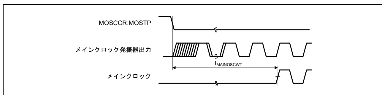
図 52.9 メインクロック発振開始タイミング
