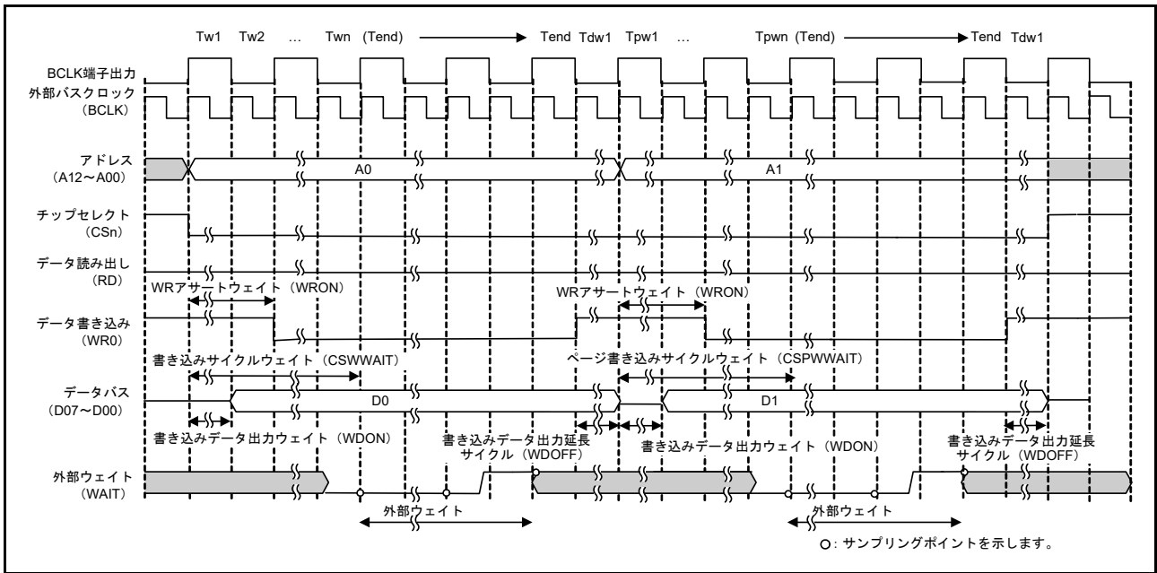
図 15.27 外部ウェイトタイミング例 (バイトストローブモード時の 8 ビットバス空間に対するページライトアクセス、BCLK 端子出力選択ビットで BCLK の 2 分周を選択した場合) (n = 0, 1, 4 ~ 7)
