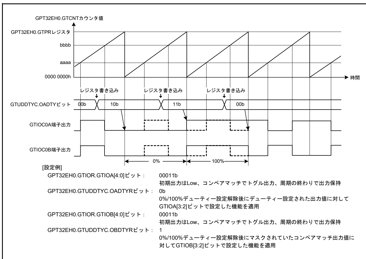
図 23.50 出力デューティ 0%、100% 機能動作例
