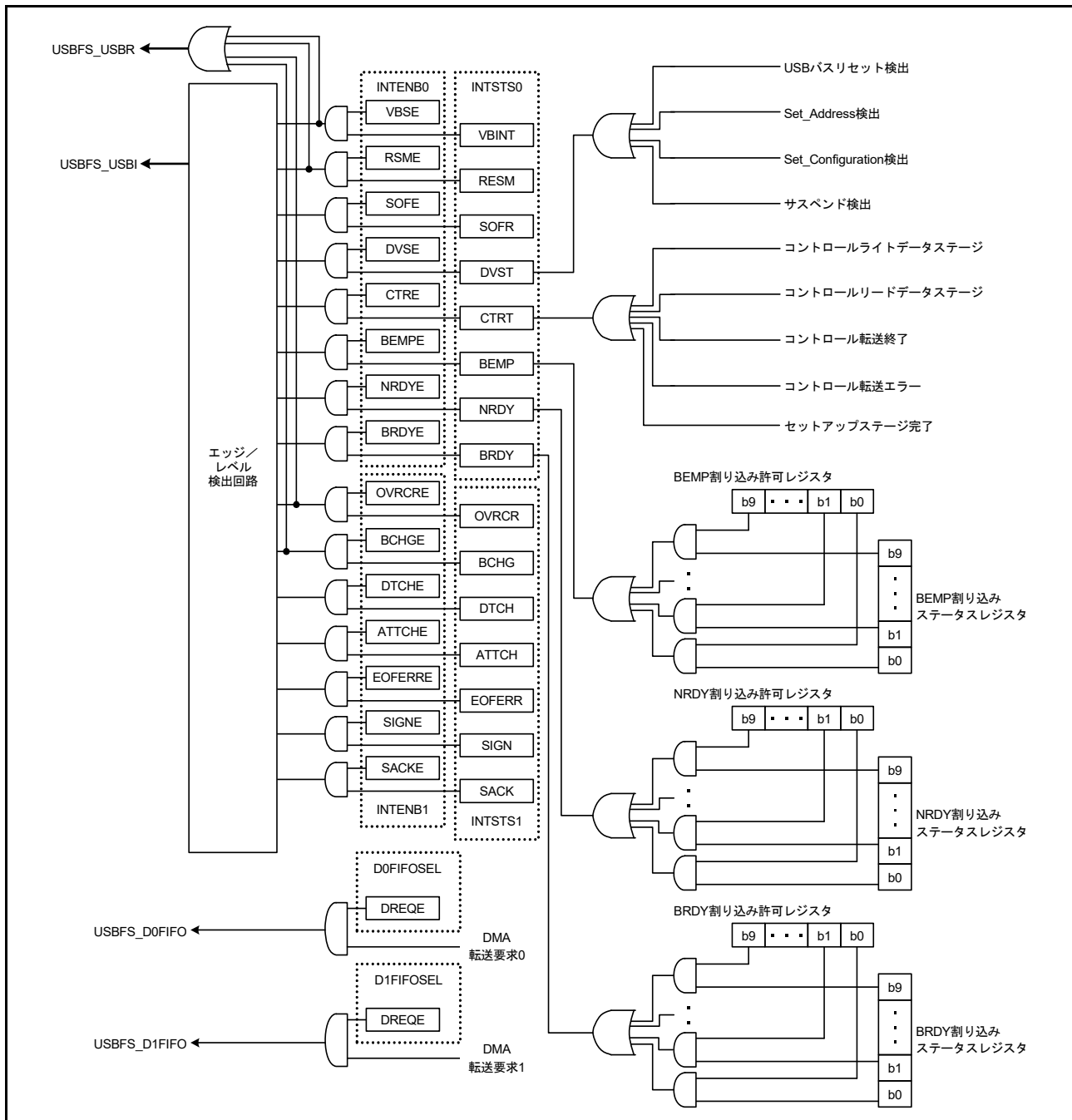
図 29.10 USBFS 割り込みに関連する回路
