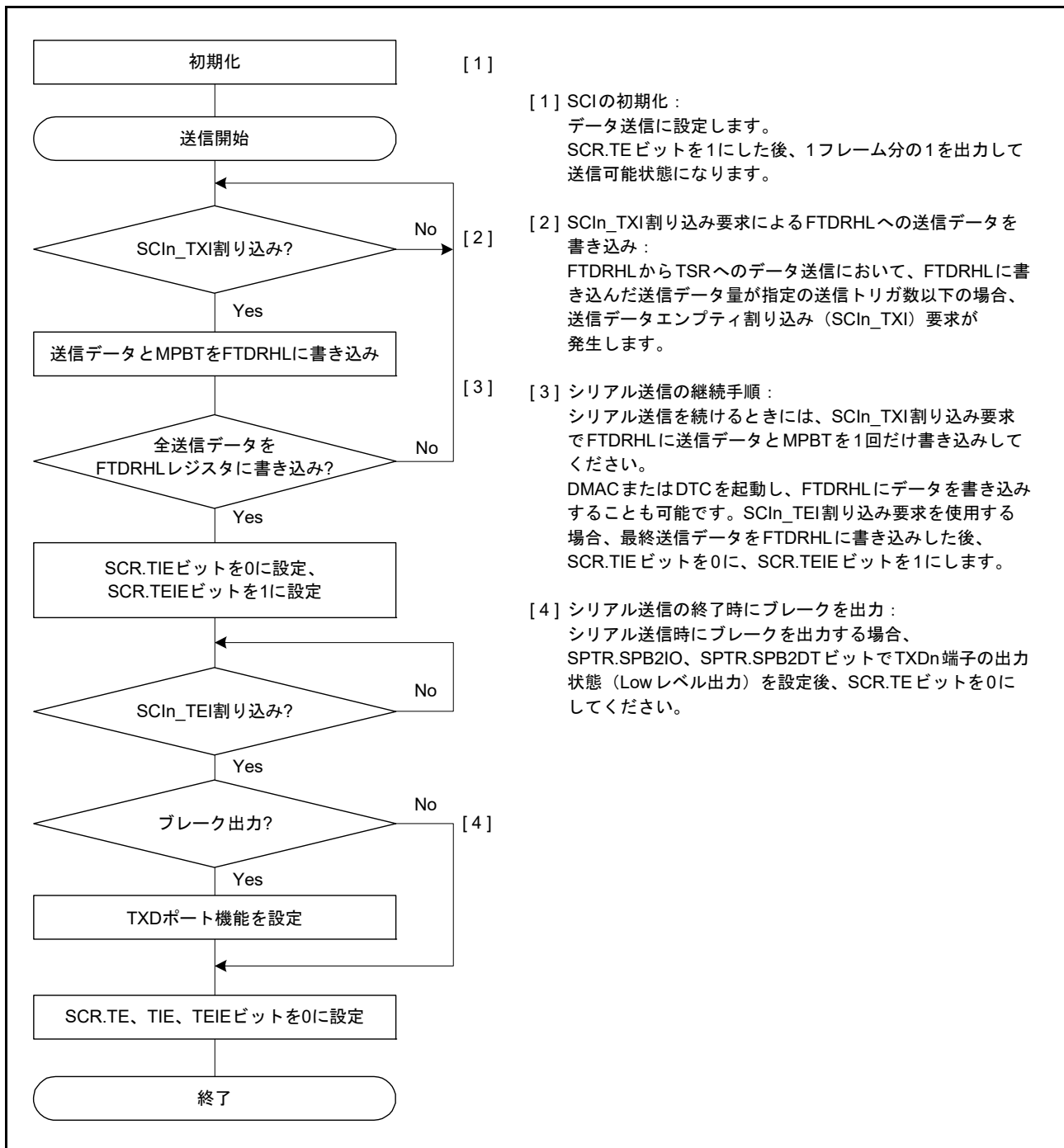
図 30.25 マルチプロセッサモードにおけるシリアル送信のフローチャート例 (FIFO 選択時)
