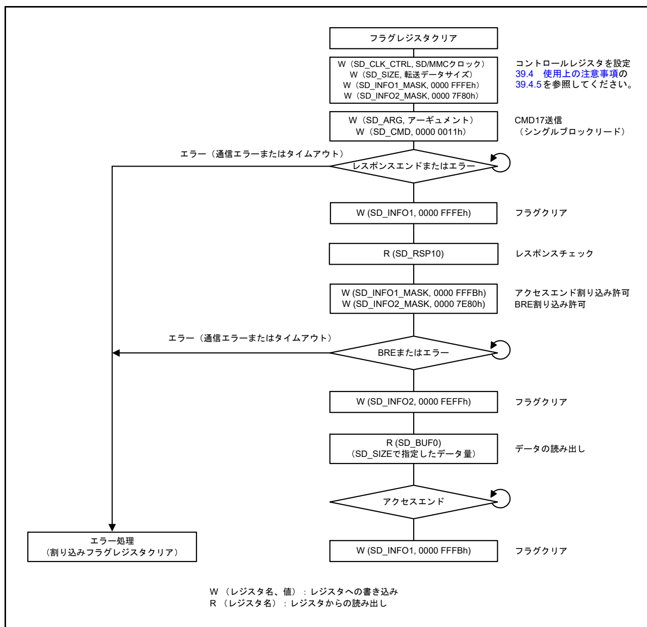
図 39.10 シングルブロックリード動作のフロー例
