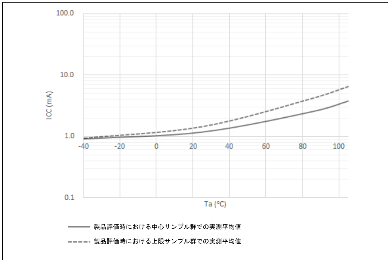
図 52.2 ソフトウェアスタンバイモード時の温度依存性 (参考データ)
