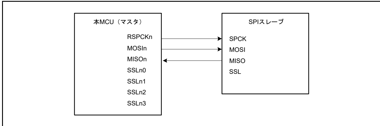
図 34.11 クロック同期式動作のマスター/スレーブの構成例 (MCU はマスター)
