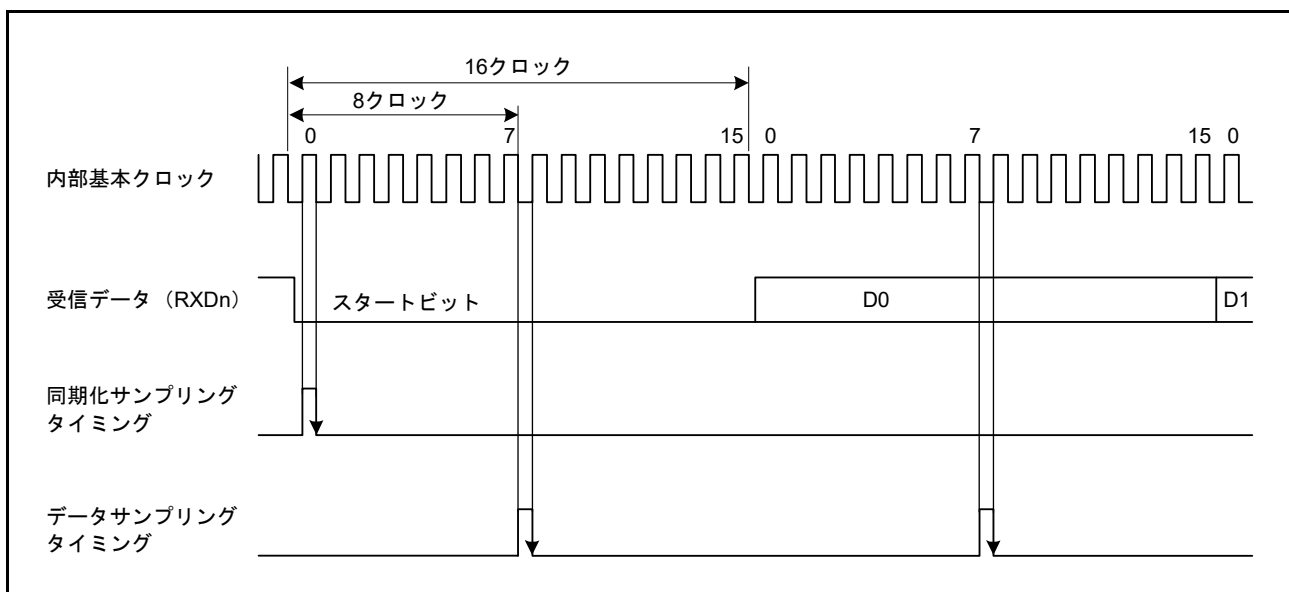
図 30.3 調歩同期式モードでの受信データのサンプリングタイミング
