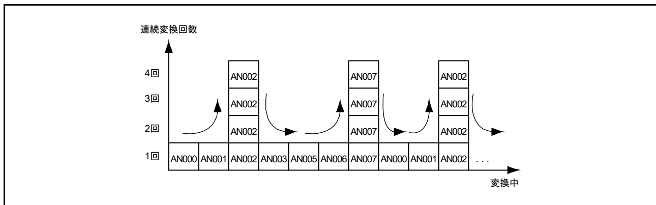
図 42.3 ADADC.ADC[2:0] = 011b、ADADS0.ADS02 = 1、ADADS0.ADS07 = 1 選択時のスキャン変換シーケンス
