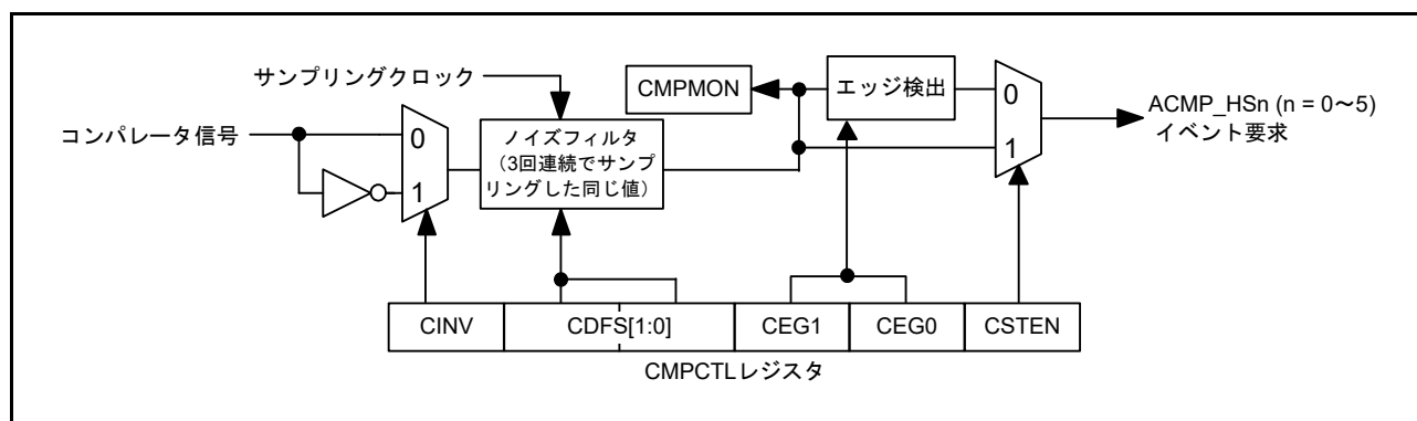
図 45.3 ノイズフィルタおよびエッジ検出の構成
