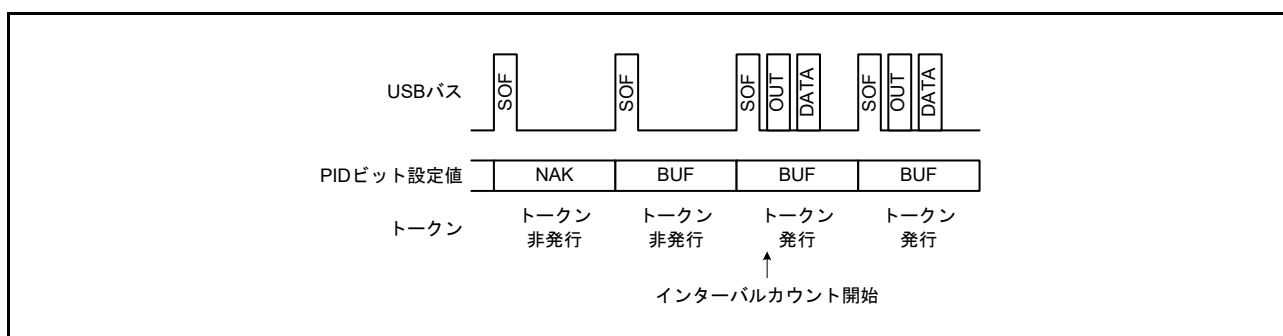
図 29.16 IITV = 0 の場合のトークン発行の有無
