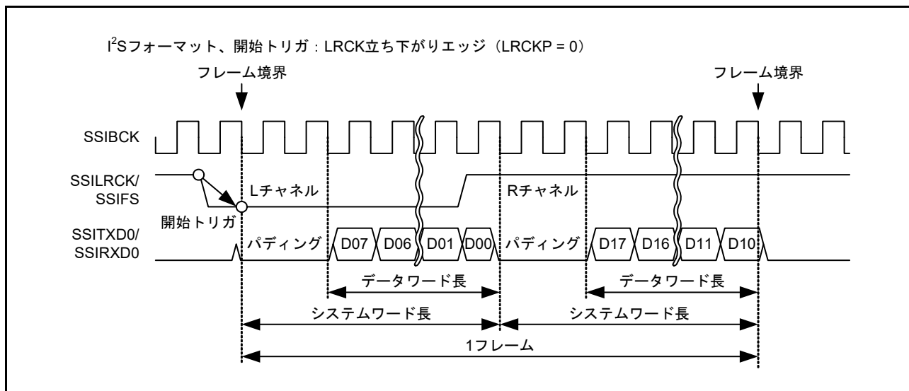
図 37.1 SSIE 通信フォーマット
