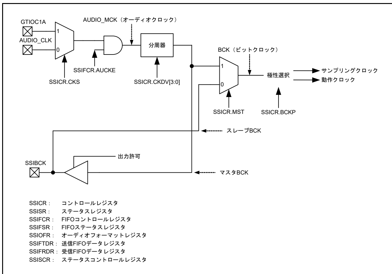
図 37.3 SSIE クロック構成
