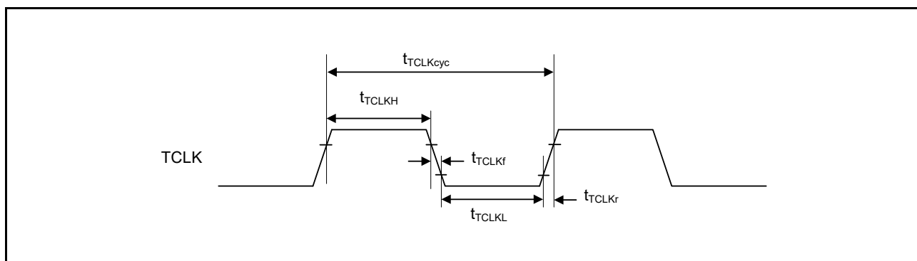
図 52.79 ETM TCLK タイミング
