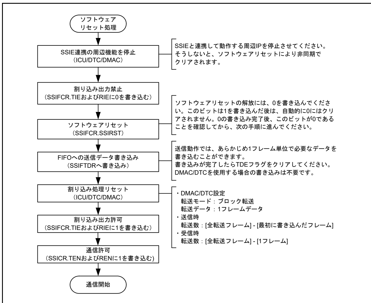
図 37.60 ソフトウェアリセット手順 (CPU 動作手順)
