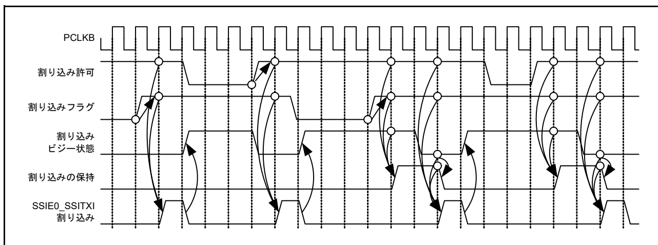
図 37.59 SSIE0_SSITXI 割り込みのタイミング図
