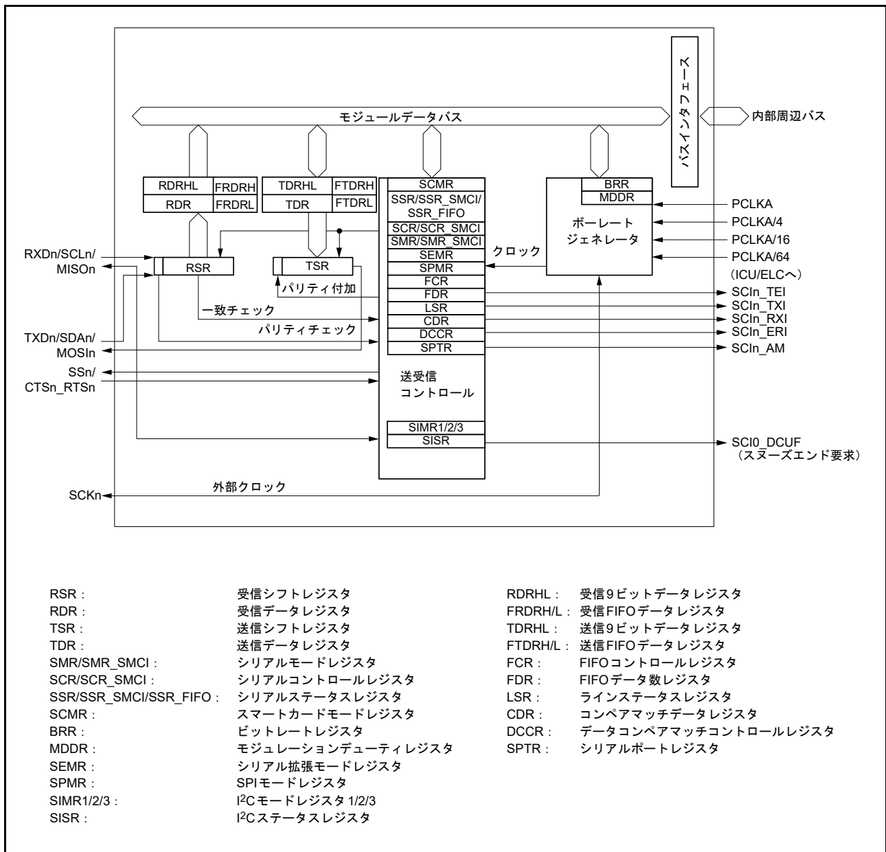
図 30.1 SCI チャンネル n のブロック図
