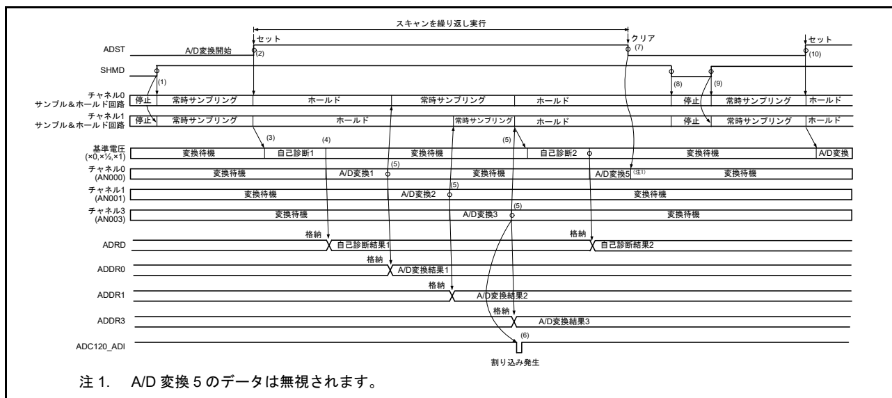
図 42.21 連続スキャンモードの動作例 (チャンネル専用サンプル&ホールド回路使用、AN000、AN001、および AN003 選択 + 自己診断、常時サンプリング有効)
