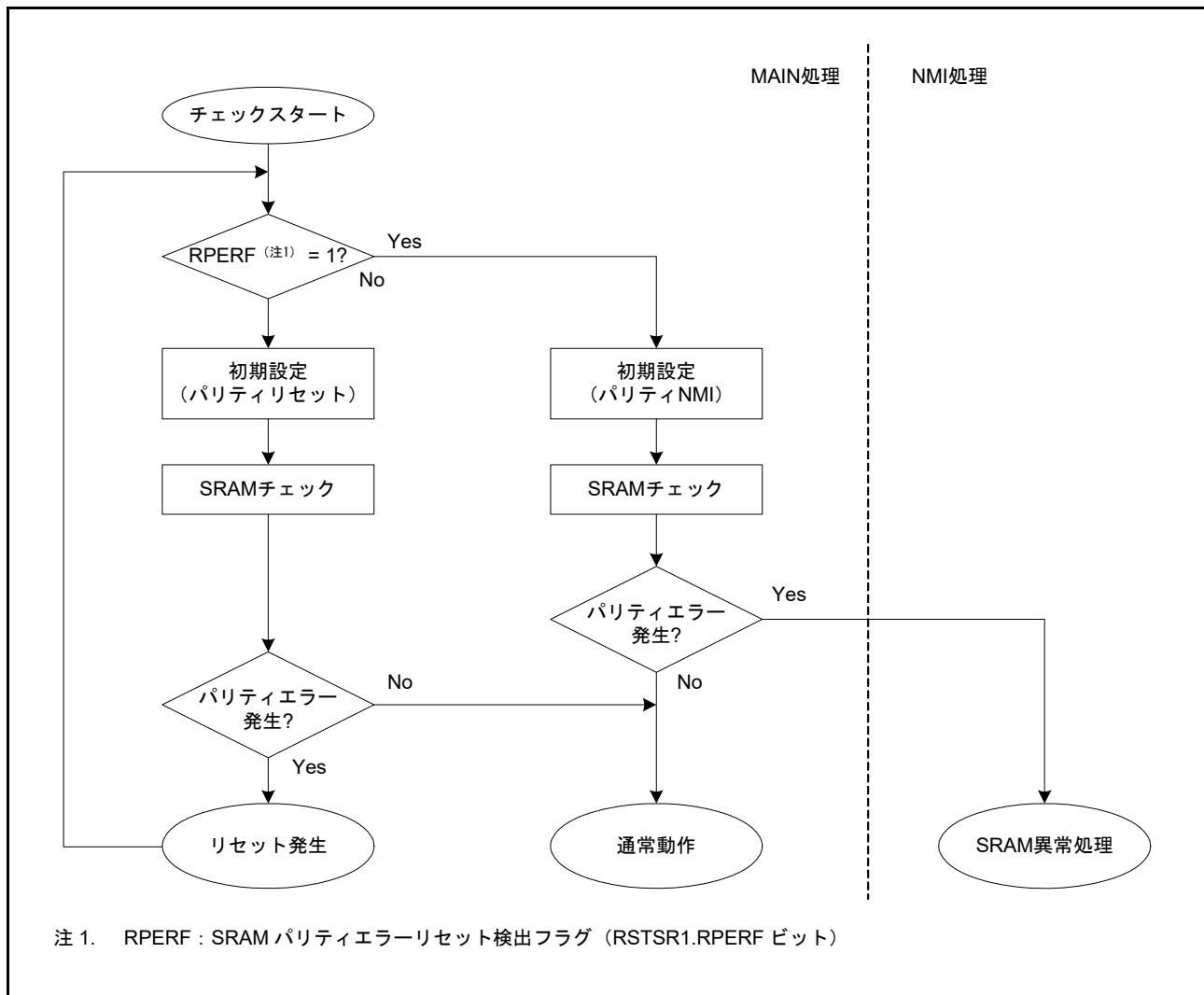
図 48.2 SRAM パリティリセット許可の場合の SRAM パリティチェックのフロー
