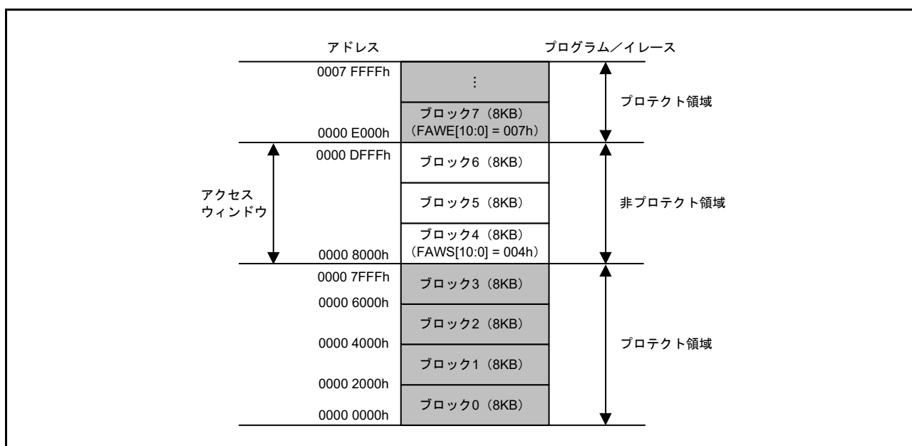
図 50.8 アクセスウィンドウに 8KB のブロックのみ含まれる場合のアクセスウィンドウの開始ブロックアドレス (FAWS) と終了ブロックアドレス (FAWE)
