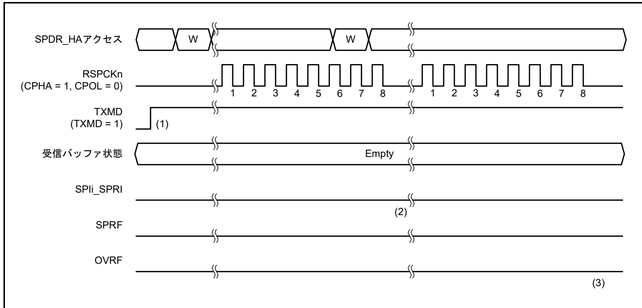
図 34.25 SPCR.TXMD = 1 の動作例
