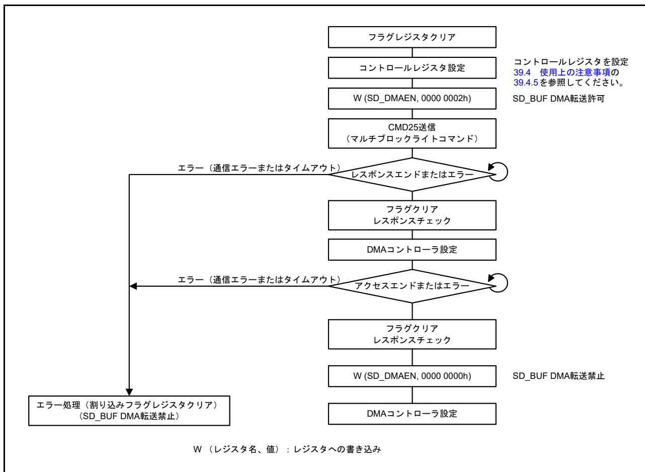
図 39.23 SD_BUF_DMA ライト動作の例
