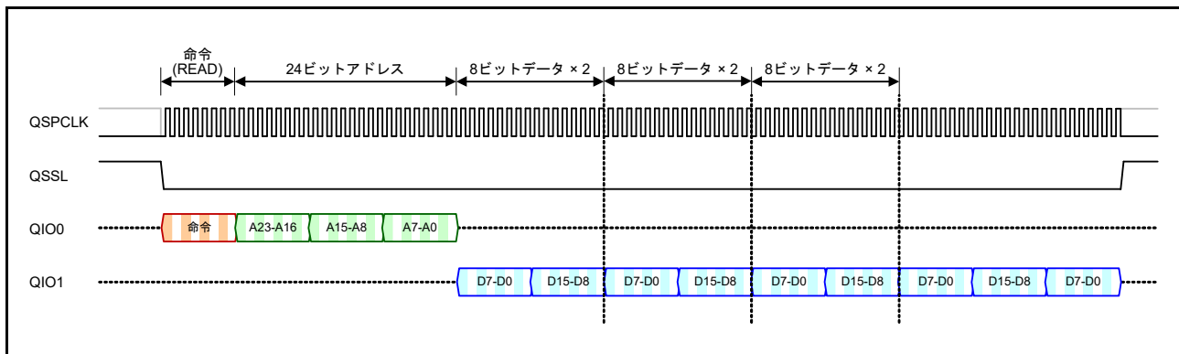
図 35.30 プリフェッチ機能を使用した連続データのリード動作
