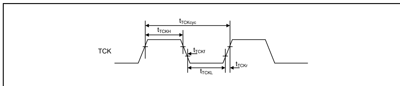
図 52.72 バウンダリスキャン TCK タイミング
