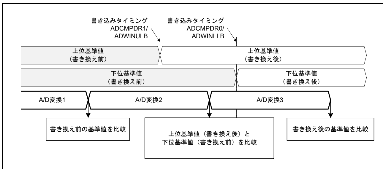
図 42.5 書き換え前後の上側基準値と下側基準値の比較
