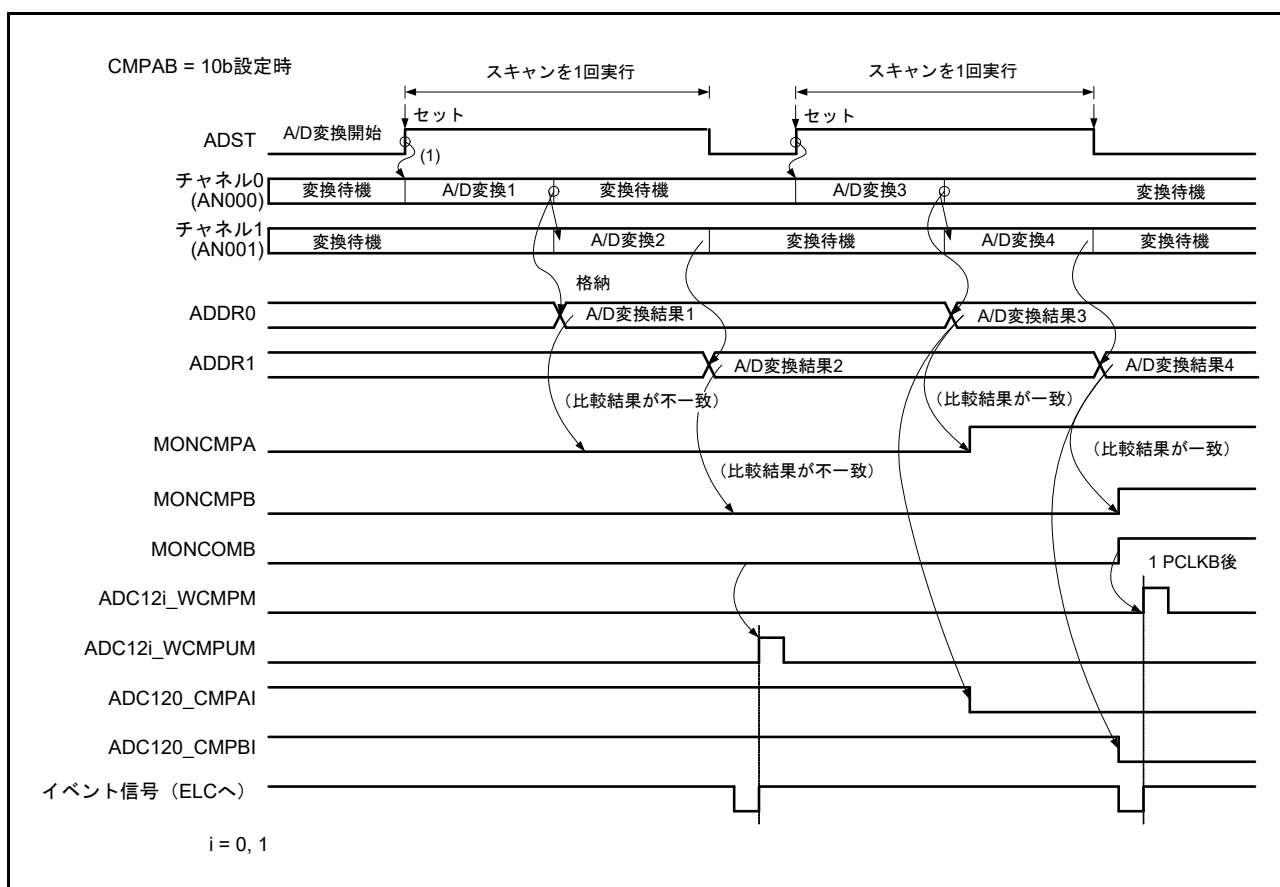
図 42.33 コンペア機能のイベント出力動作例 (AN000 ~ AN001 を比較)
