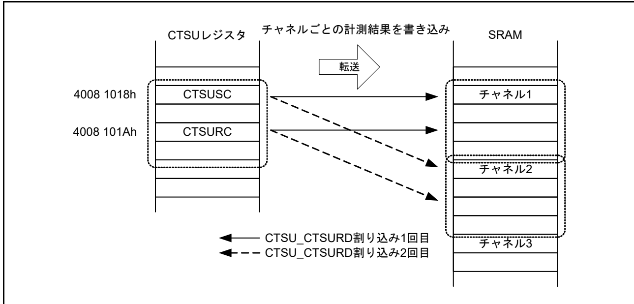
図 46.20 CTSU_CTSURD 割り込みを用いた DTC 転送動作例
