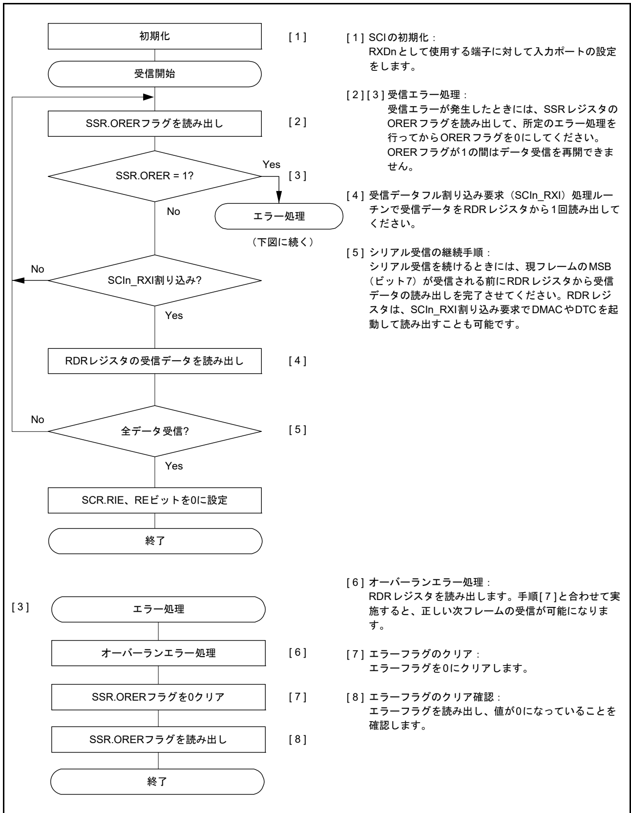
図 30.41 クロック同期式モードにおけるシリアル受信のフローチャート例 (非 FIFO 選択時)
