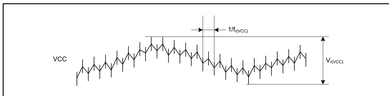
図 52.6 リップル波形
