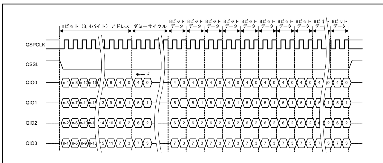
図 35.25 XIP モード時のファストリード Quad I/O バスサイクル
