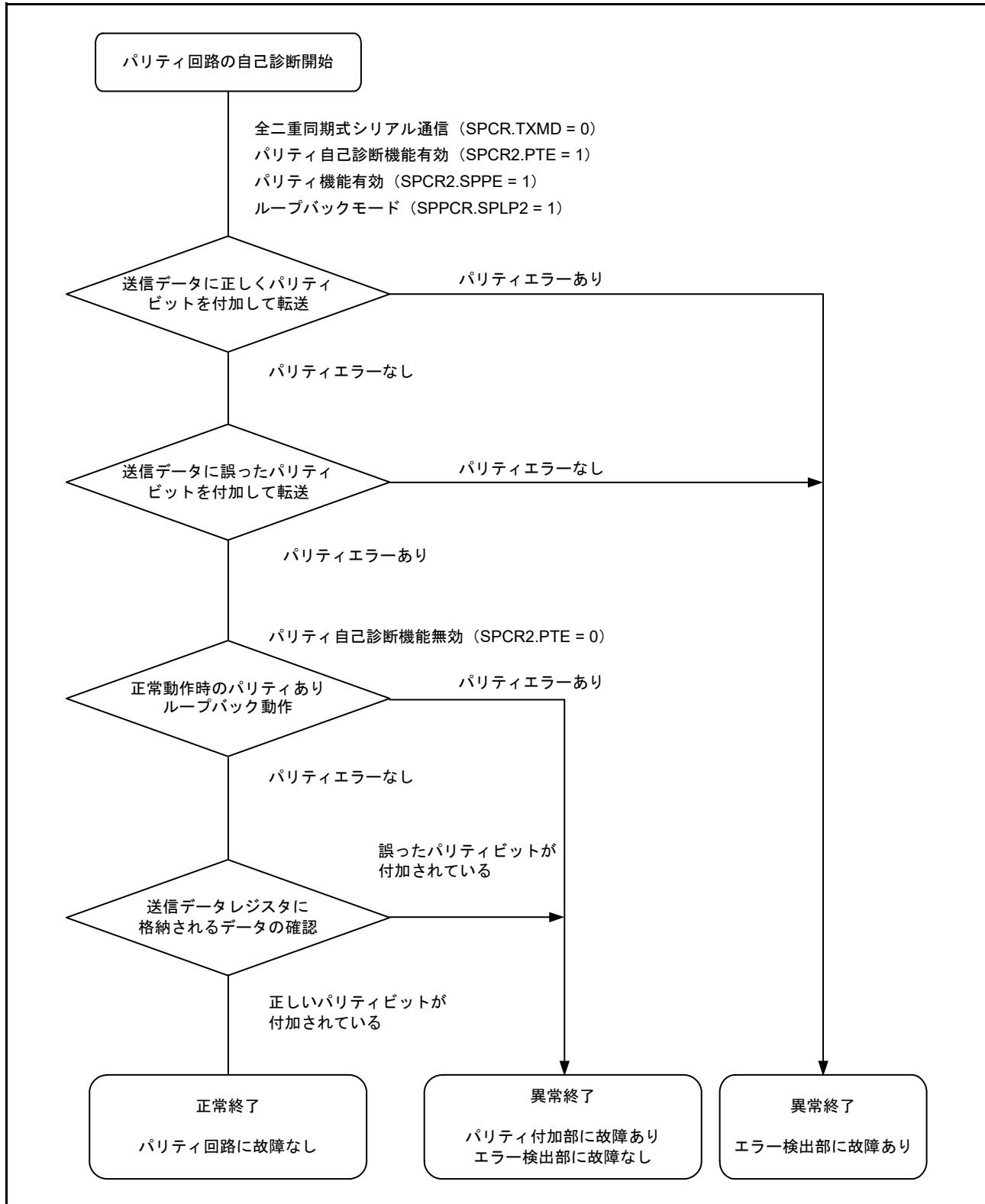
図 34.50 パリティ回路の自己診断フロー
