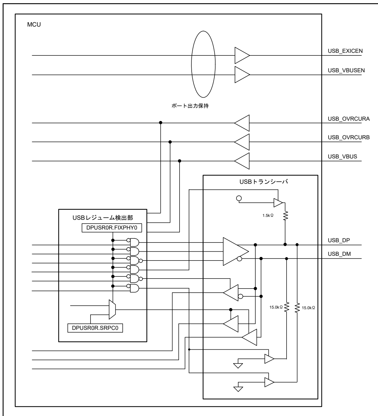
図 29.6 USB レジューム検出部と USB 用の入出力端子の接続
