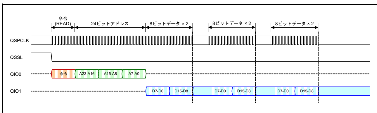
図 35.31 SPI バスサイクル拡張を使用した連続データのリード動作
