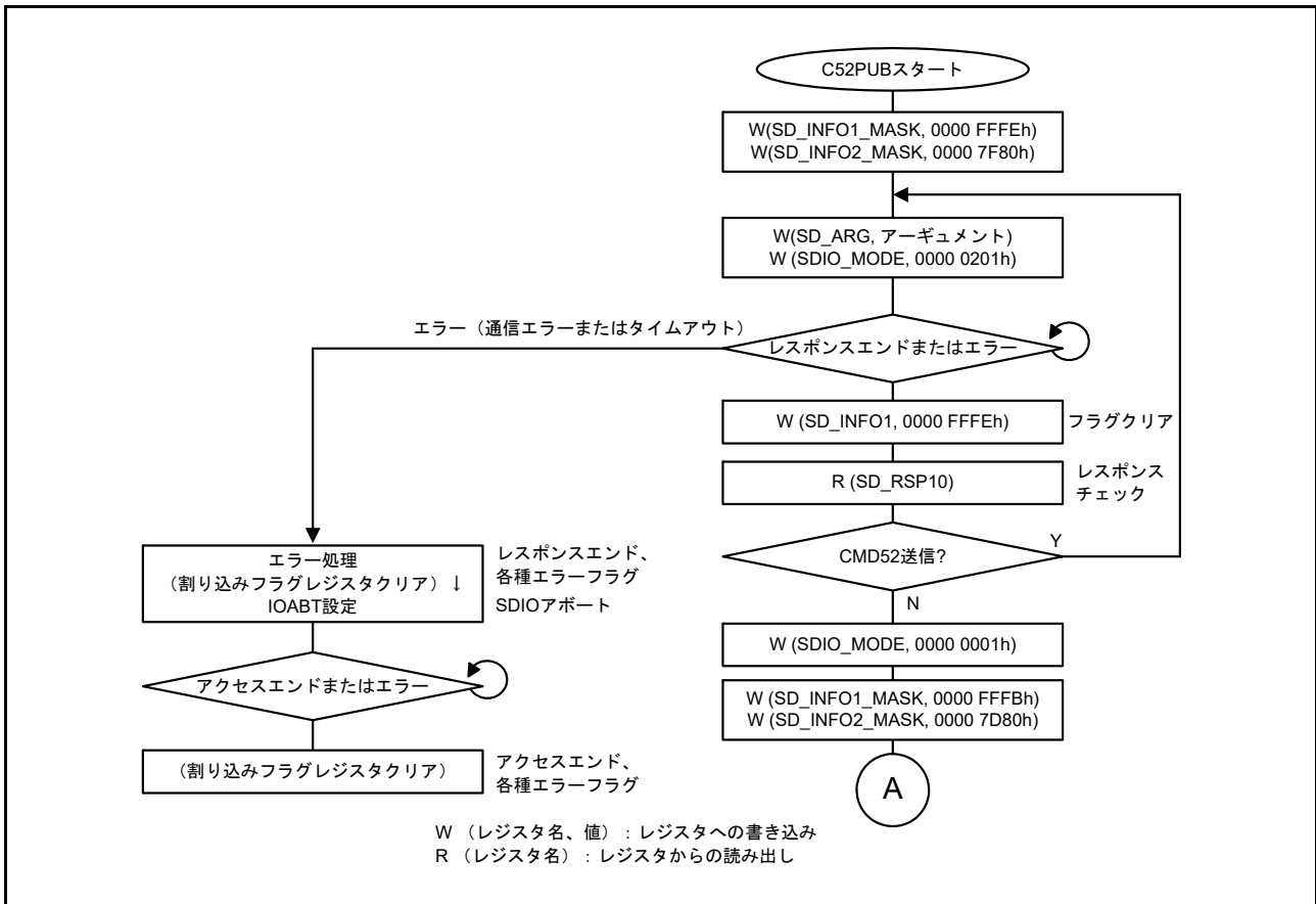
図 39.21 CMD53 マルチブロックライト時に CMD52 (SDIO none abort) が送信される場合のフロー
