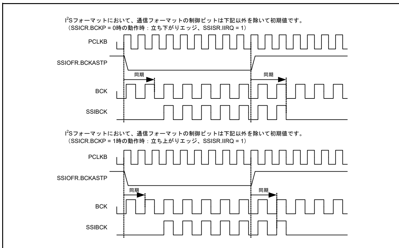
図 37.44 SSIOFR.BCKASTP ビットによる SSIBCK 出力の停止例
