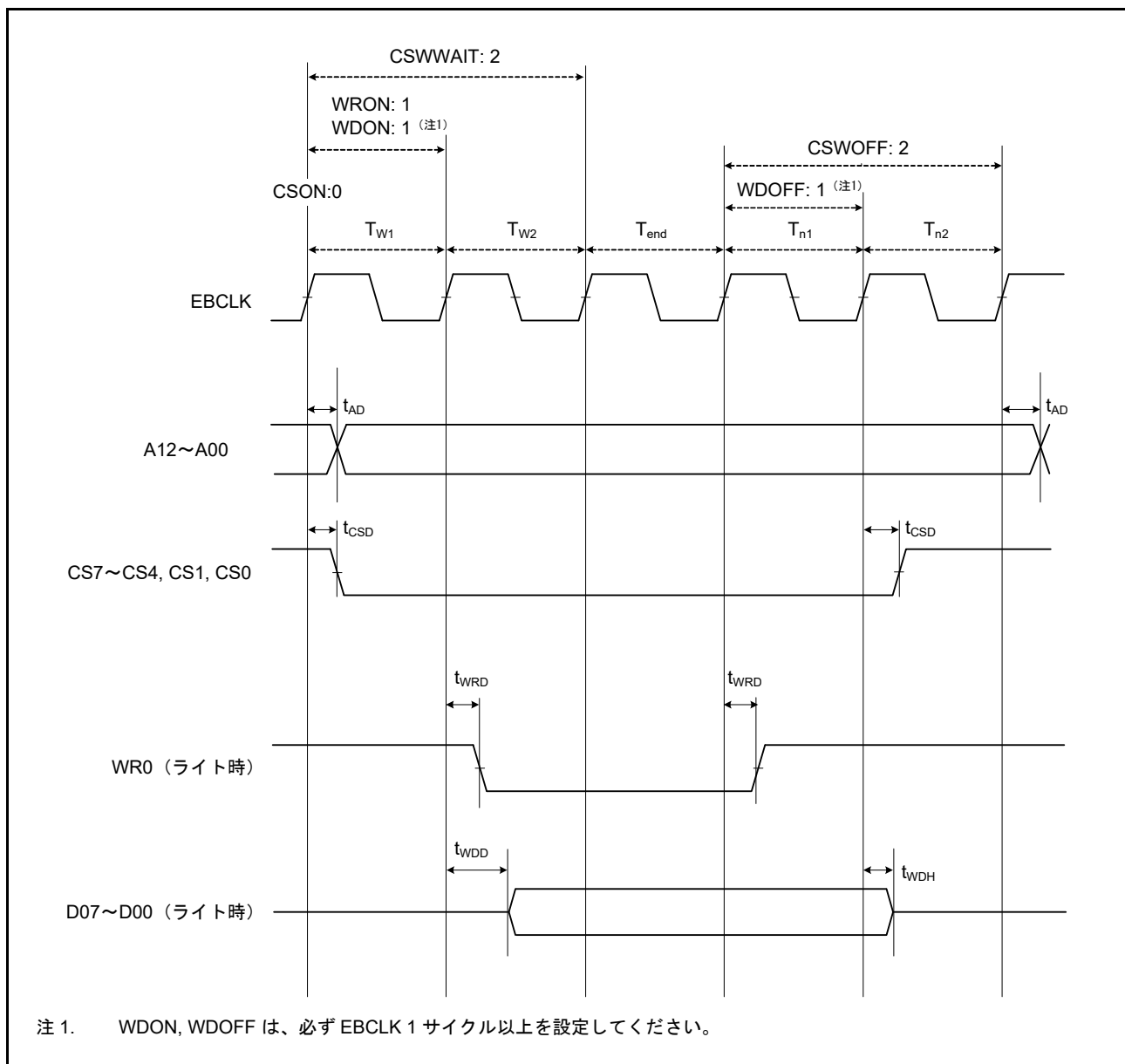
図 52.23 バスクロック同期を使用したノーマルライトサイクルの外部バスタイミング
