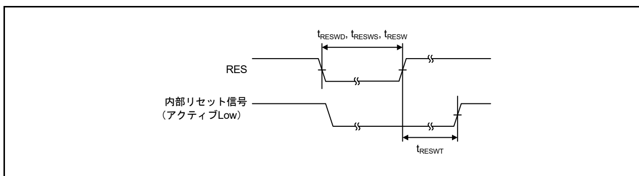
図 52.14 リセット入力タイミング
