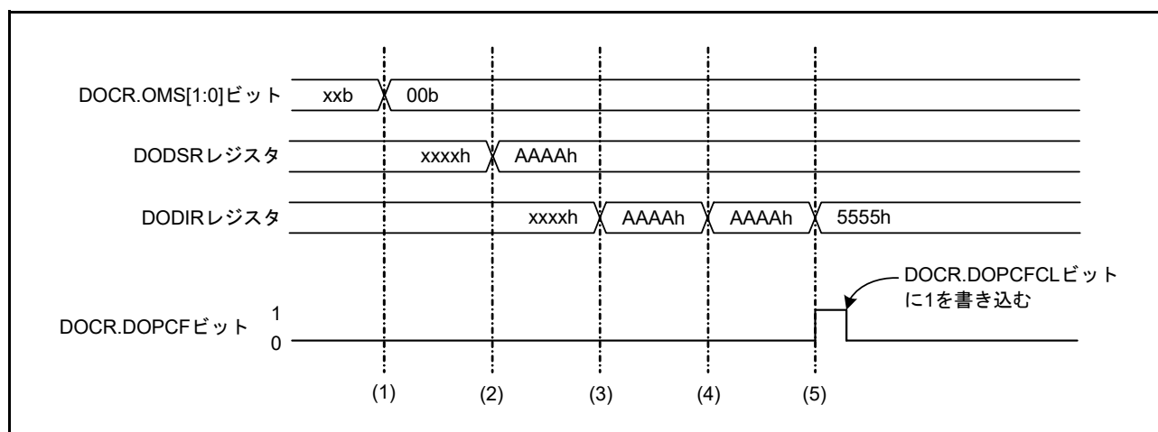
図 47.2 データ比較モードの動作例
