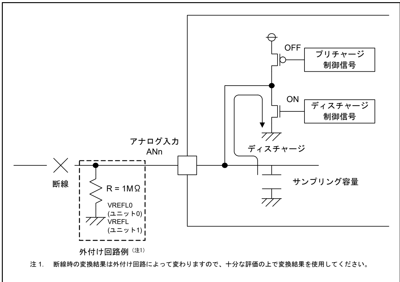
図 42.38 ディスチャージを選択した場合の断線検出例
