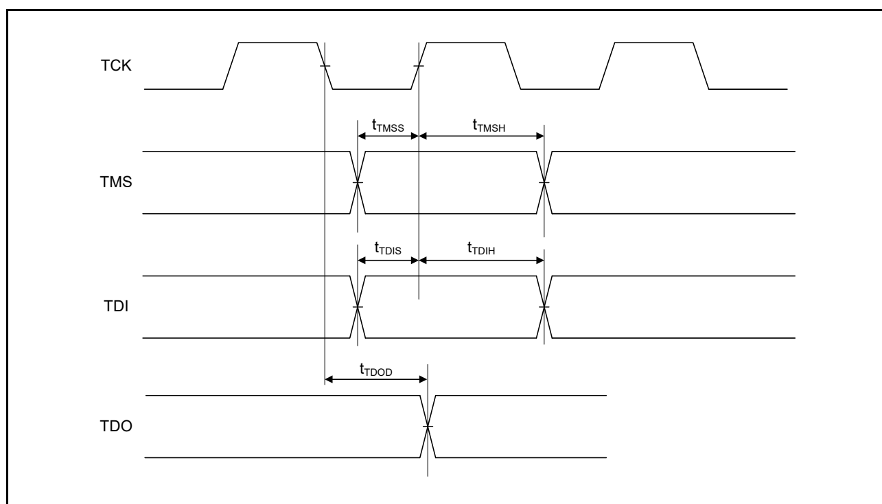
図 52.76 JTAG 入出力タイミング
