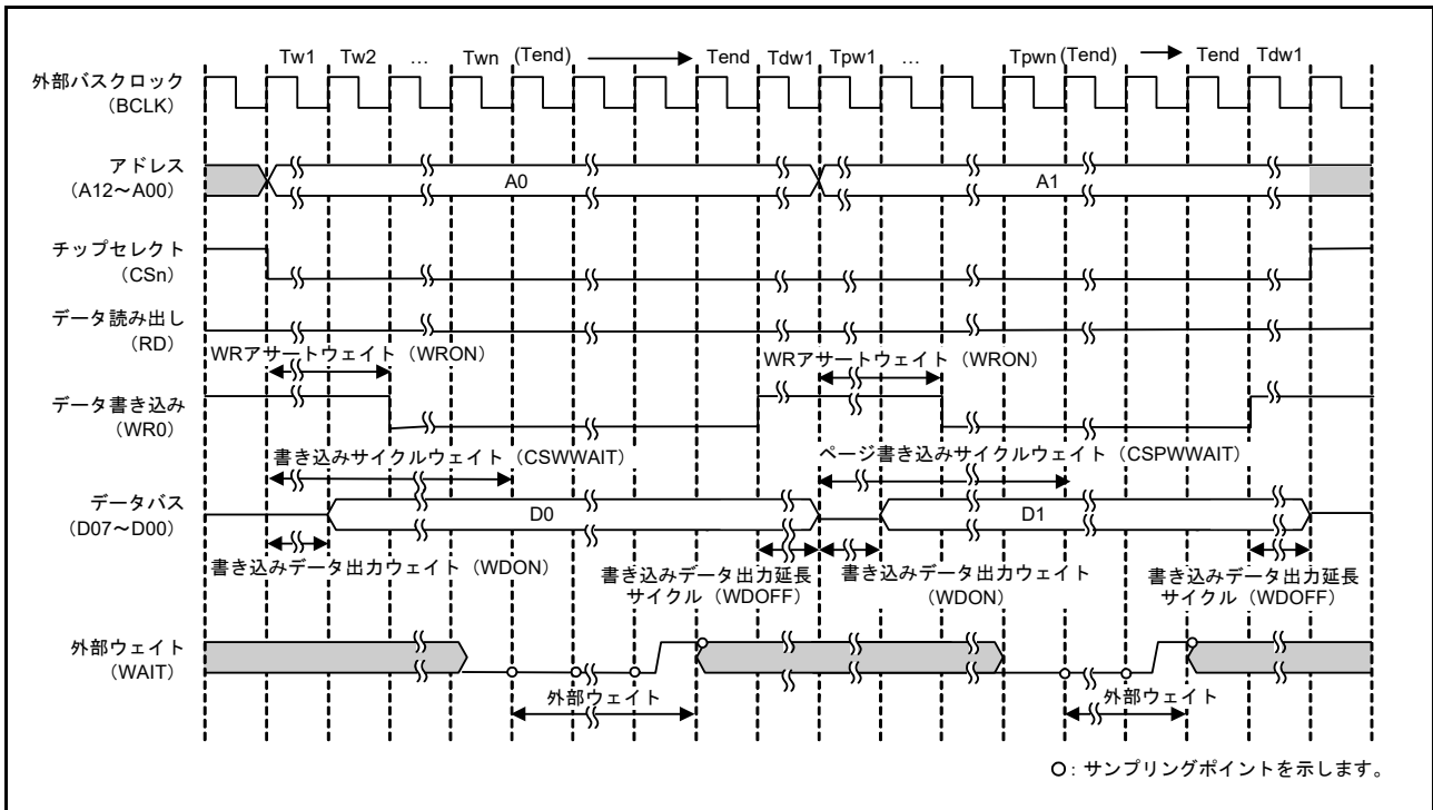
図 15.26 外部ウェイトタイミング例 (バイトストローブモード時の 8 ビットバス空間に対するページライトアクセス、BCLK 端子出力選択ビットで BCLK の 1 分周を選択した場合) (n = 0, 1, 4 ~ 7)
