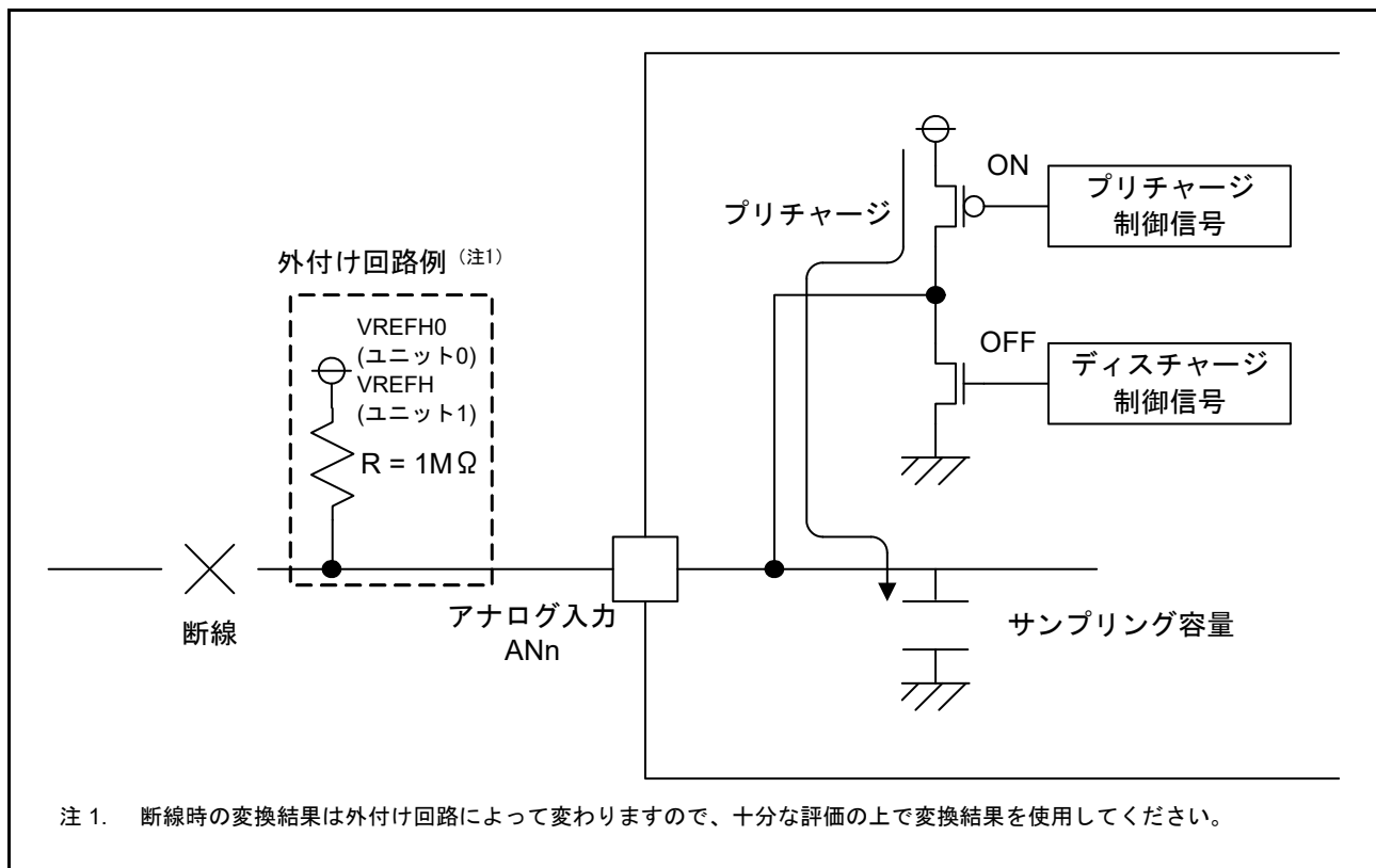
図 42.37 プリチャージを選択した場合の断線検出例
