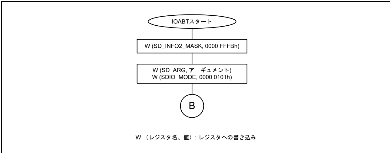
図 39.20 CMD53 マルチブロックライト時に CMD52 (SDIO Abort) が送信される場合のフロー
