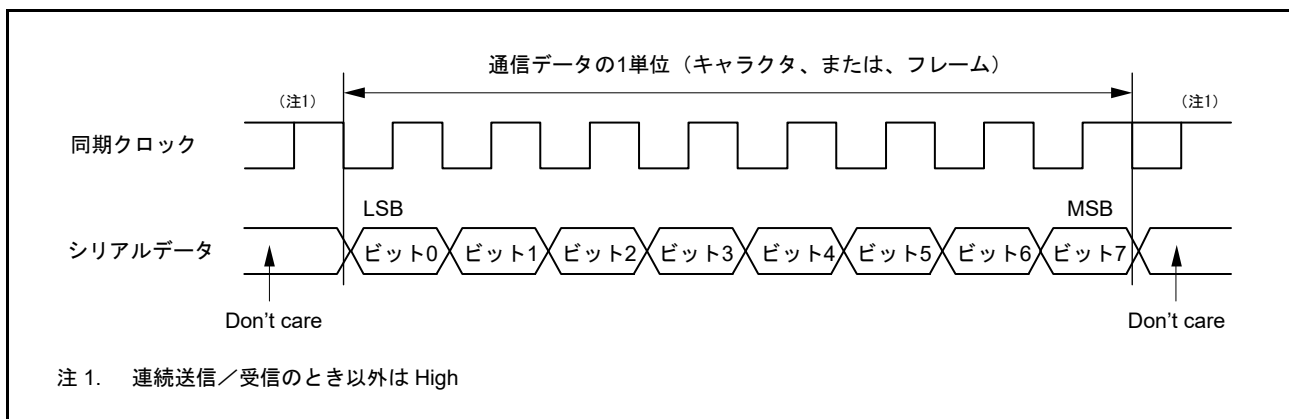
図 30.31 クロック同期式シリアル通信のデータフォーマット (LSB ファーストの場合)
