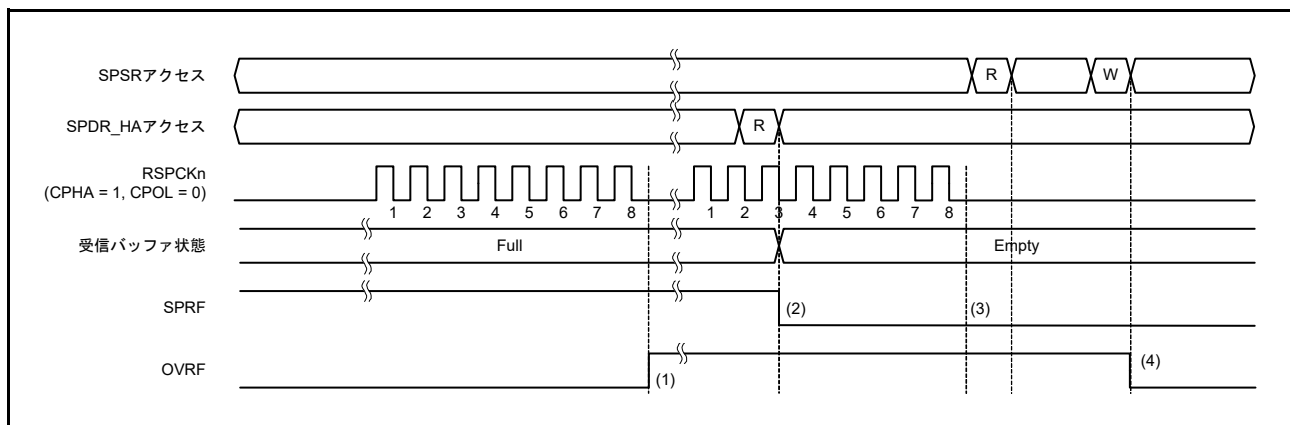
図 34.28 OVRF フラグおよび SPRF フラグの動作例
