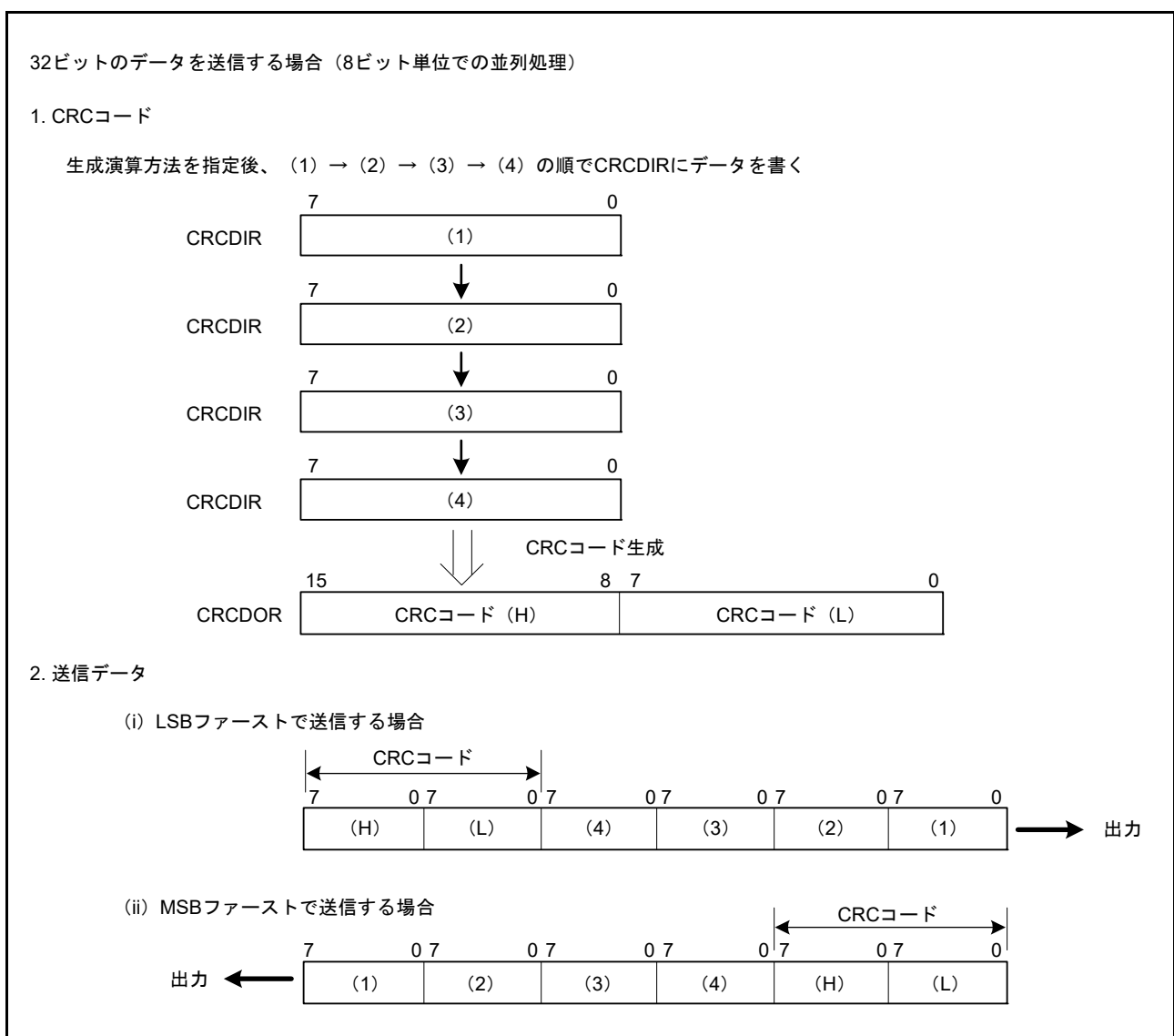
図 36.6 LSB ファーストと MSB ファーストのデータ送信
