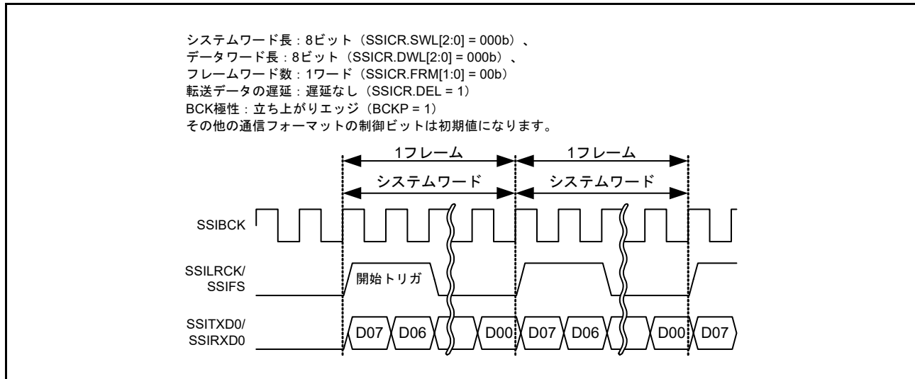
図 37.39 モノラルフォーマットでのロングフレーム (パディングなし)
