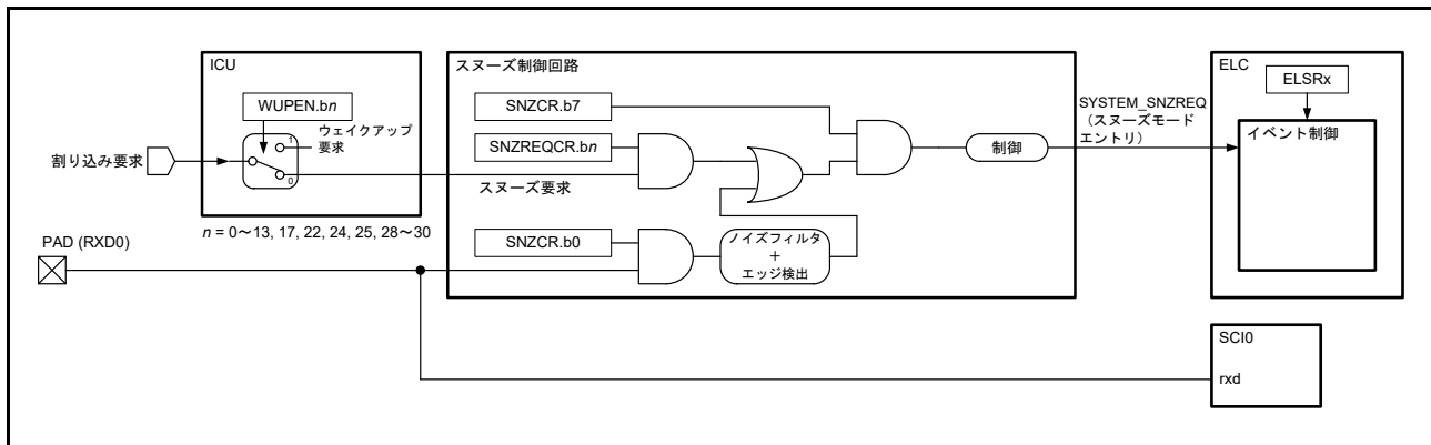
図 11.5 スヌーズエントリの構成
