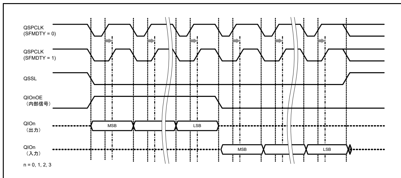
図 35.9 SFMDTY ビットを使用した QSPCLK 信号デューティ比の補正例 (PCLKA を 3 通倍した場合)
