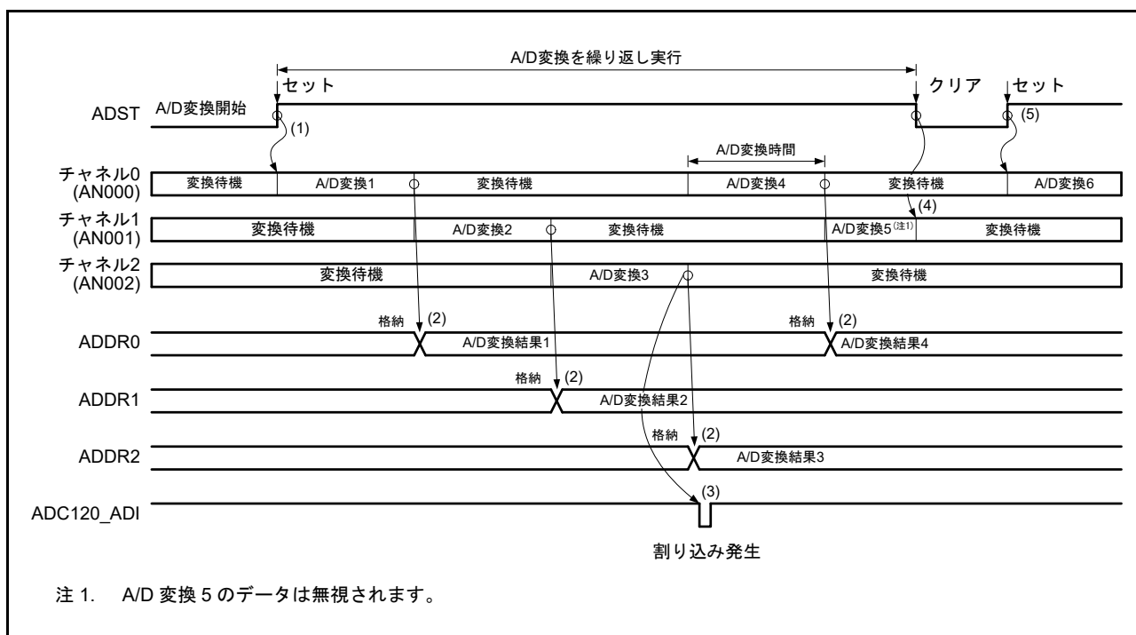
図 42.16 連続スキャンモードの基本動作例 (AN000 ~ AN002 選択)
