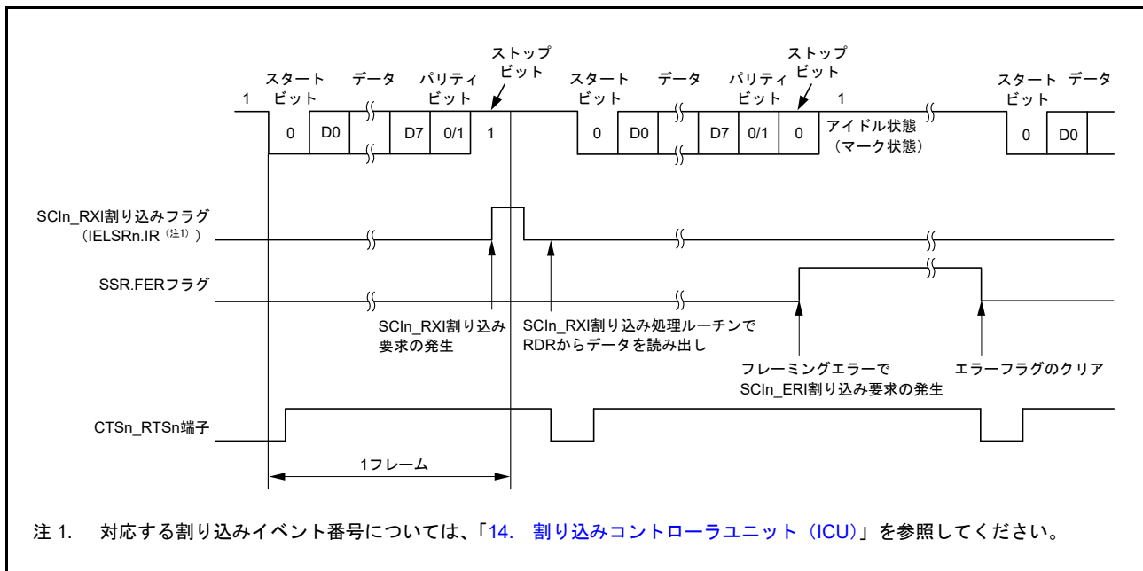
図 30.16 調歩同期式モードにおけるシリアル受信の動作例 (2) (RTS 機能を使用する場合) (8 ビットデータ / パリティあり / 1 ストップビットの場合)
