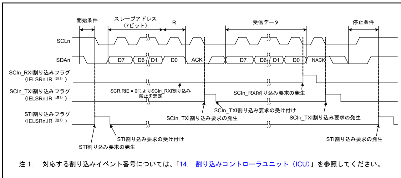
図 30.67 簡易 IIC モードにおけるマスタ受信の動作例 (7 ビットスレーブアドレス、送信割り込み、受信割り込み使用時)
