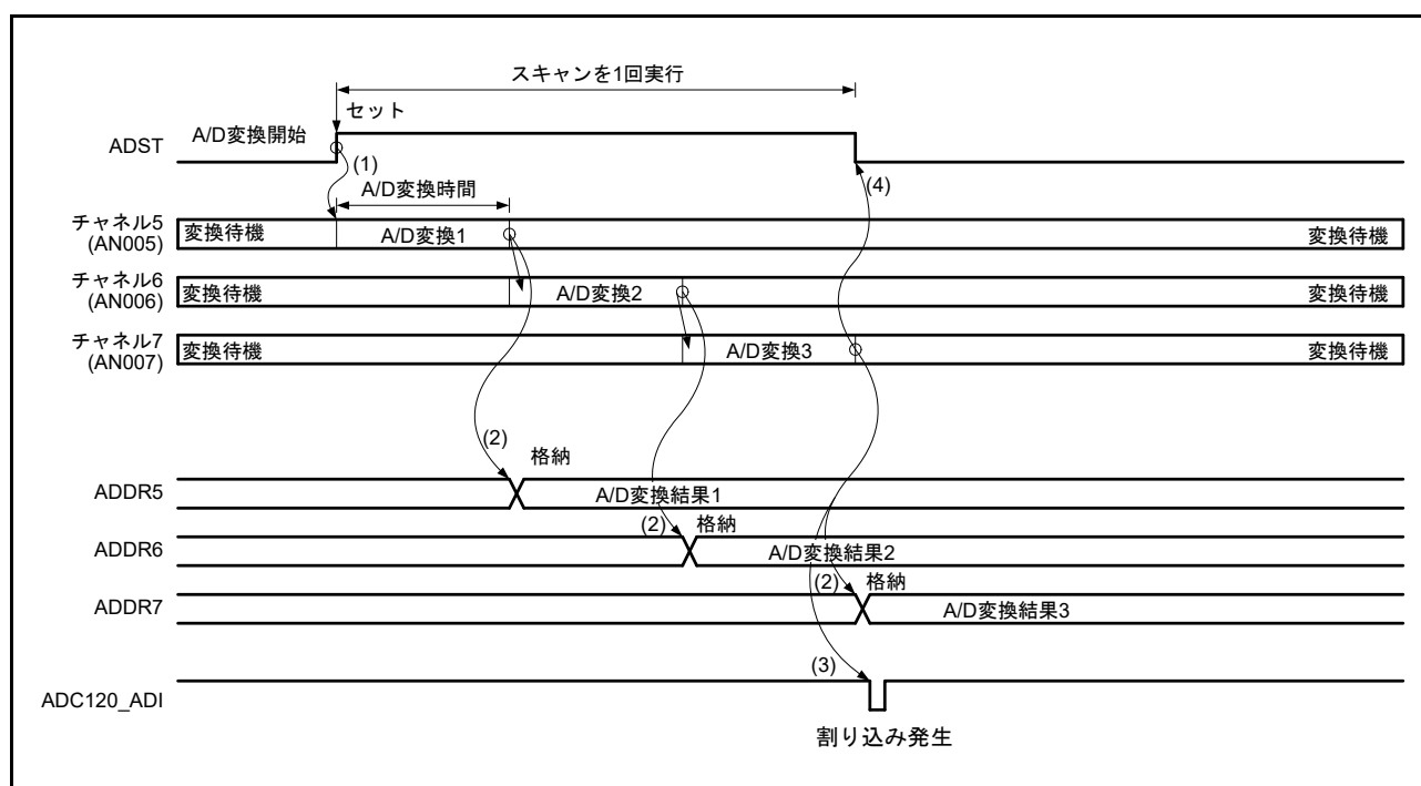
図 42.7 シングルスキャンモードの基本動作例 (AN005 ~ AN007 選択)
