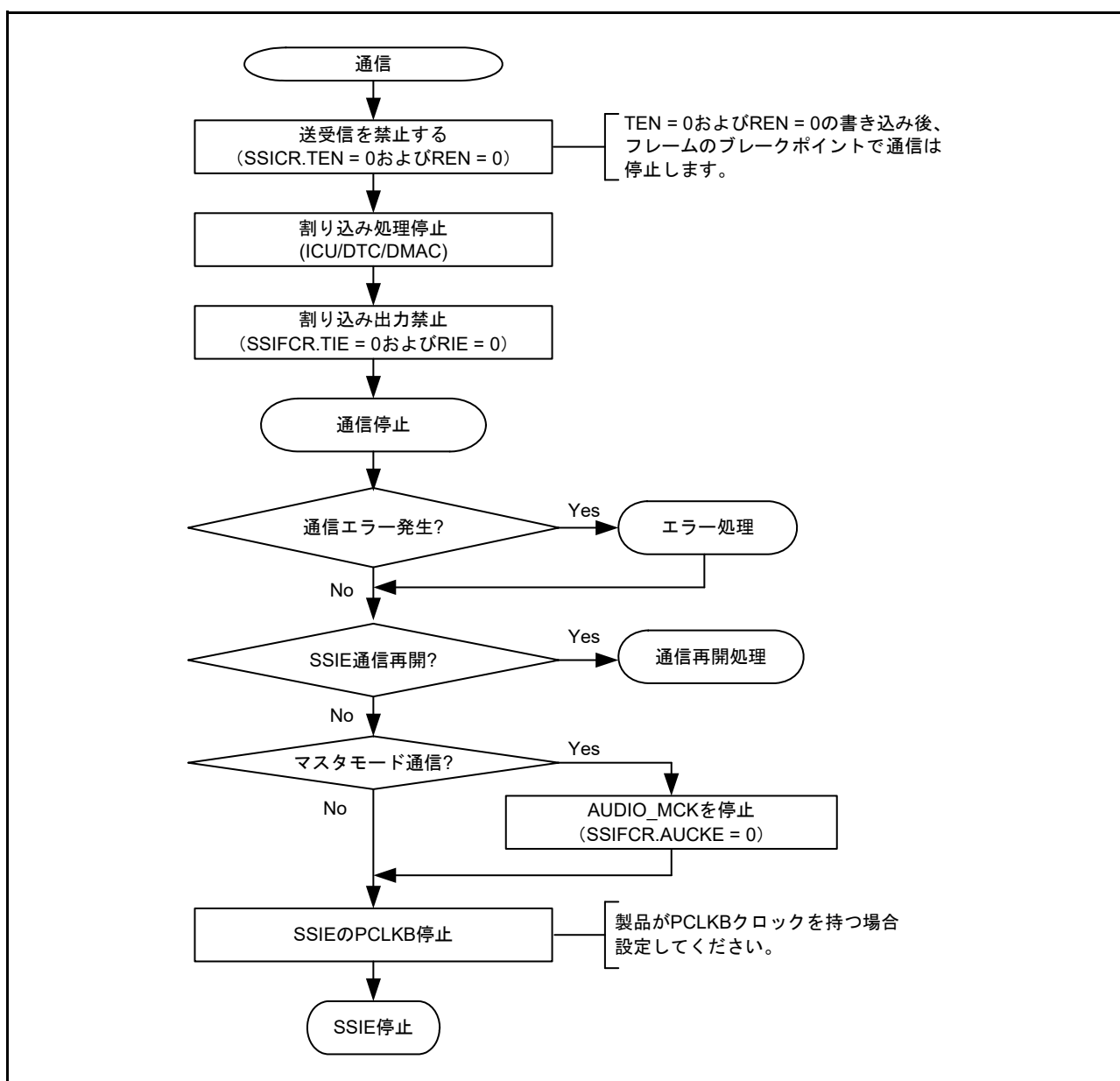
図 37.55 通信停止手順 (CPU 動作手順)
