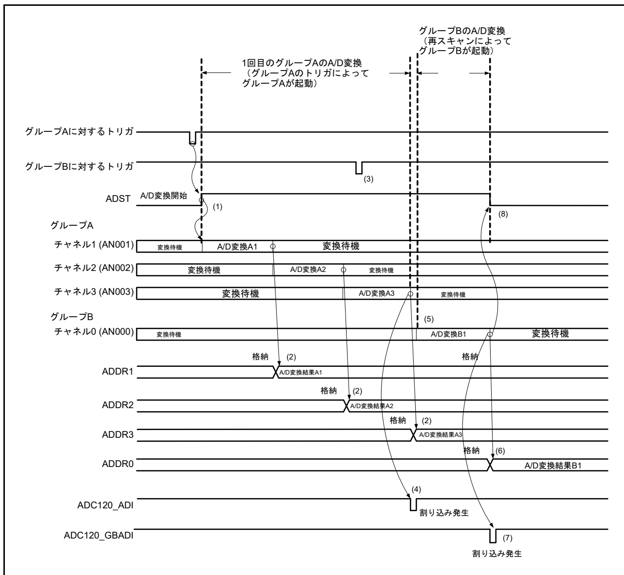
図 42.28 グループ A 優先制御の動作例 (3) (ADGSPCR.GBRSCN = 1、ADGSPCR.GBRP = 0 の場合)
