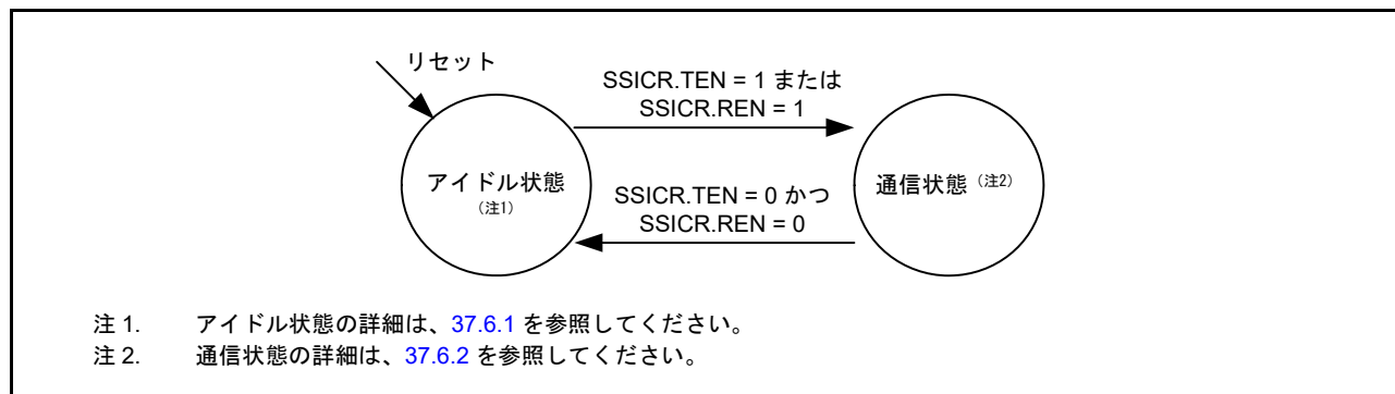
図 37.42 SSIE の状態遷移
