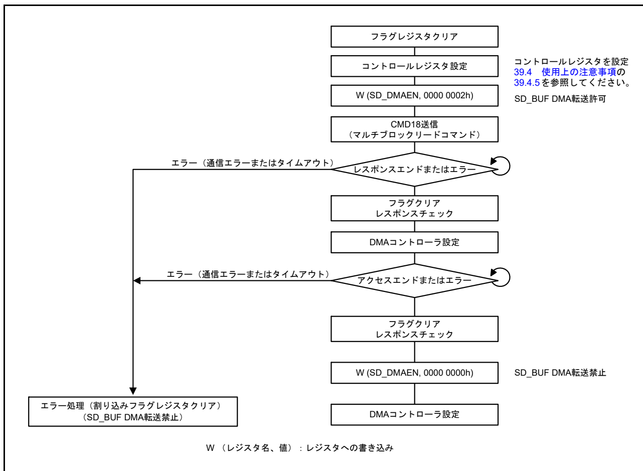
図 39.22 SD_BUF_DMA リード動作の例
