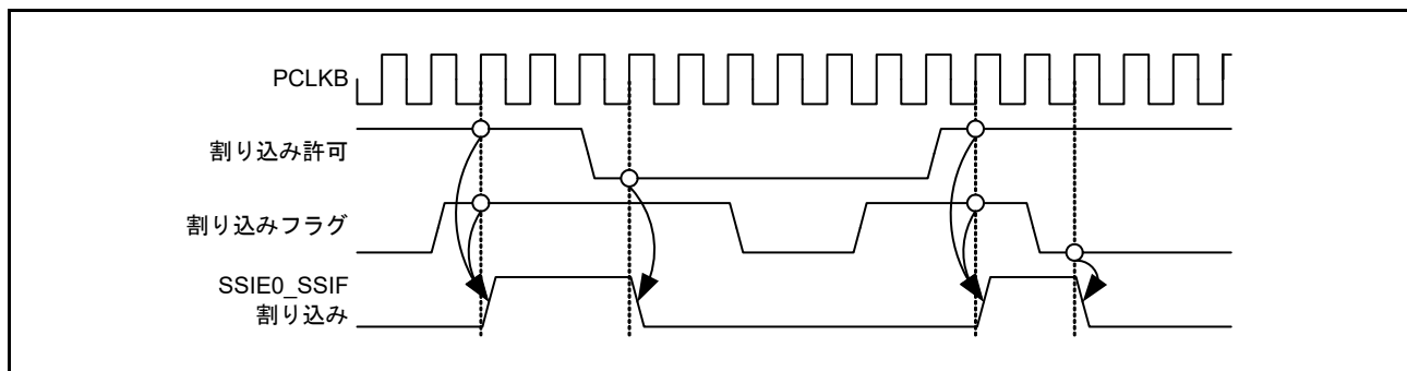
図 37.58 割り込み要因共通のタイミング図 (SSIE0_SSIF)
