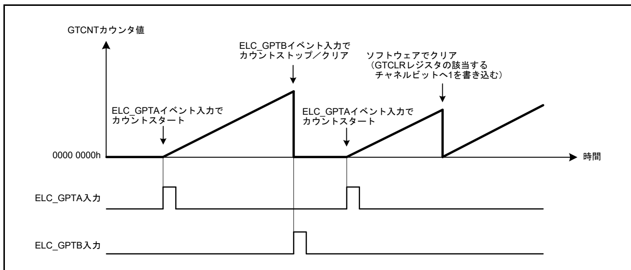
図 23.57 ハードウェア要因によるカウンタクリア動作例 (のこぎり波アップカウント、ELC_GPTA イベント入力でスタート、ELC_GPTB イベント入力でストップ/クリアの場合)
