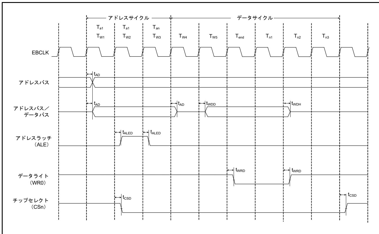
図 52.21 アドレス/データマルチプレクスバスのライトアクセスタイミング
