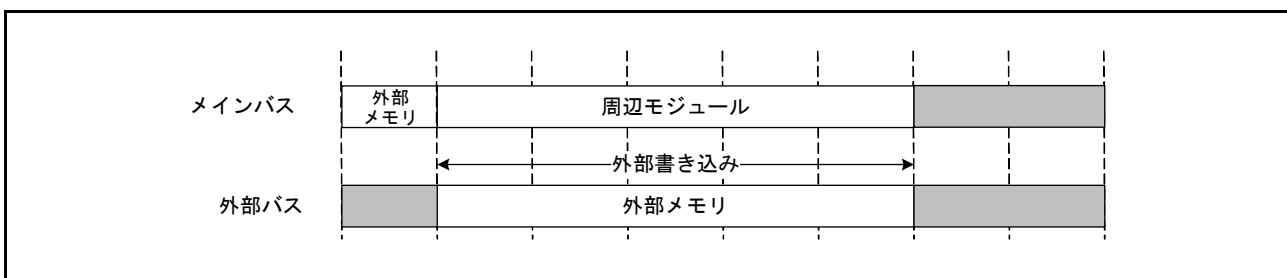
図 15.35 ライトバッファ機能使用時の動作例
