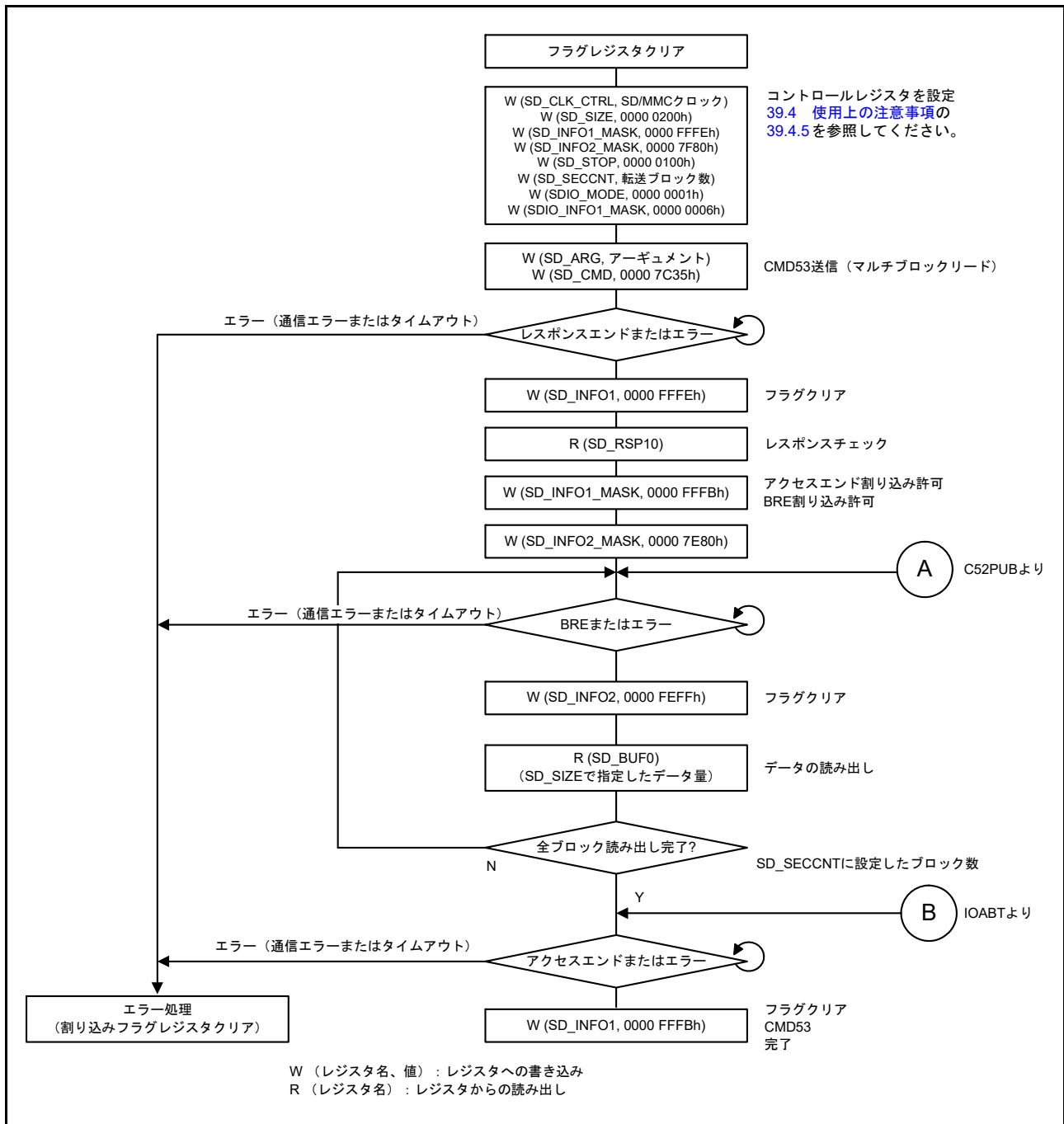
図 39.16 マルチブロックリード動作の IO_RW_EXTENDED コマンド (CMD53) の例
