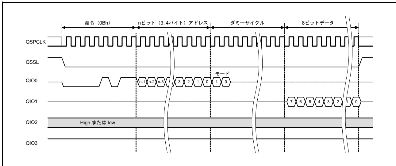
図 35.16 ファストリードバスサイクル
