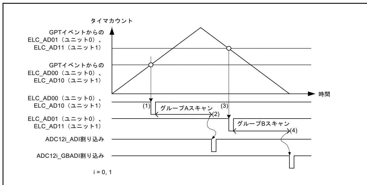
図 42.23 グループスキャンモードの基本動作例 (ELC からの同期トリガ使用)
