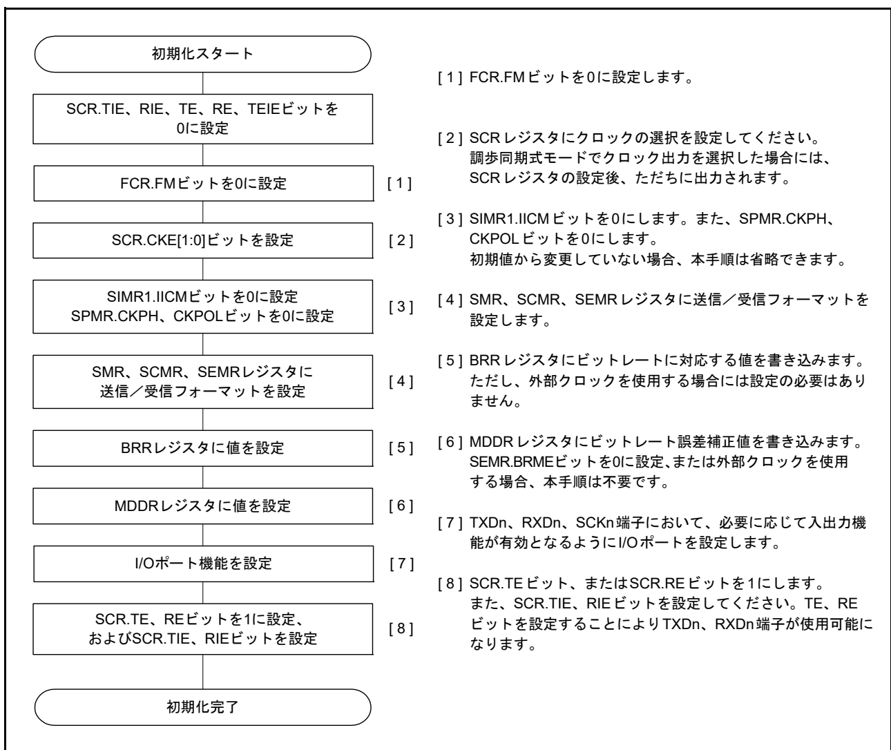
図 30.7 調歩同期式モードにおける SCI の初期化フローチャート例 (非 FIFO 選択時)
