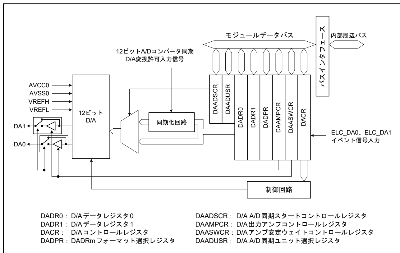
図 43.1 DAC12のブロック図
