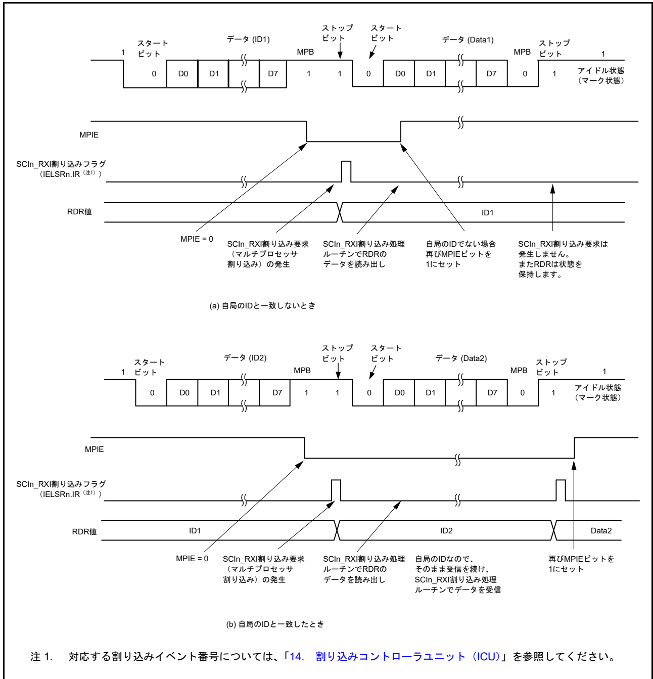
図 30.26 SCI の受信時の動作例 (8 ビットデータ/マルチプロセッサビットあり/1 ストップビットの場合)
