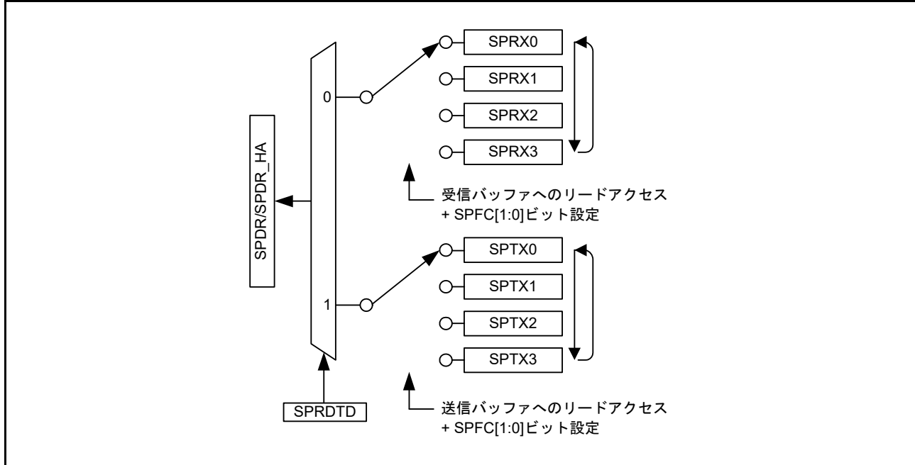
図 34.4 読み出し時の SPDR/SPDR_HA レジスタの構成図
