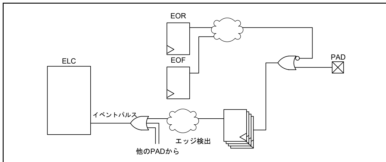
図 20.4 イベントパルスの発生
