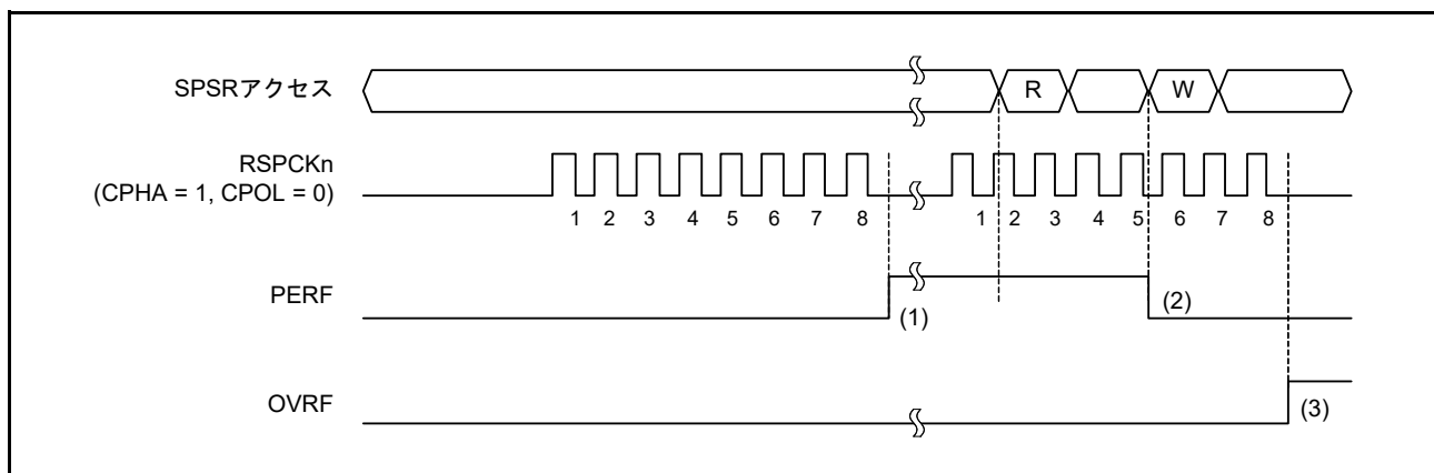
図 34.31 PERF フラグの動作例
