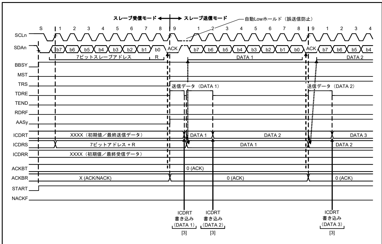
図 32.16 スレーブ送信の動作タイミング (1) (7 ビットアドレスフォーマット)
