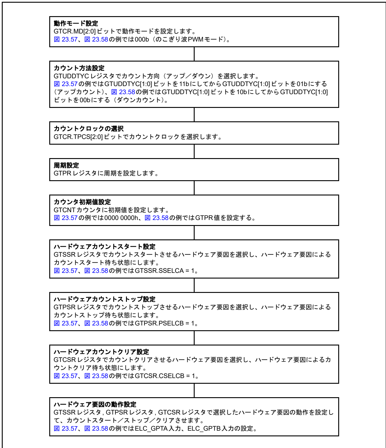
図 23.59 ハードウェア要因によるカウントクリア動作設定例
