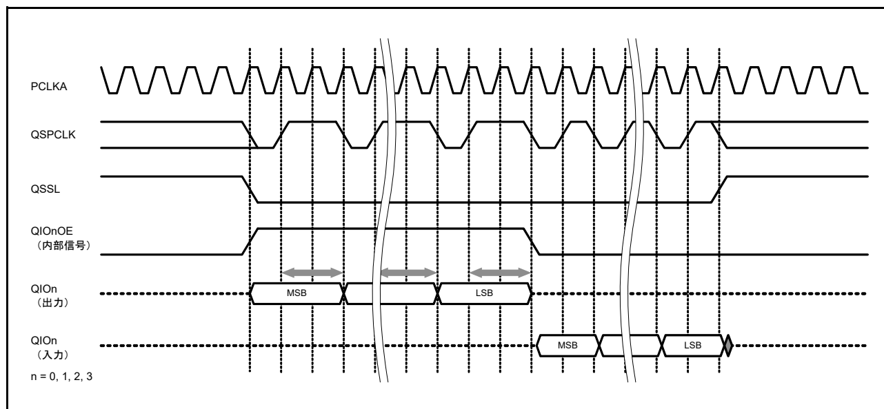
図 35.14 SFMOHW ビットを使用したシリアルデータ出力のホールド時間調整
