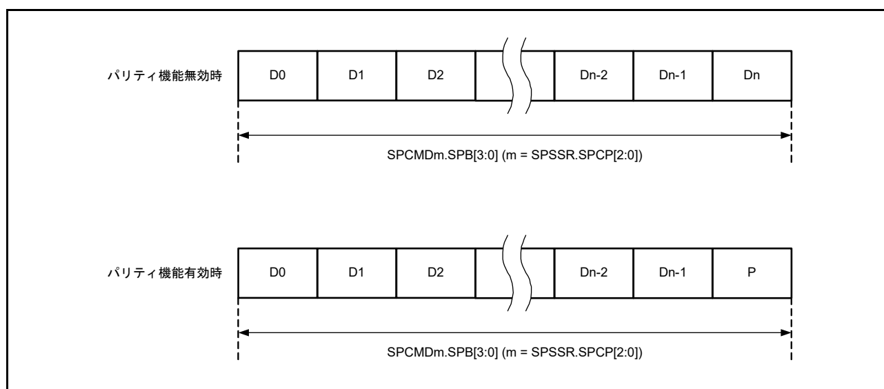
図 34.13 パリティ機能無効時と有効時のデータフォーマット
