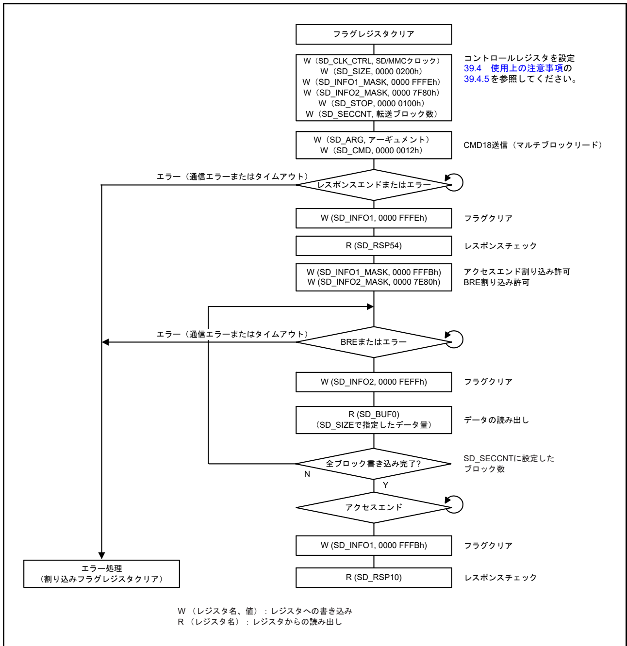
図 39.12 マルチブロックリード動作の例
