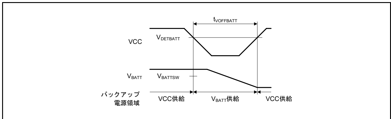
図 52.70 バッテリバックアップ機能特性
