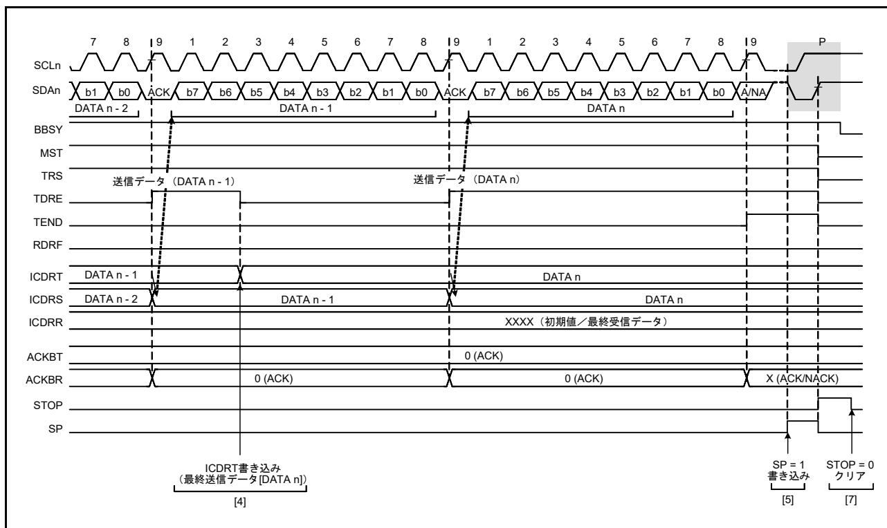
図 32.9 マスタ送信の動作タイミング (3)
