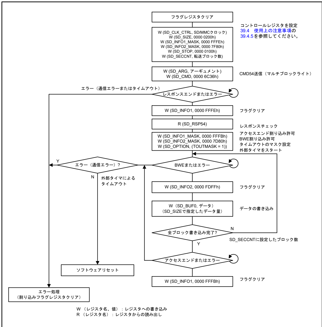
図 39.14 外付けタイマによるマルチブロックライト動作の例
