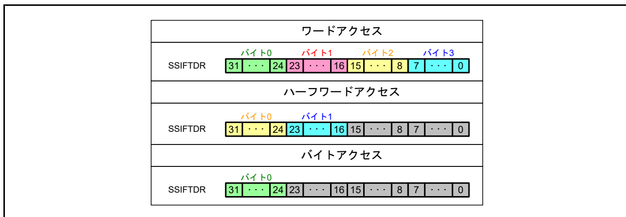
図 37.29 送信 FIFO データレジスタへのレジスタアクセス例
