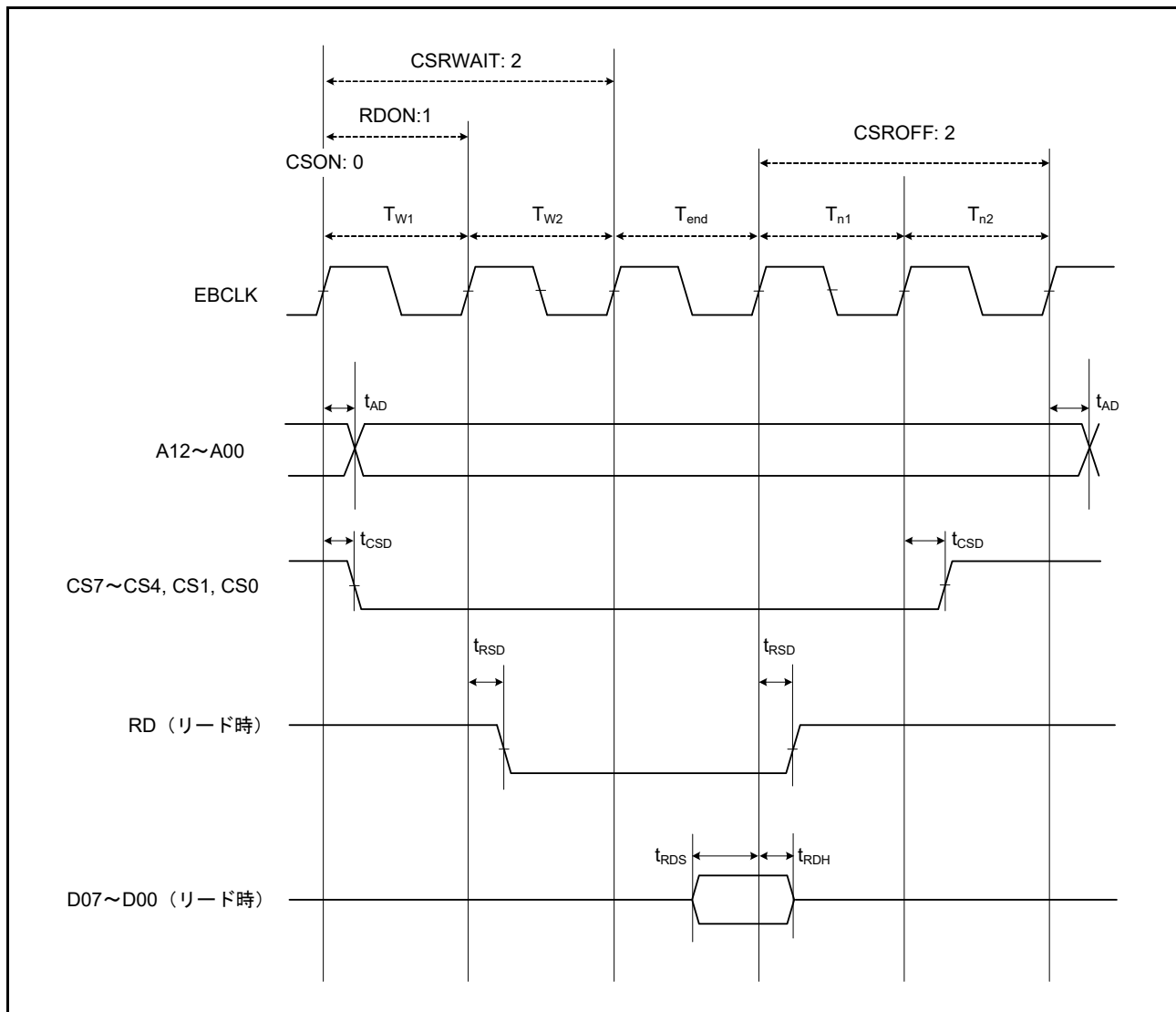
図 52.22 バスクロック同期を使用したノーマルリードサイクルの外部バスタイミング
