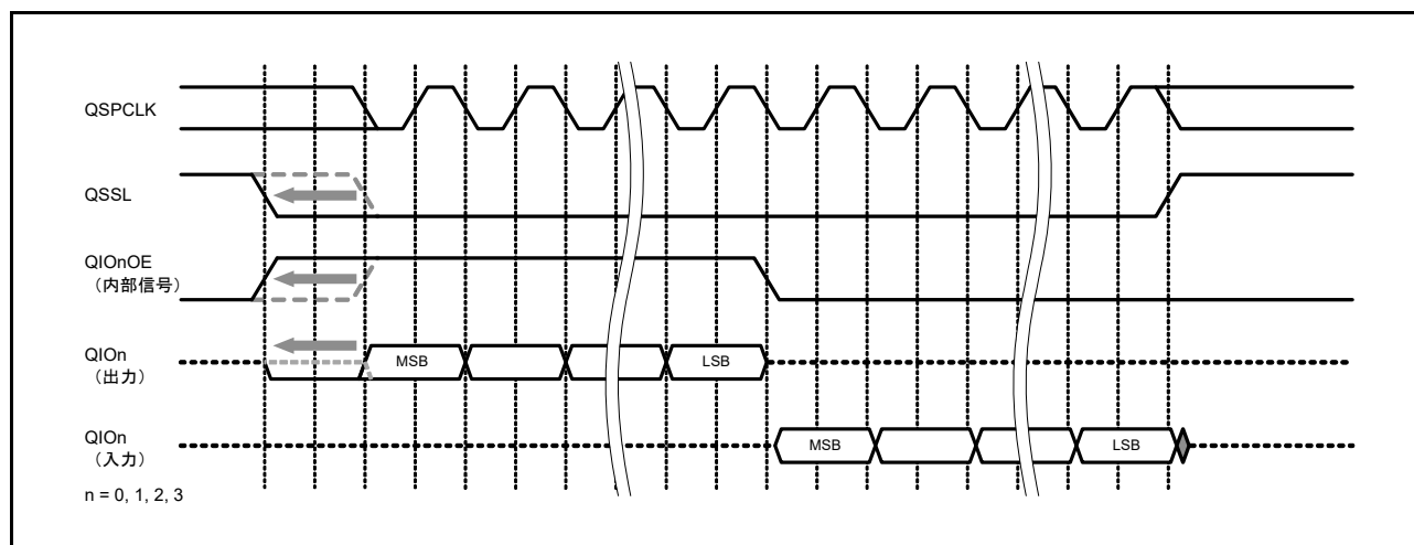
図 35.10 SFMSLD ビットを使用した QSSL 信号のセットアップ時間調整
