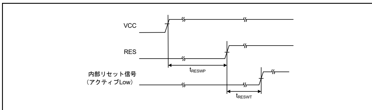
図 52.13 パワーオンリセットタイミング
