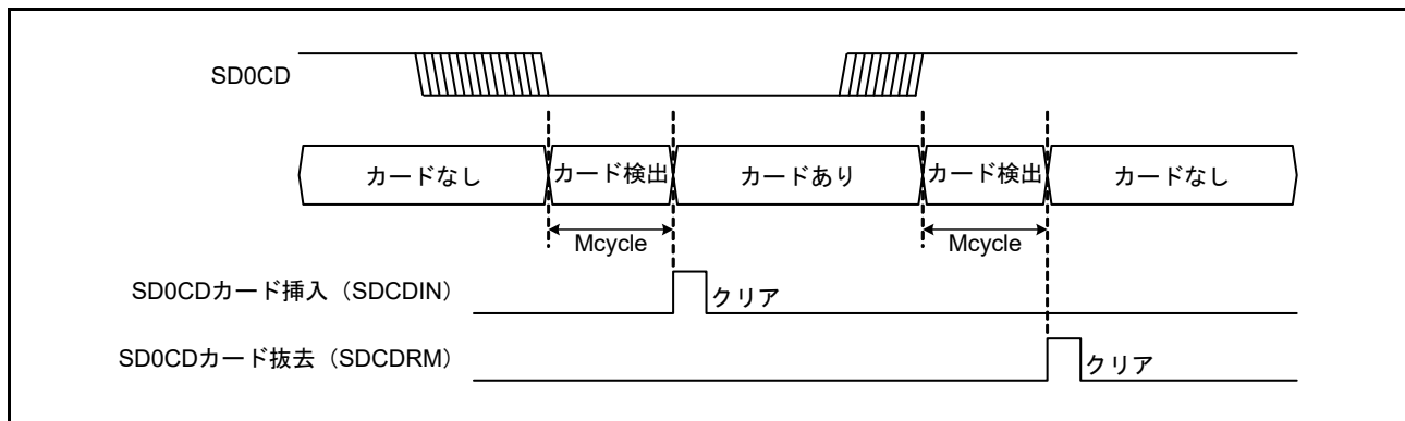
図 39.6 SD0CD によるカード検出例
