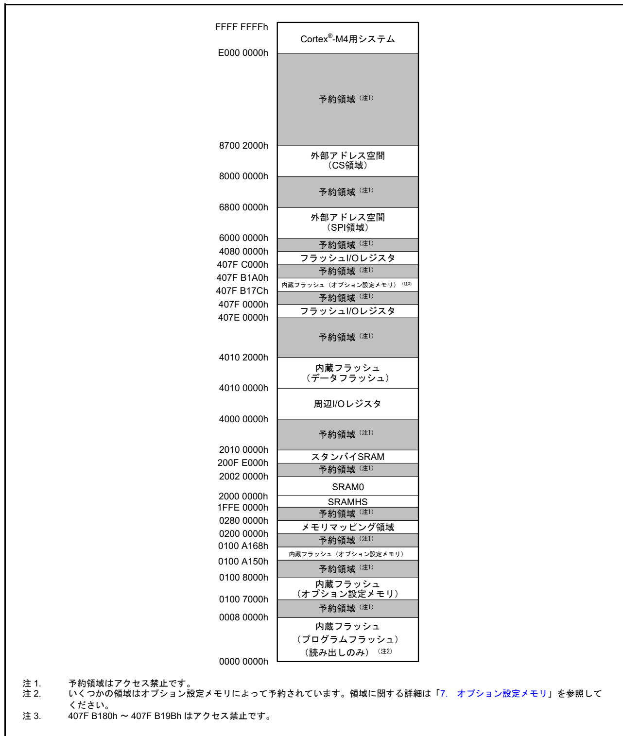
図 4.1 メモリマップ
