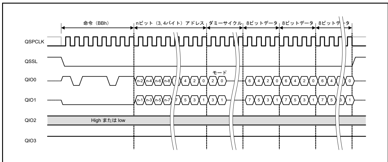
図 35.20 ファストリード Dual I/O バスサイクル
