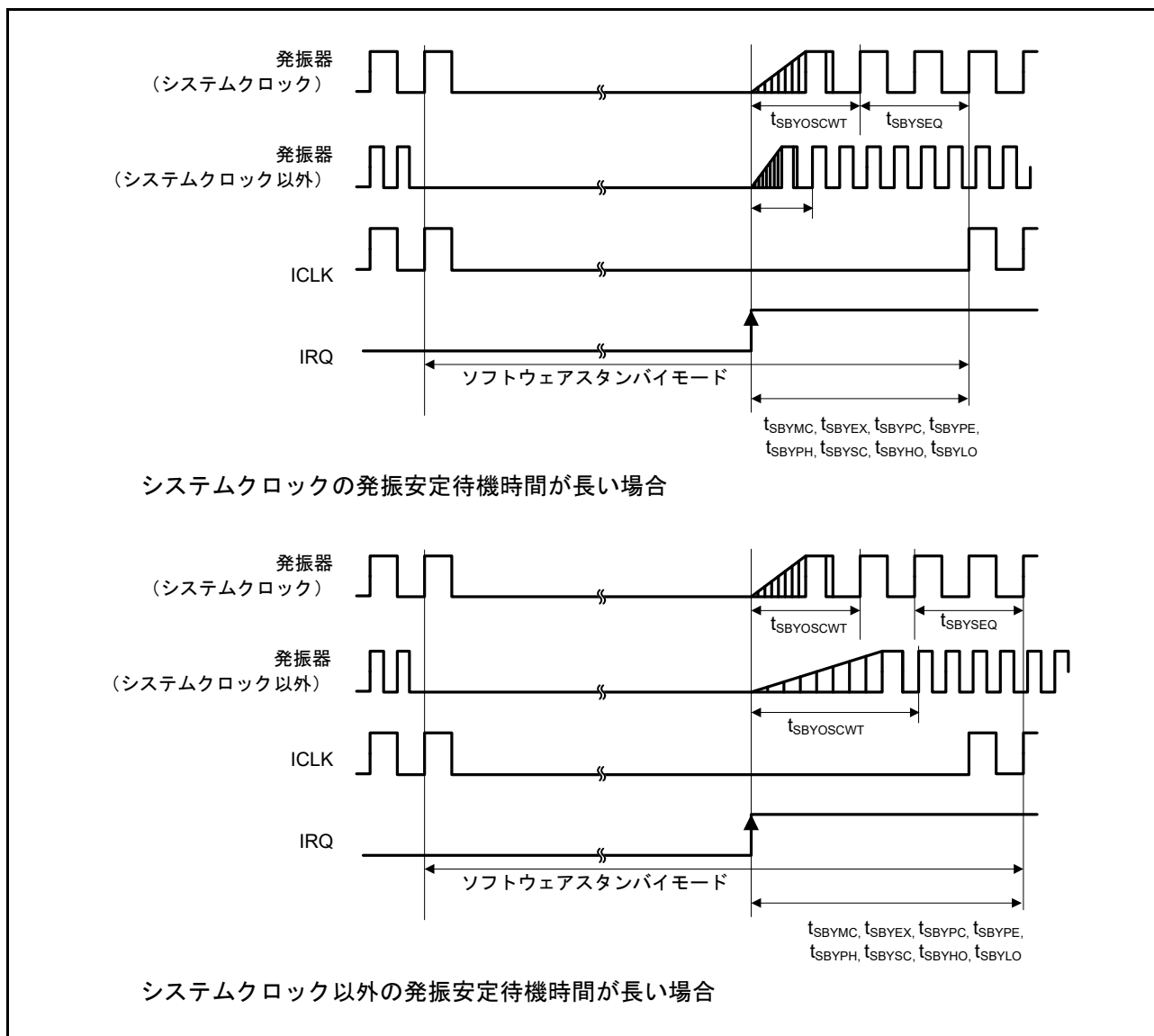
図 52.15 ソフトウェアスタンバイモード解除タイミング
