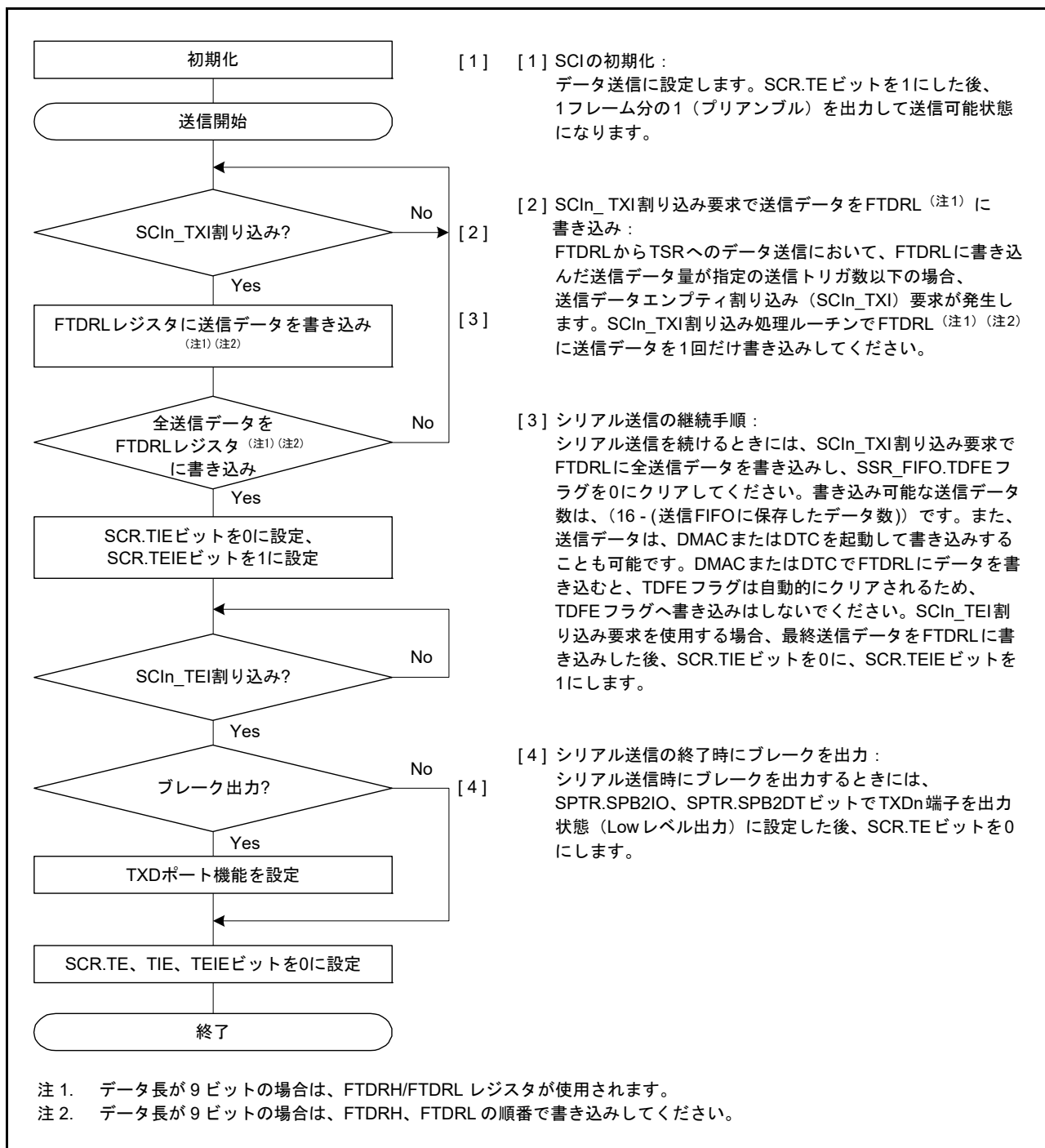
図 30.14 調歩同期式モードにおけるシリアル送信のフローチャート例（FIFO 選択時）
