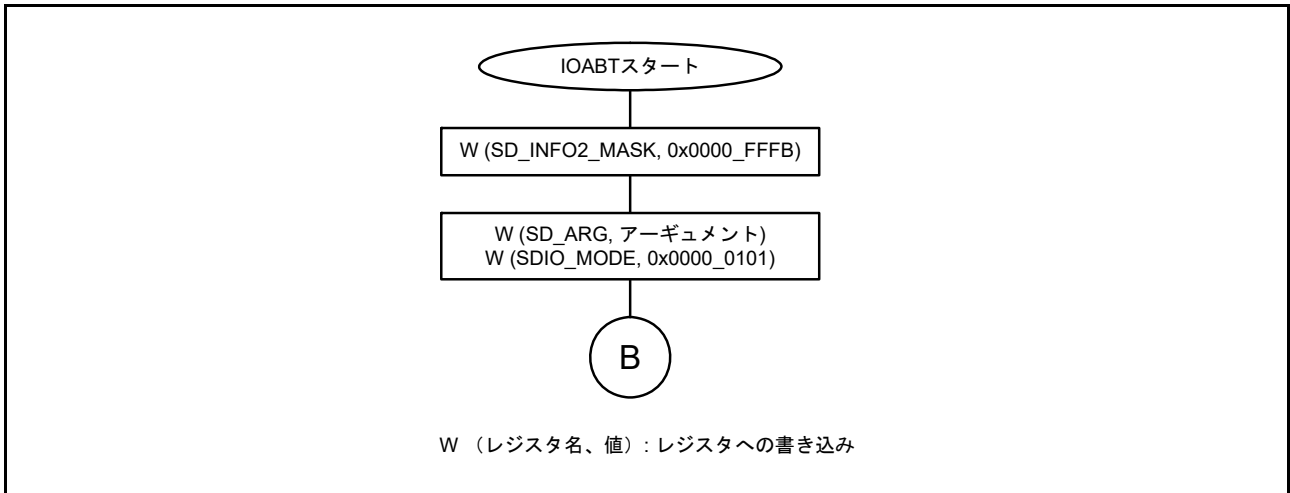
図 39.17 CMD53 マルチブロックリード時に CMD52 (SDIO abort) が送信される場合のフロー
