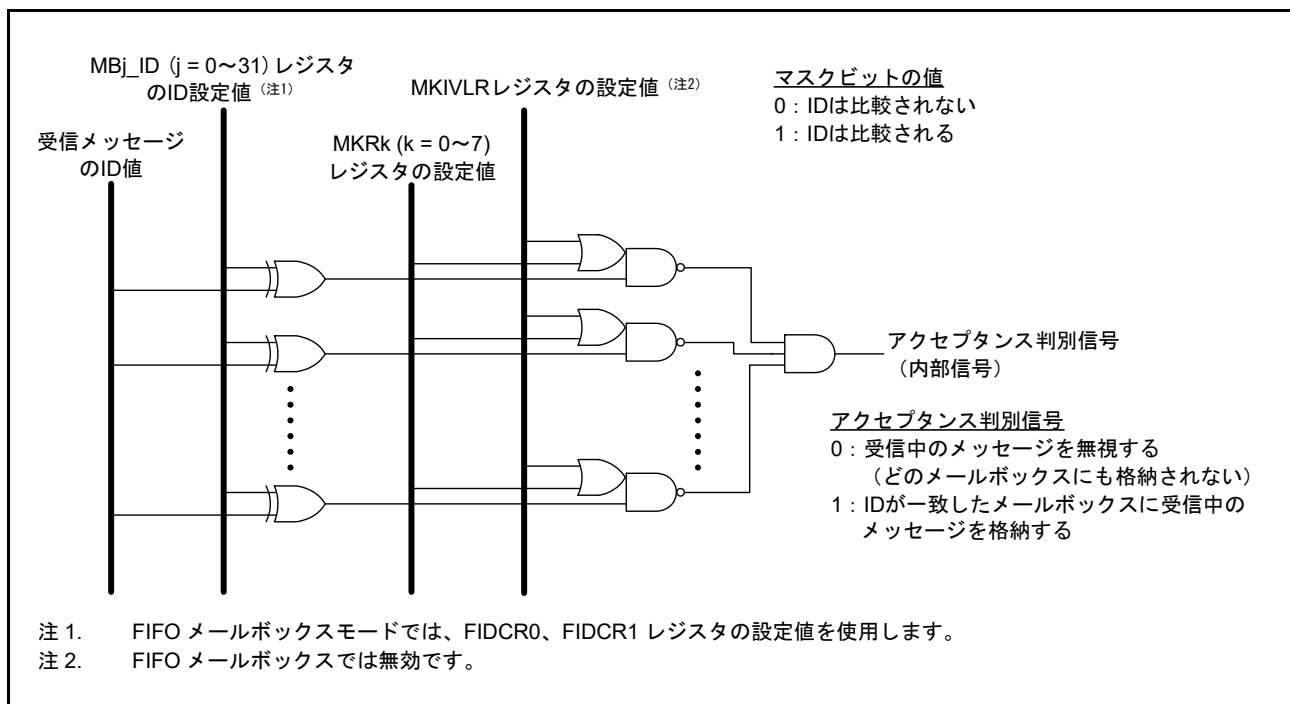
図 33.17 アクセプタンスフィルタ機能
