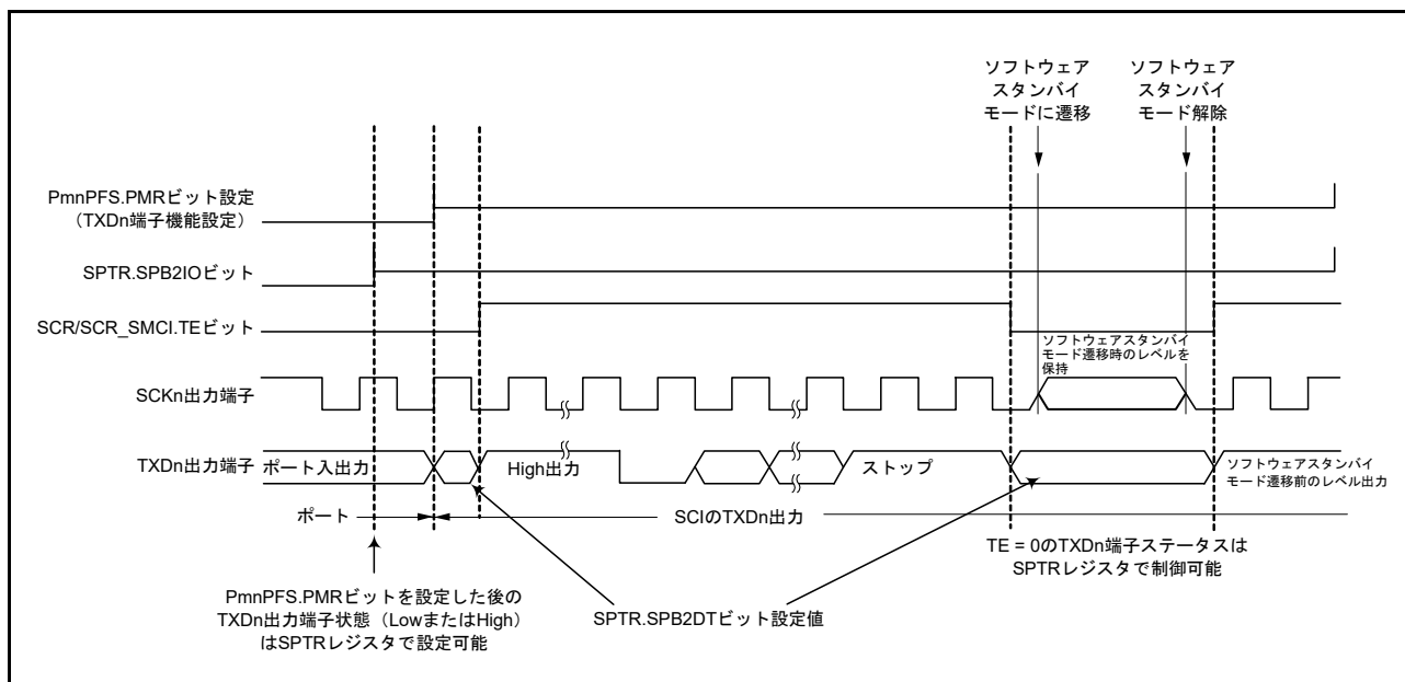
図 30.74 ソフトウェアスタンバイモード遷移中のポートの端子状態 (内部クロック、調歩同期送信)
