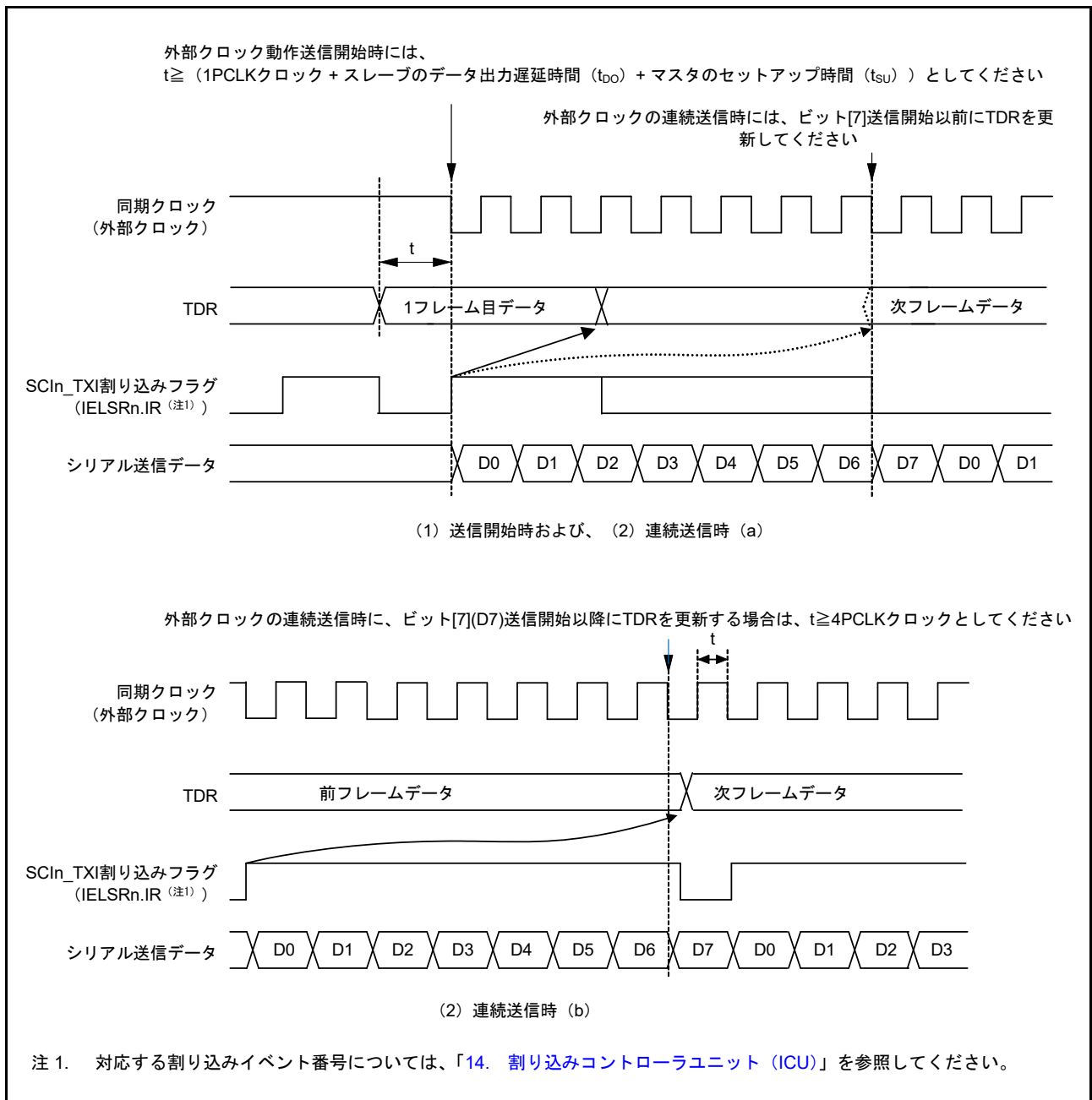
図 30.78 クロック同期送信時の外部クロック使用に関する制限事項
