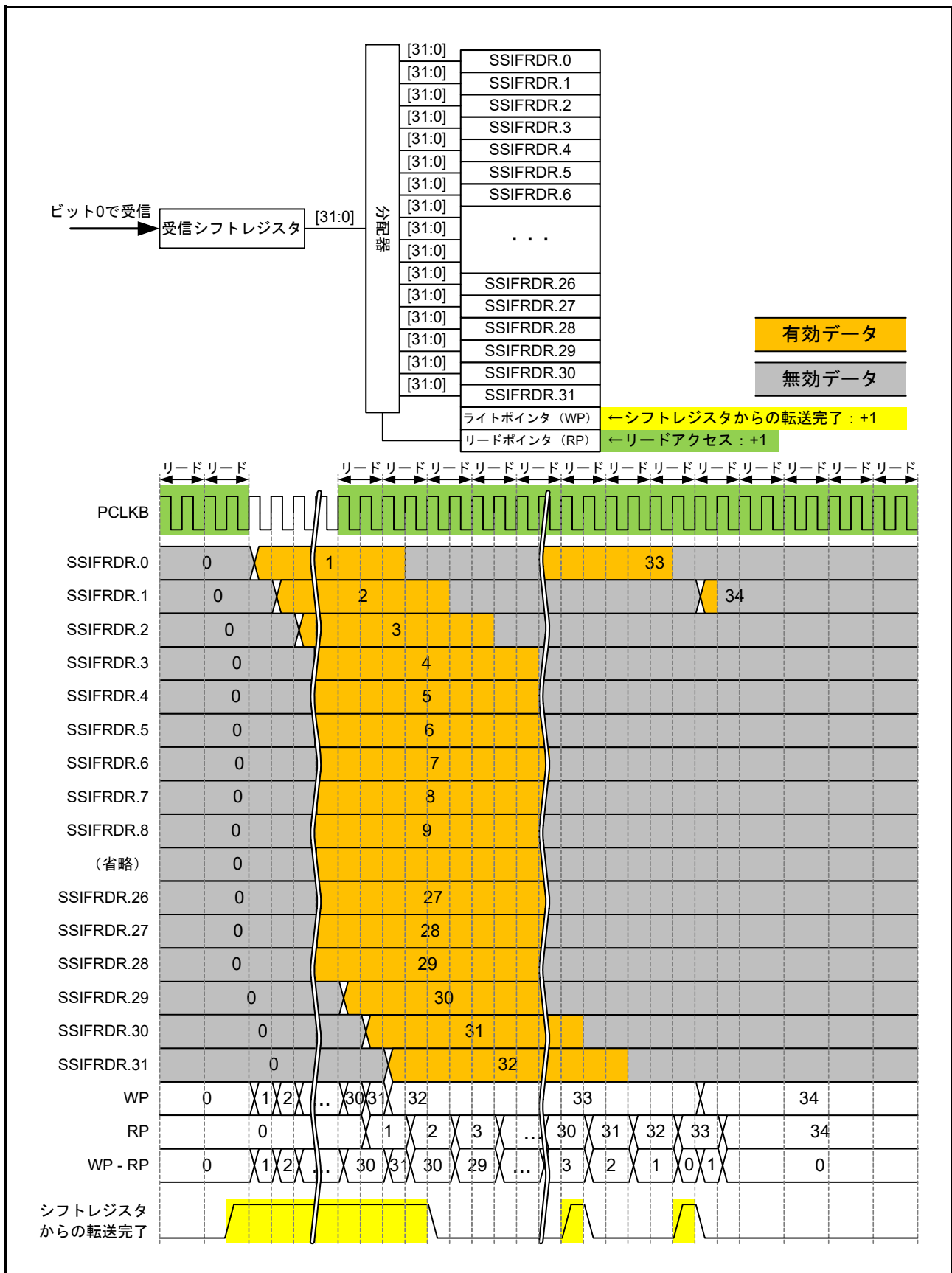
図 37.31 受信 FIFO データレジスタと受信シフトレジスタの構成および FIFO 動作例
