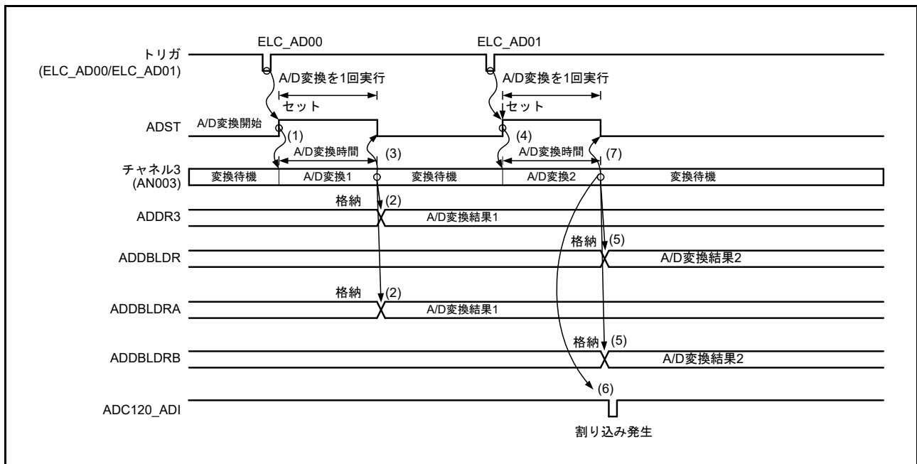
図 42.15 ダブルトリガモードの拡張動作例 (1) (AN003 の 2 重化を選択、ELC_AD00/ELC_AD01 選択)
