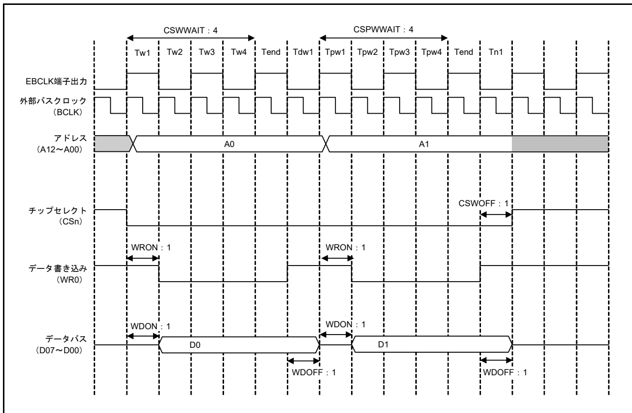
図 15.20 ページライトアクセスの動作例 (EBCLK 端子出力選択ビットで BCLK の 2 分周を設定した場合、および 1 転送要求に対して 2 回バスアクセスが発生する場合、バイトストローブモード時) ( n = 0, 1, 4 \sim 7 )
