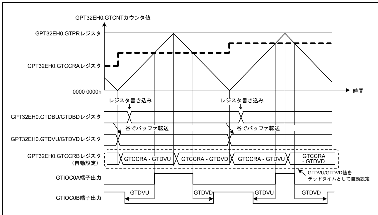
図 23.45 デッドタイム付きコンペアマッチ値の自動設定機能の動作例 (三角波 PWM モード 1、GTDVU/GTDGD レジスタはバッファ動作、アクティブ High の場合)
