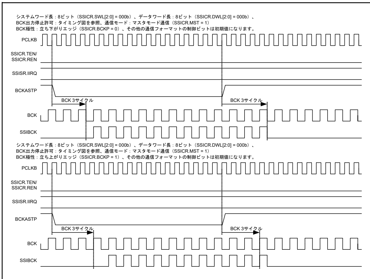
図 37.33 BCKASTP ビットの動作例 (アイドル状態の場合)
