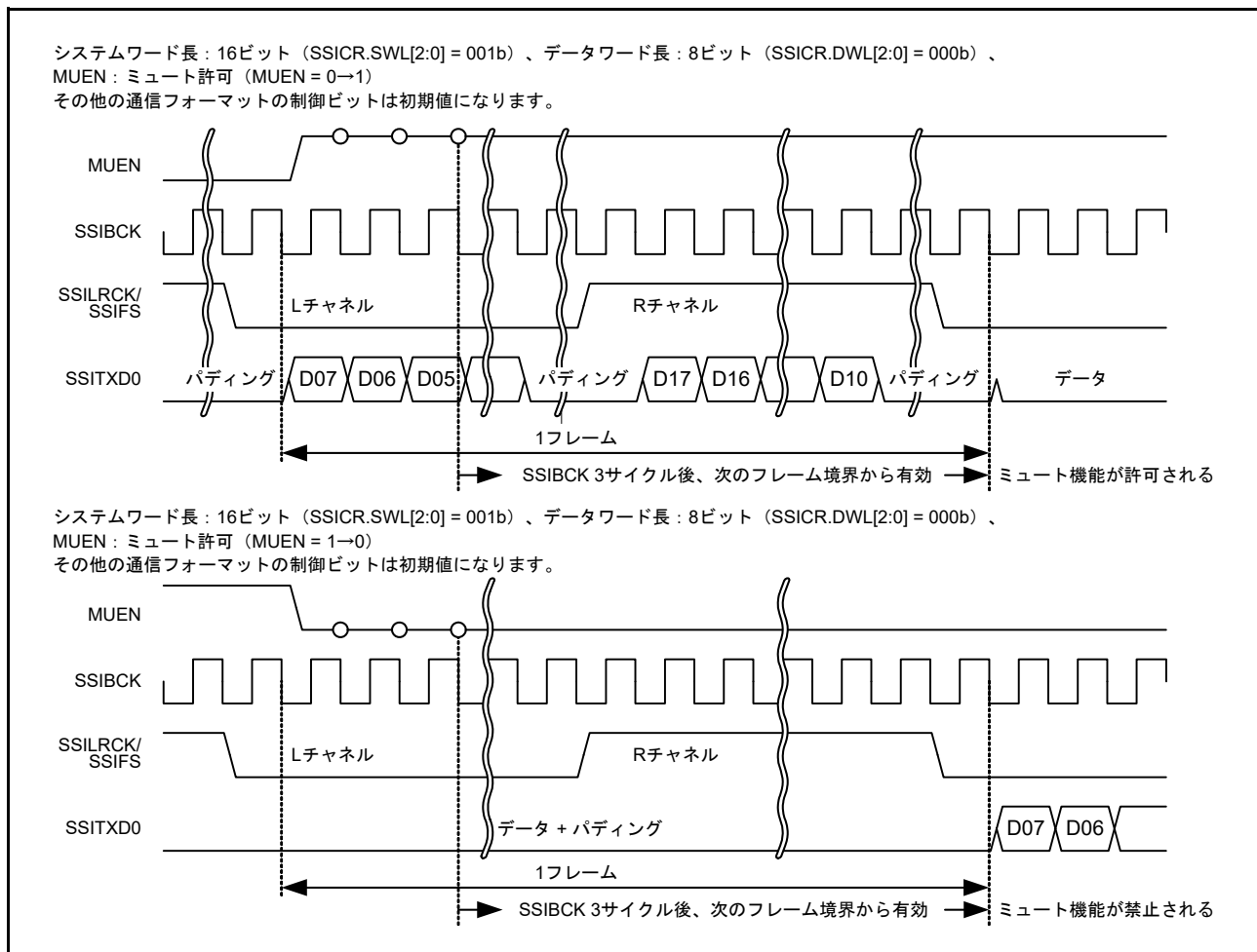
図 37.4 ミュート機能設定時の送信データ
