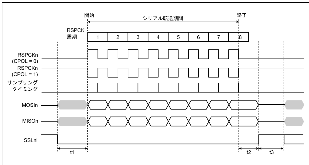
図 34.23 SPI 転送フォーマット (CPHA ビット = 1)
