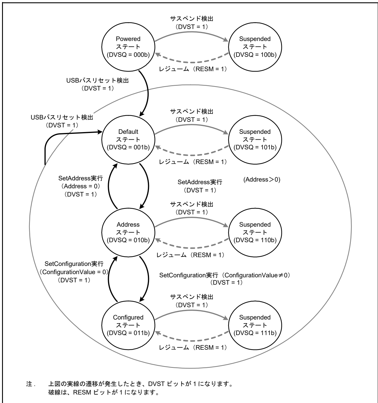
図 29.14 デバイスステートの遷移
