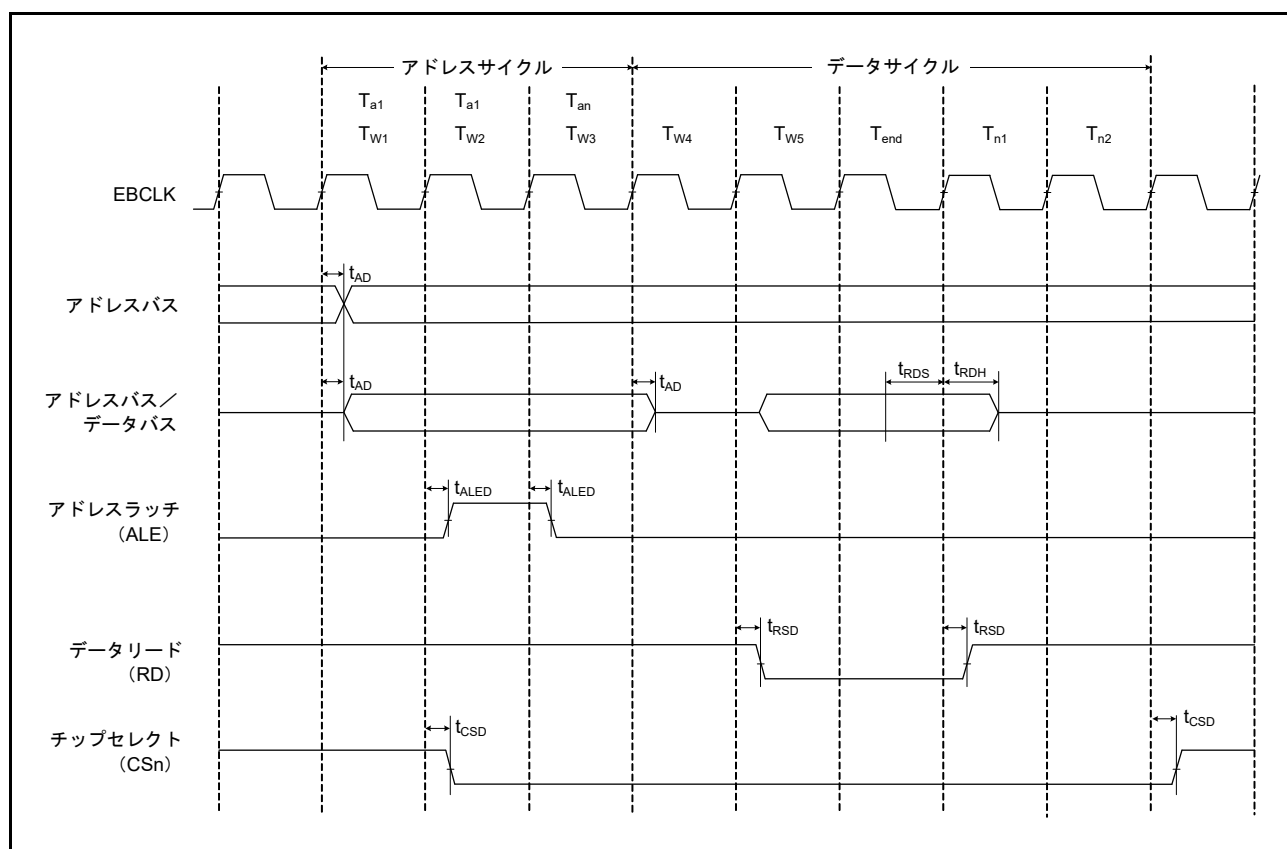
図 52.20 アドレス/データマルチプレクスバスのリードアクセスタイミング
