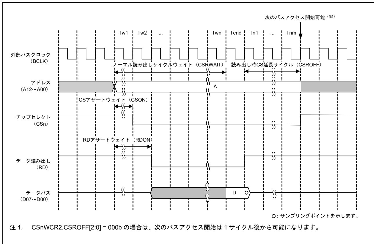
図 15.5 ノーマルリードアクセスのバスタイミング (n = 0, 1, 4 ~ 7)
