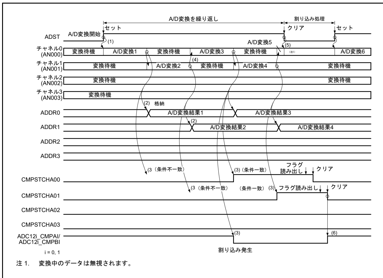
図 42.31 コンペア機能の動作例 (AN000 ~ AN003 を比較)
