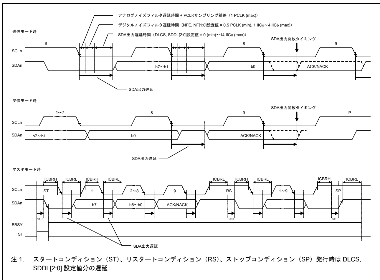
図 32.22 SDA 出力遅延機能
