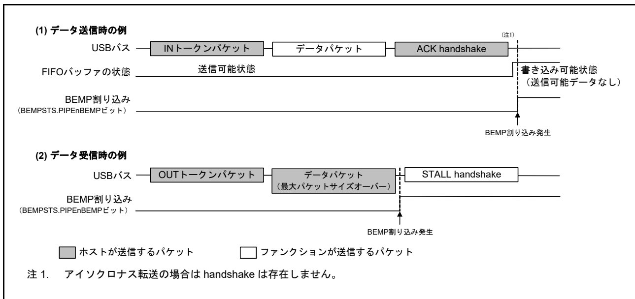
図 29.13 デバイスコントローラモード時の BEMP 割り込み発生タイミング
