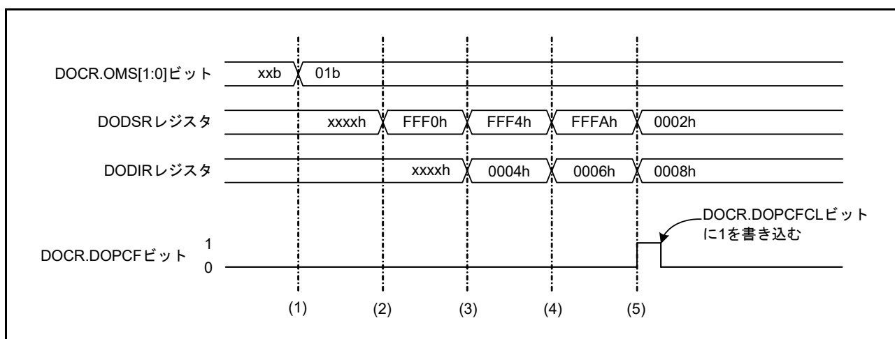
図 47.3 データ加算モードの動作例
