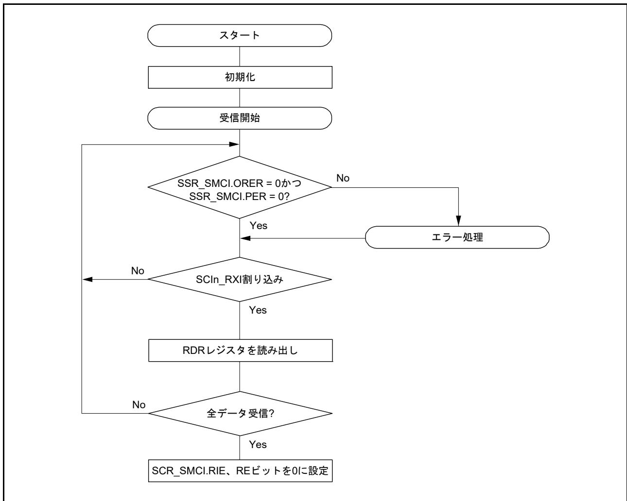
図 30.56 スマートカードインタフェース受信のフローチャート例
