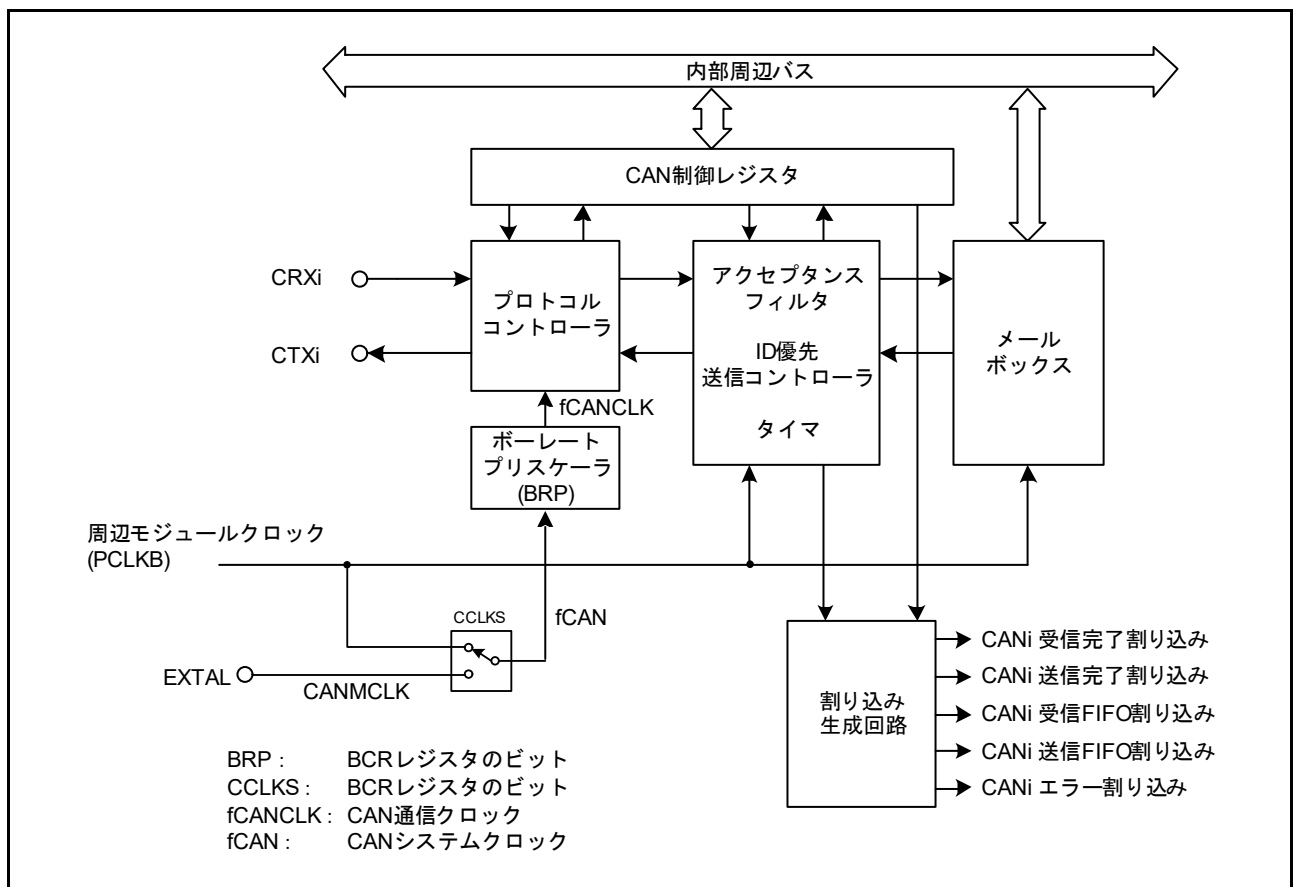
図 33.1 CAN モジュールブロック図 (i = 0, 1)
