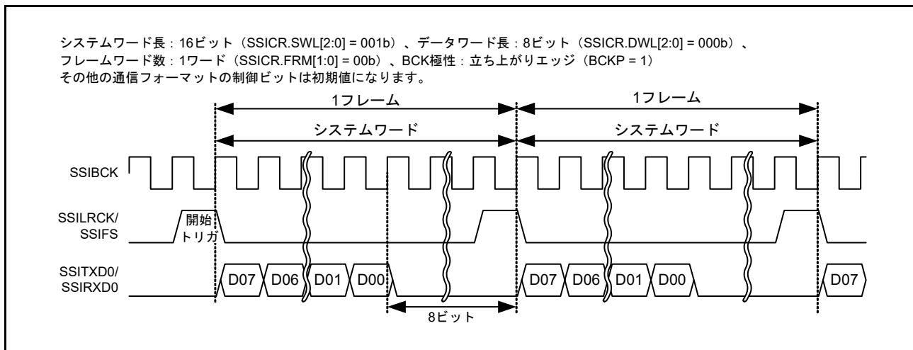
図 37.38 モノラルフォーマットでのショートフレーム (パディングあり、システムワード長 > データワード長)
