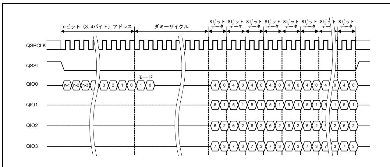
図 35.23 XIP モード時のファストリード Quad 出力バスサイクル
