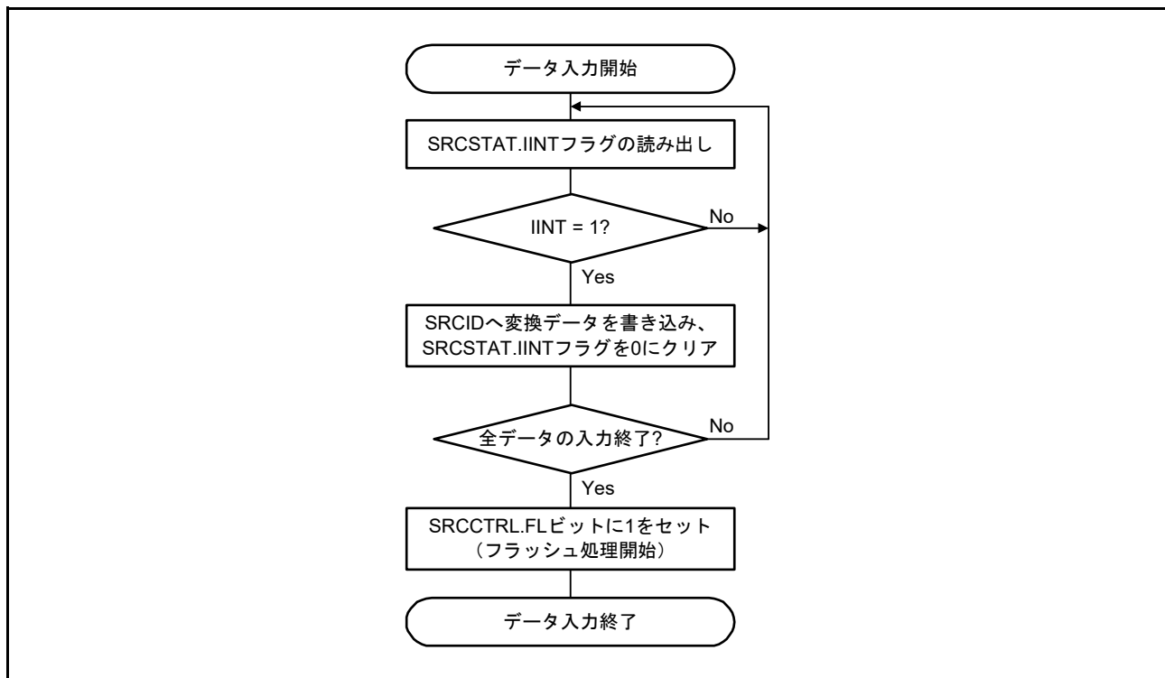
図 38.3 データ入力フロー
