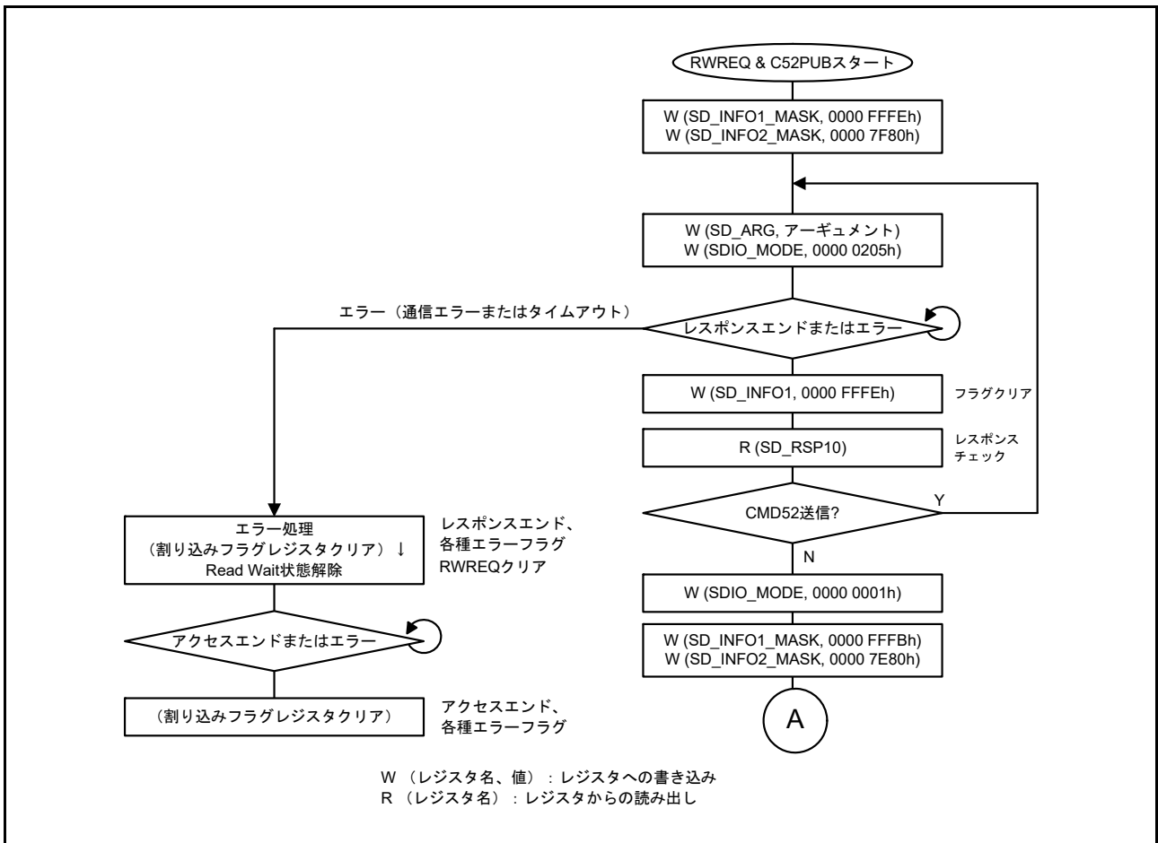
図 39.18 SD ホストインタフェースが Read Wait 状態で、CMD53 マルチブロックリード時に CMD52 (SDIO none abort) が送信される場合のフロー
