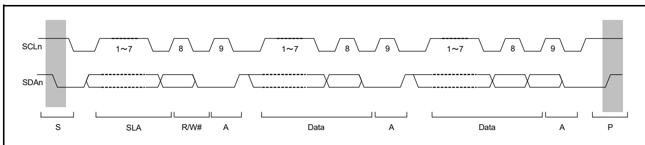
図 32.4 I 2 C バスタイミング (SLA 設定値 = 7 ビットの場合)
