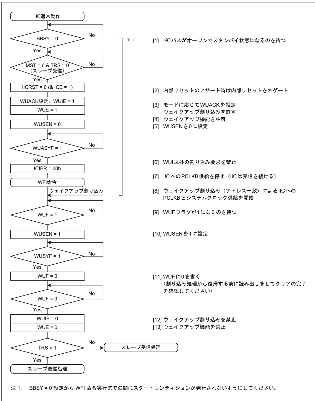
図 32.33 ノーマルウェイクアップモード 2 の動作例 (スレーブアドレス一致時のウェイクアップ割り込みによるウェイクアップの場合)
