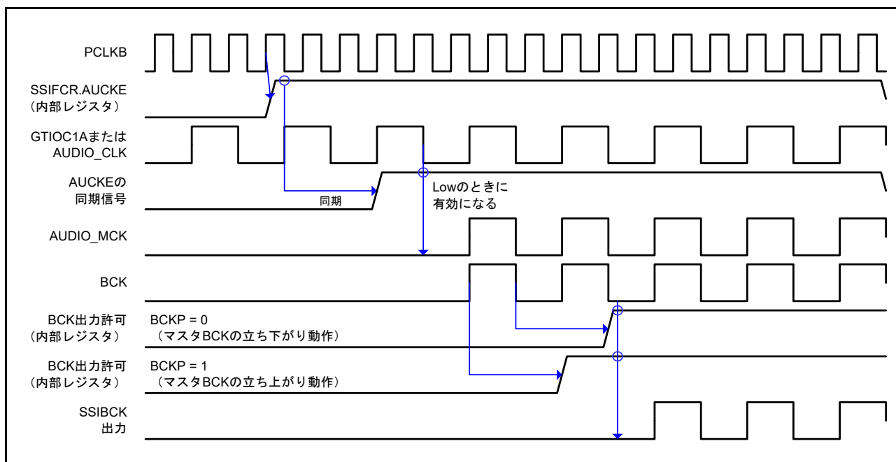
図 37.25 システムリセットからマスタモード通信開始までの動作のタイミング図
