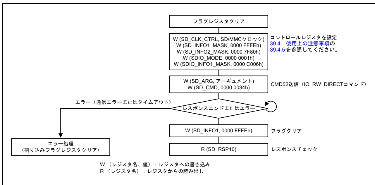
図 39.15 IO_RW_DIRECT コマンド (CMD52) 動作の例
