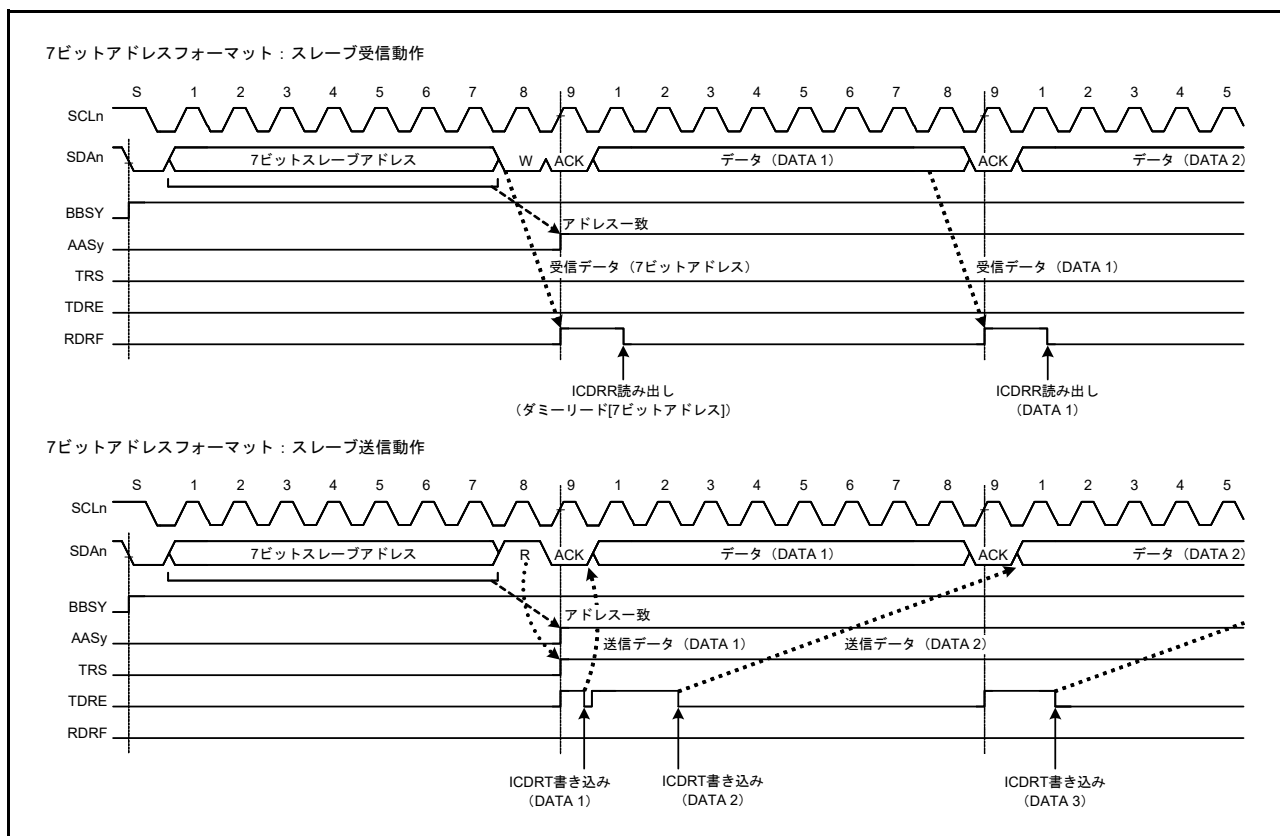
図 32.24 AAS y フラグが 1 になるタイミング (7 ビットアドレスフォーマット)
