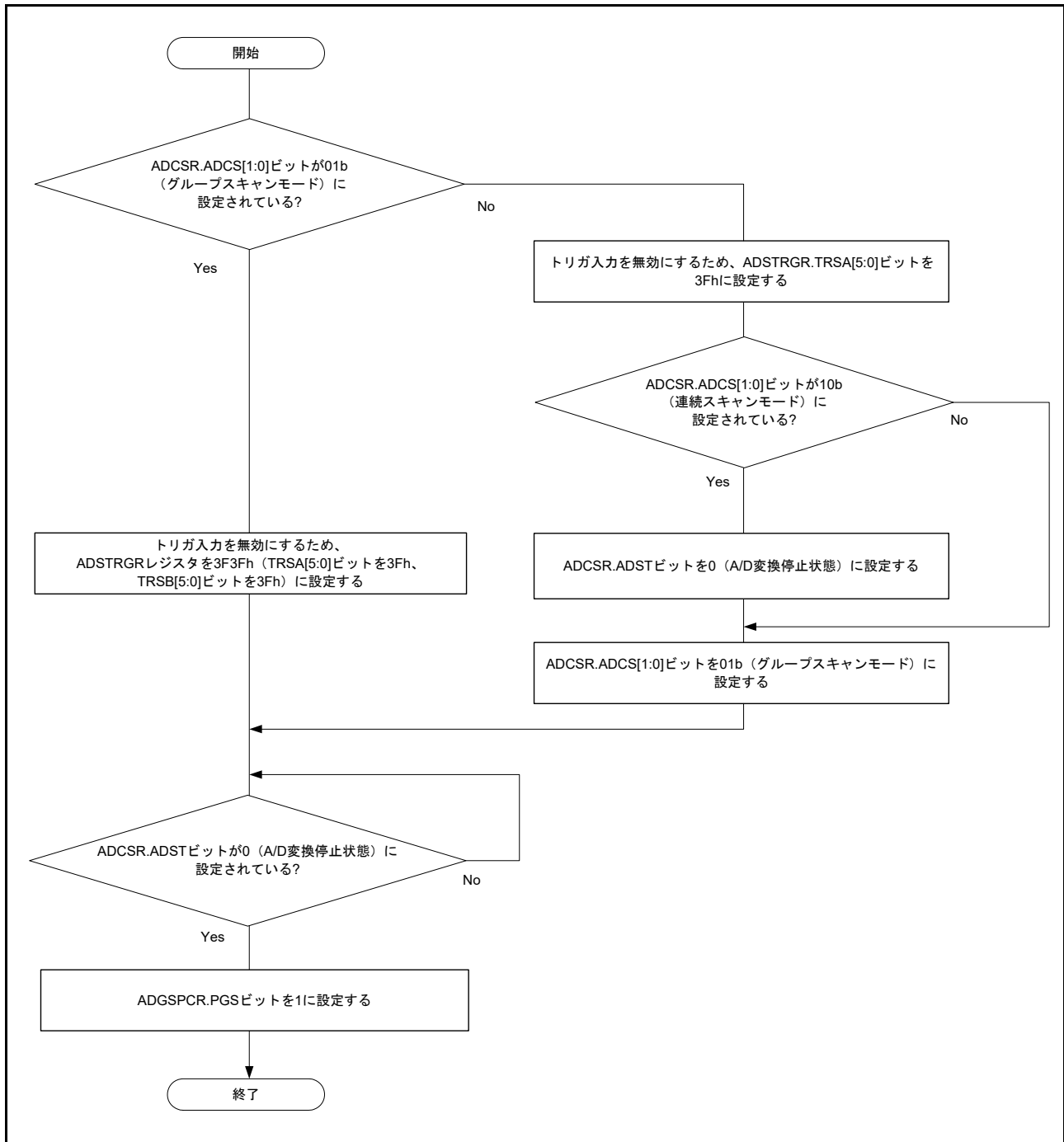
図 42.25 ADGSPCR.PGS ビット設定時のフロー
