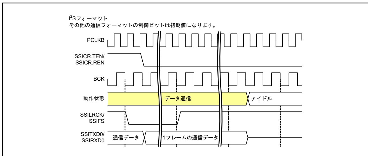
図 37.47 データ通信からの停止 (パディングビットなし)
