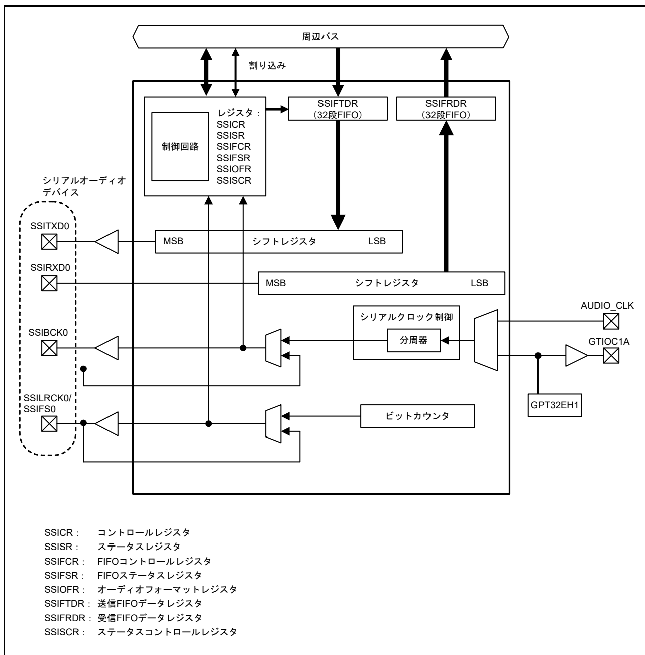
図 37.2 全二重通信の SSIE ブロック図 (SSIE0)
