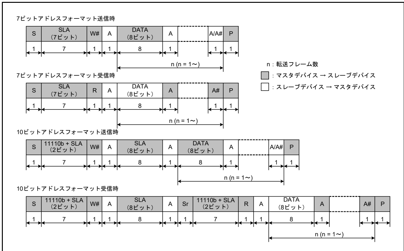
図 30.58 I 2 C バスフォーマット
