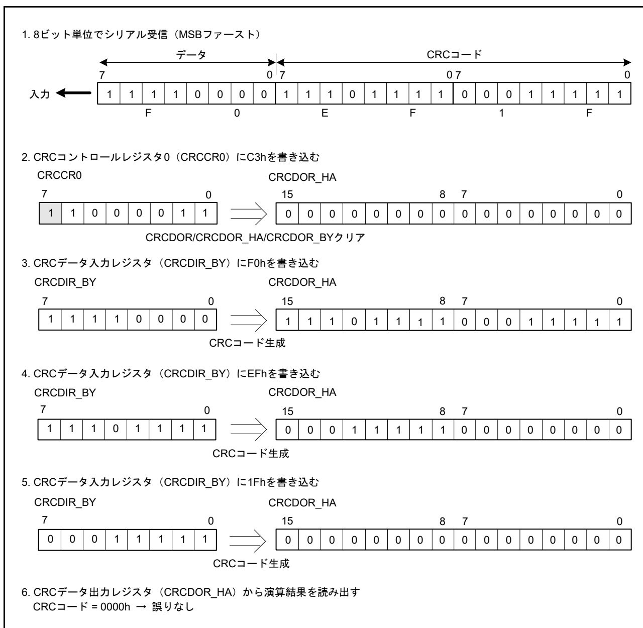
図 36.5 MSB ファーストのデータ受信
