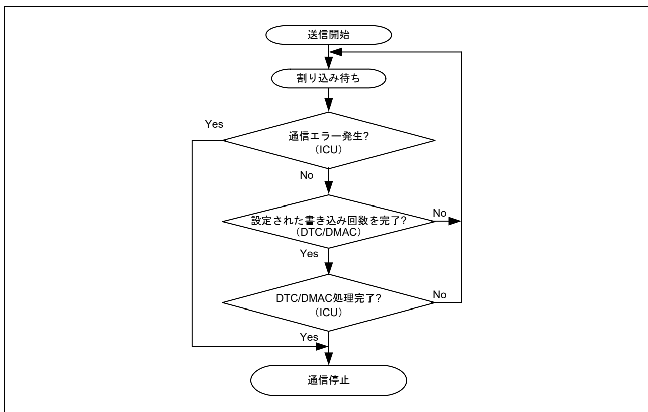
図 37.53 送信手順
