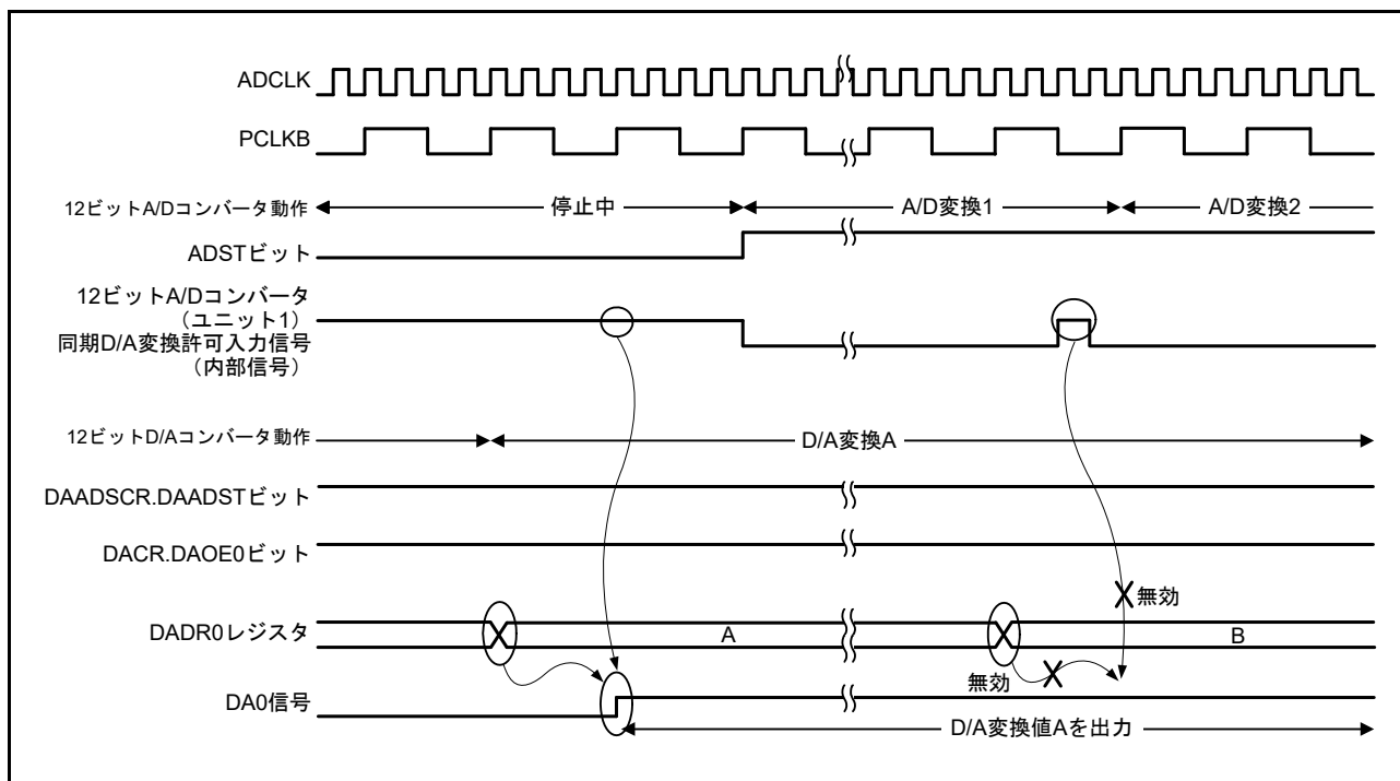
図 43.4 DAC12 が ADC12 (ユニット 1) からの同期 D/A 変換許可入力信号を取り込めない場合の例
