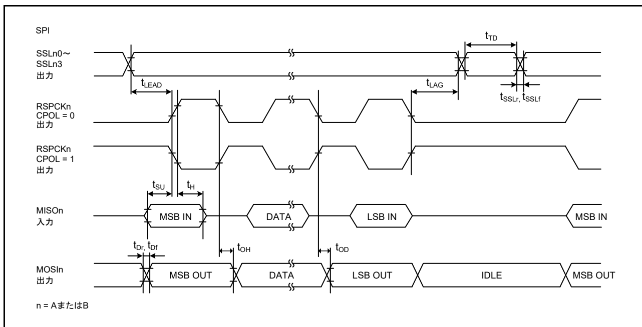
図 52.45 CPHA = 0 の場合におけるマスタの SPI タイミング
