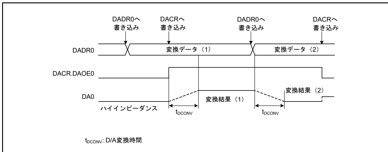
図 43.2 DAC12の動作例
