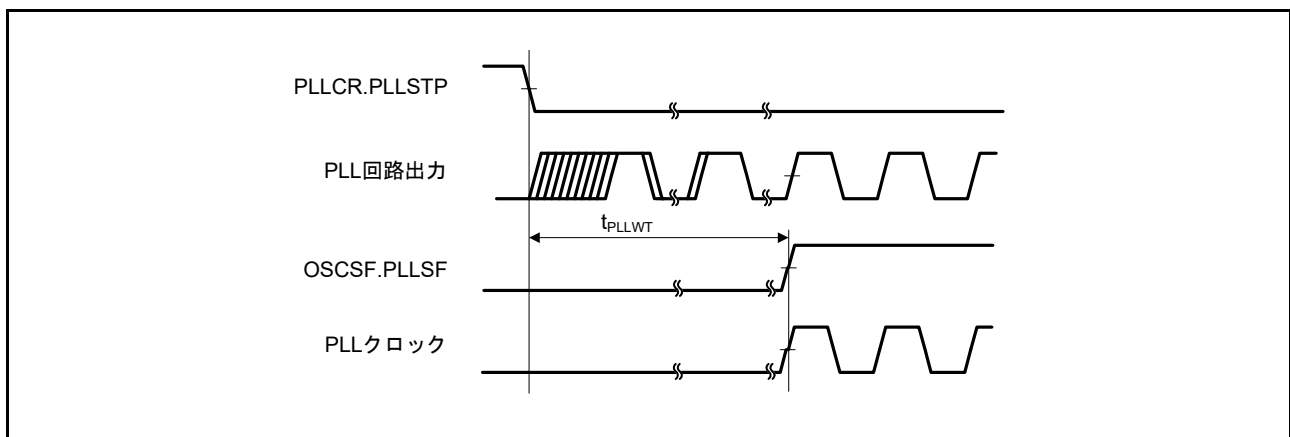
図 52.11 PLL クロック発振開始タイミング
