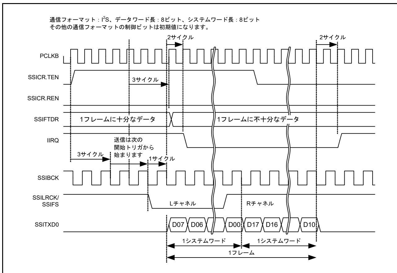
図 37.13 IIRQ 設定タイミング (送信)
