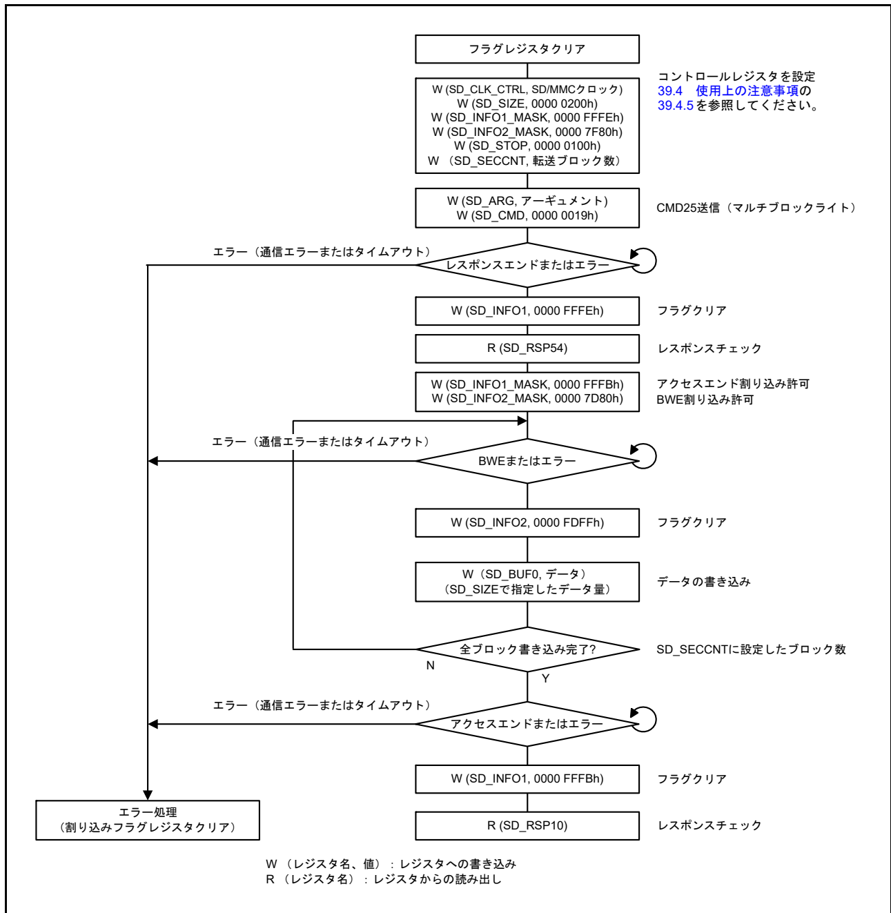
図 39.13 内蔵タイマによるマルチブロックライト動作の例
