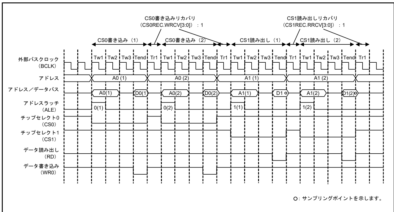
図 15.34 アドレス/データマルチプレクス I/O インタフェース時、バスアクセスが分割された場合のリカバリサイクルの挿入例
