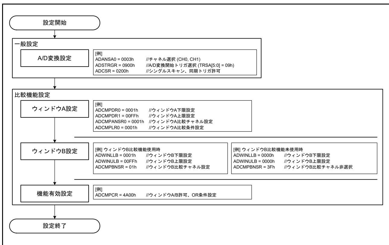
図 42.32 コンペア機能のイベント出力使用時の設定例
