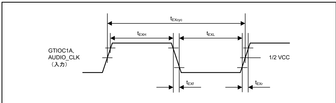
図 52.55 クロック入力タイミング
