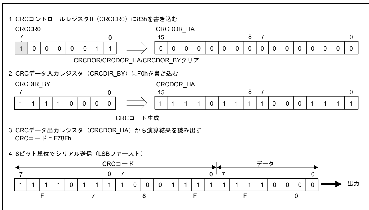
図 36.2 LSB ファーストのデータ送信
