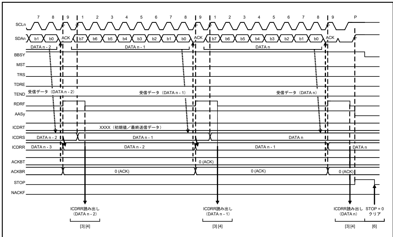
図 32.20 スレーブ受信の動作タイミング (2) (RDRFS = 0 の場合)
