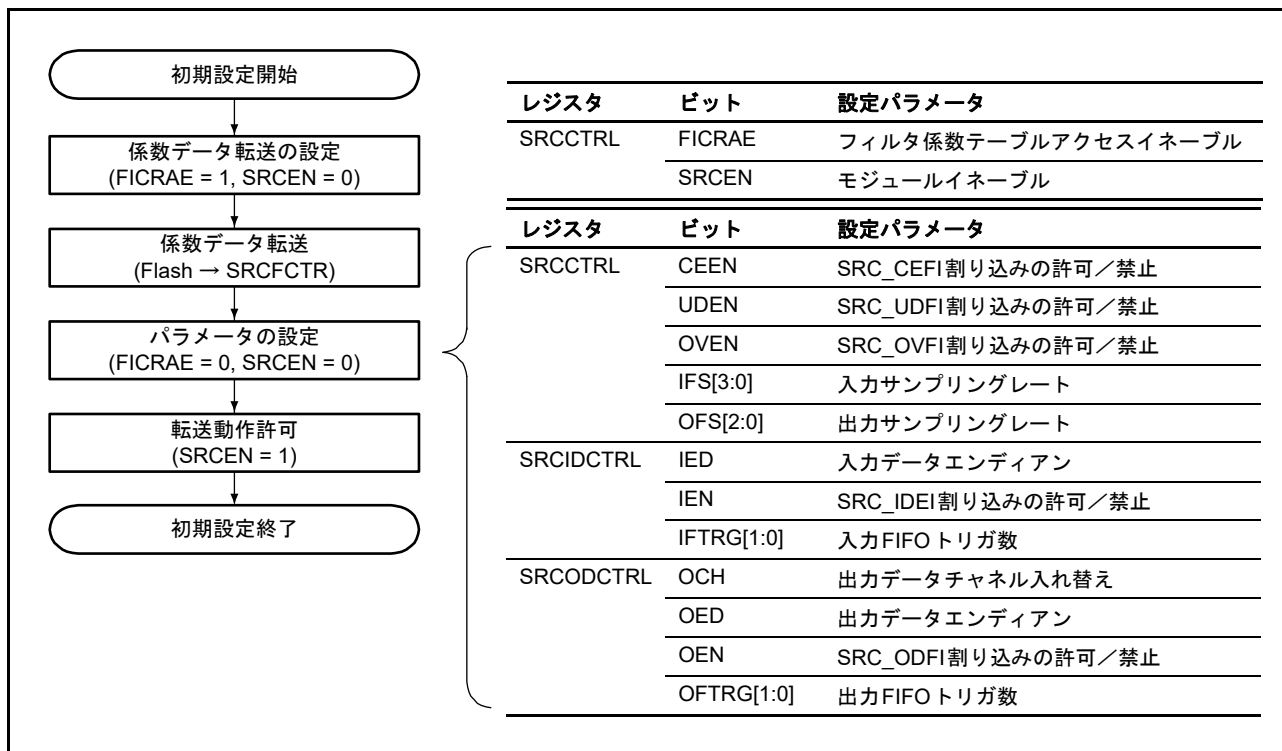
図 38.2 初期設定のフロー例
