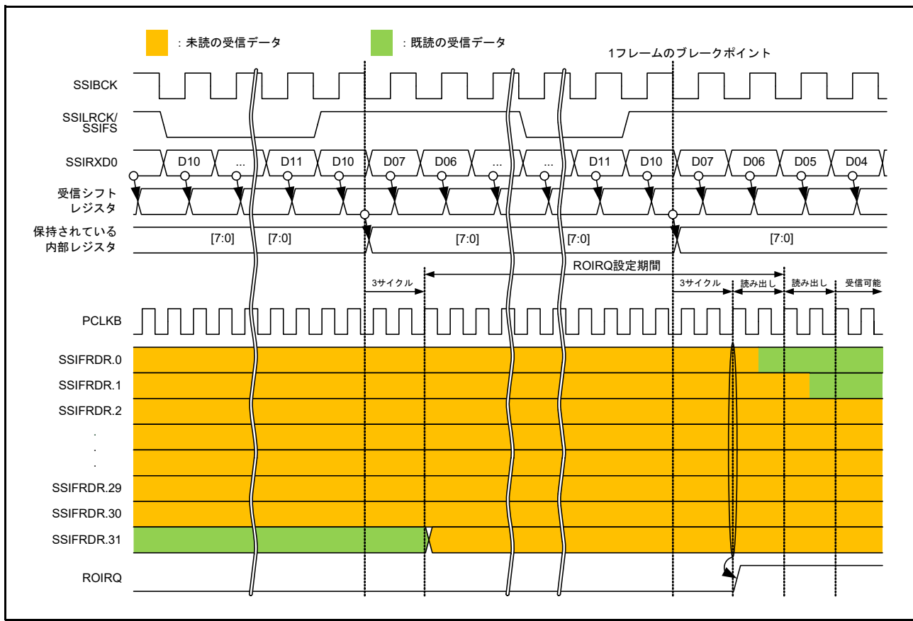
図 37.15 ROIRQ 設定タイミング
