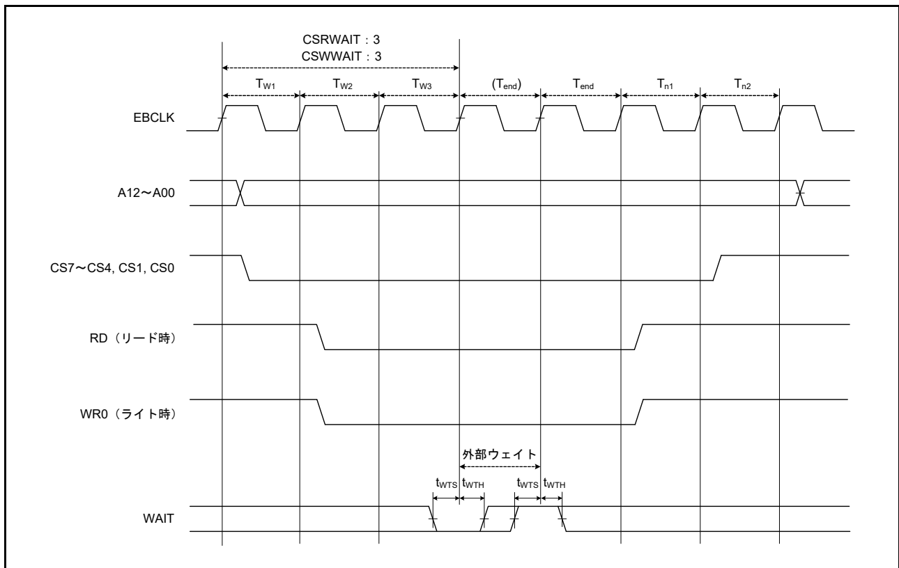
図 52.26 外部ウェイト制御の外部バスタイミング
