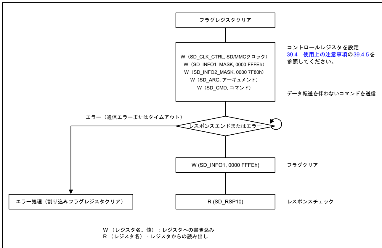
図 39.9 データがないコマンドのフロー例
