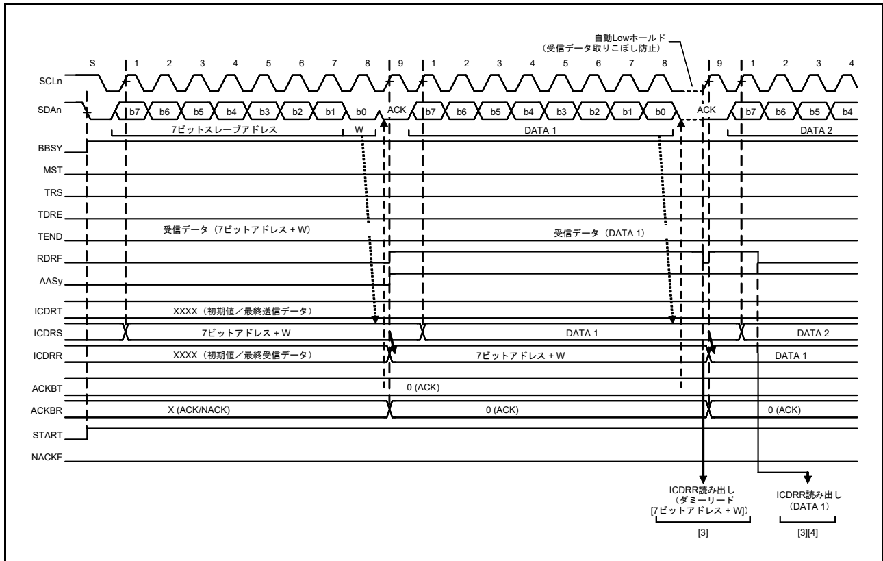
図 32.19 スレーブ受信の動作タイミング (1) (7 ビットアドレスフォーマットで RDRFS = 0 の場合)
