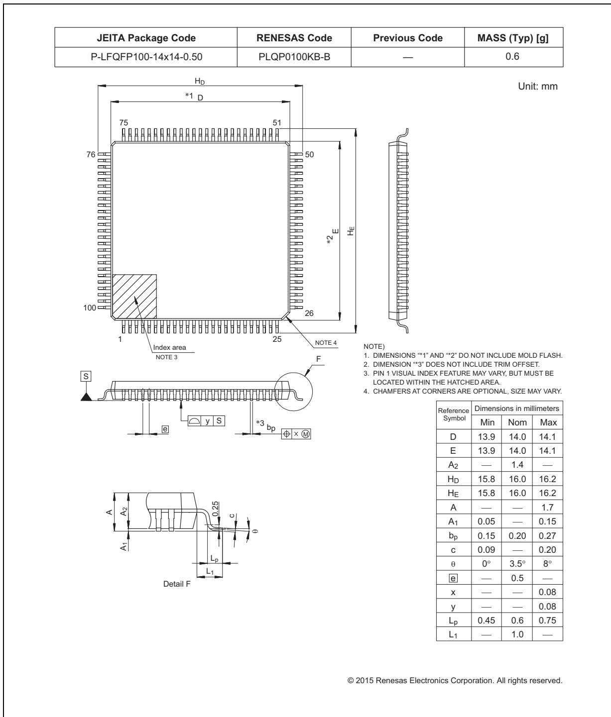
図 2.2 100 ピン LQFP
