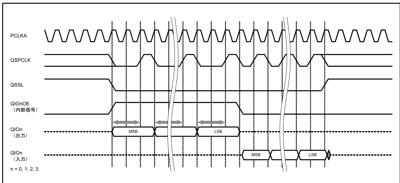
図 35.13 SFMOSW ビットを使用したシリアルデータ出力のセットアップ時間調整
