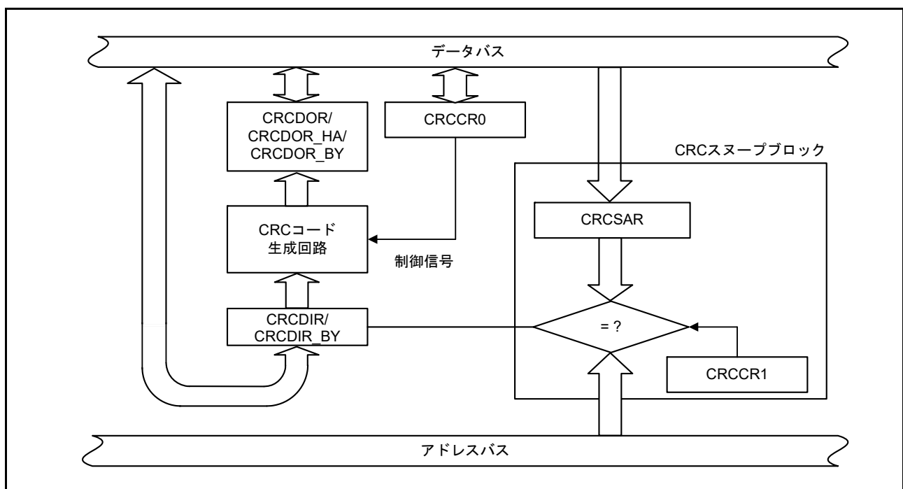
図 36.1 CRC 演算器のブロック図
