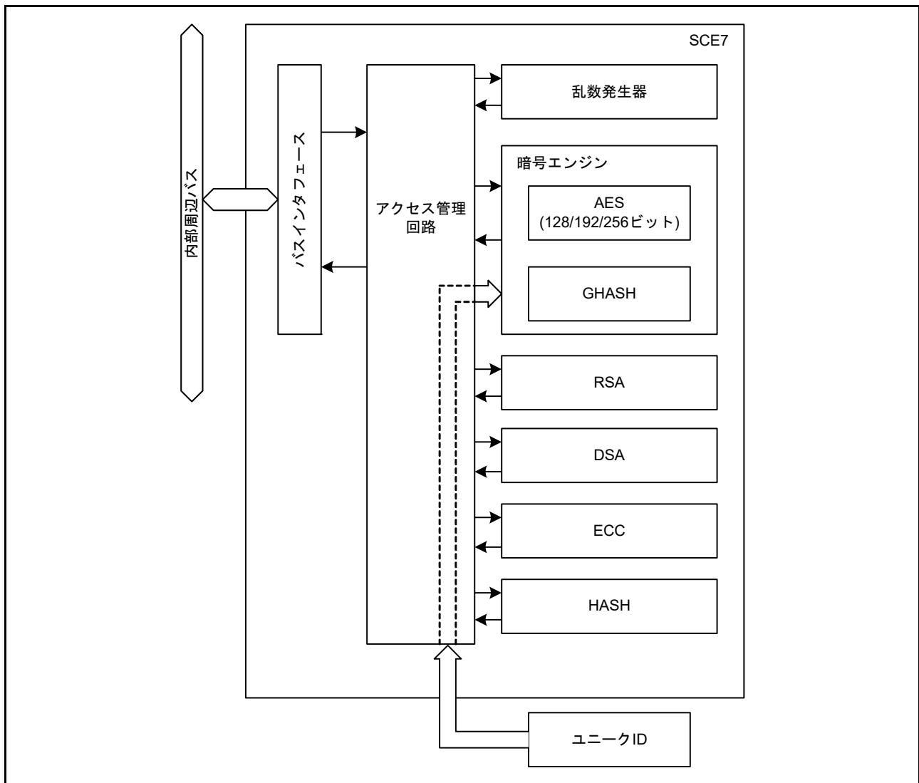
図 41.1 SCE7 ブロック図
