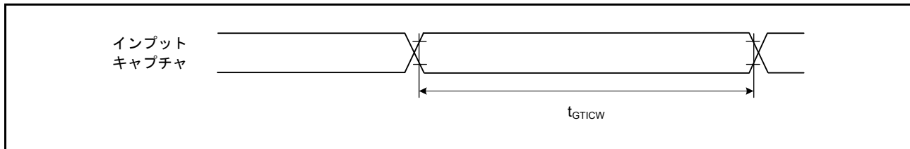
図 52.29 GPT32 インพุットキャプチャタイミング
