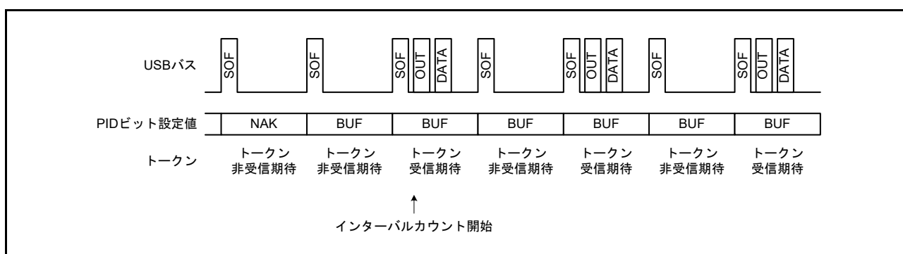
図 29.19 IITV[2:0] ≠ 0 の場合のフレームとトークン受信期待の関係
