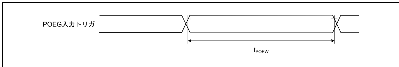
図 52.28 POEG 入力トリガタイミング
