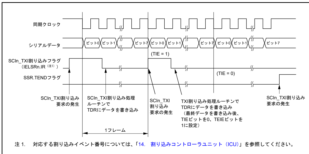
図 30.36 クロック同期式モードにおけるシリアル送信の動作例 (送信中～送信終了時)
