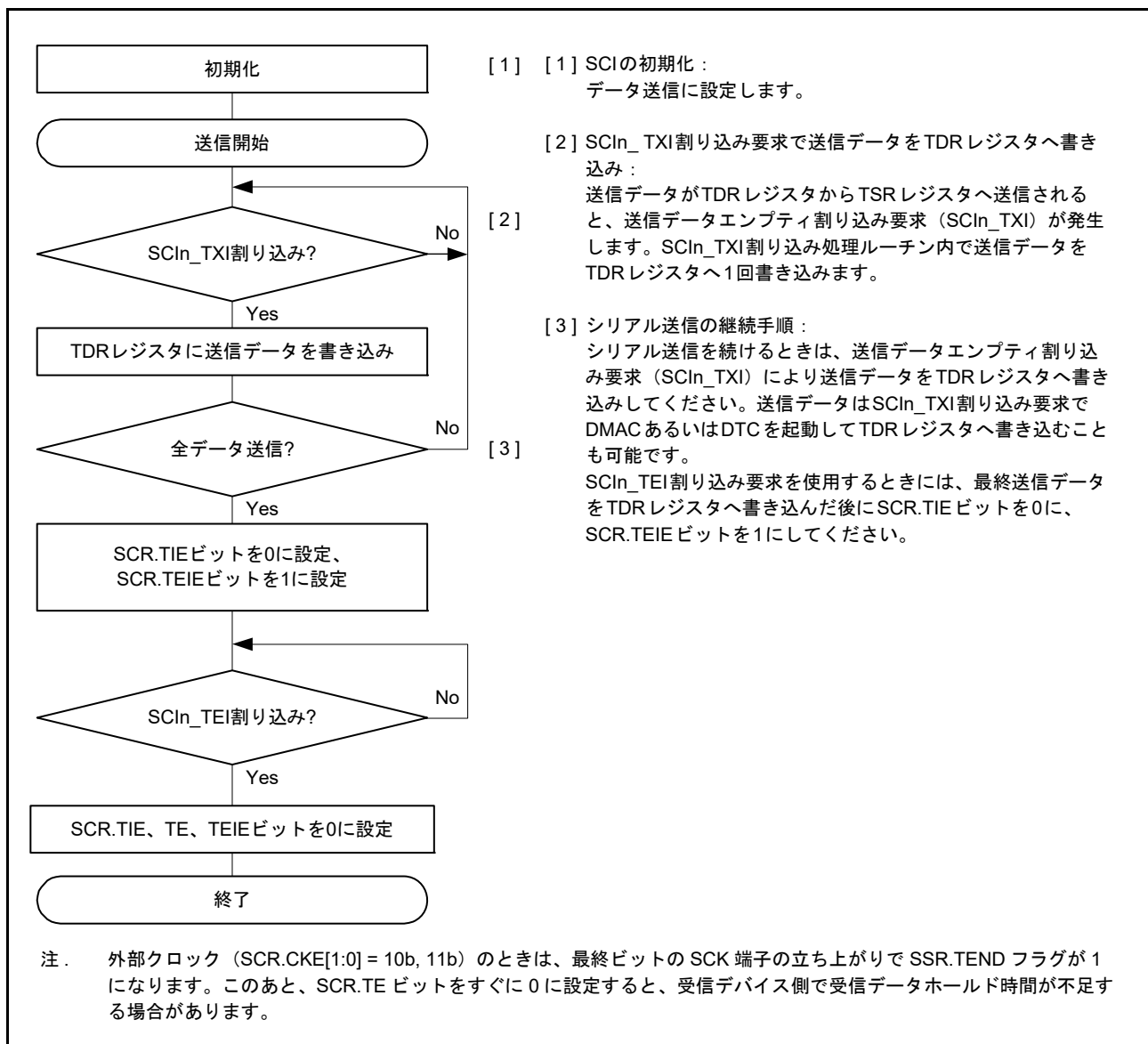
図 30.37 クロック同期式モードにおけるシリアル送信のフローチャート例 (非 FIFO 選択時)
