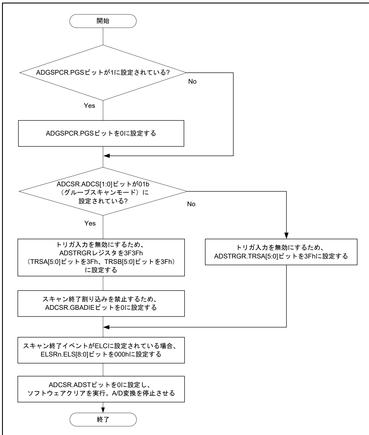
図 42.40 ソフトウェアによる ADCSR.ADST ビットのクリア手順
