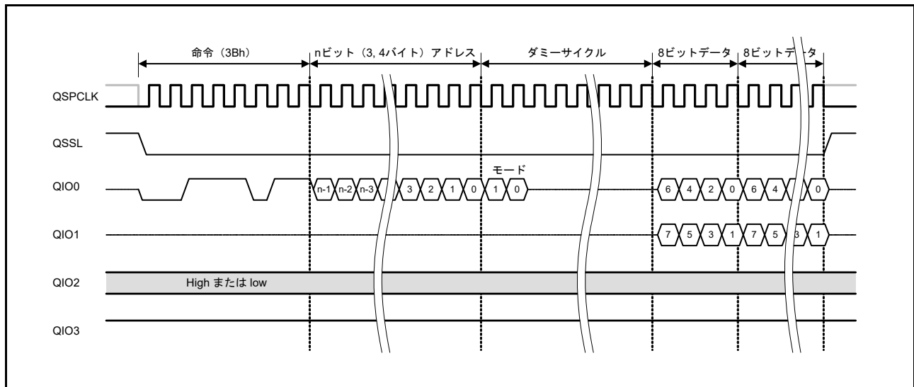
図 35.18 ファストリード Dual 出力バスサイクル
