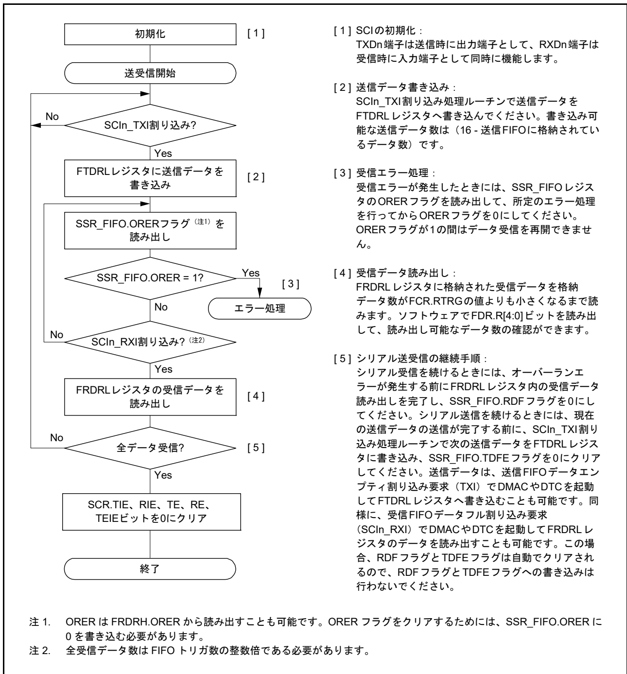
図 30.44 クロック同期モードにおけるシリアル同時送受信動作のフローチャート例 (FIFO 選択時)
