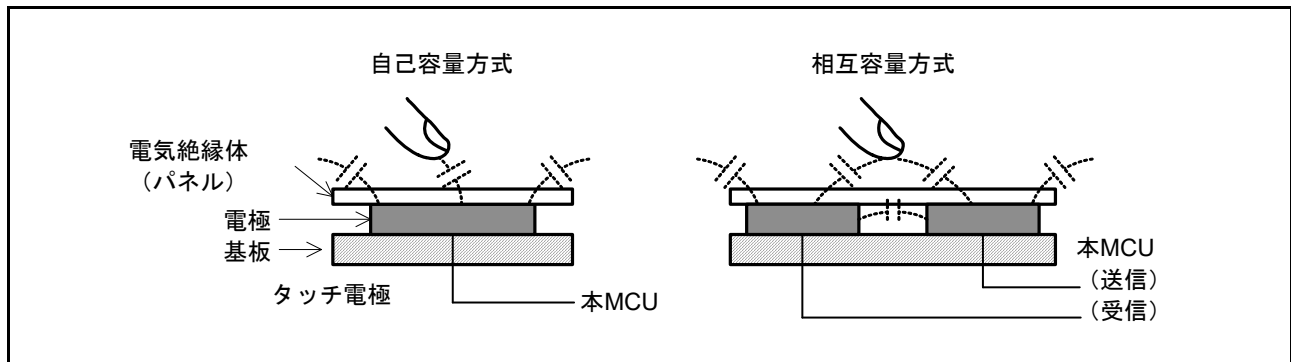
図 46.2 自己容量方式と相互容量方式
