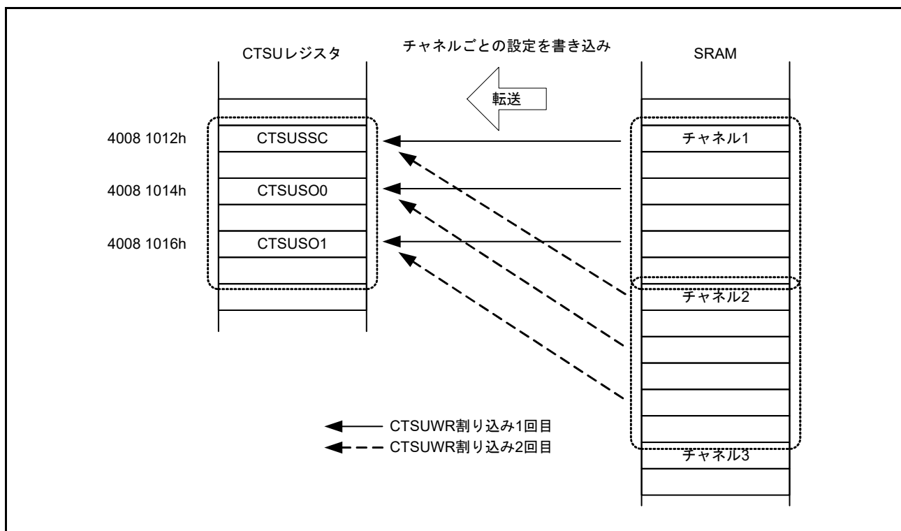
図 46.19 CTSUS_CTSUWR 割り込みを用いた DTC 転送動作例
