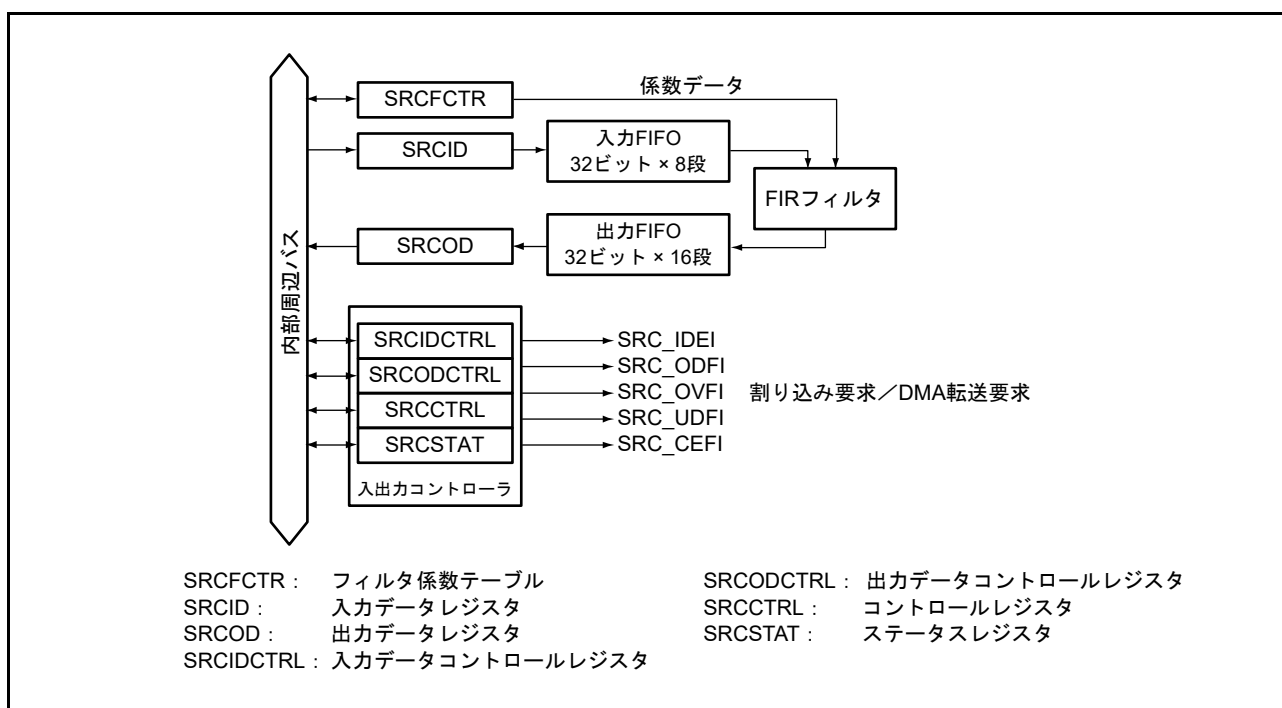
図 38.1 SRCのブロック図
