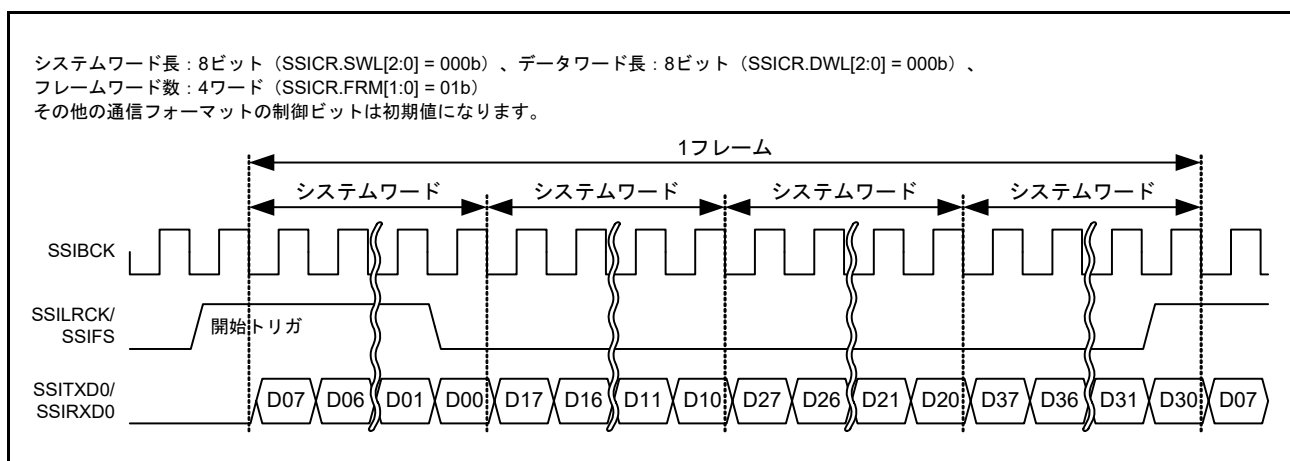
図 37.40 TDM フォーマット (パディングなし、システムワード長 = データワード長)
