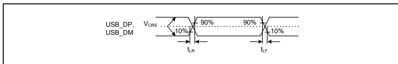
図 52.60 Low-speed モードにおける USB_DP、USB_DM の出力タイミング
