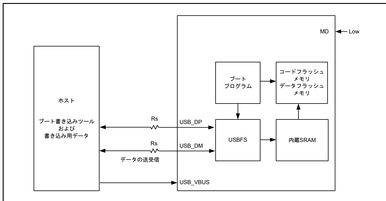
図 50.13 USB ブートモード時のシステム構成
