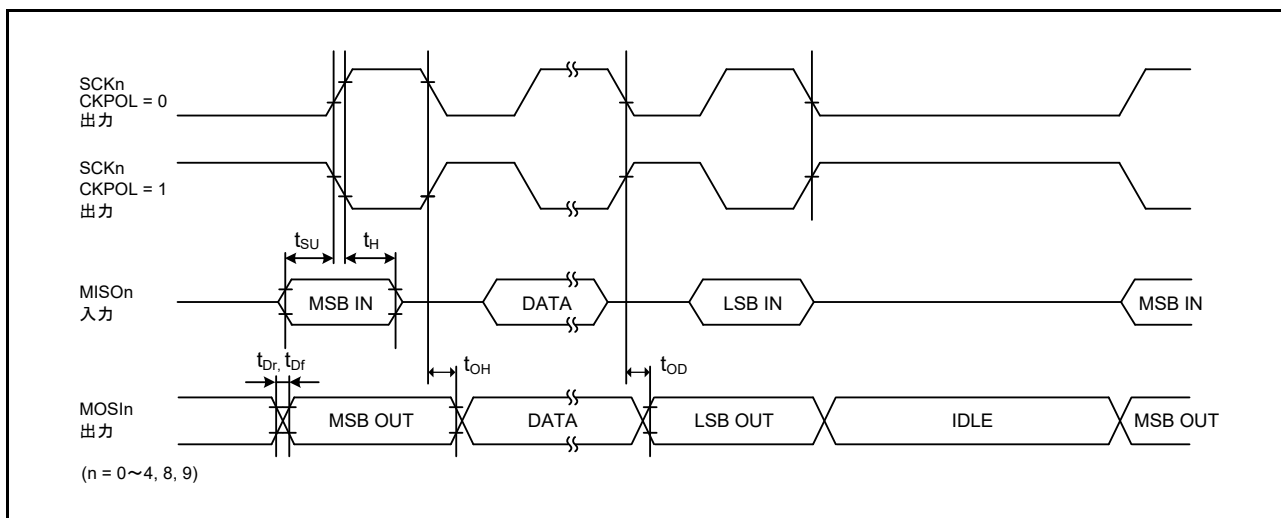
図 52.39 CKPH = 1 の場合におけるマスタの SCI 簡易 SPI モードタイミング
