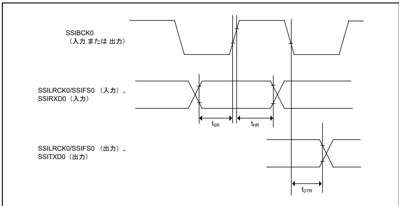
図 52.56 SSICR.BCKP = 0 の場合の SSIE データ送受信タイミング
