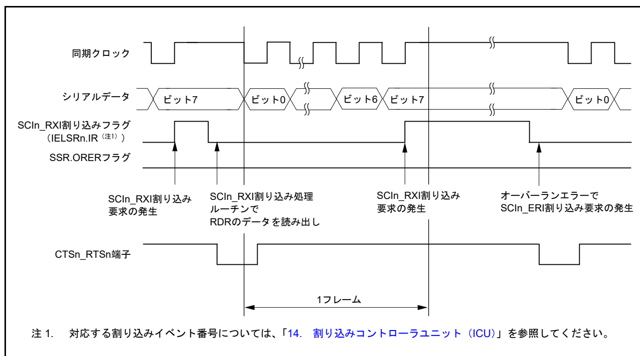
図 30.40 クロック同期式モードにおけるシリアル受信の動作例 (2) (RTS 機能を使用する場合)
