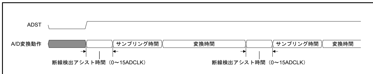
図 42.36 断線検出アシスト機能を使用した場合のA/D変換動作
