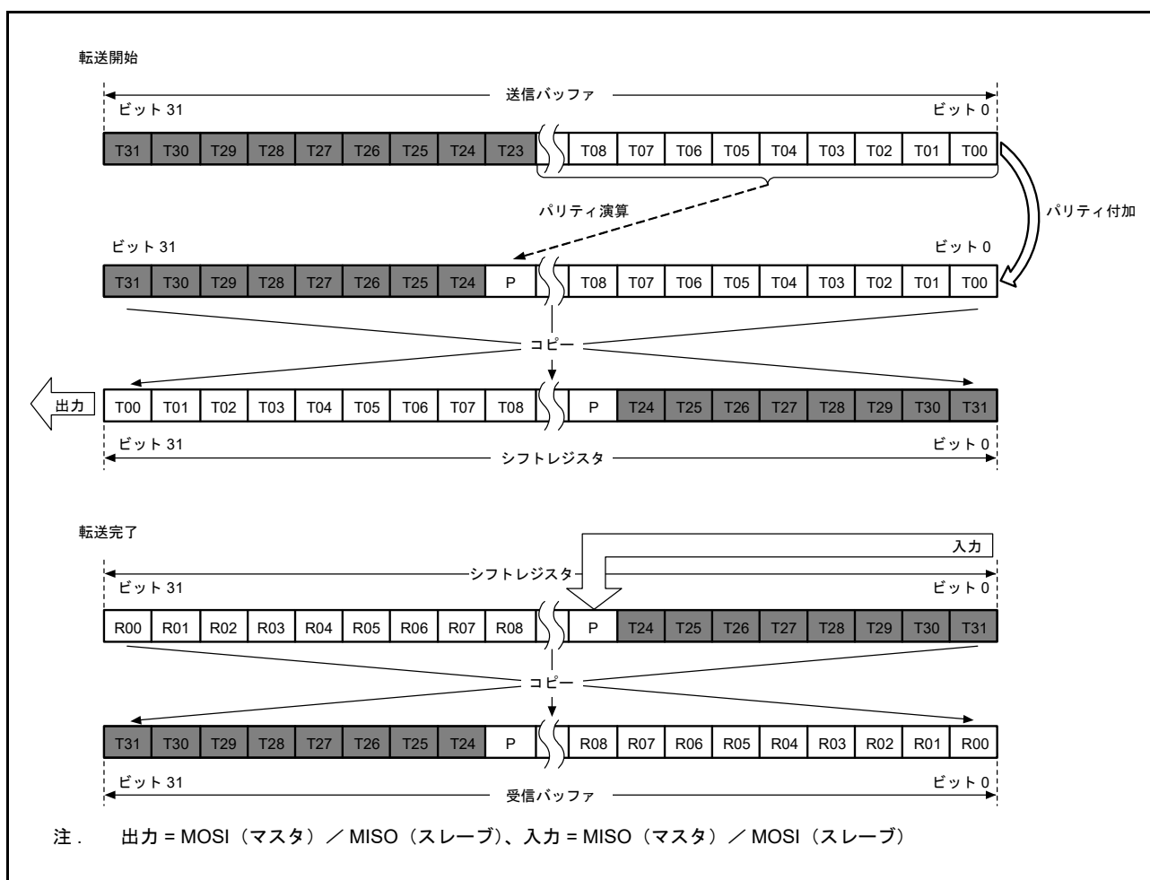
図 34.21 LSB ファースト転送 (24 ビットデータ / パリティ機能有効)
