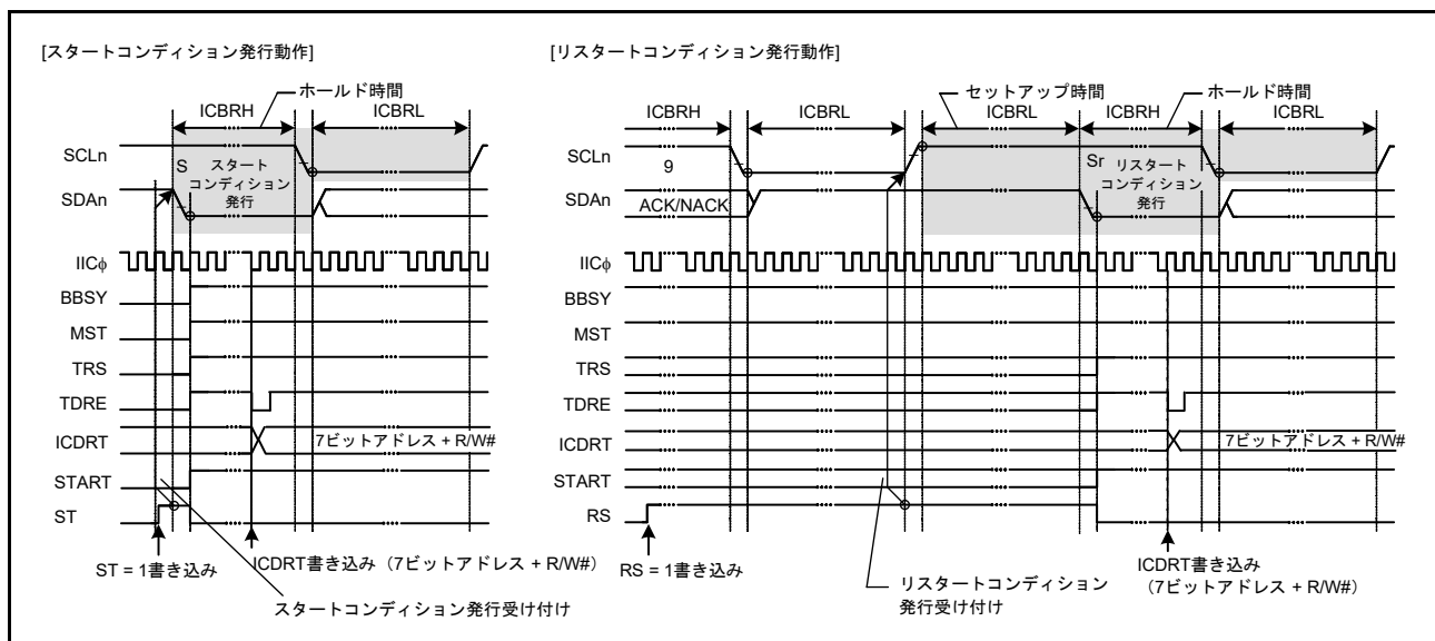
図 32.45 スタートコンディション、リスタートコンディションの発行動作タイミング (ST および RS ビットの使用)
