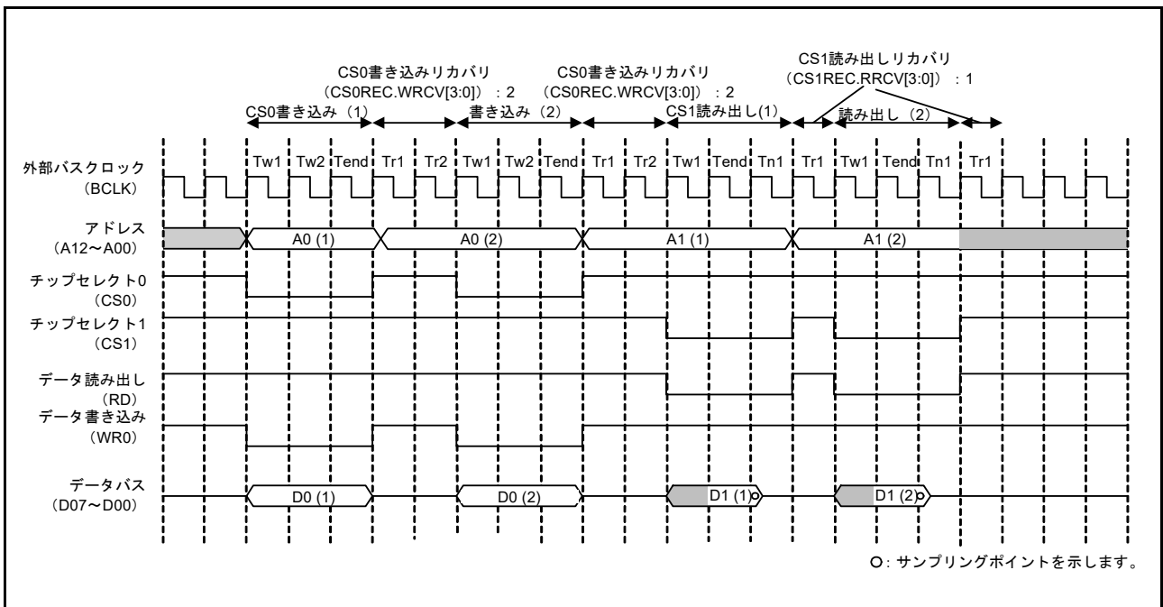
図 15.30 バスアクセスが分割された場合のリカバリサイクルの挿入例 (セパレートバスインタフェースによるノーマルアクセスの場合)
