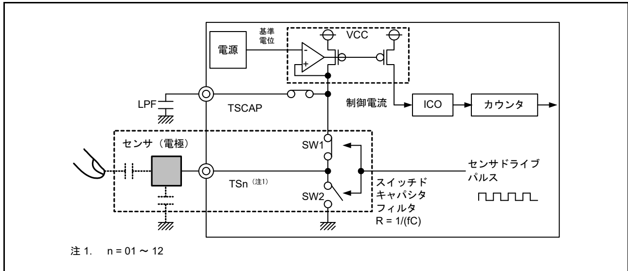
図 46.4 計測部回路
