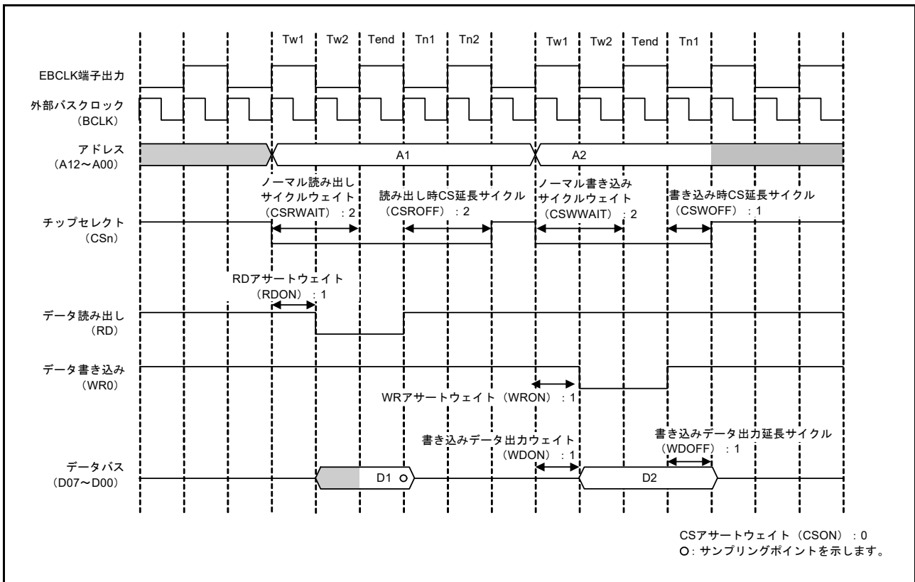
図 15.10 ノーマルアクセスの動作例 (EBCLK 端子出力選択ビットで BCLK の 2 分周を設定した場合) (n = 0, 1, 4 ~ 7)
