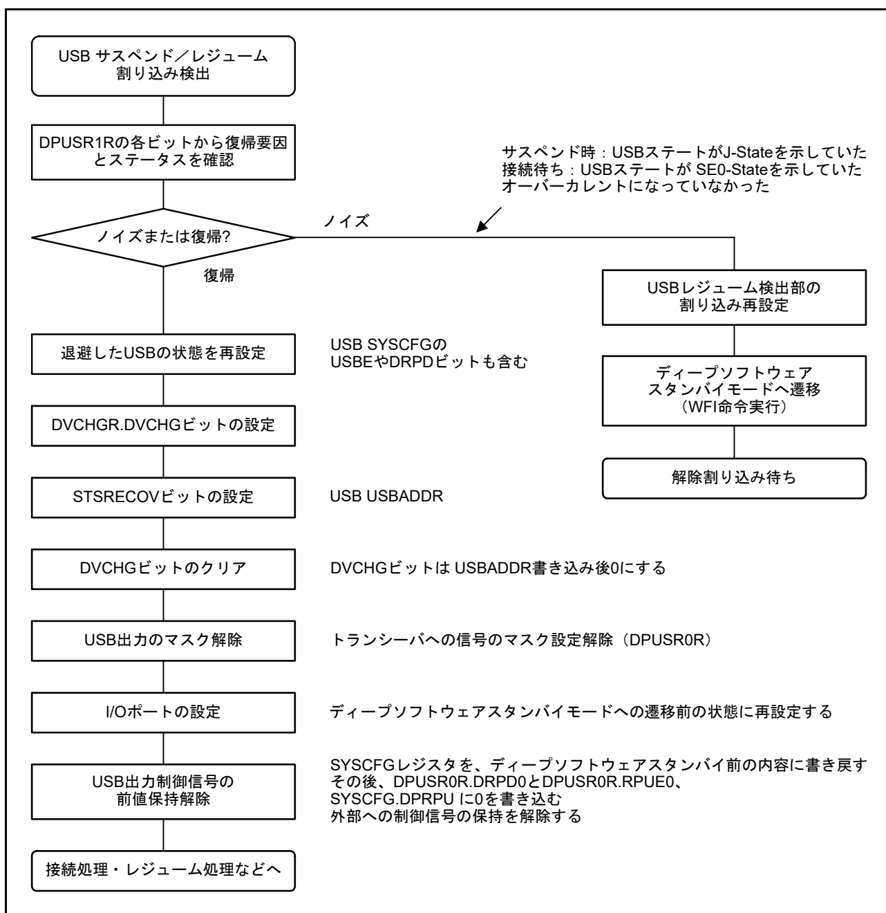
図 29.8 ホストコントローラ機能選択時におけるディープソフトウェアスタンバイモード解除時の USBFS 設定フロー
