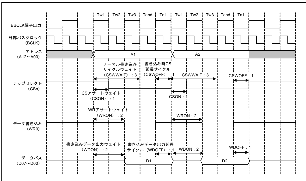
図 15.14 ノーマルライトアクセスの動作例 (EBCLK 端子出力選択ビットで BCLK の 2 分周を設定した場合、および 1 転送要求に対して 2 回バスアクセスが発生する場合) (n = 0, 1, 4 ~ 7)
