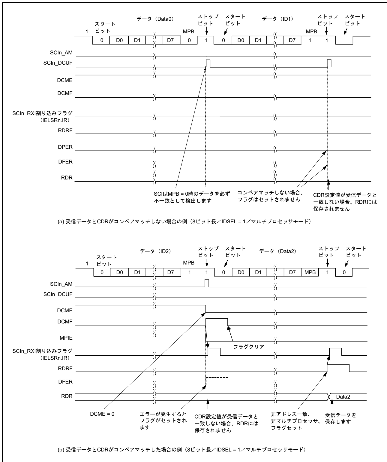
図 30.6 アドレス一致検出の例 (2) (マルチプロセッサモード)
