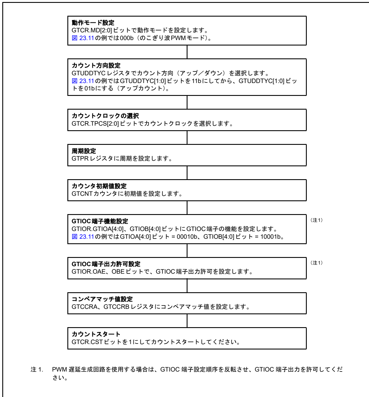
図 23.12 Low 出力 / High 出力動作設定例
