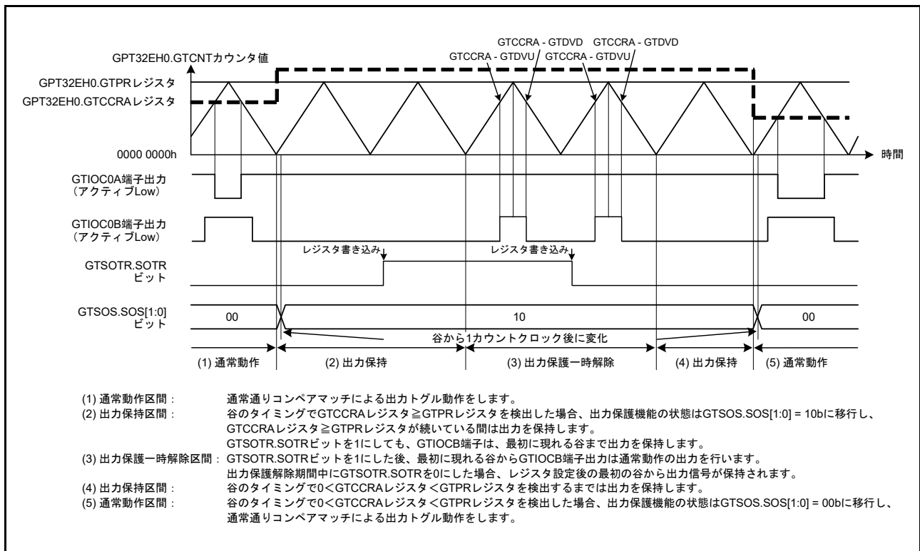
図 23.106 谷でのバッファ転送中に GTCRA レジスタ \geq GTPR レジスタとなった場合の出力保護機能一時解除例 (谷でのバッファ転送中に 0 < GTCRA レジスタ < GTPR レジスタを回復、アクティブ Low の場合)
