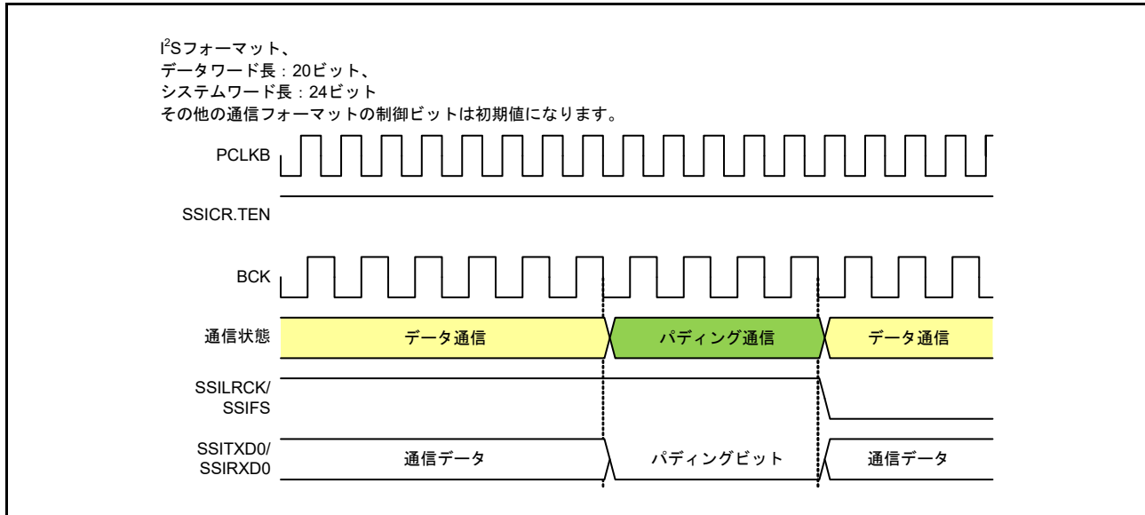
図 37.48 データ通信からパディング通信への遷移
