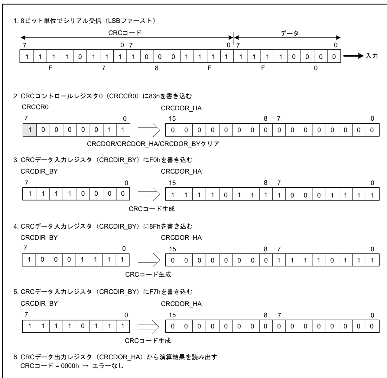
図 36.4 LSB ファーストのデータ受信
