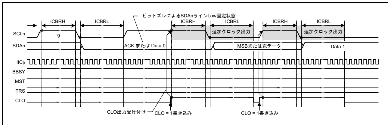
図 32.49 SCL クロック追加出力機能 (CLO ビットの使用)
