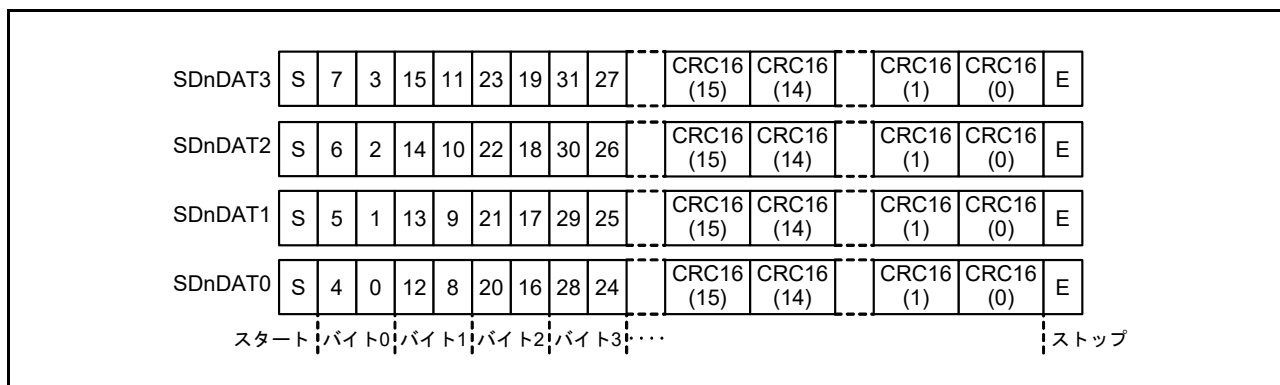
図 39.3 4 ビット幅モードの SDnDAT
