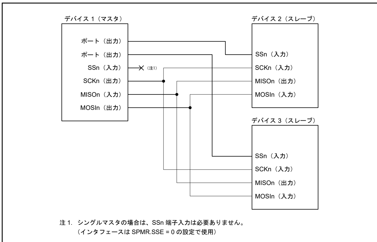
図 30.69 簡易 SPI モードでの接続例 (シングルマスタ時、SPMR.SSE ビット = 0)
