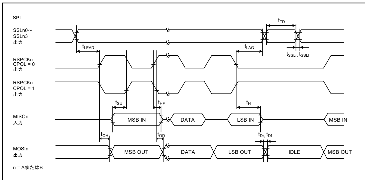
図 52.48 CPHA = 1 で、PCLKA/2 にビットレートが設定されている場合におけるマスタの SPI タイミング
