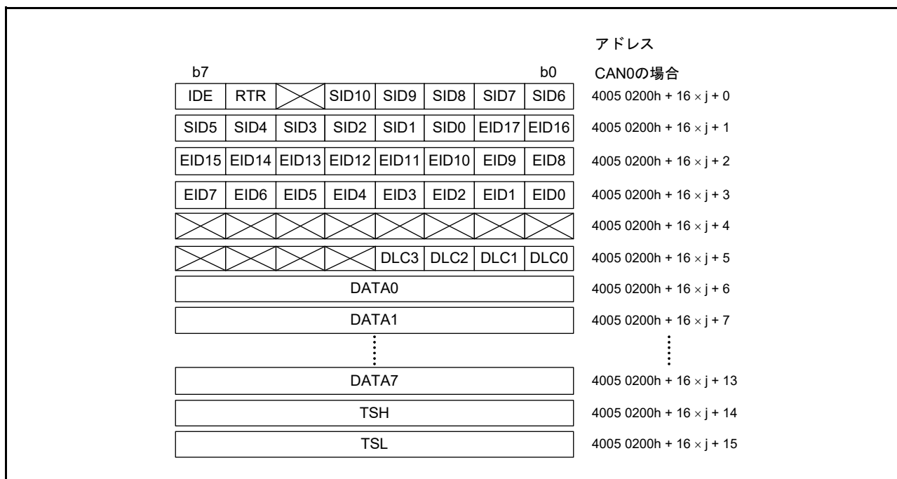
図 33.13 メールボックスレジスタの構成 (j = 0 ~ 31)
