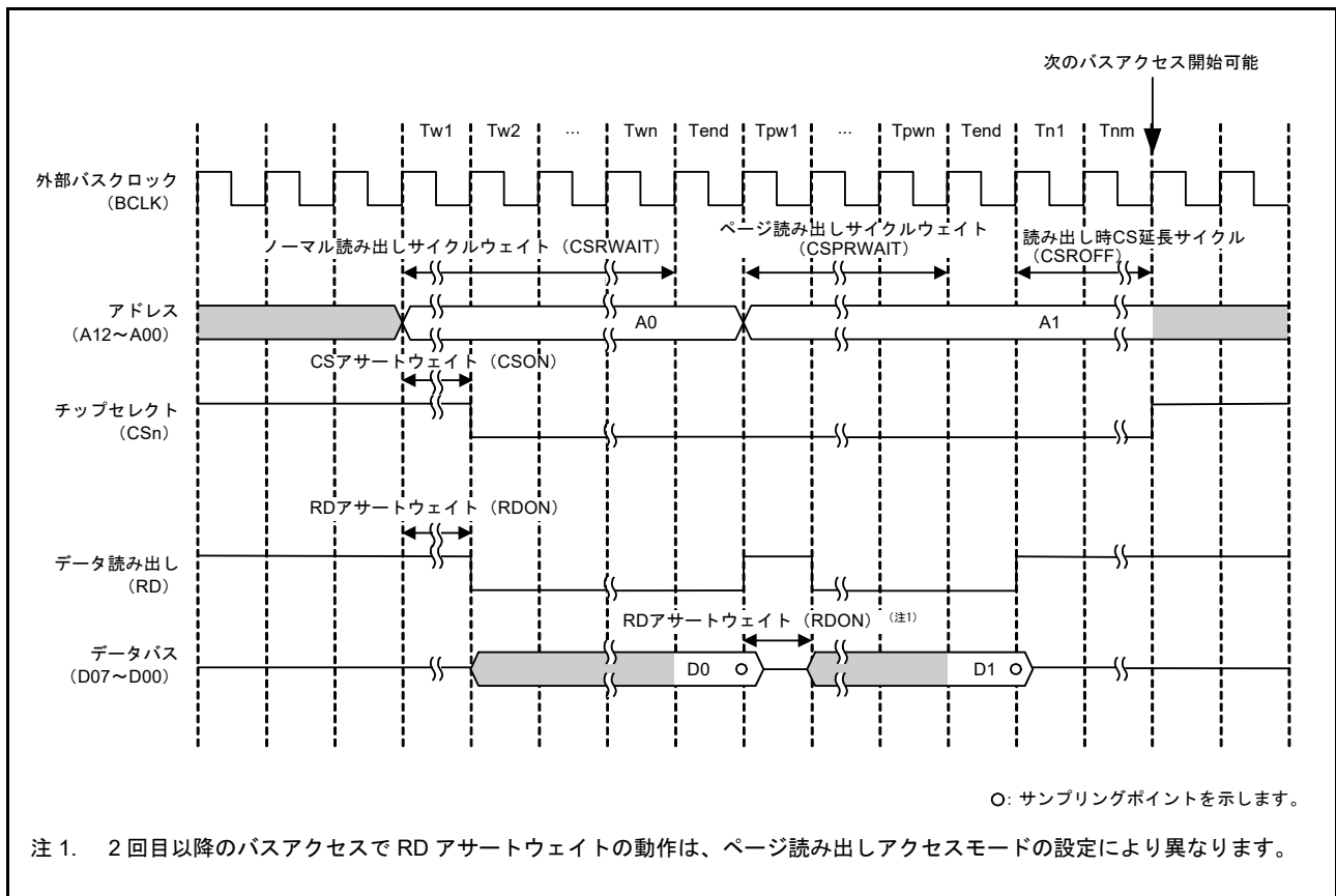
図 15.15 ページリードアクセスのタイミング (n = 0, 1, 4 ~ 7)
