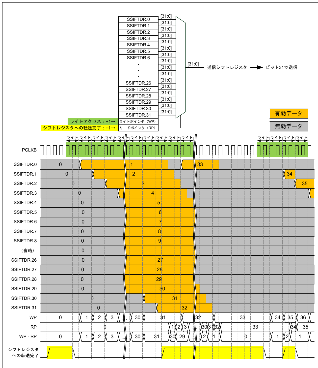
図 37.30 送信 FIFO データレジスタと送信シフトレジスタの構成および FIFO 動作例
