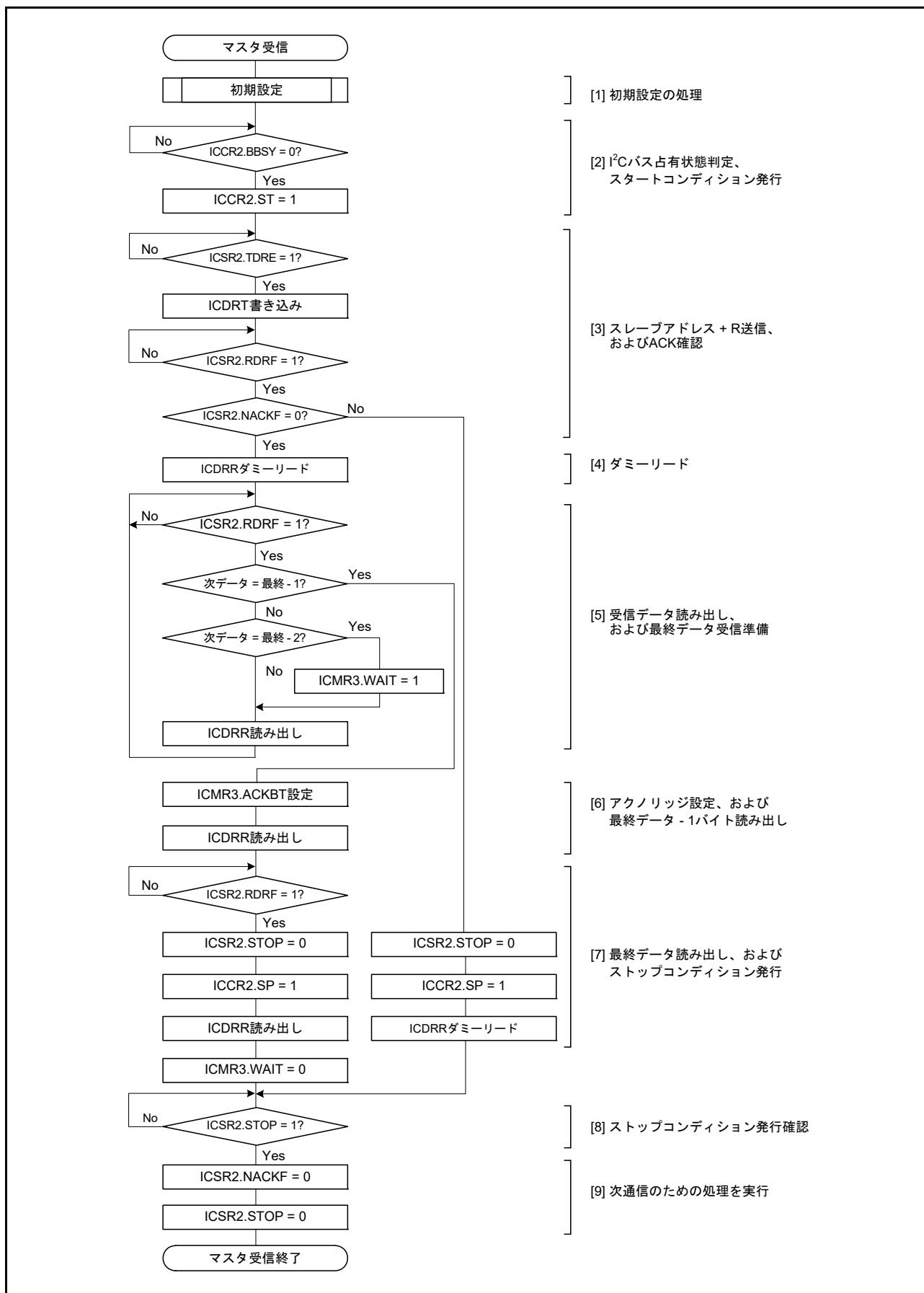
図 32.11 マスタ受信のフローチャート例 (7ビットアドレスフォーマットで3バイト以上受信の場合)
