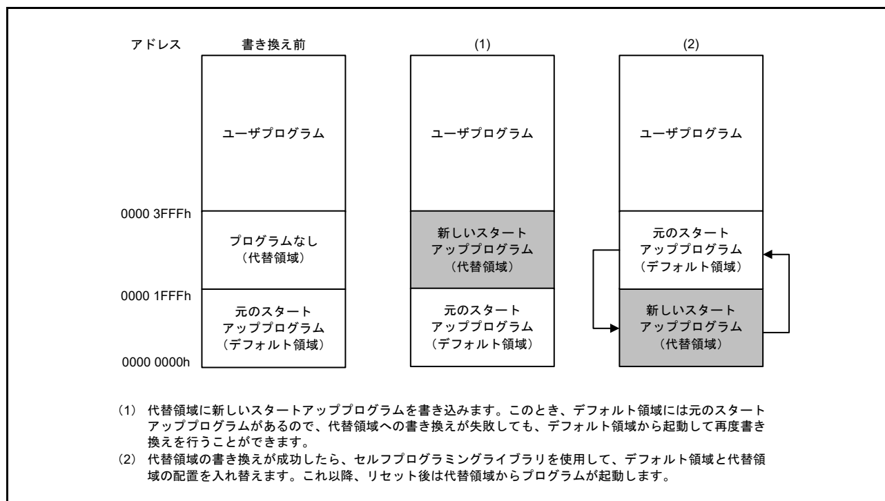
図 50.7 スタートアッププログラムプロテクションの概要
