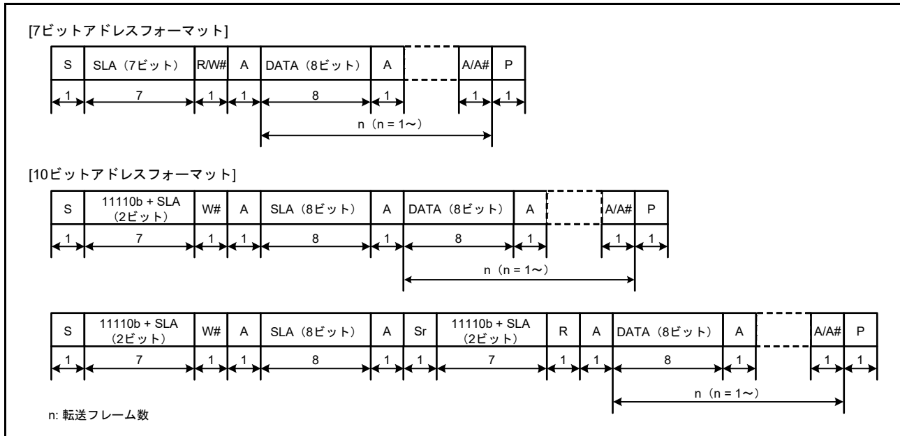
図 32.3 I 2 C バスフォーマット
