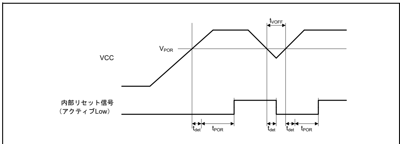
図 52.66 パワーオンリセットタイミング
