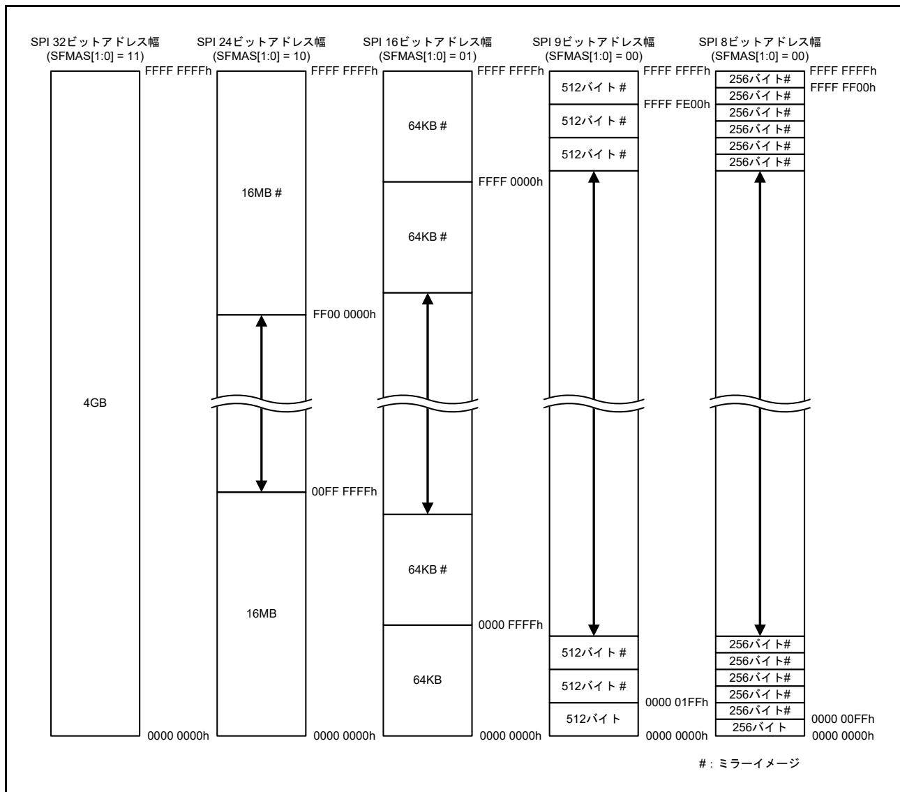
図 35.3 SPI 空間のメモリマップ
