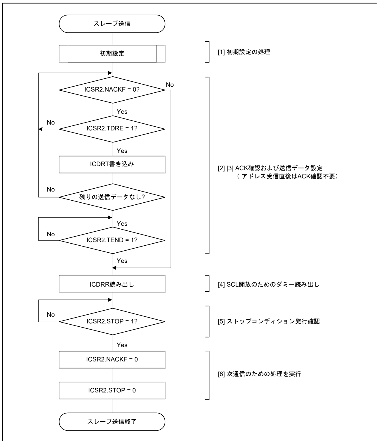
図 32.15 スレーブ送信のフロー例
