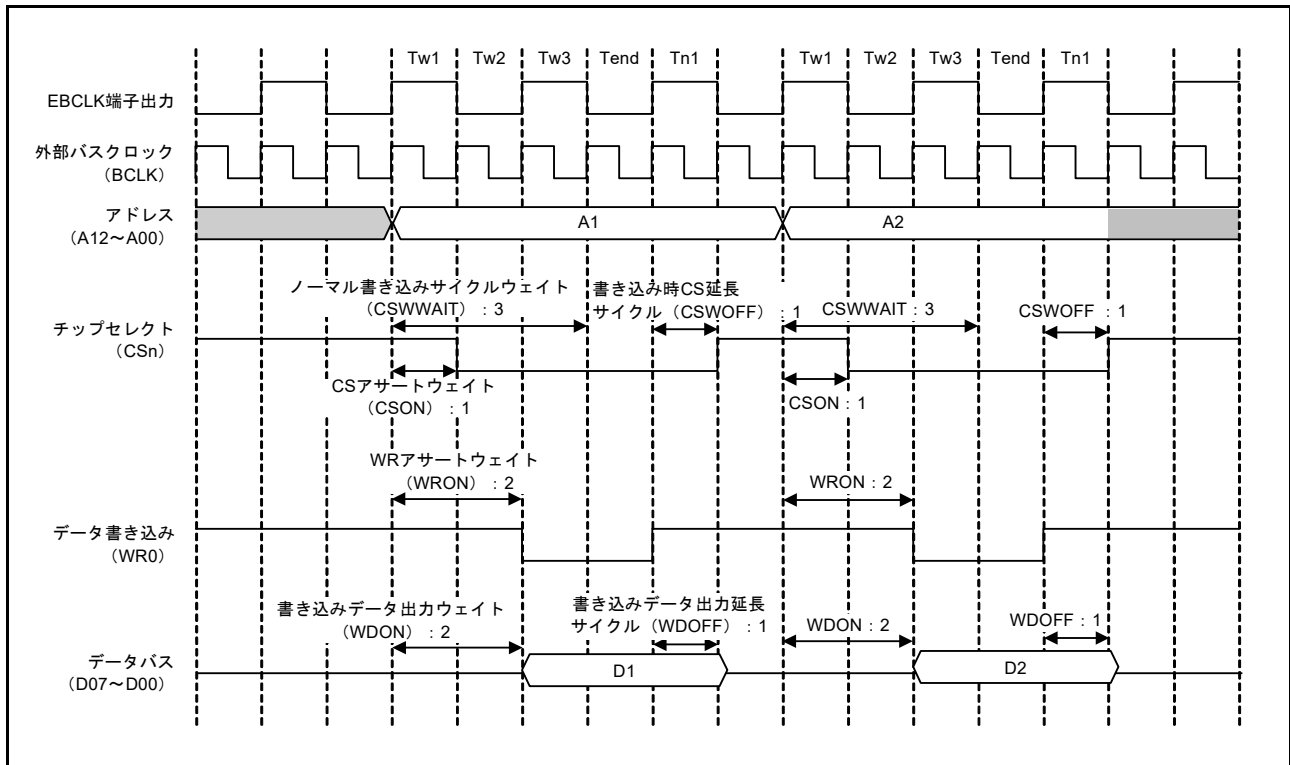
図 15.12 ノーマルライトアクセスの動作例 (EBCLK 端子出力選択ビットで BCLK の 2 分周を設定した場合) (n = 0, 1, 4 ~ 7)
