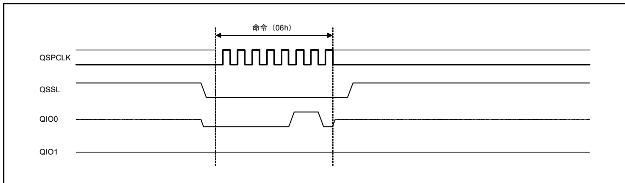
図 35.28 ライトイネーブルバスサイクル
