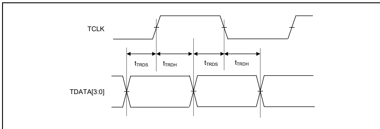
図 52.80 ETM 出力タイミング
