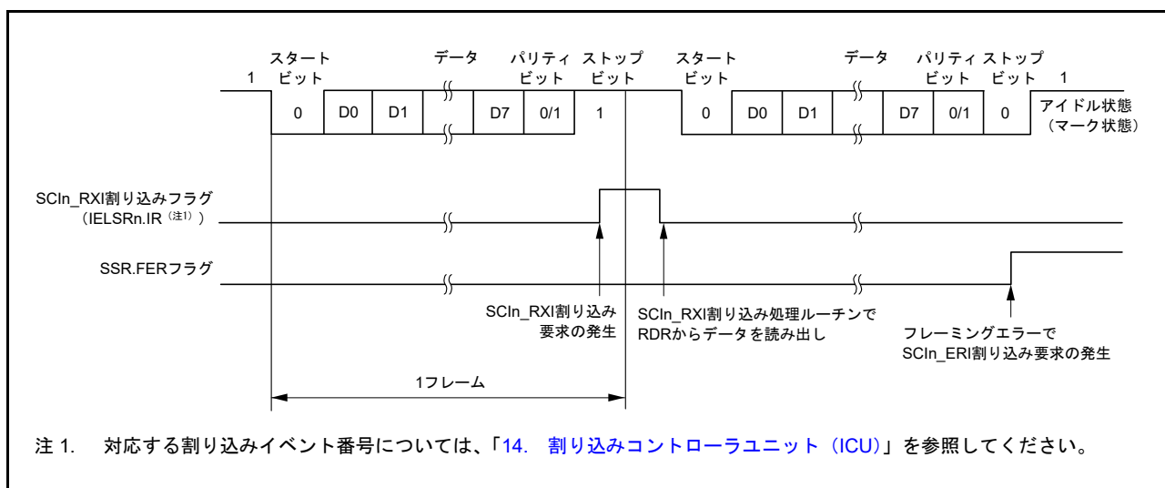
図 30.15 調歩同期式モードにおけるシリアル受信の動作例 (1) (RTS 機能を使用しない場合) (8 ビットデータ / パリティあり / 1 ストップビットの場合)
