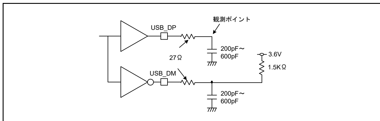
図 52.61 Low-speed モードにおける測定回路
