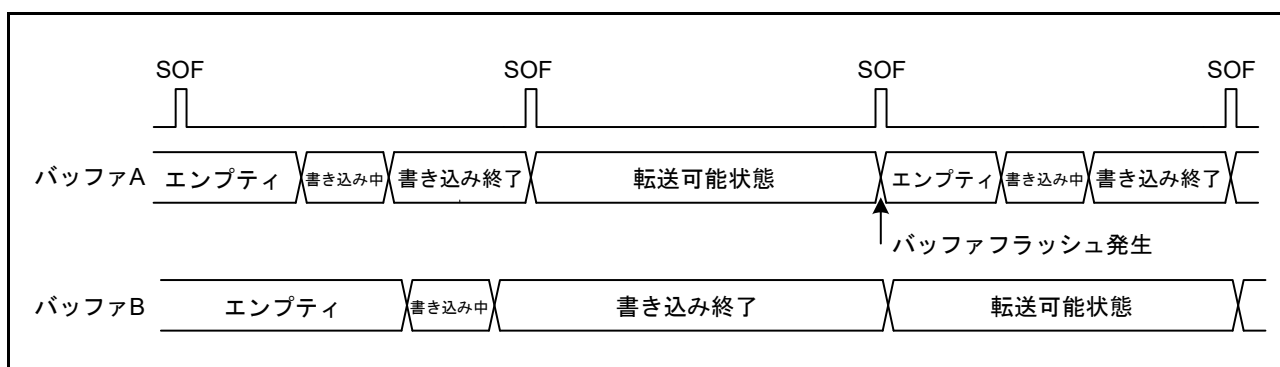
図 29.21 バッファフラッシュ動作例
