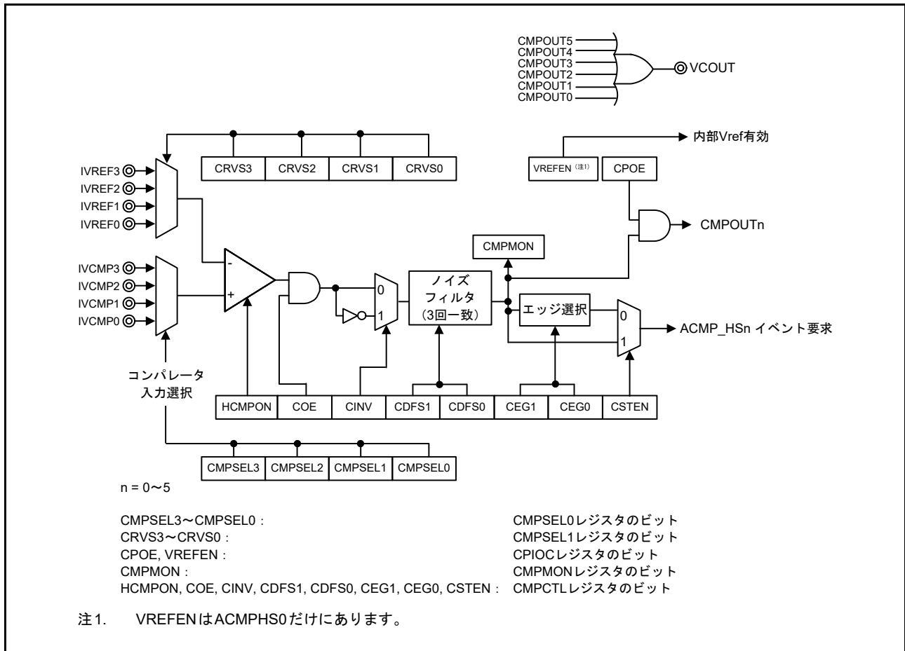
図 45.1 ACMPHS のブロック図
