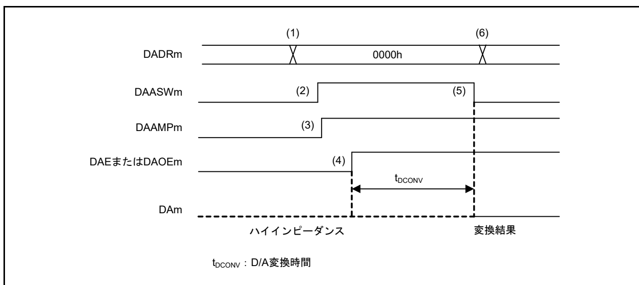
図 43.5 出力アンプを使用した DAC12 の初期化フロー例
