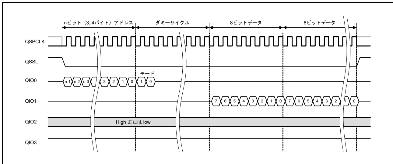
図 35.17 XIP モード時のファストリードバスサイクル
