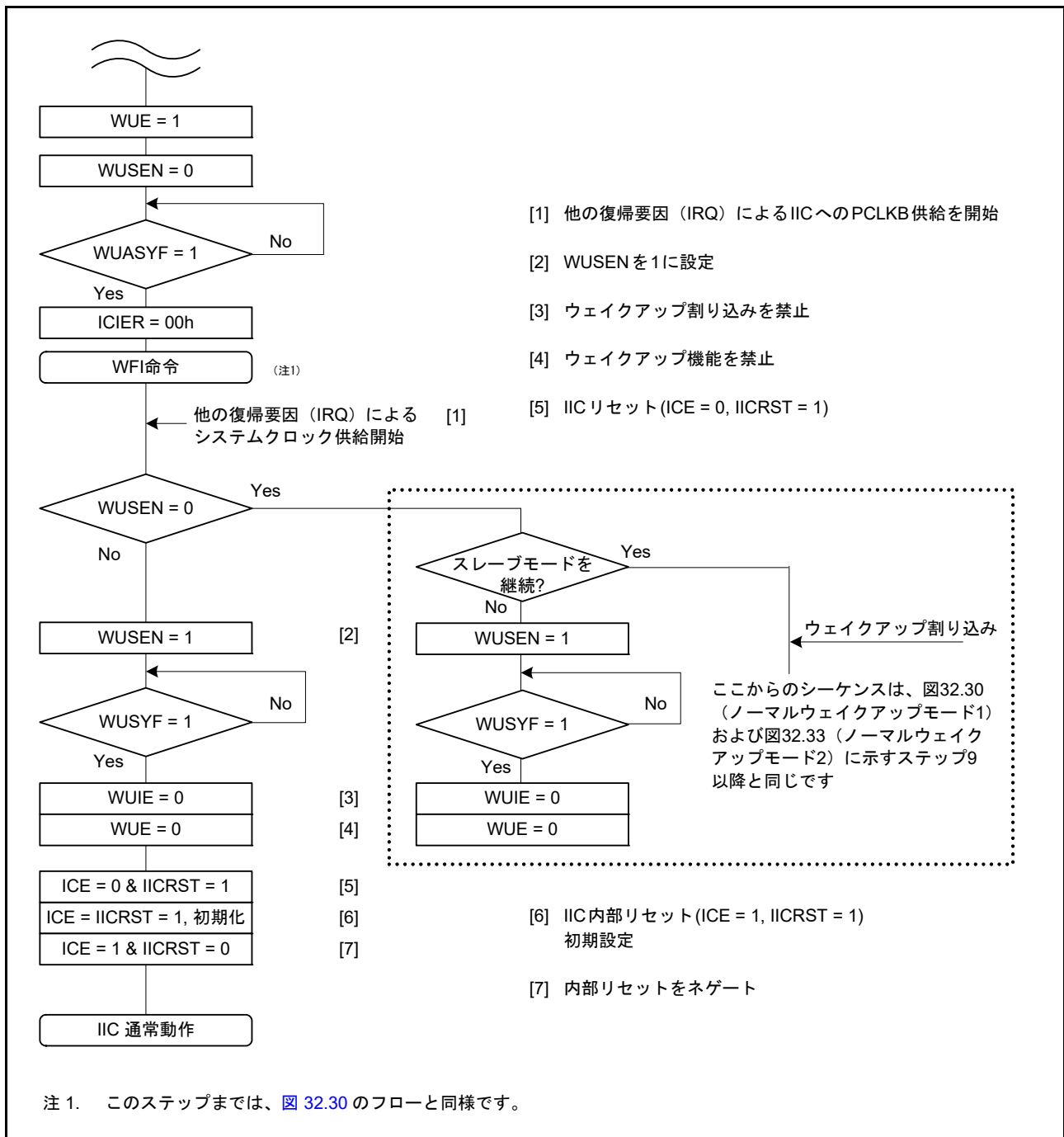
図 32.31 ノーマルウェイクアップモード 1 および 2 の動作例 (IIC ウェイクアップ割り込み以外の割り込み (たとえば IRQn) によるウェイクアップの場合)
