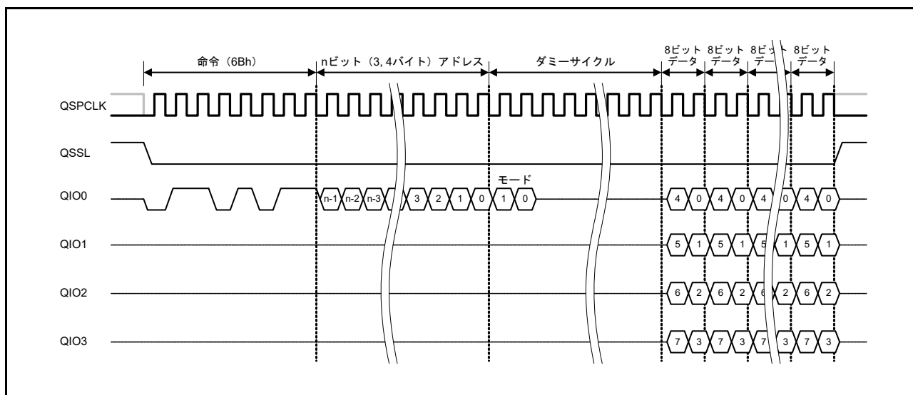
図 35.22 ファストリード Quad 出力バスサイクル
