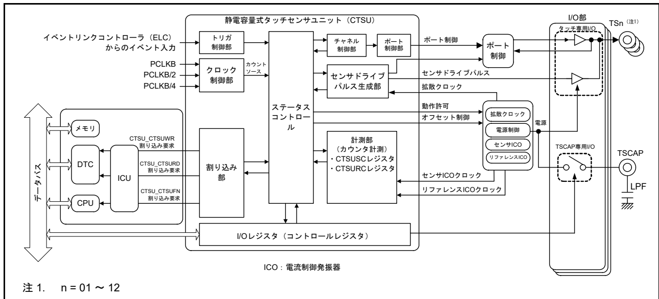
図 46.3 CTSUSのブロック図
