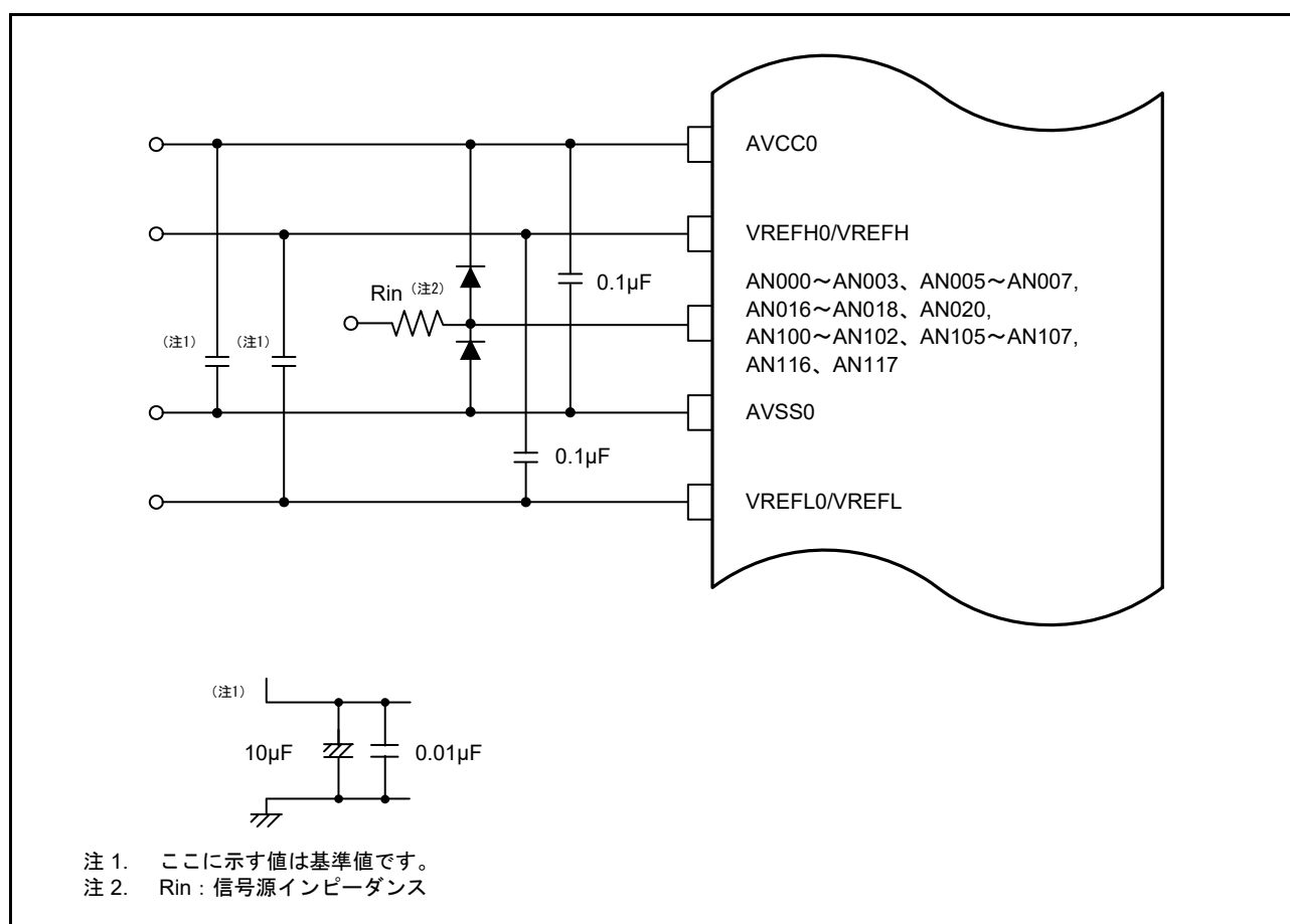
図 42.42 アナログ入力用保護回路例
