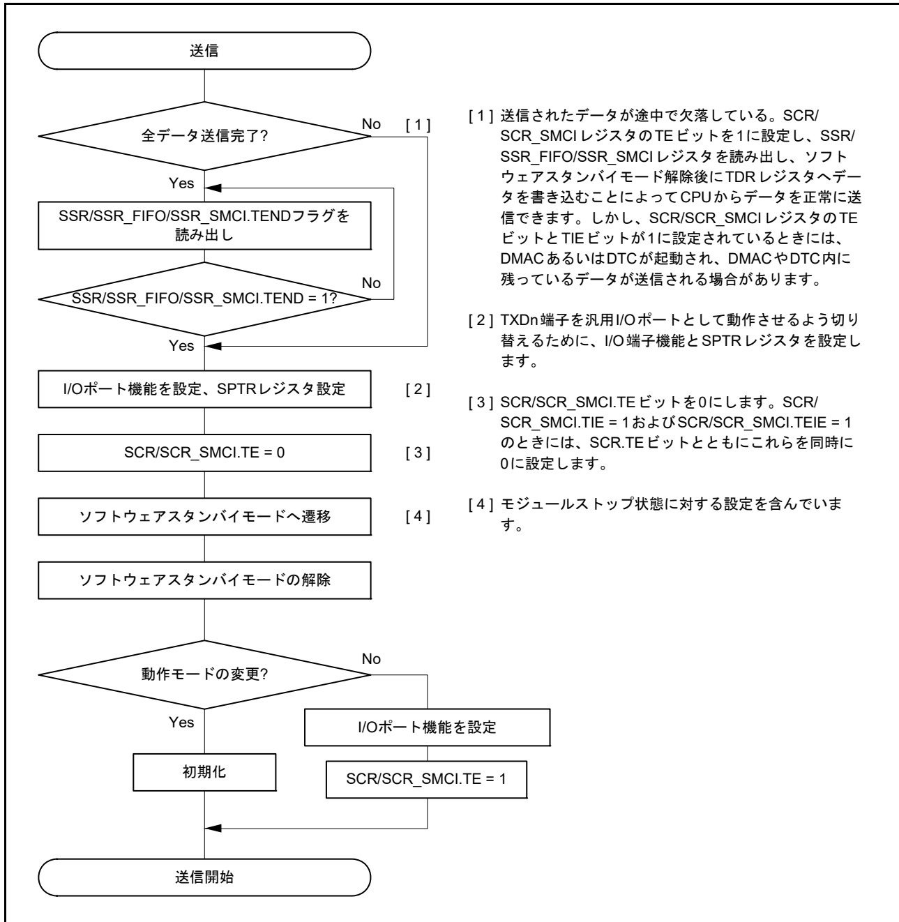
図 30.73 送信中にソフトウェアスタンバイモードへ遷移する場合のフローチャート例
