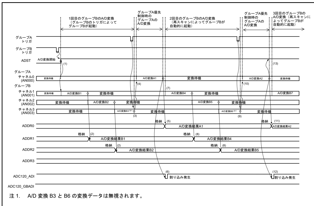
図 42.27 グループ A 優先制御の動作例 (2) (ADGSPCR.GBRSCN = 1、ADGSPCR.GBRP = 0 の場合)
