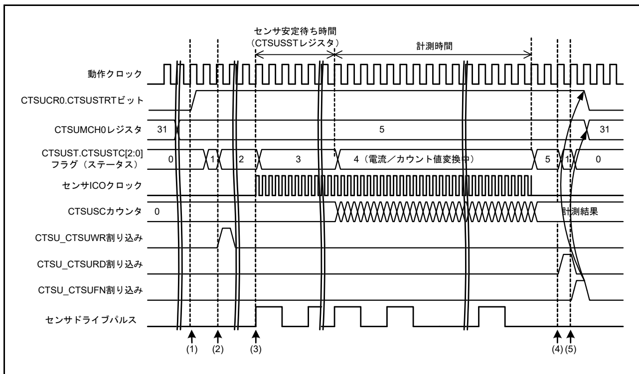
図 46.13 自己容量シングルスキャンモードのタイミング (計測開始条件がソフトウェアトリガの場合)
