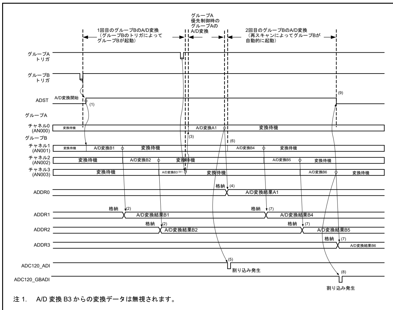
図 42.26 グループ A 優先制御の動作例 (1) (ADGSPCR.GBRSCN = 1、ADGSPCR.GBRP = 0 の場合)
