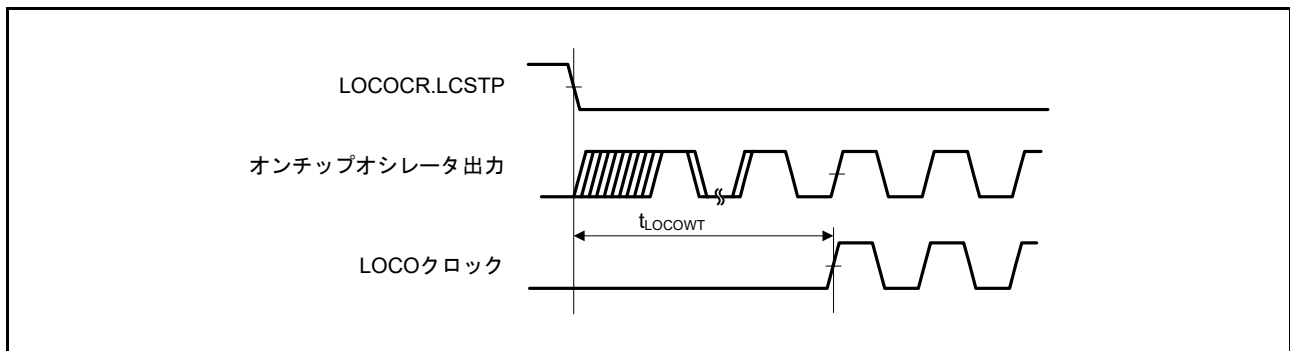
図 52.10 LOCO クロック発振開始タイミング
