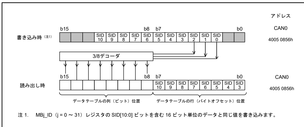
図 33.5 AFSR レジスタに対する書き込みと読み出し
