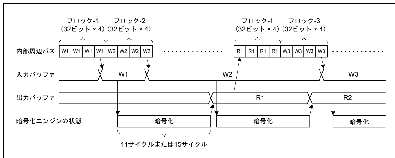
図 41.3 暗号化と復号タイミング (AES)
