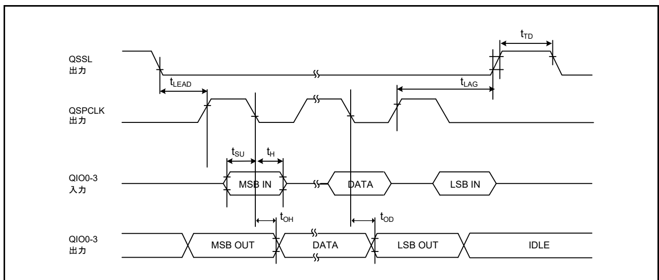
図 52.52 送受信タイミング
