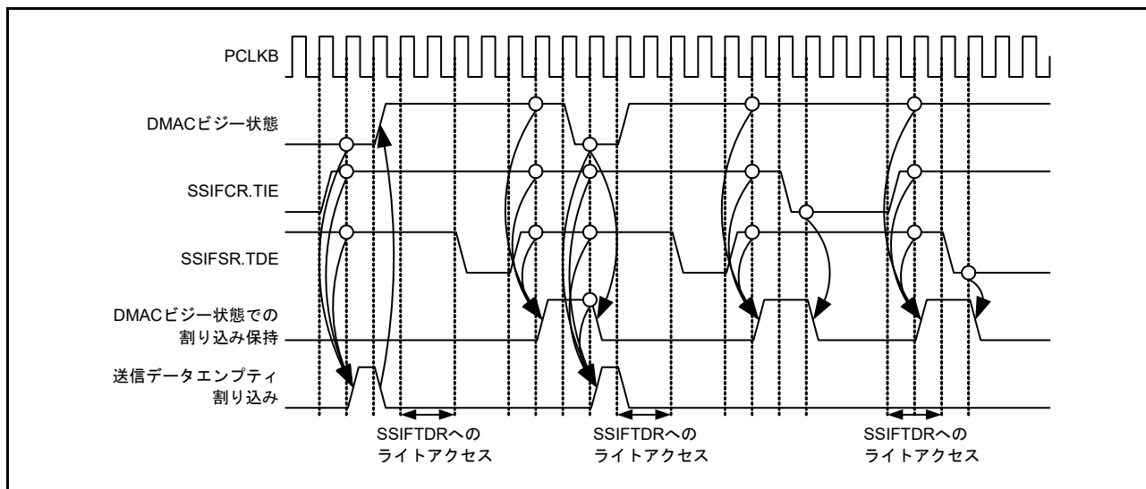
図 37.22 送信データエンプティ割り込みのタイミング
