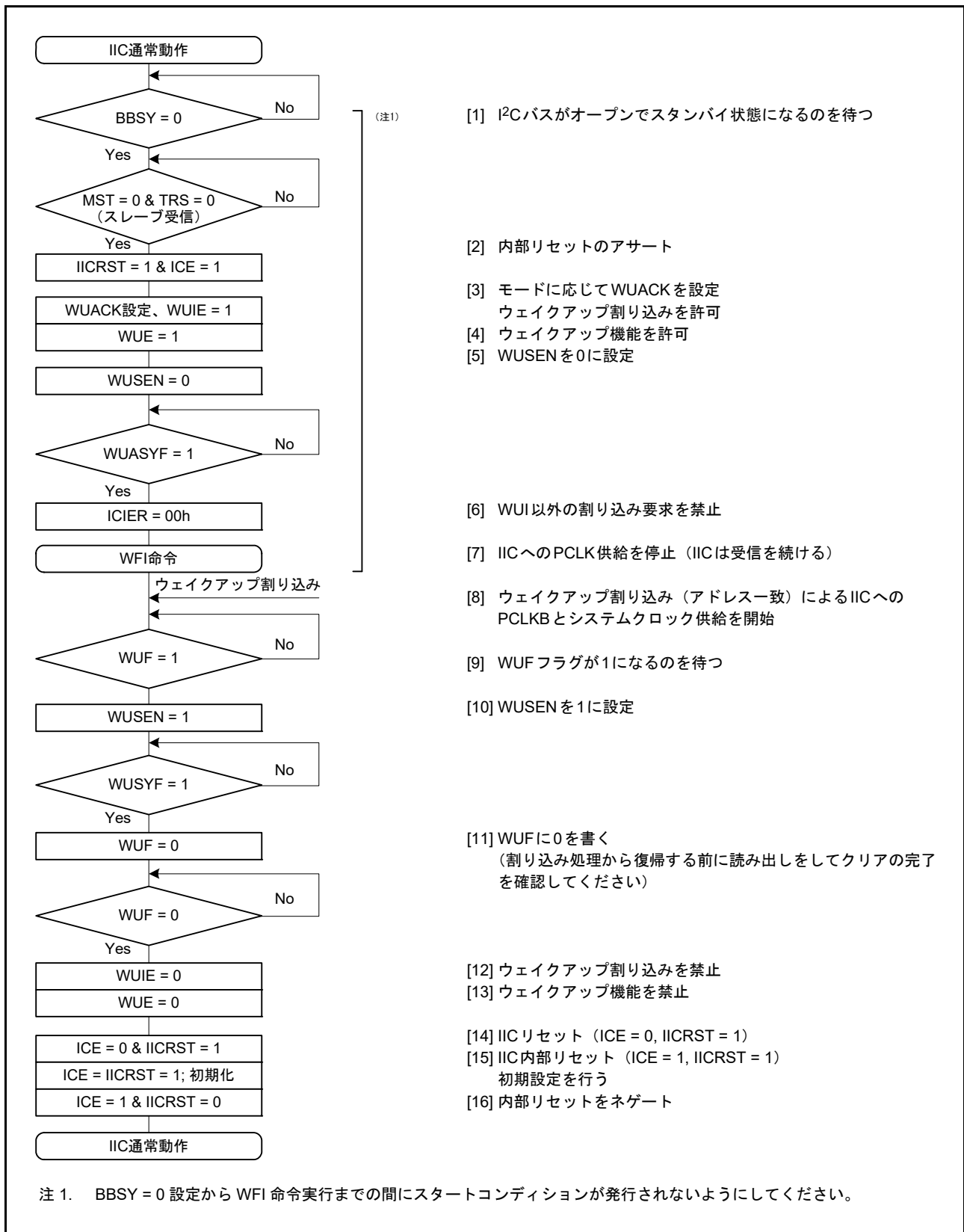
図 32.35 コマンドリカバリモードとEEP 応答モードの動作例 (スレーブアドレス一致時のウェイクアップ割り込みによるウェイクアップの場合)
