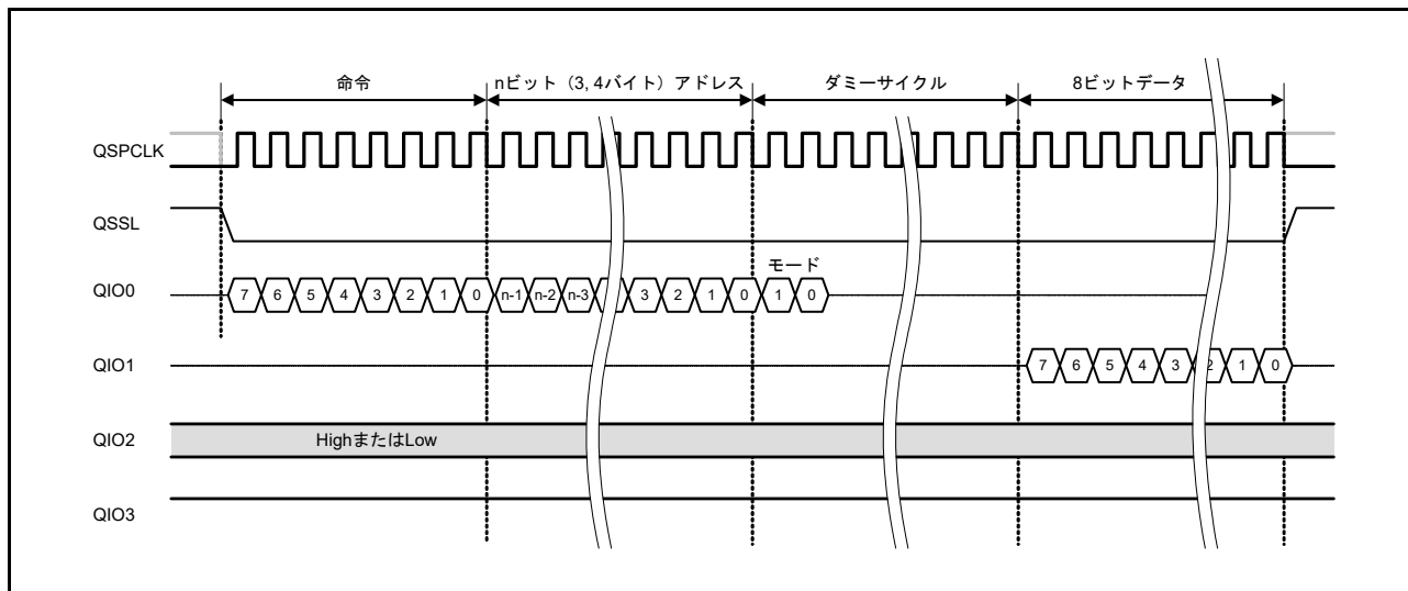
図 35.4 拡張 SPI プロトコル例 1 (ファストリード)
