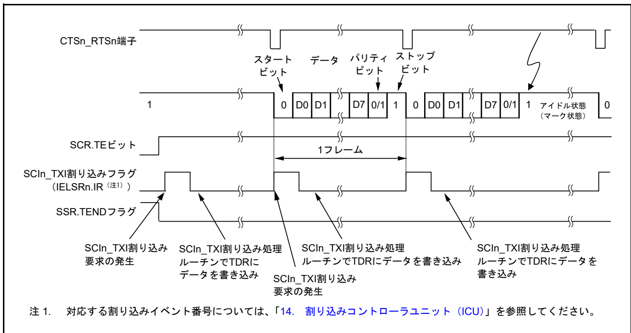
図 30.10 調歩同期式モードにおけるシリアル送信の動作例 (2) (8 ビットデータ/パリティあり/1ストップビット/CTS 機能使用/送信開始時)
