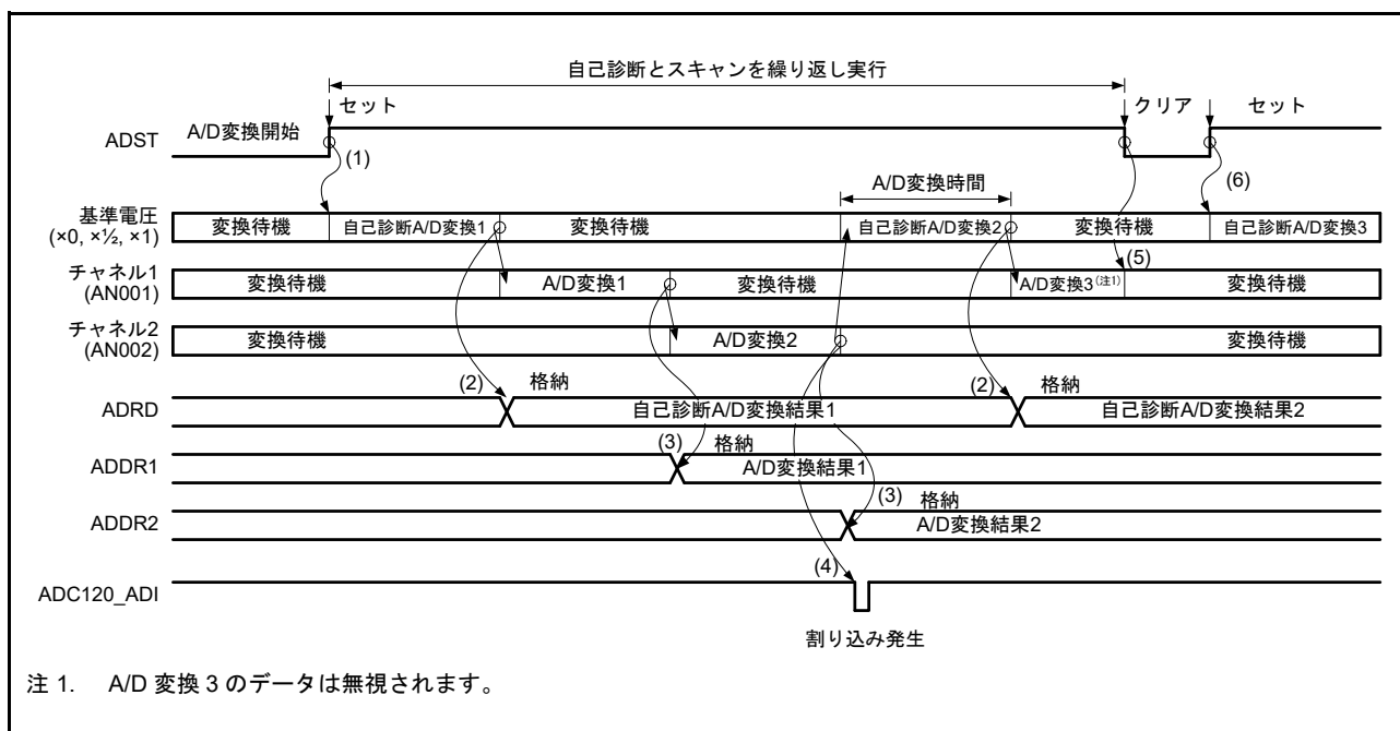
図 42.19 連続スキャンモードの基本動作例 (AN001 および AN002 選択 + 自己診断)
