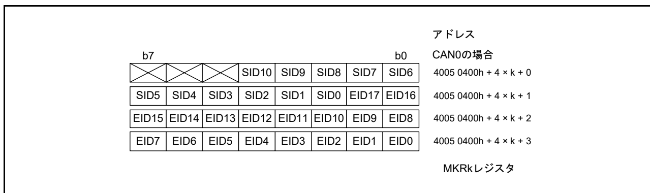
図 33.14 MKR k レジスタの構成 (k = 0 ~ 7)
