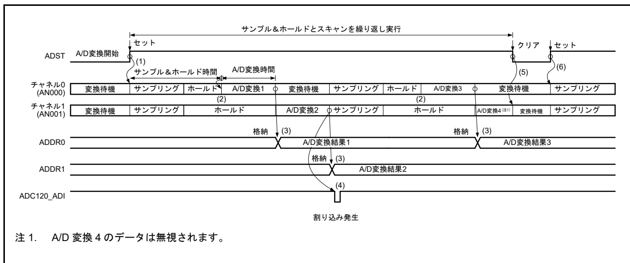
図 42.17 連続スキャンモードの動作例 (チャンネル専用サンプル&ホールド回路使用、AN000 および AN001 選択)
