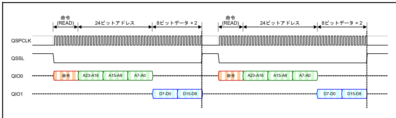
図 35.29 個々の変換に基づく連続データリード動作
