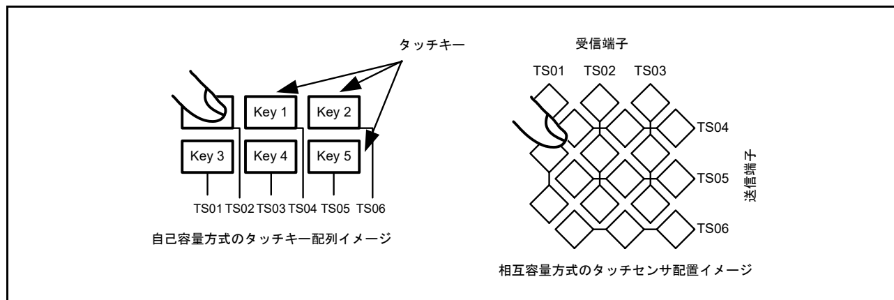
図 46.8 自己容量方式と相互容量方式の概要
