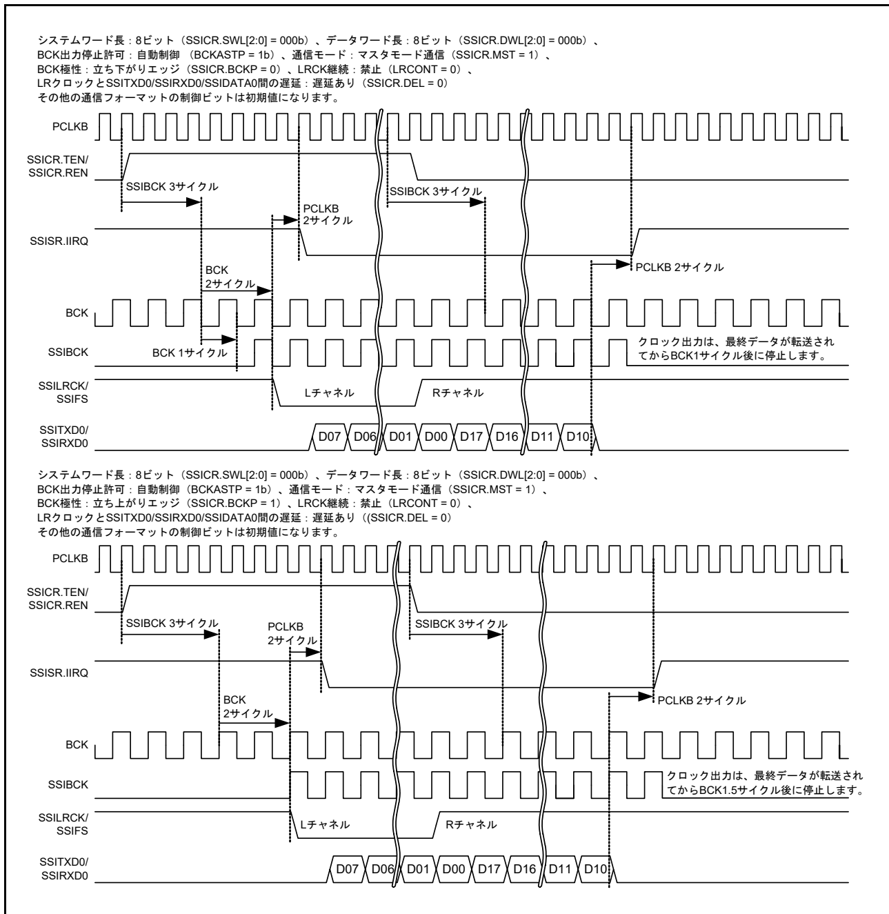
図 37.34 BCKASTP ビットの動作例 (BCKASTP = 1 での通信動作の場合)
