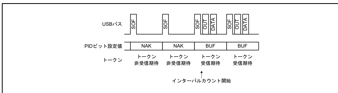
図 29.18 IITV[2:0] = 0 の場合のフレームとトークン受信期待の関係
