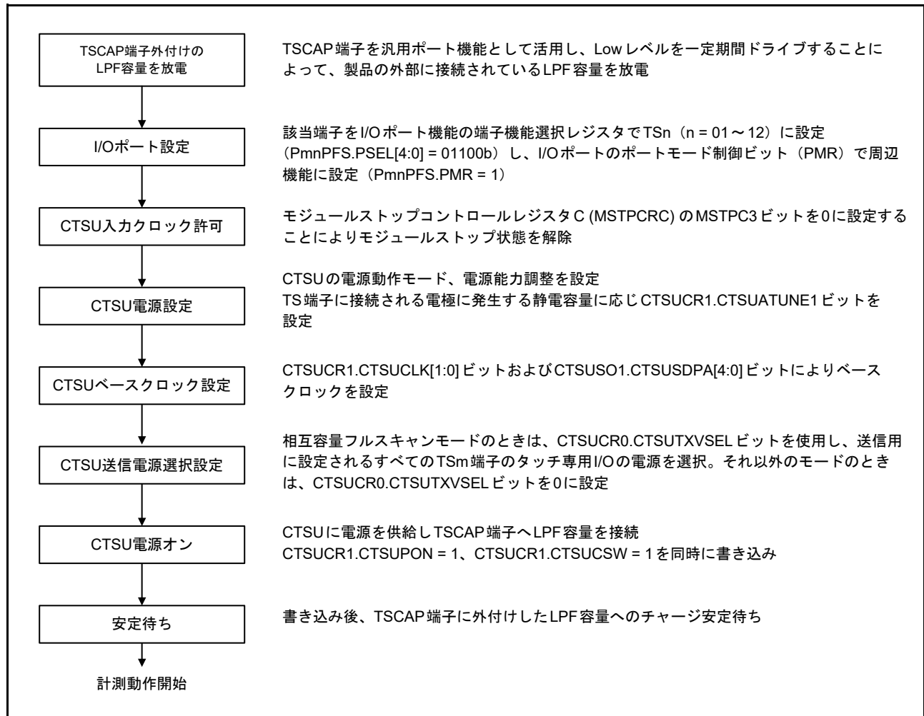
図 46.9 CTSU 初期設定フロー
