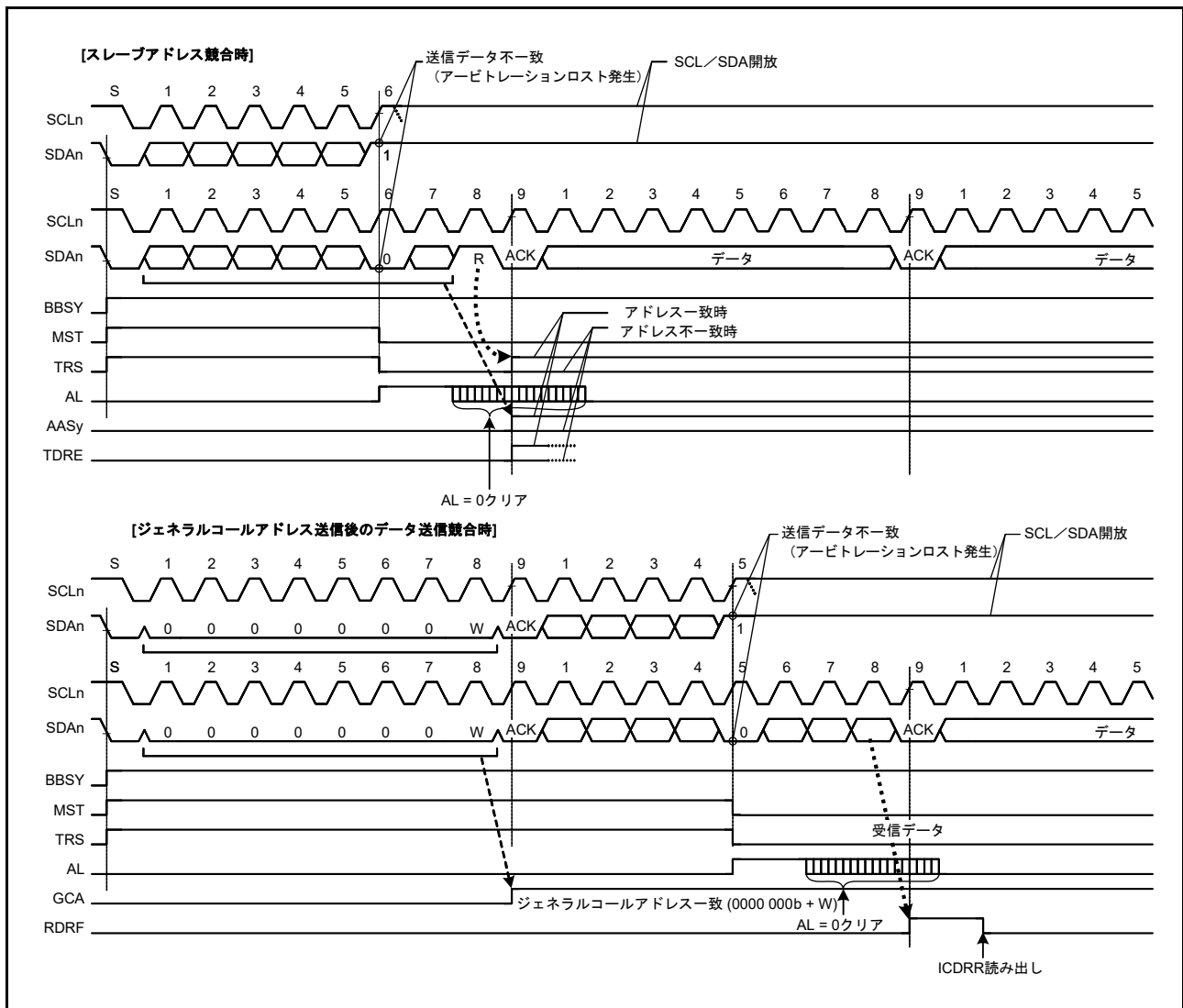
図 32.41 マスタアビトラージョンロスト検出の動作例 (MALE = 1 の場合)
