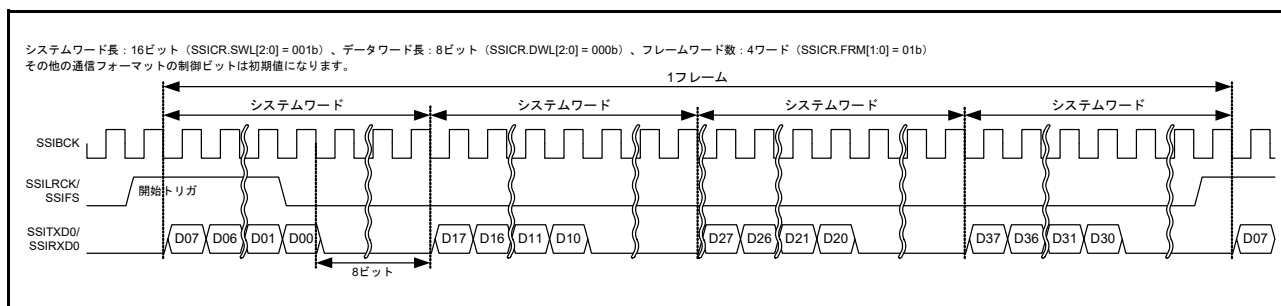
図 37.41 TDM フォーマット (パディングあり、システムワード長>データワード長)
