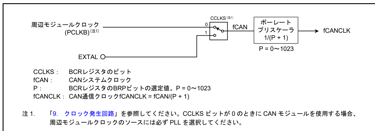
図 33.11 CAN クロック発生回路のブロック図
