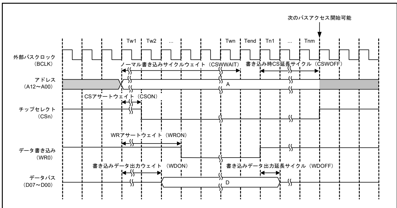
図 15.6 ノーマルライトアクセスのバスタイミング (1 ライトストローブモード) (n = 0, 1, 4 ~ 7)
