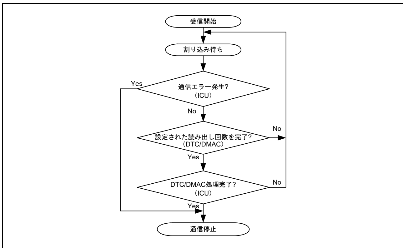
図 37.54 受信手順
