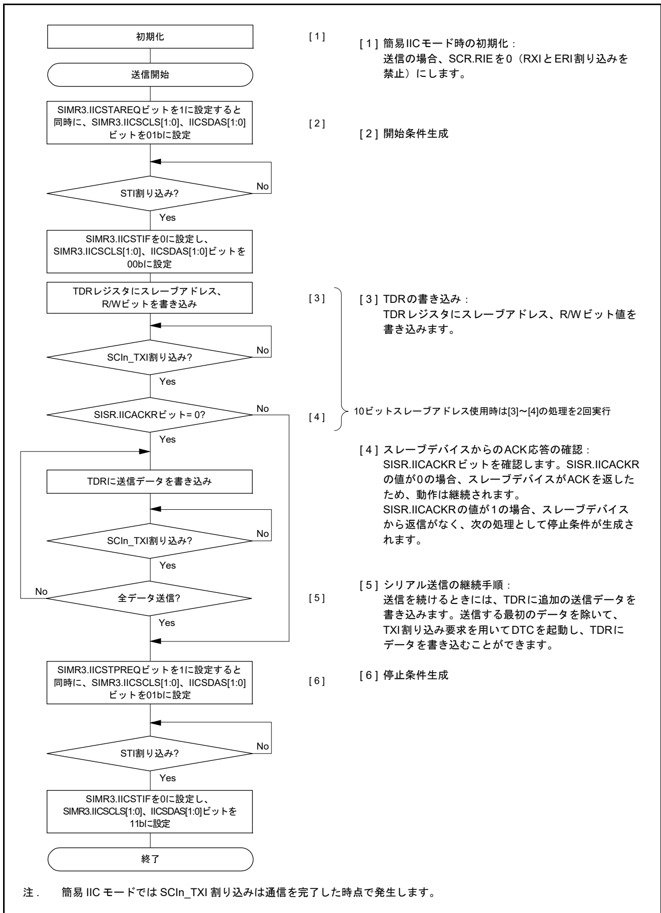
図 30.66 簡易 IIC モードにおけるマスタ送信のフローチャート例（送信割り込み、受信割り込み使用時）
