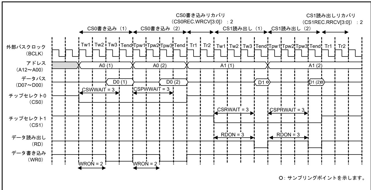
図 15.31 バスアクセスが分割された場合のリカバリサイクルの挿入例 (セパレートバスインタフェースによるページアクセスの場合)
