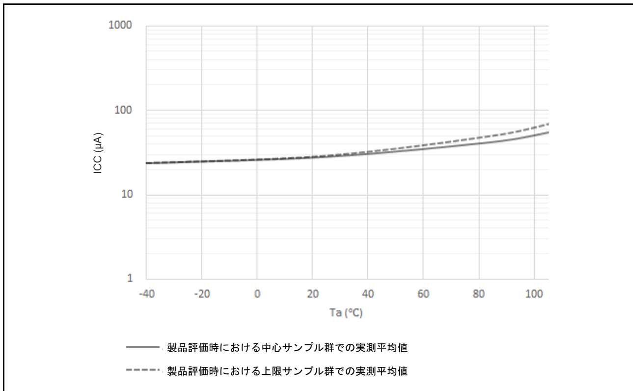
図 52.3 ディープソフトウェアスタンバイモード時の温度依存性：スタンバイ SRAM および USB レジューム検出部への電源供給あり（参考データ）
