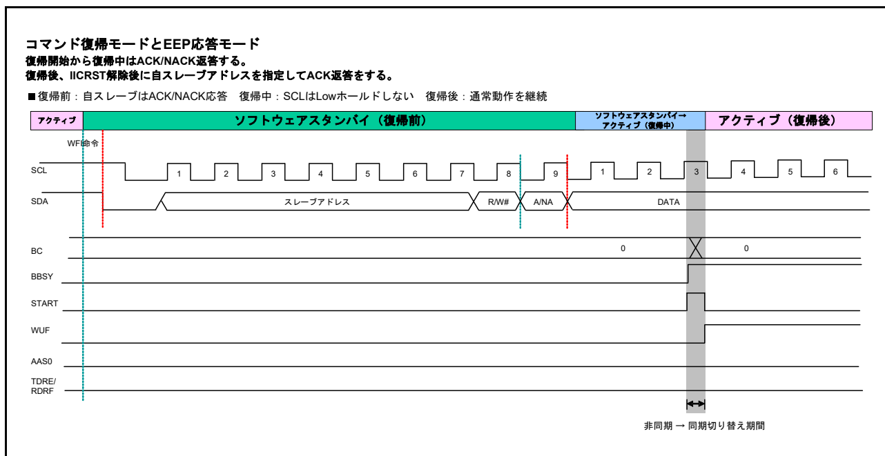
図 32.37 コマンドリカバリモードとEEP 応答モードのタイミング
