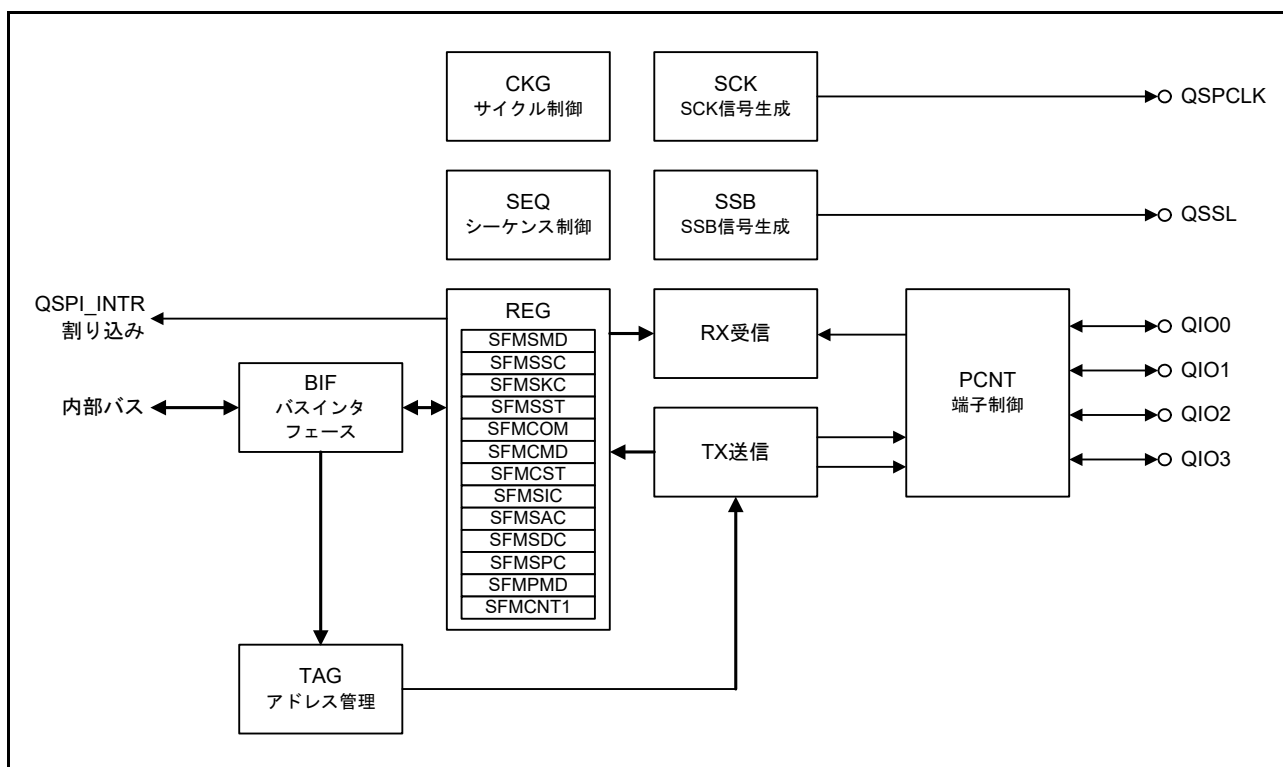
図 35.1 QSPIのブロック図
