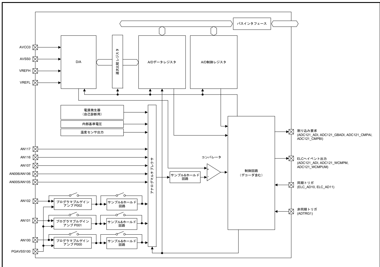
図 42.2 ADC12 (ユニット1) のブロック図
