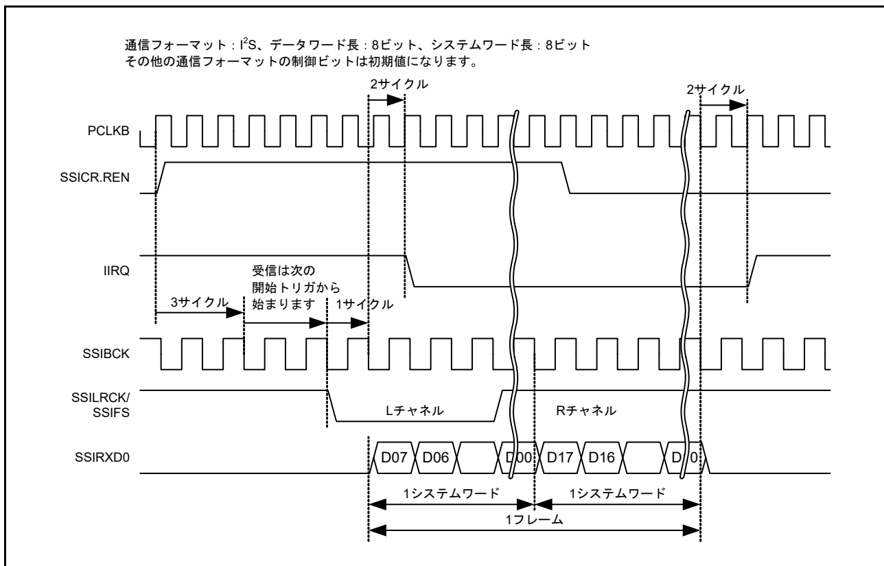
図 37.14 IIRQ 設定タイミング (受信)
