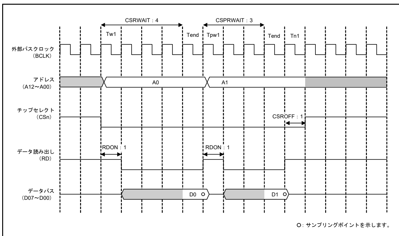
図 15.17 ページリードアクセスの動作例 (8 ビットバス空間に対する 16 ビットアクセスの場合) ( n = 0, 1, 4 \sim 7 )
