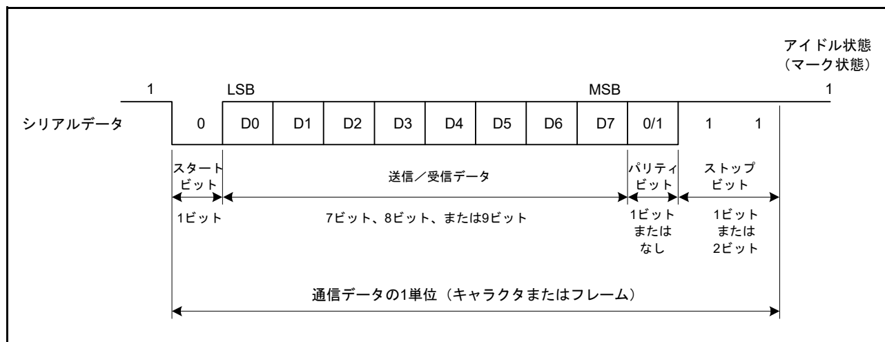
図 30.2 調歩同期式シリアル通信のデータフォーマット (8 ビットデータ/パリティあり/2 ストップビットの場合)
