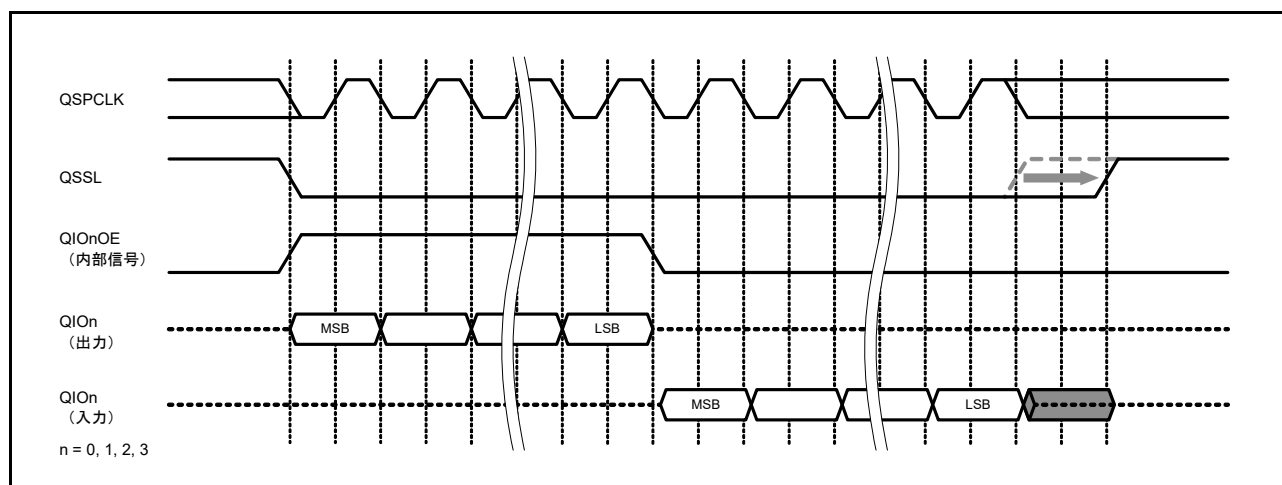
図 35.11 SFMSHD ビットを使用した QSSL 信号のホールド時間調整
