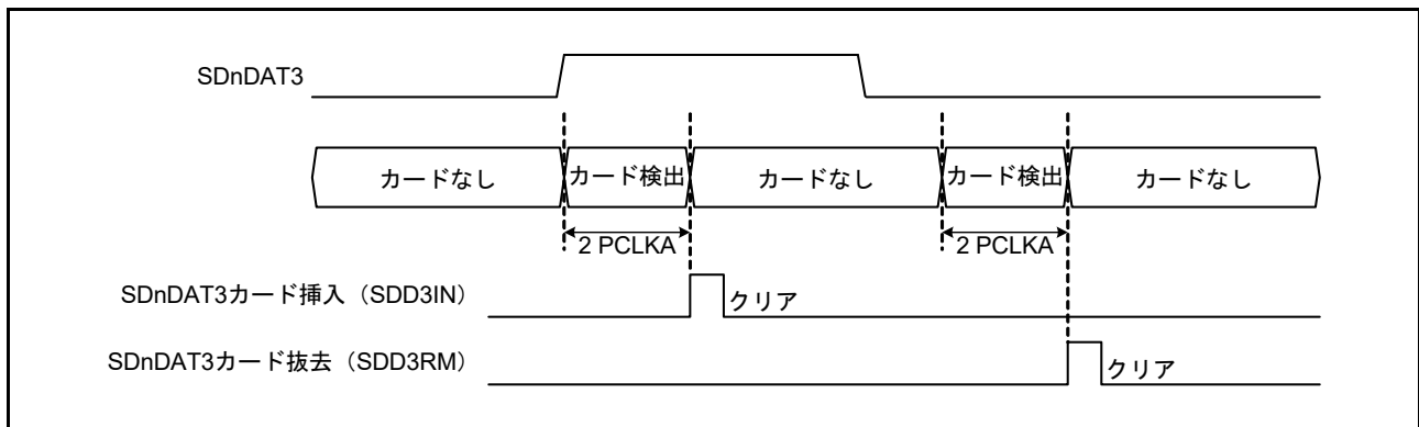
図 39.7 SDnDAT3 による SD カード検出
