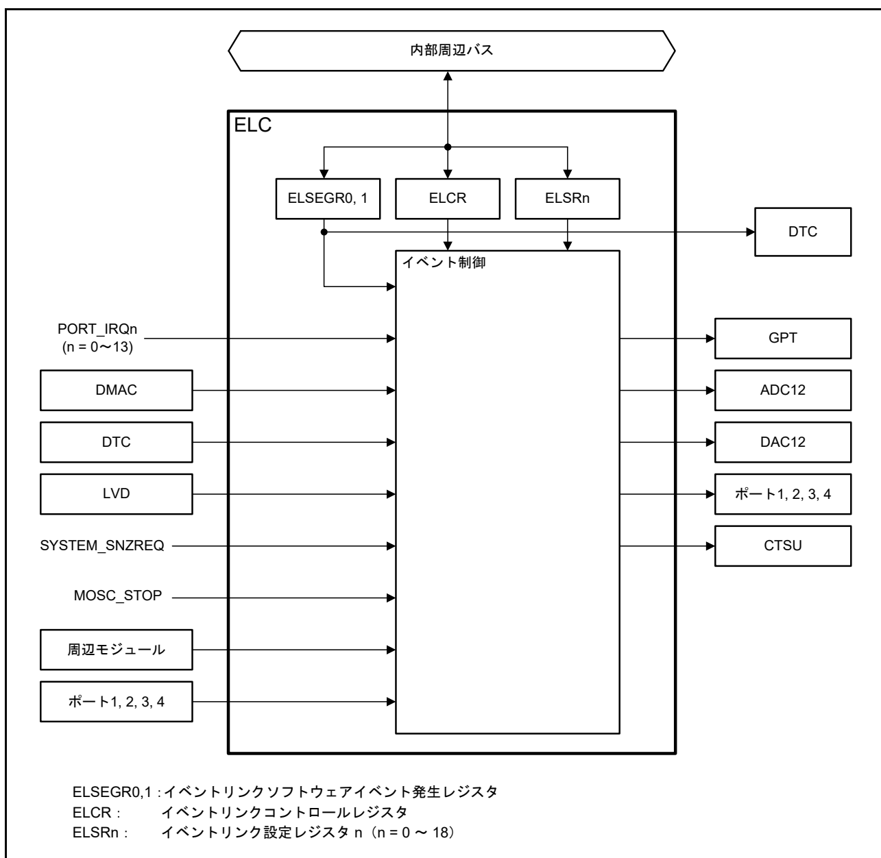
図 19.1 ELCのブロック図
