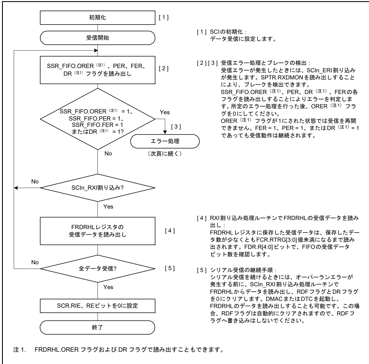
図 30.20 調歩同期式モードにおけるシリアル受信のフローチャート例 (FIFO 選択時) (1)
