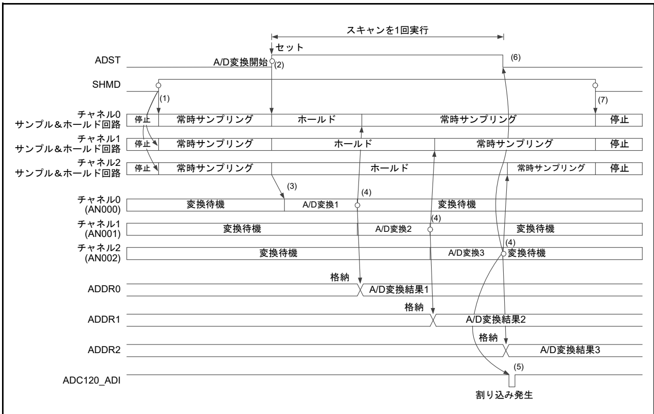
図 42.9 シングルスキャンモードの動作例 (チャンネル専用サンプル&ホールド回路使用、AN000 ~ AN002 選択、常時サンプリング有効)
