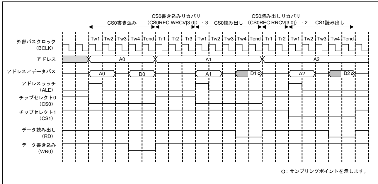
図 15.33 アドレス/データマルチプレクス I/O インタフェース時のリカバリサイクルの挿入例
