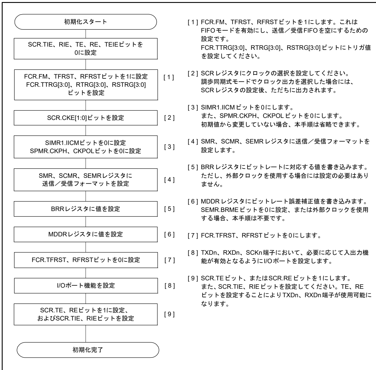
図 30.8 調歩同期式モードにおける SCI の初期化フローチャート例 (FIFO 選択時)
