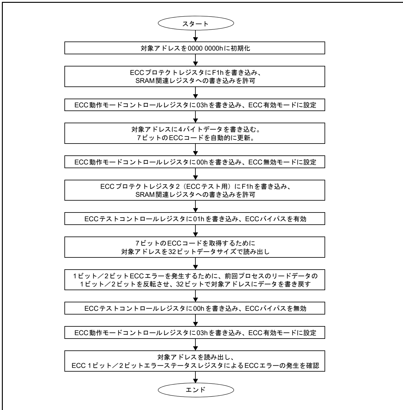
図 48.1 ECC デコーダのテスト方法
