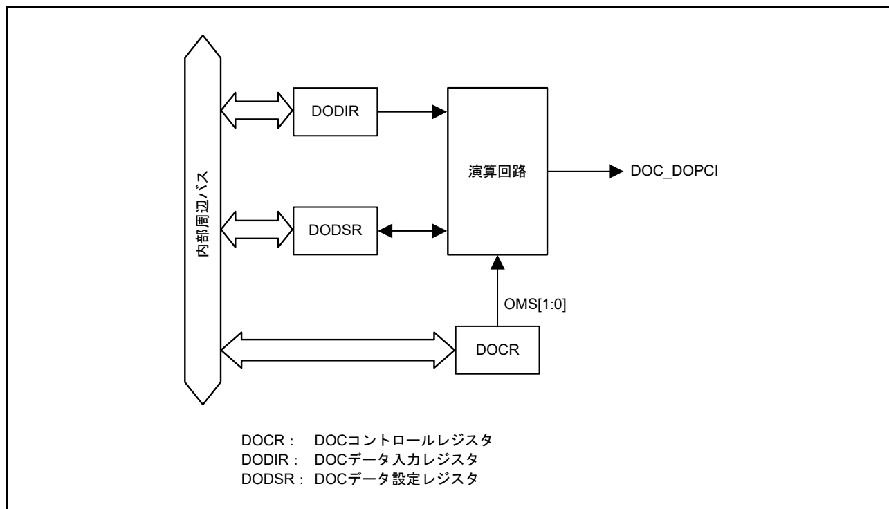
図 47.1 DOC ブロック図
