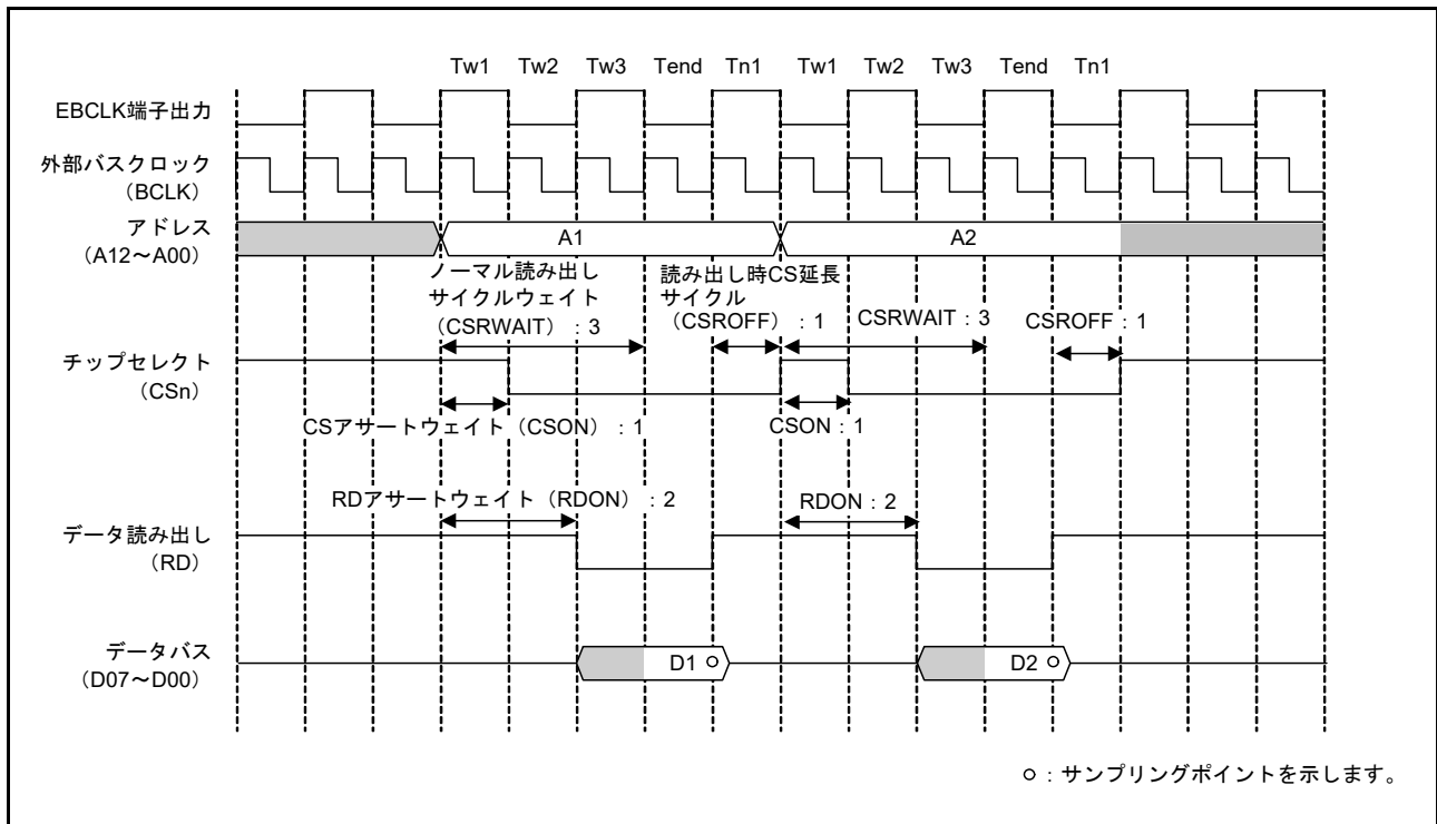
図 15.13 ノーマルリードアクセスの動作例 (EBCLK 端子出力選択ビットで BCLK の 2 分周を設定した場合、および 1 転送要求に対して 2 回バスアクセスが発生する場合) (n = 0, 1, 4 ~ 7)
