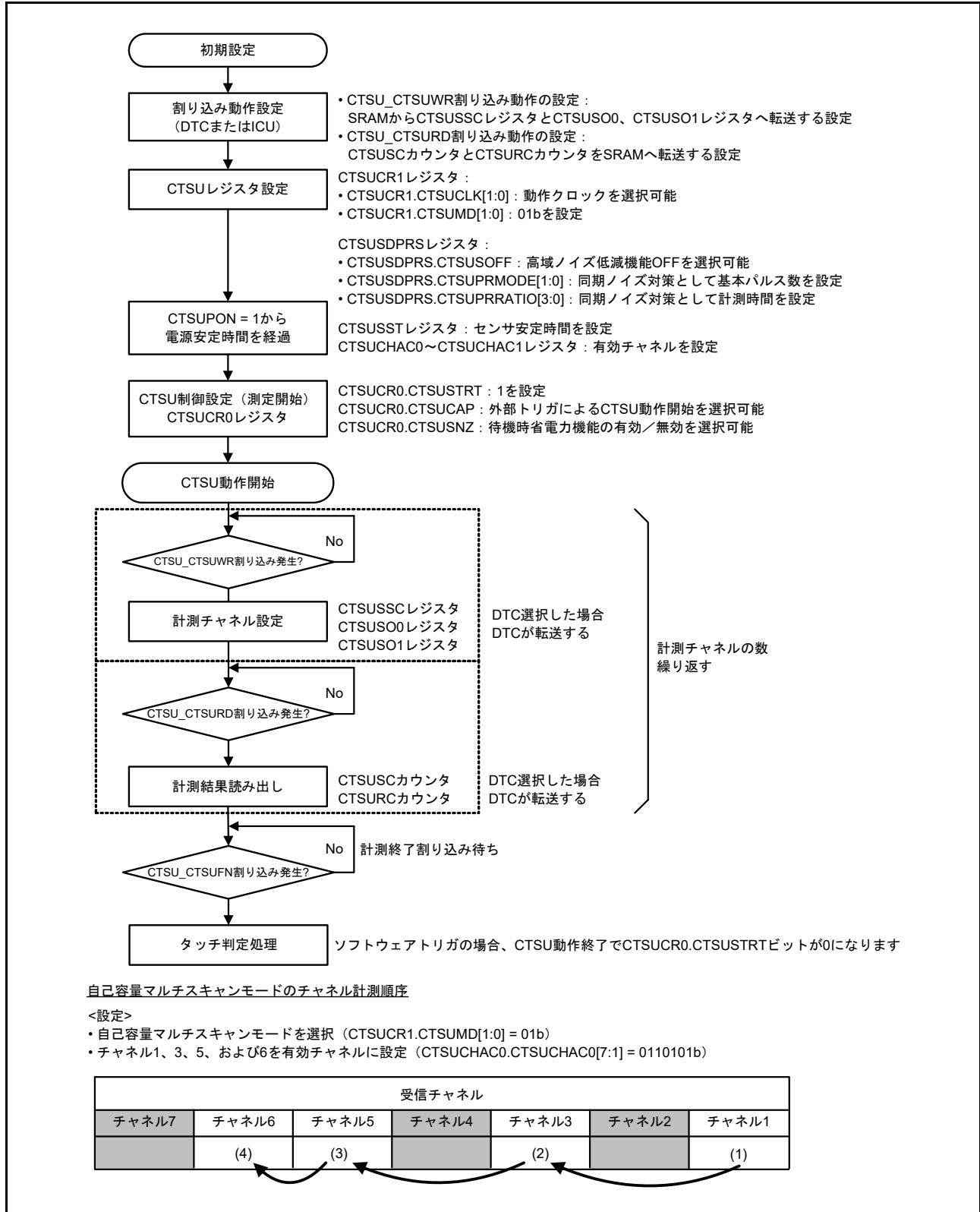
図 46.14 自己容量マルチスキャンモードのソフトウェアフローと動作例
