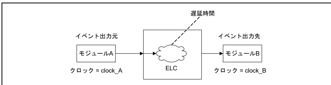
図 19.2 ELC 遅延時間
