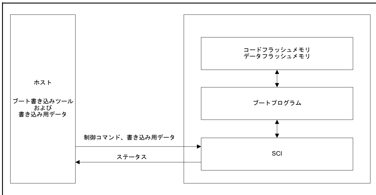
図 50.12 SCI ブートモード時のシステム構成
