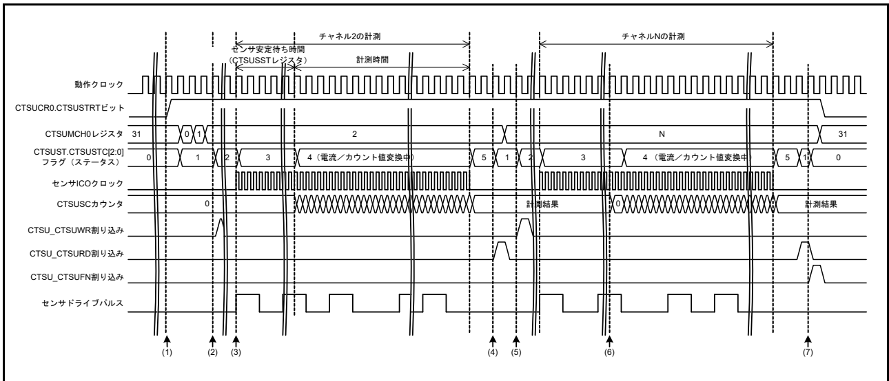
図 46.15 自己容量マルチスキャンモードのタイミング (計測開始条件がソフトウェアトリガの場合)
