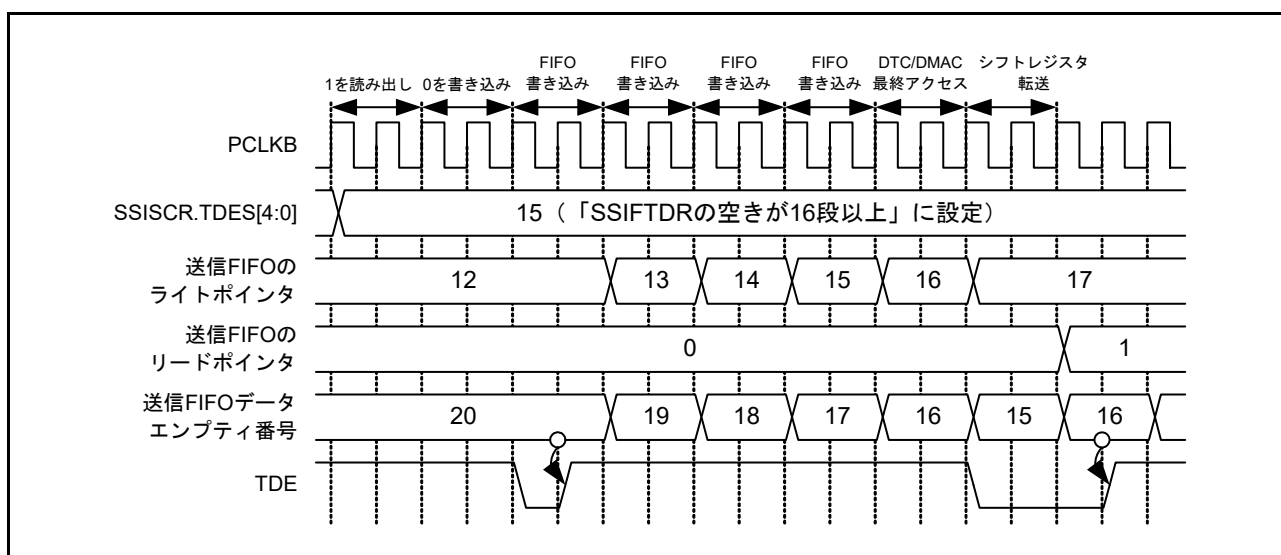
図 37.28 TDE の設定およびクリアのタイミング図
