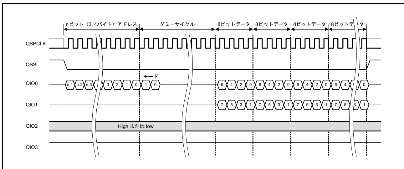
図 35.19 XIP モード時のファストリード Dual 出力バスサイクル
