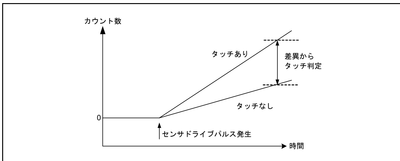
図 46.7 接触／非接触による計測値の変化
