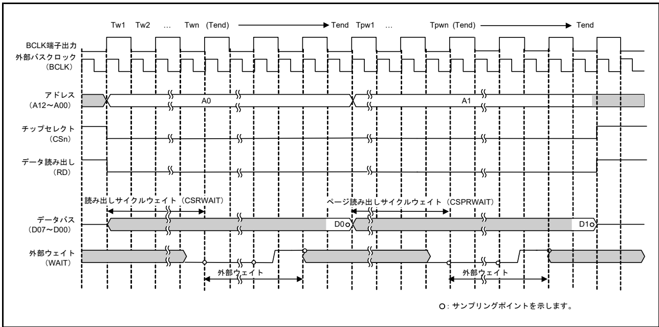
図 15.25 外部ウェイトタイミング例 (8 ビットバス空間に対するページリードアクセス、BCLK 端子出力選択ビットで BCLK の 2 分周を選択した場合) (n = 0, 1, 4 ~ 7)
