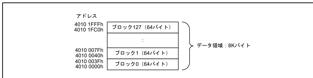
図 50.3 データフラッシュメモリマッピング
