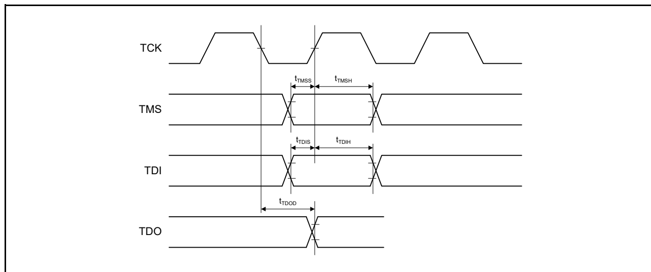
図 52.73 バウンダリスキャン入出力タイミング
