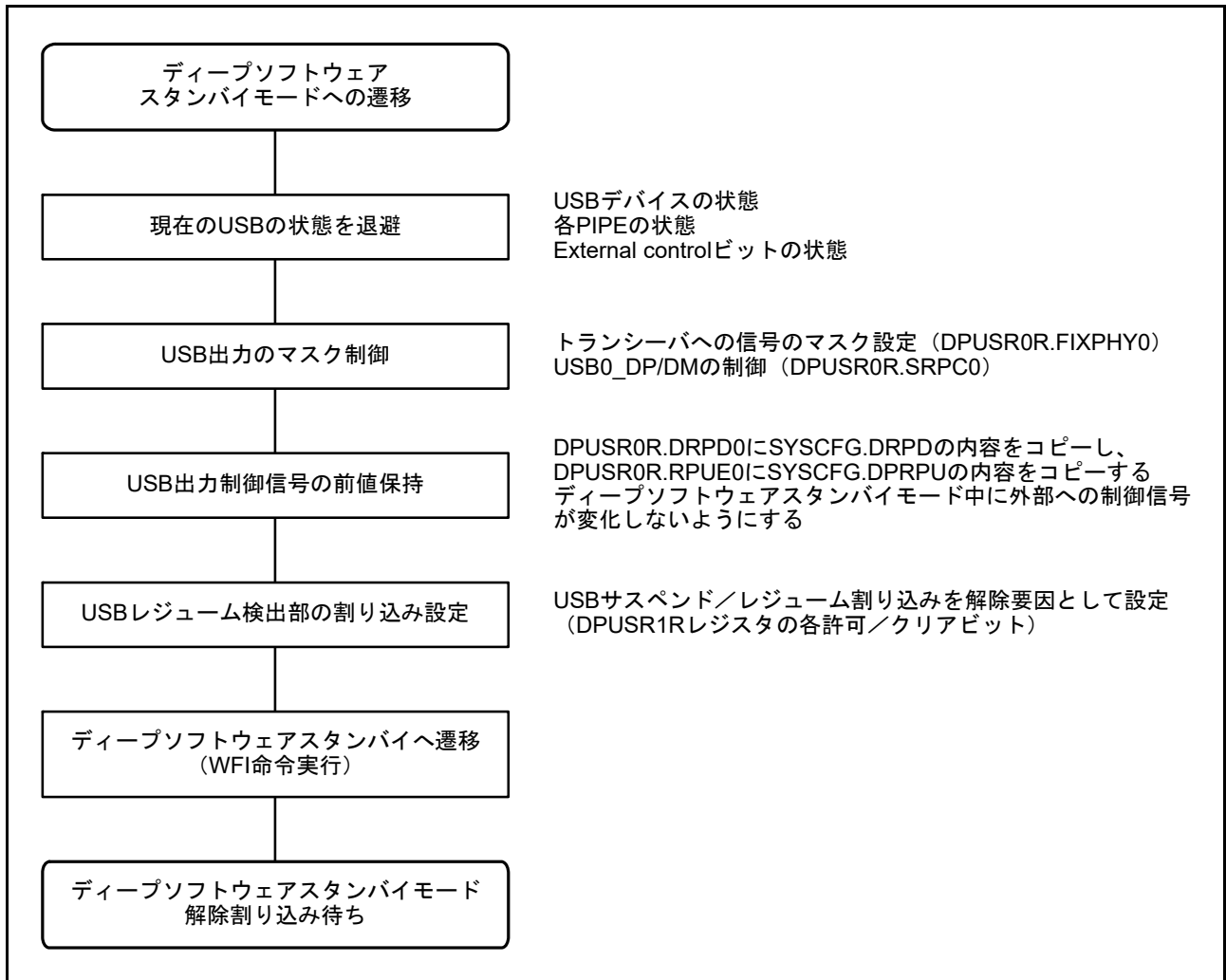
図 29.7 ホストコントローラ機能またはデバイスコントローラ機能選択時におけるディープソフトウェアスタンバイモード遷移時の USBFS 設定フロー
