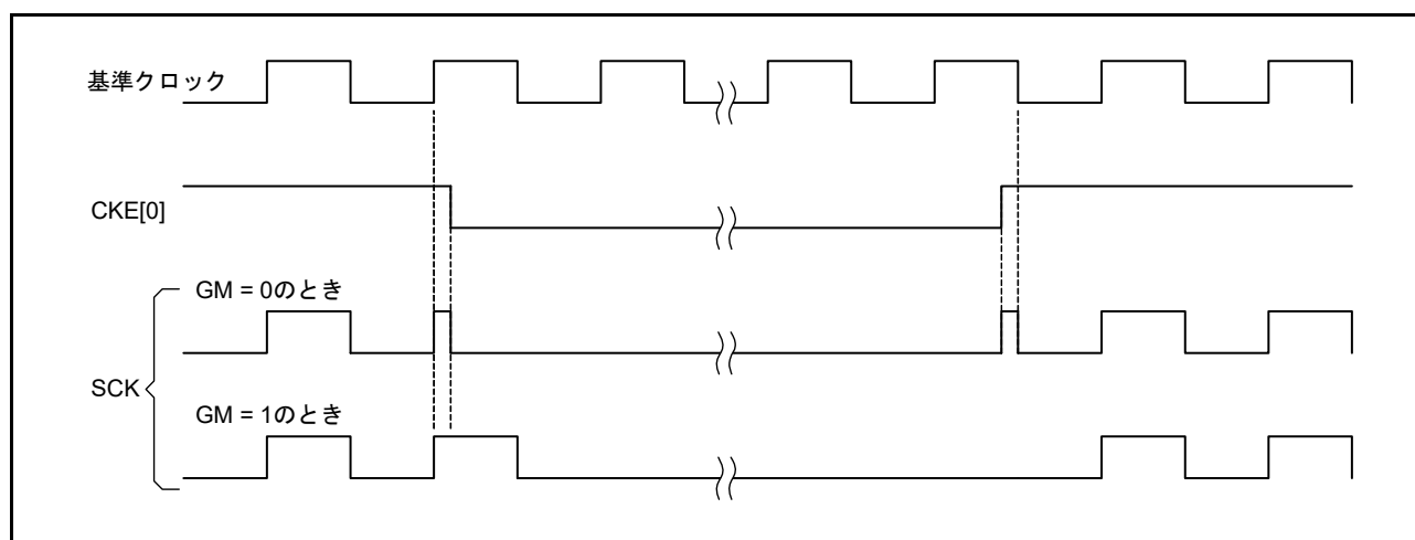
図 30.57 クロック出力制御
