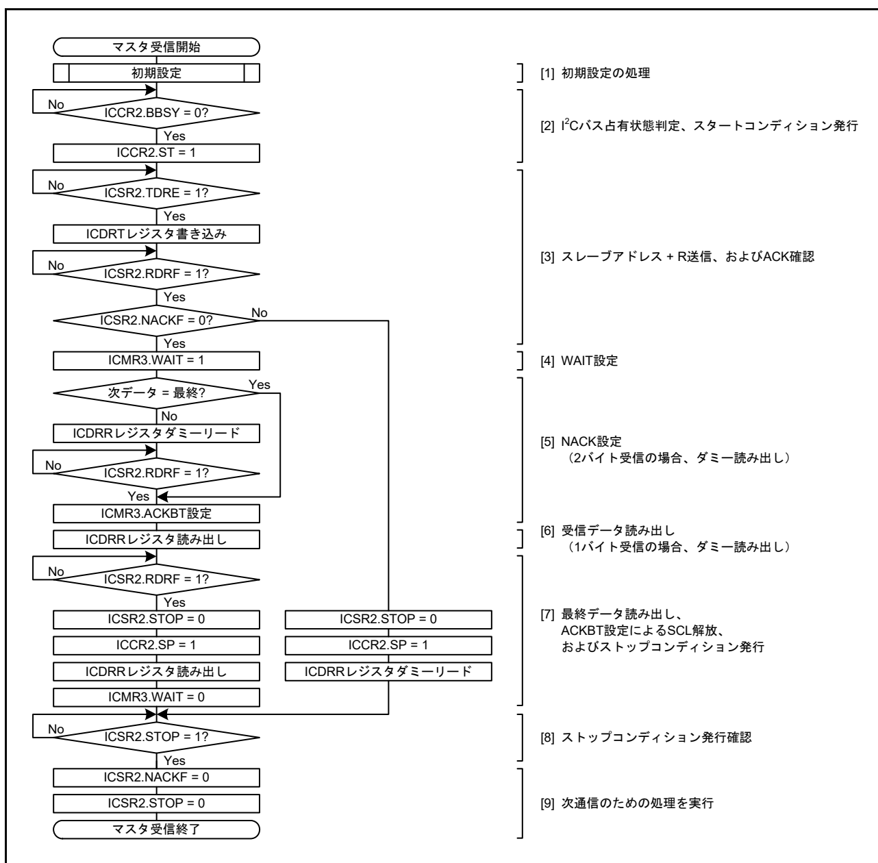
図 32.10 マスタ受信のフローチャート例 (7ビットアドレスフォーマットで1または2バイト受信の場合)
