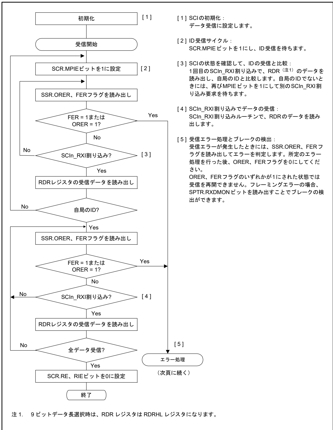
図 30.27 マルチプロセッサシリアル受信のフローチャート例 (非 FIFO 選択時) (1)
