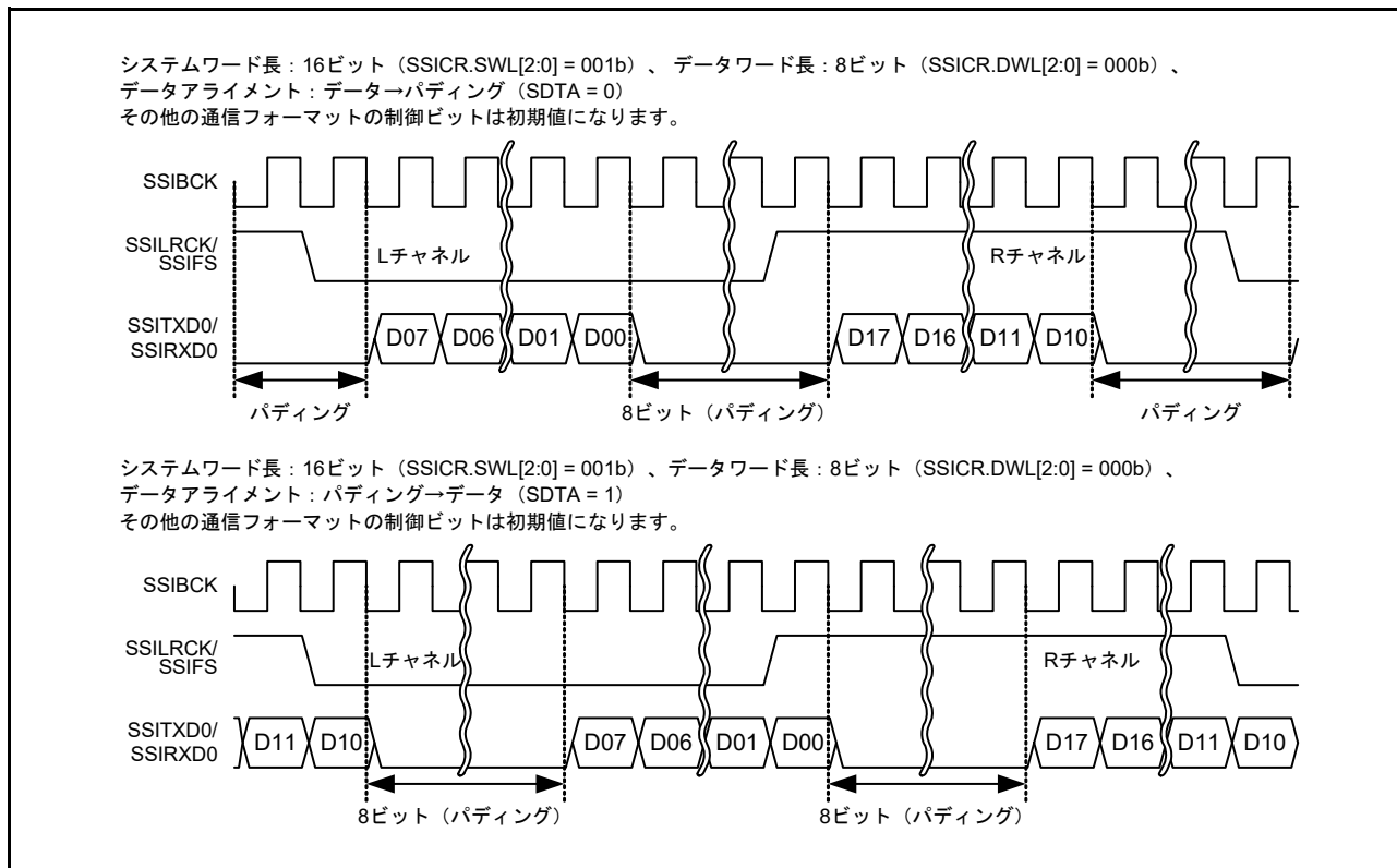
図 37.9 パディングビットのあるシリアルデータのアライメント設定
