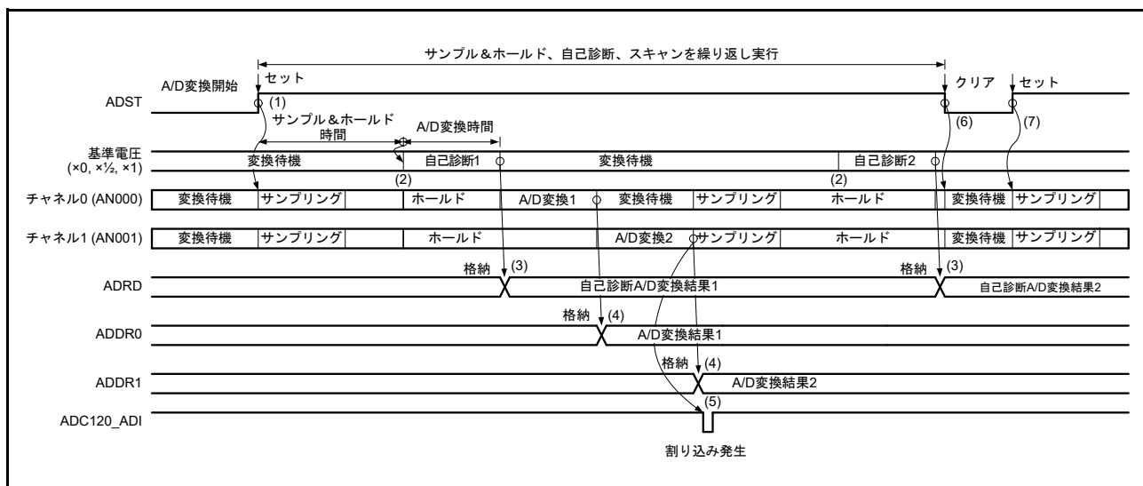
図 42.20 連続スキャンモードの動作例 (チャネル専用サンプル&ホールド回路使用、AN000 および AN001 選択 + 自己診断)
