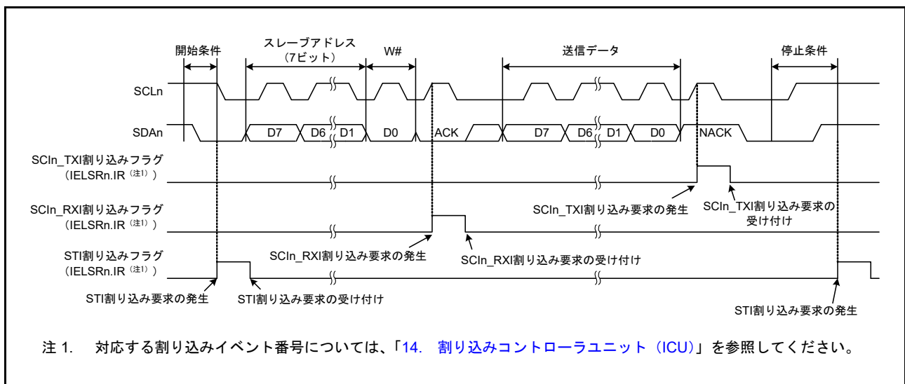
図 30.65 簡易 IIC モードにおけるマスタ送信の動作例 2 (7 ビットスレーブアドレス、ACK 割り込み、NACK 割り込み使用時)
