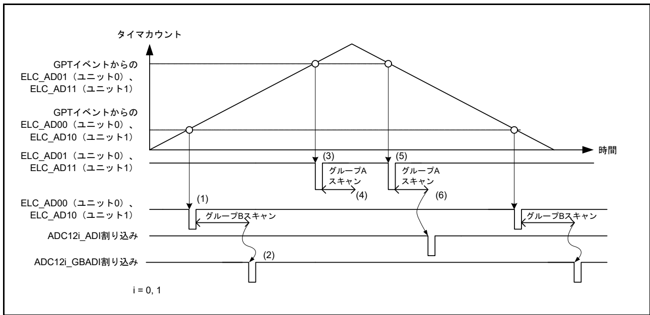
図 42.24 グループスキャンモードでダブルトリガモードを使用する場合の基本動作例 (ELC からの同期トリガ使用時)
