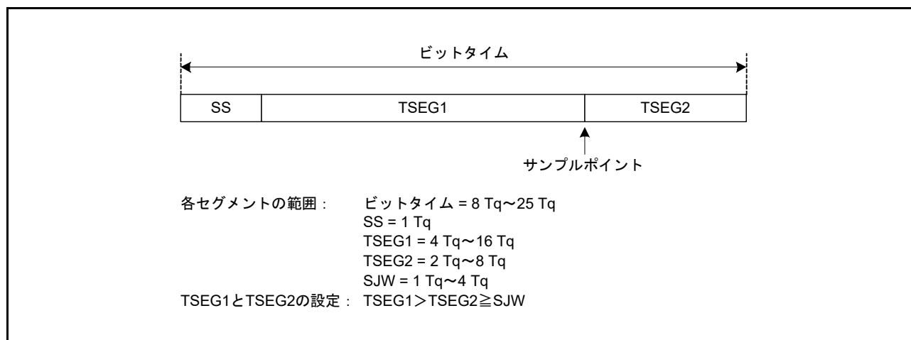
図 33.12 ビットタイミング
