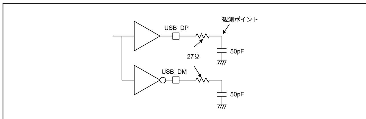
図 52.63 フルスピードモードにおける測定回路
