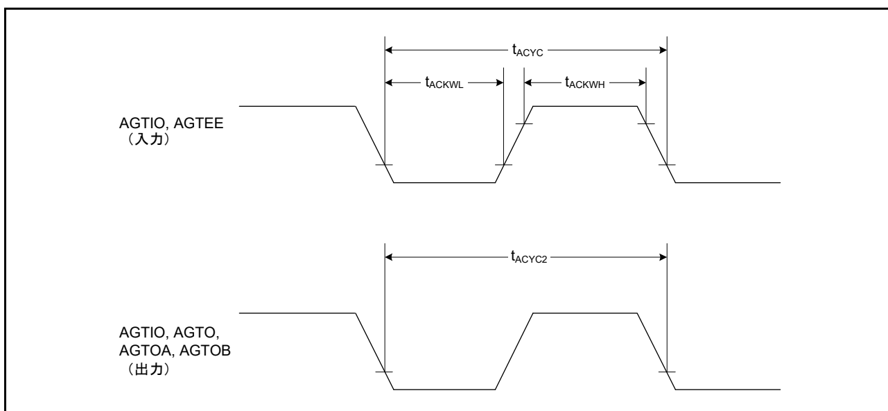
図 52.33 AGT 入出力タイミング
