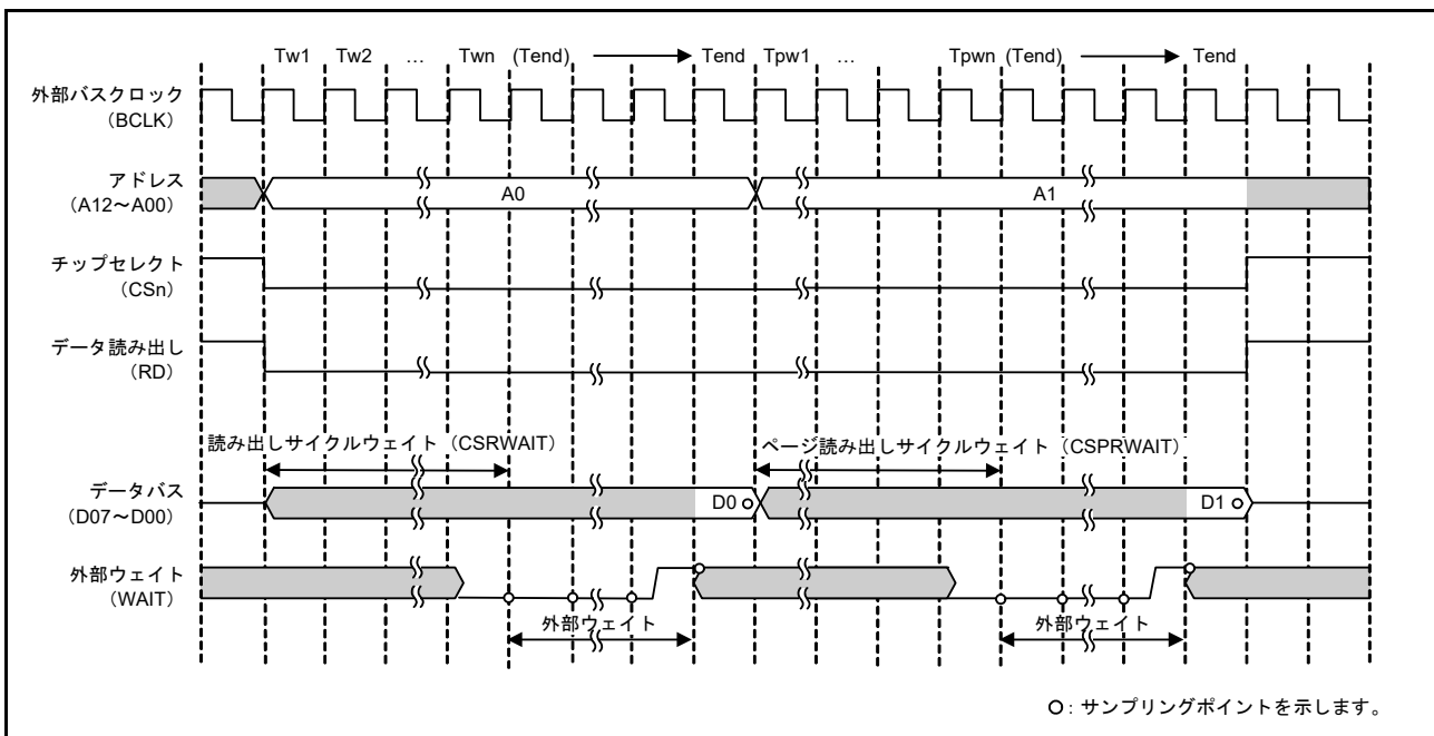
図 15.24 外部ウェイトタイミング例 (8 ビットバス空間に対するページリードアクセス、BCLK 端子出力選択ビットで BCLK の 1 分周を選択した場合) (n = 0, 1, 4 ~ 7)
