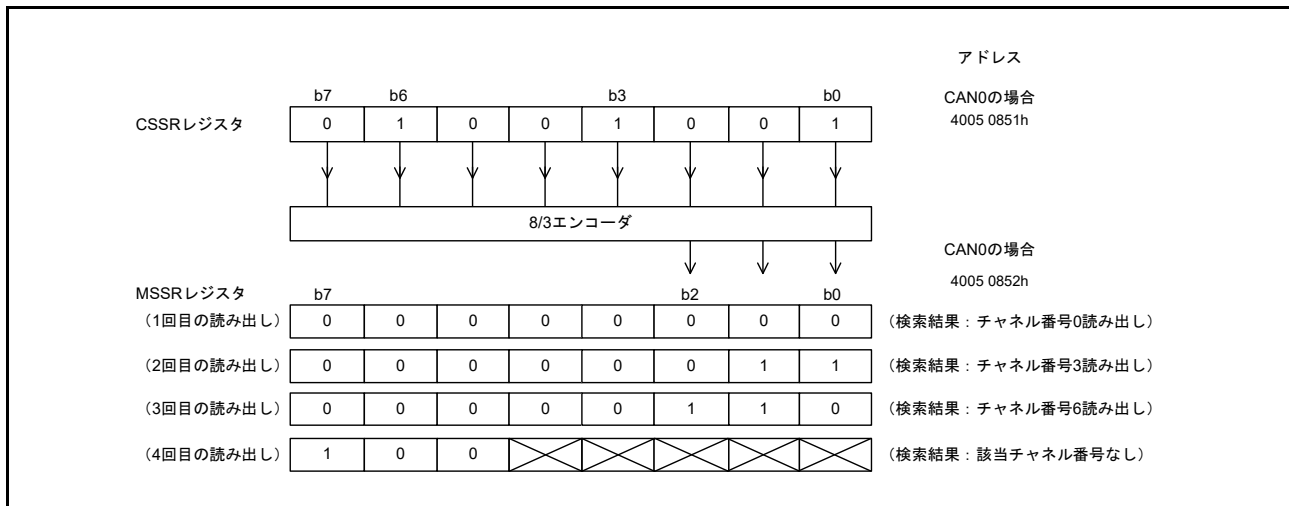
図 33.4 CSSR および MSSR レジスタに対する書き込みと読み出し
