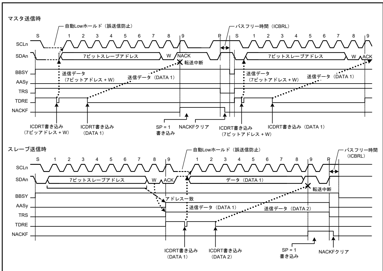
図 32.39 NACK 受信時のデータ転送中断動作 (NACKE = 1 の場合)
