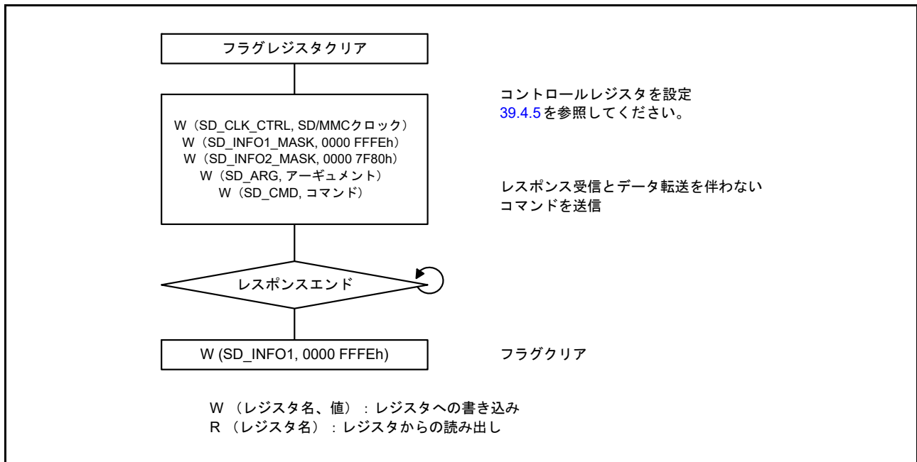
図 39.8 レスポンスまたはデータがないコマンドのフロー例
