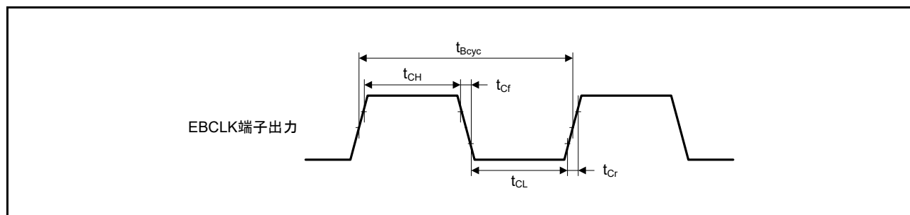
図 52.7 EBCLK 出カタイミング
