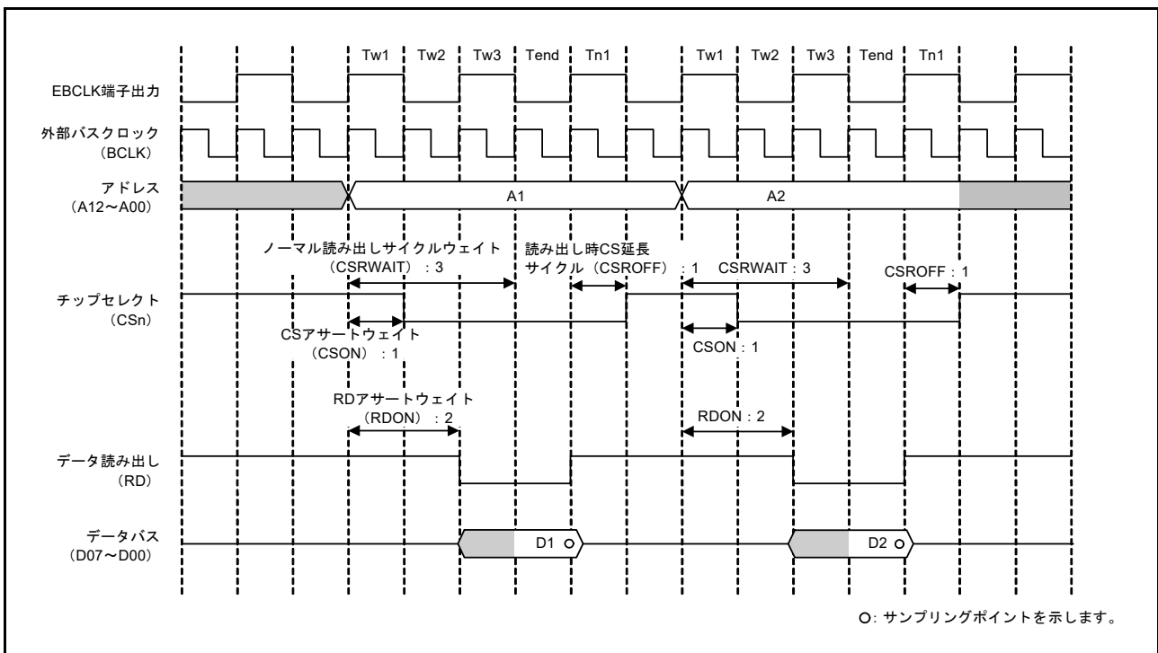
図 15.11 ノーマルリードアクセスの動作例 (EBCLK 端子出力選択ビットで BCLK の 2 分周を設定した場合) (n = 0, 1, 4 ~ 7)
