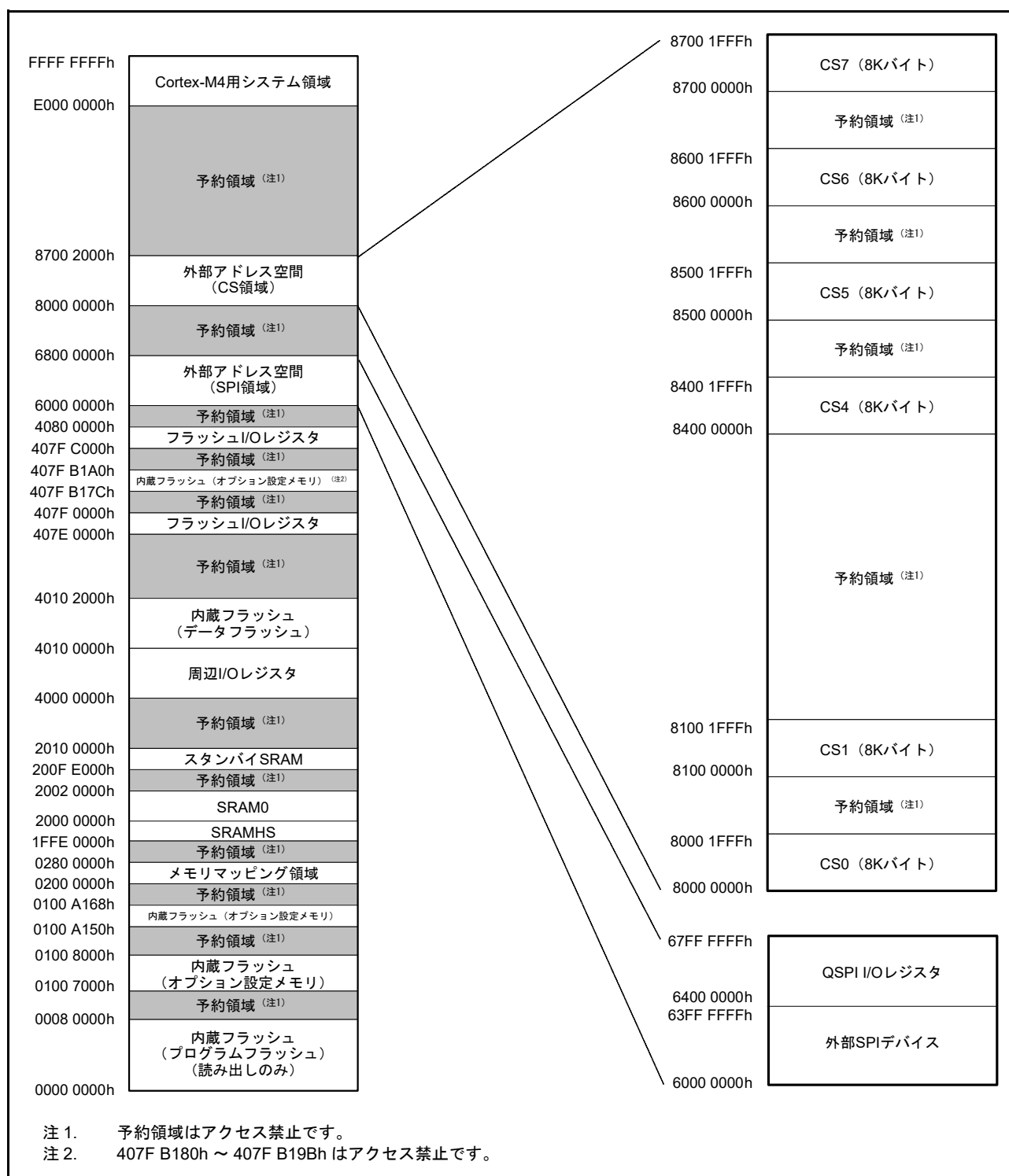
図 4.2 外部アドレス空間と CS 領域の対応
