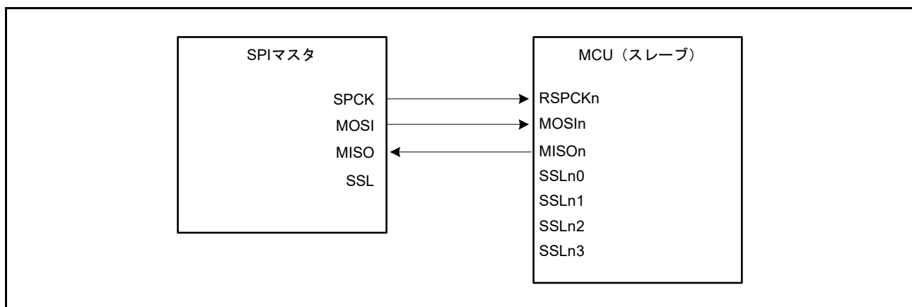
図 34.12 クロック同期式動作のマスター/スレーブの構成例 (MCU はスレーブ、CPHA = 1)
