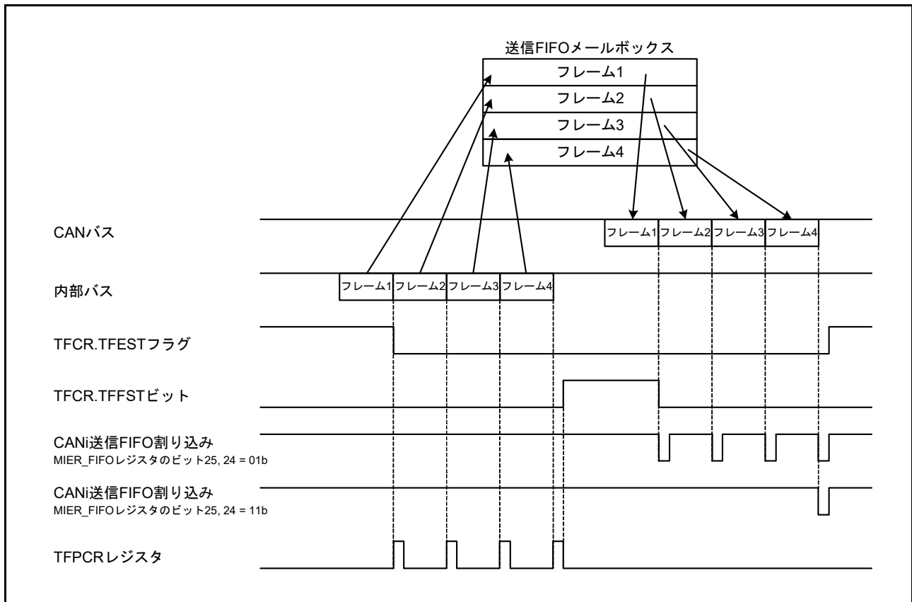
図 33.3 送信 FIFO メールボックスの動作 (MIER_FIFO レジスタのビット 25、24 が 01b または 11b のとき)
