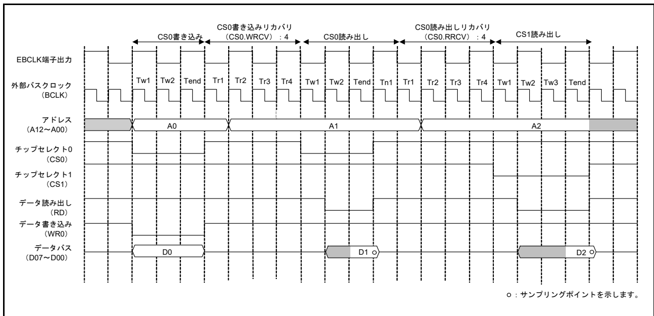
図 15.32 EBCLK 端子出力選択ビットで BCLK の 2 分周を選択した場合のリカバリサイクルの動作例 (セパレートバスインタフェースによるノーマルアクセスの場合)
