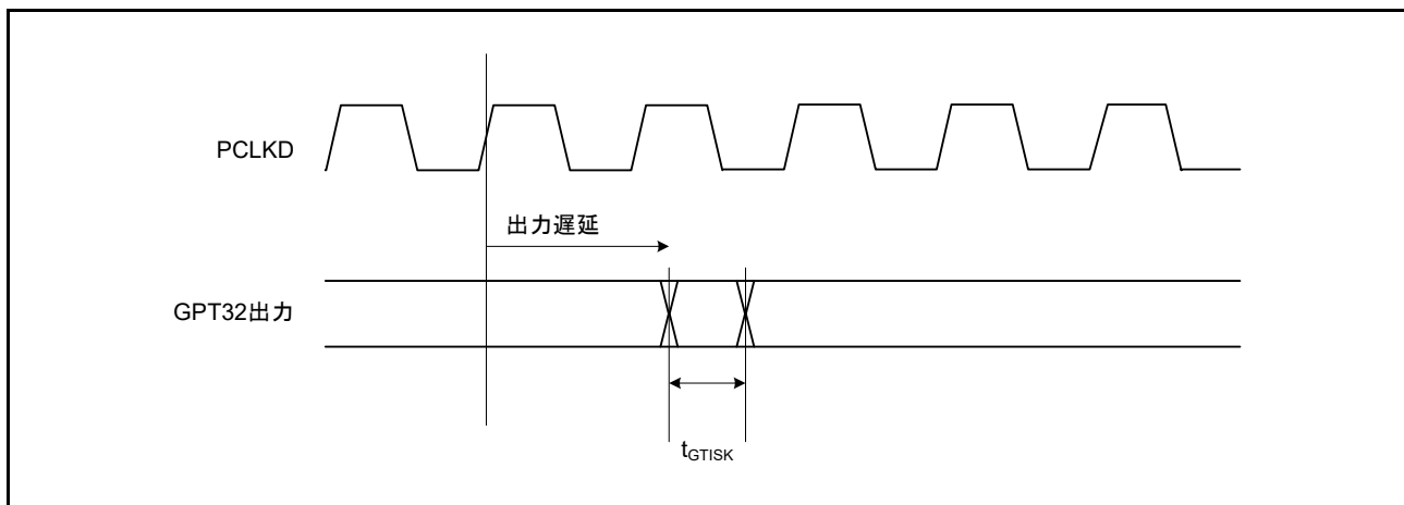
図 52.30 GPT32 出力遅延スキュー
