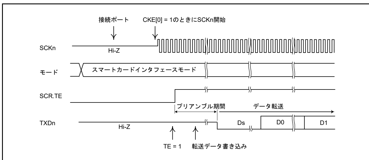
図 30.51 スマートカードインタフェースモードにおけるデータ送信のタイミング例
