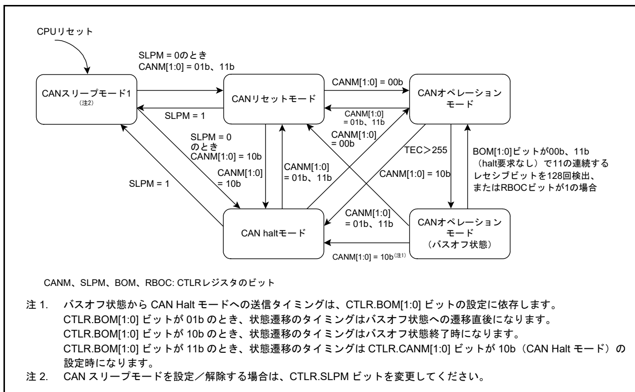
図 33.9 各動作モード間の遷移
