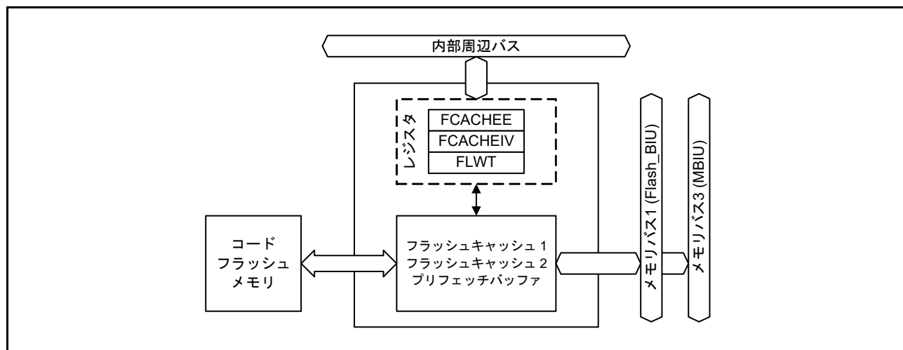
図 50.4 FCACHE のブロック図
