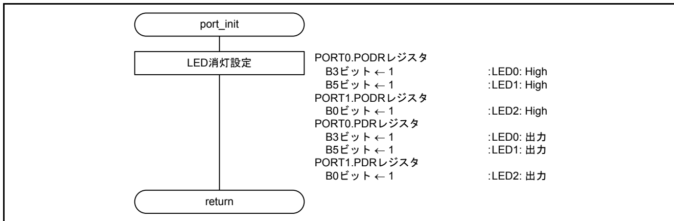
図 5.7 ポート初期設定
