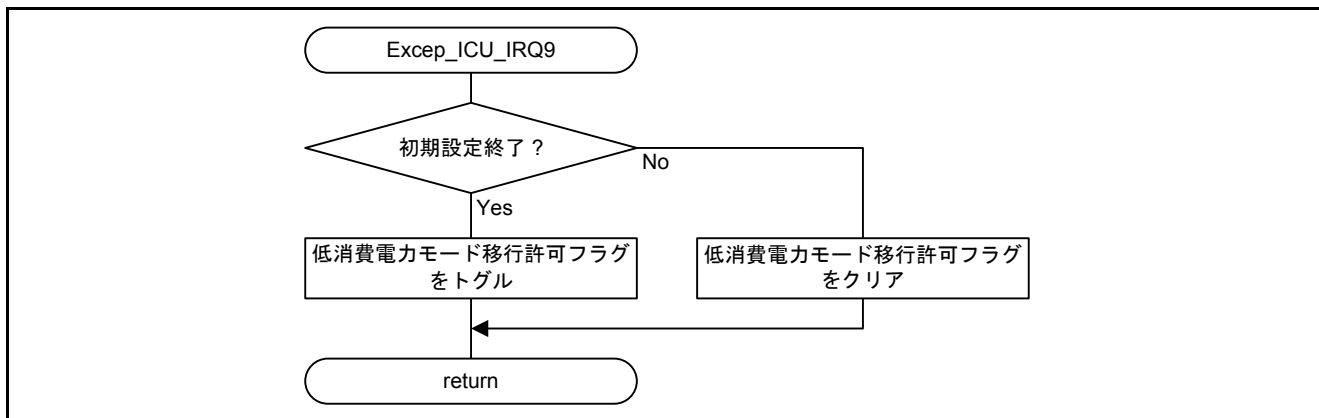
図 5.17 IRQ9 割り込み処理
