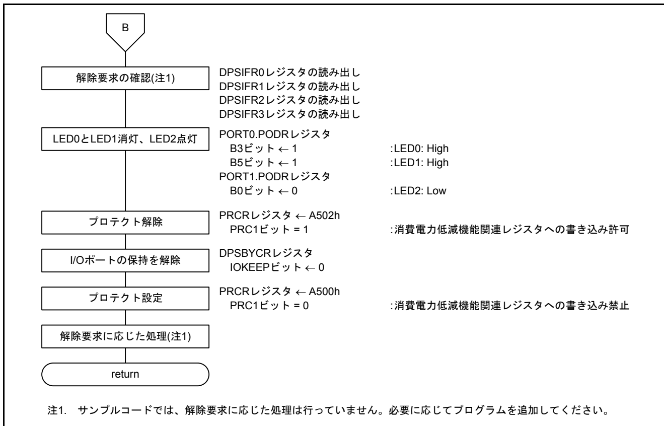
図 5.14 ディープソフトウェアスタンバイモード移行(3/3)
