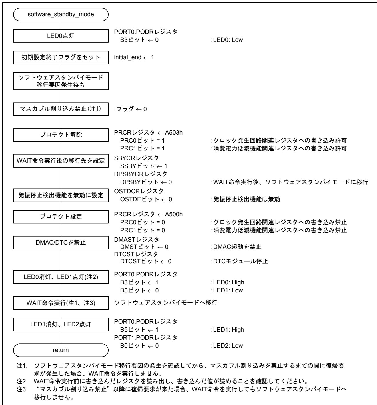
図 5.11 ソフトウェアスタンバイモード移行
