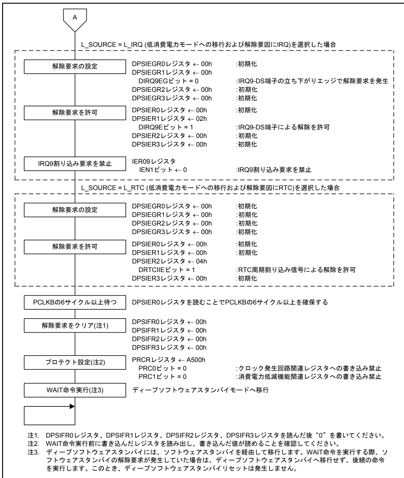
図 5.13 ディープソフトウェアスタンバイモード移行(2/3)
