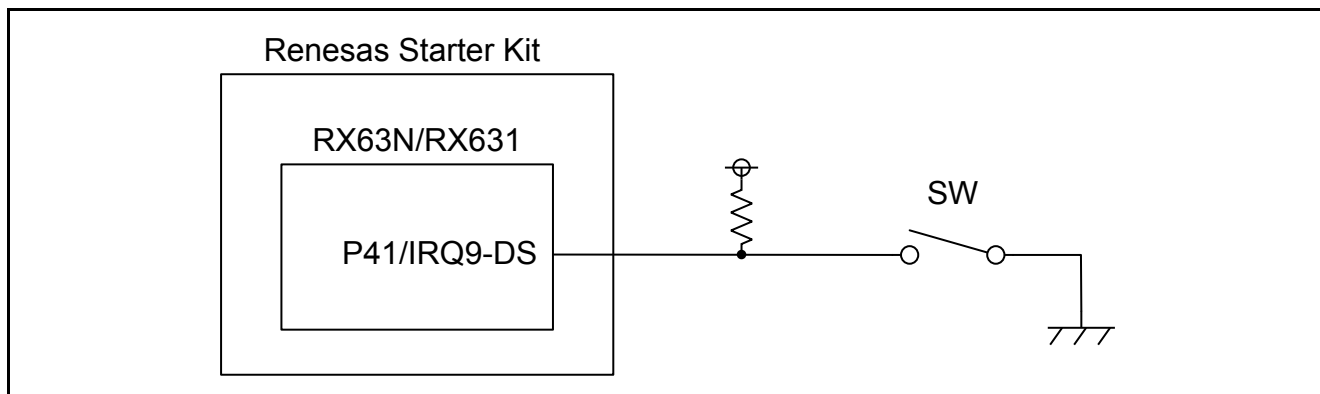
図 4.1 接続例
