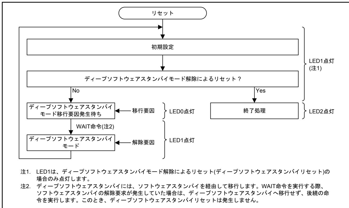
図 5.3 ディープソフトウェアスタンバイモードの動作概要
