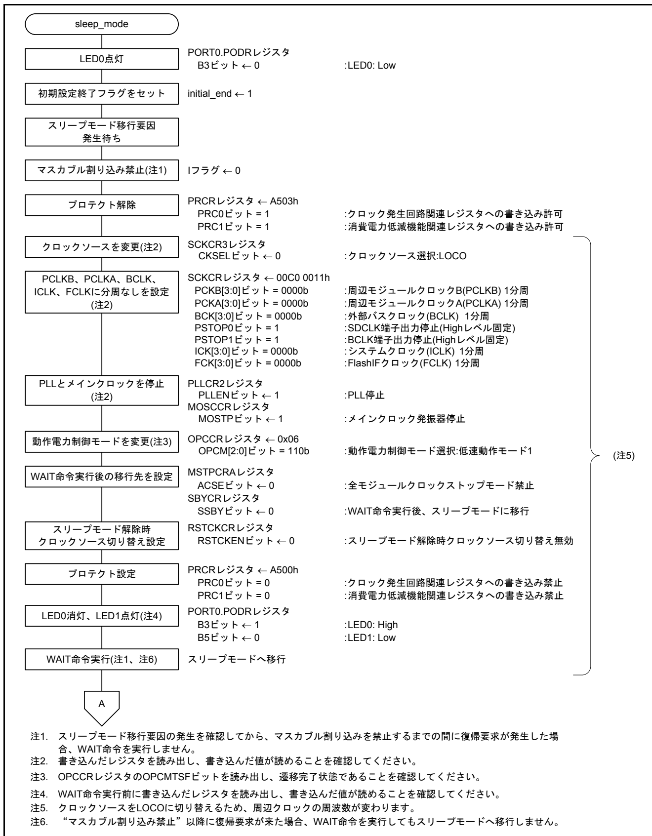
図 5.9 スリープモード移行(1/2)
