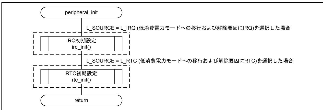
図 5.8 周辺機能初期設定
