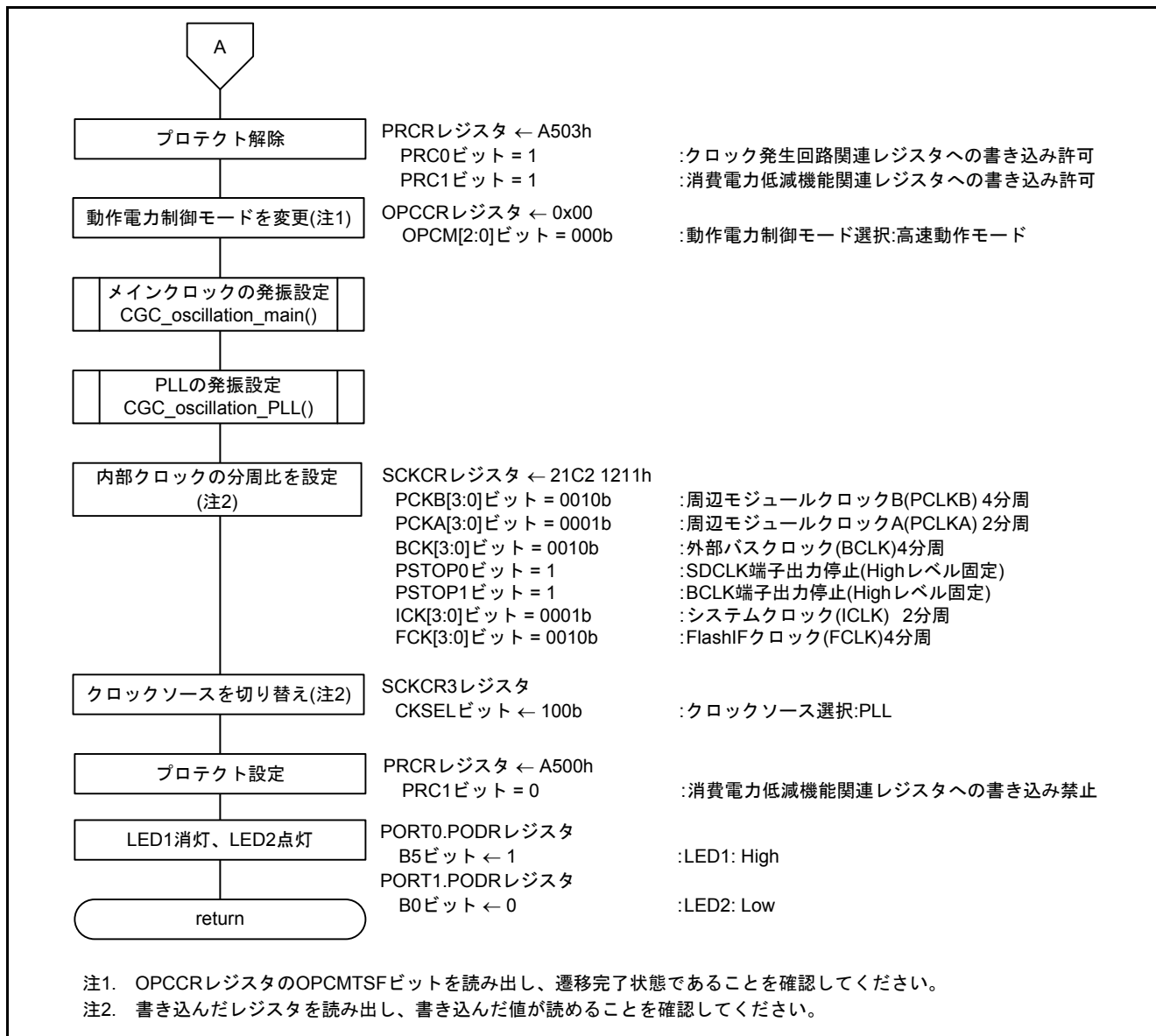
図 5.10 スリープモード移行(2/2)
