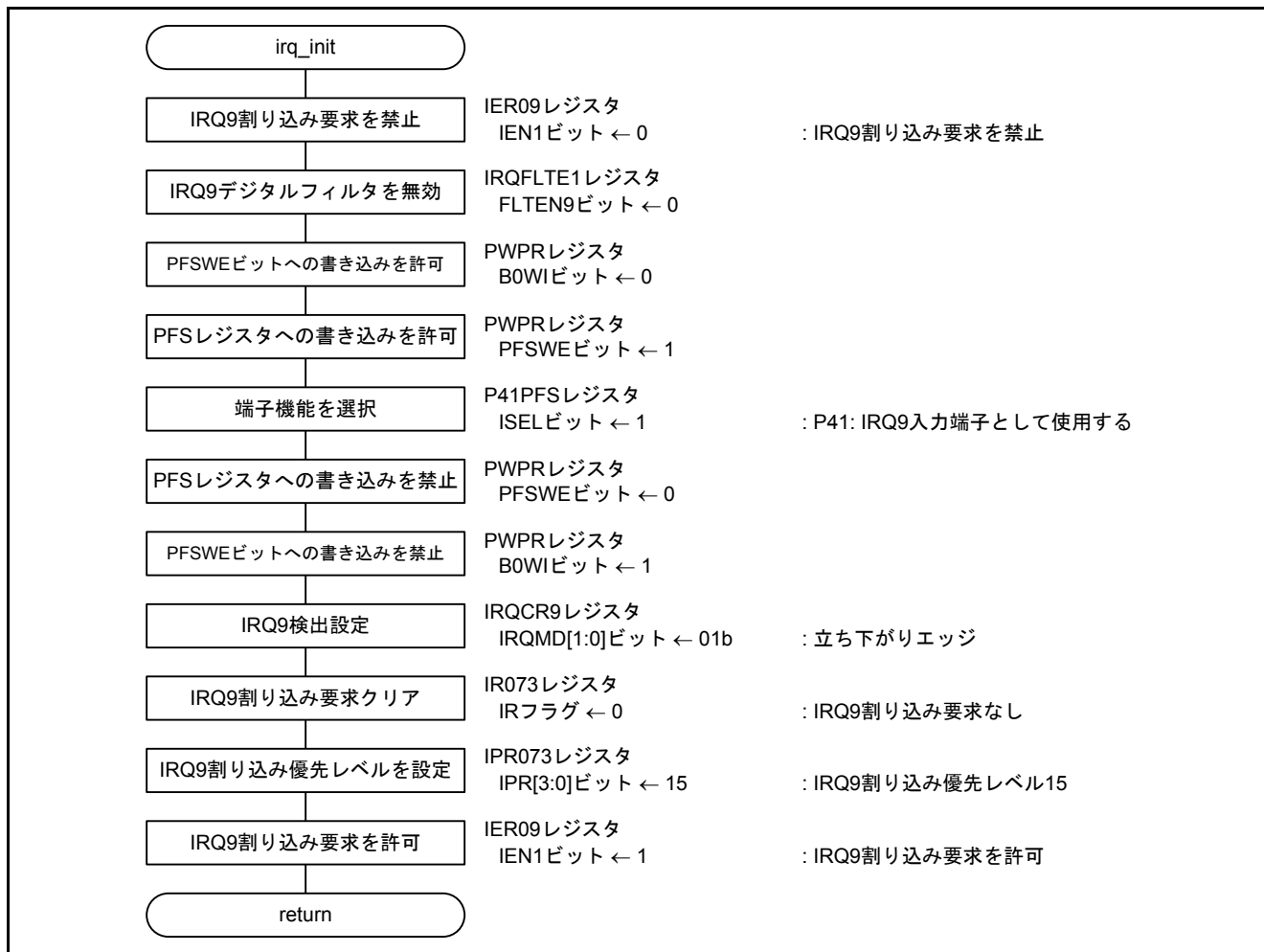
図 5.15 IRQ 初期設定
