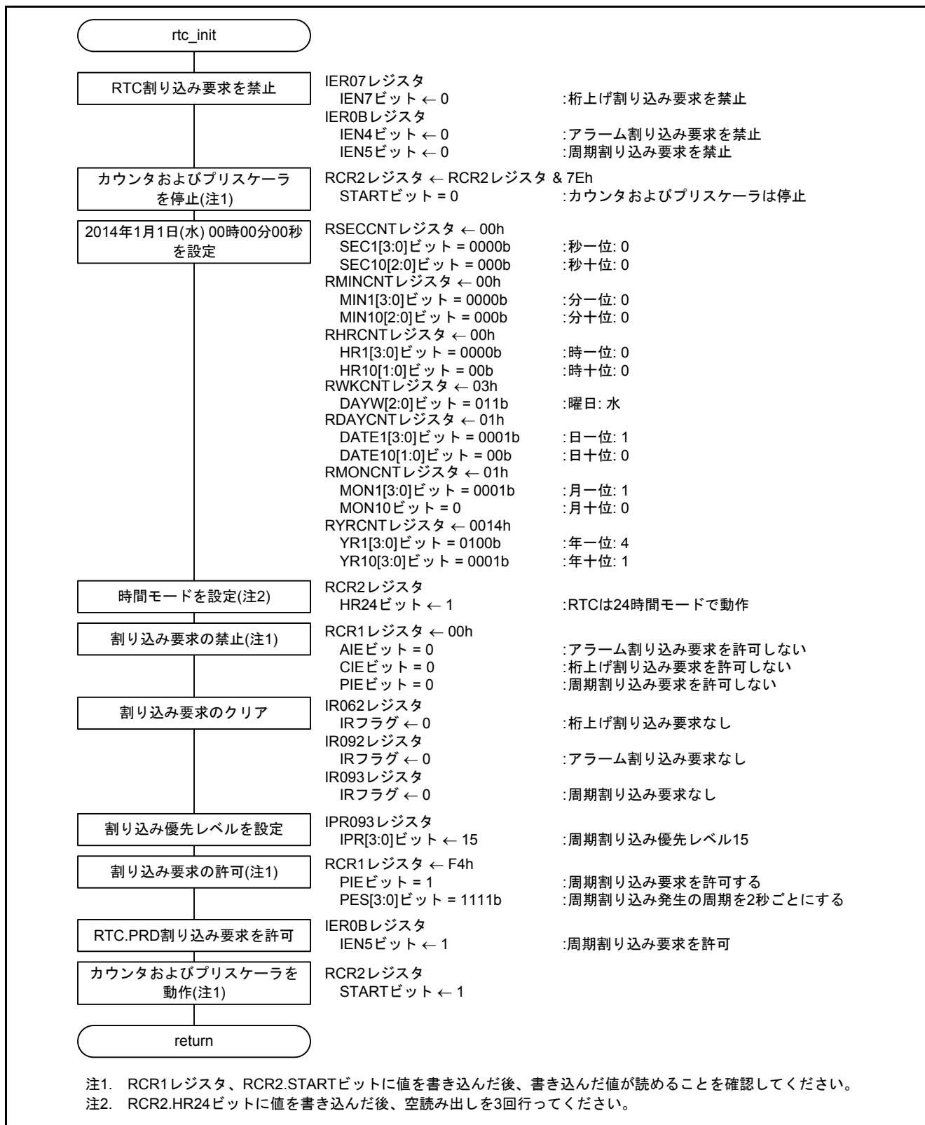
図 5.16 RTC 初期設定
