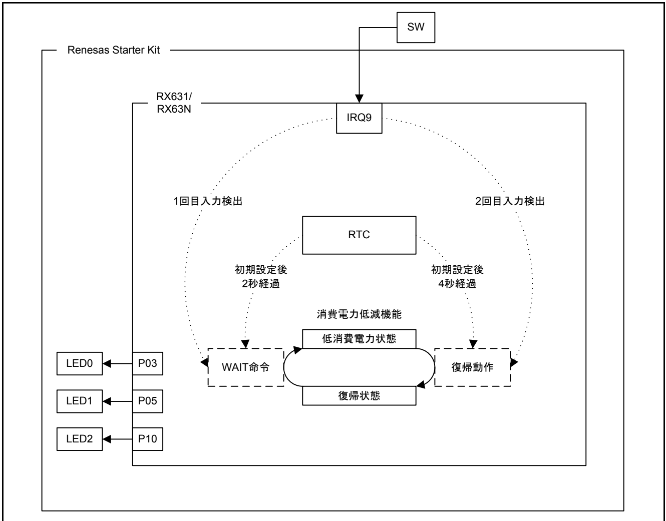
図 1.1 ブロック図
