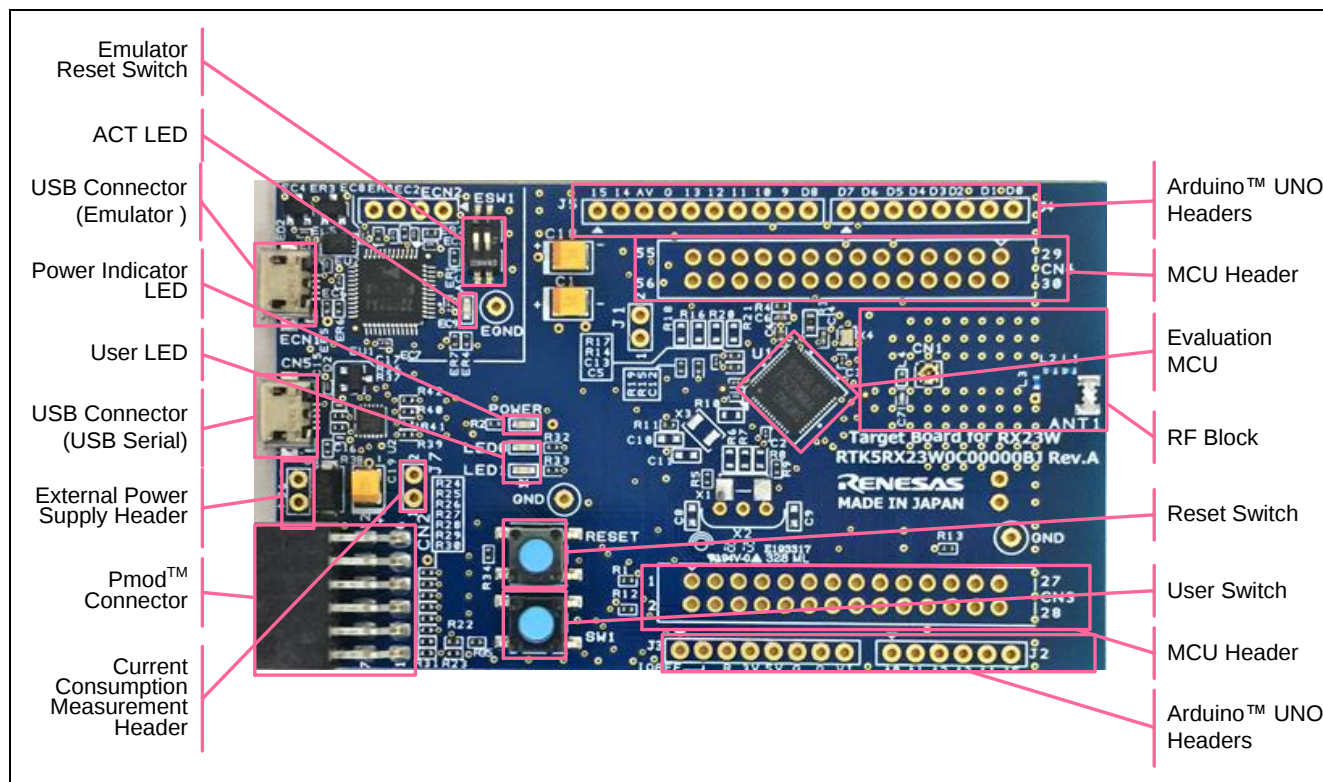
図 1-1 Target Board 外観
