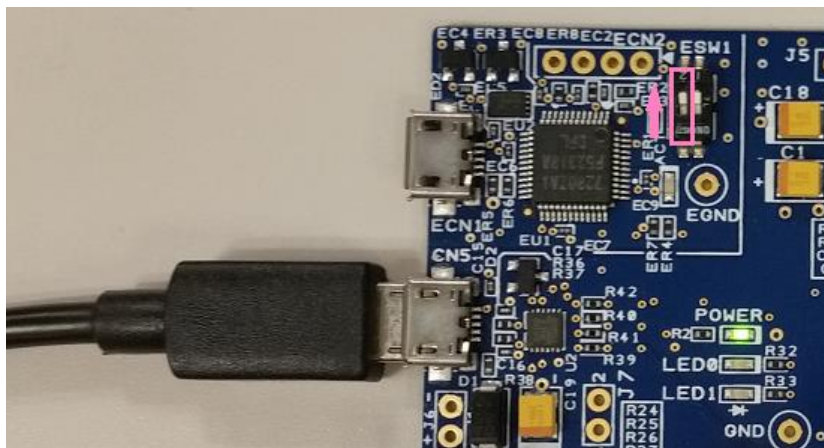
図 2-1 USB コネクタ CN5
