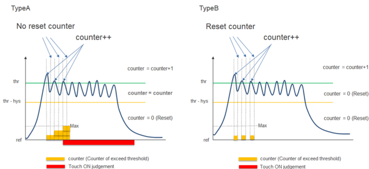
図 1 チャタリング抑制動作例
