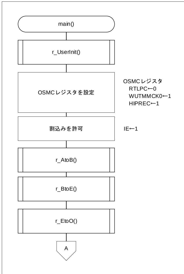
図 4-2 メイン処理 (1/2)
