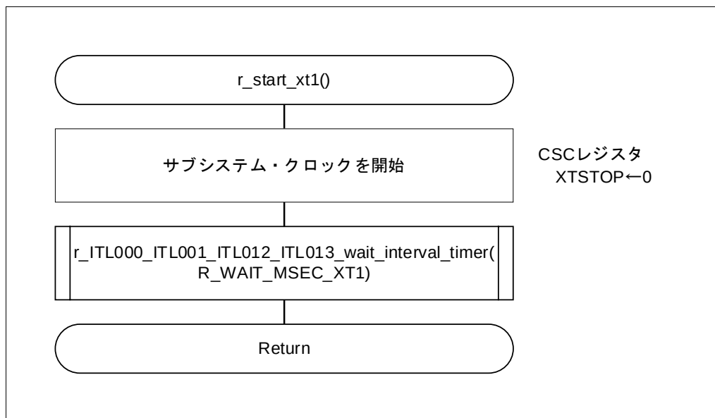
図 4-54 サブシステム・クロック動作開始
