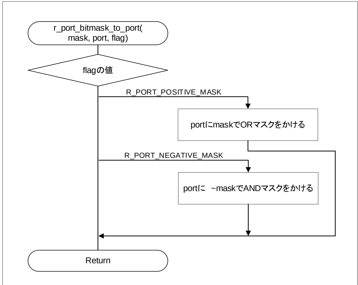
図 4-74 ポート出力制御
