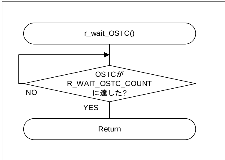
図 4-65 ウェイト処理 (OSTC レジスタ)
