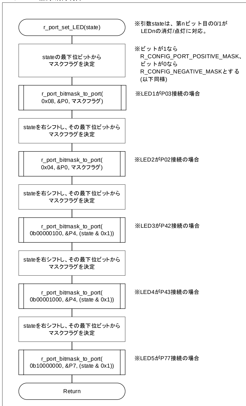
図 4-73 LED 点灯/消灯制御
