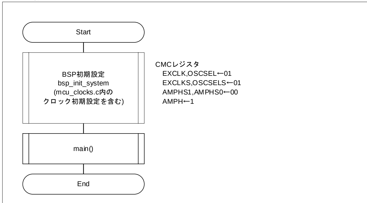
図 4-1 全体フロー
