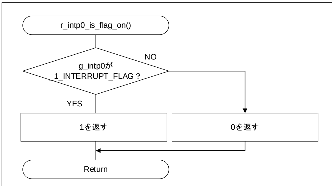
図 4-70 INTP0 割込みフラグ確認
