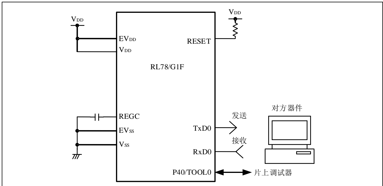
图 4.1 硬件配置
