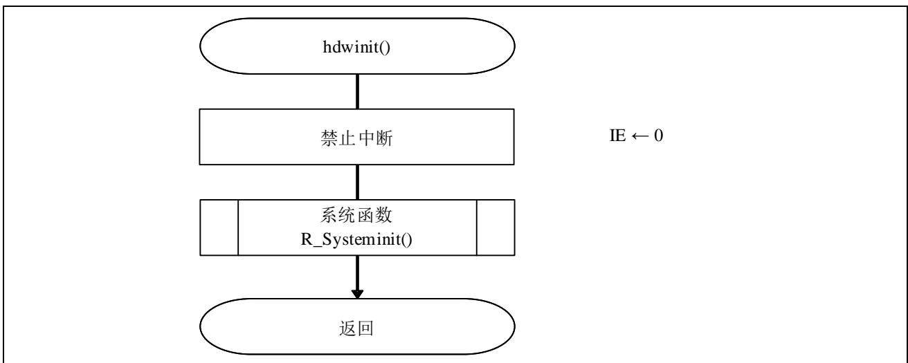
图 5.2 初始化函数
