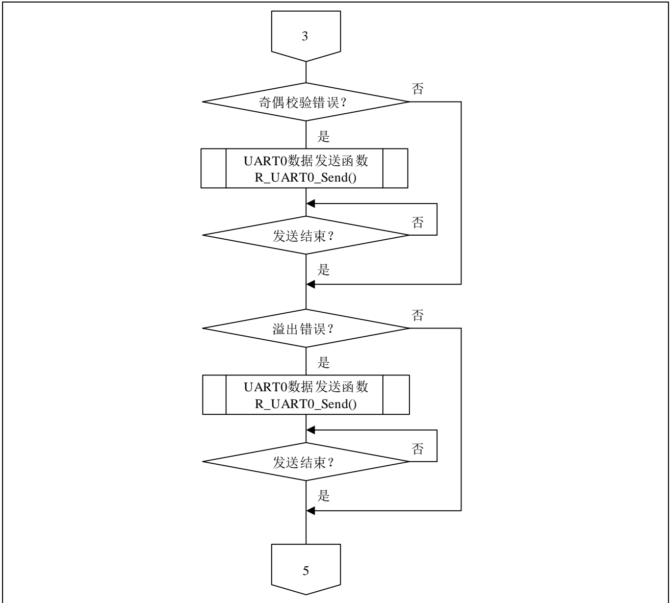
图 5.11 主函数处理 (2/3)
