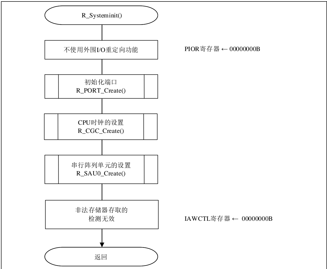
图 5.3 系统函数
