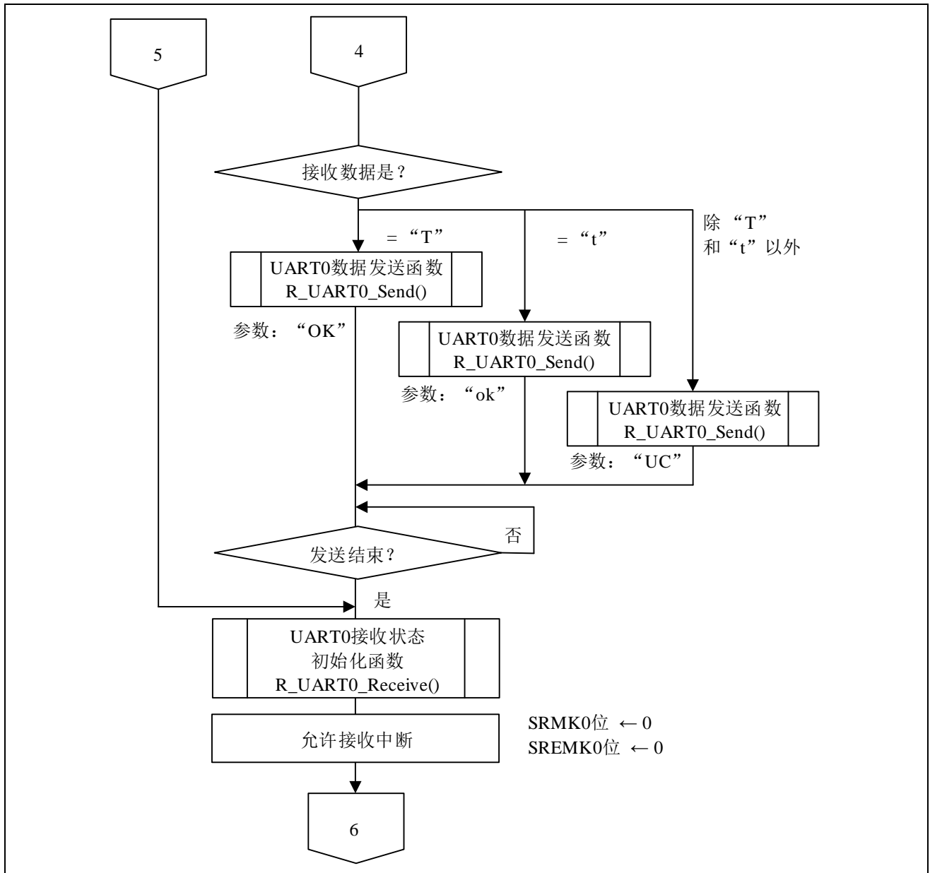
图 5.12 主函数处理 (3/3)
