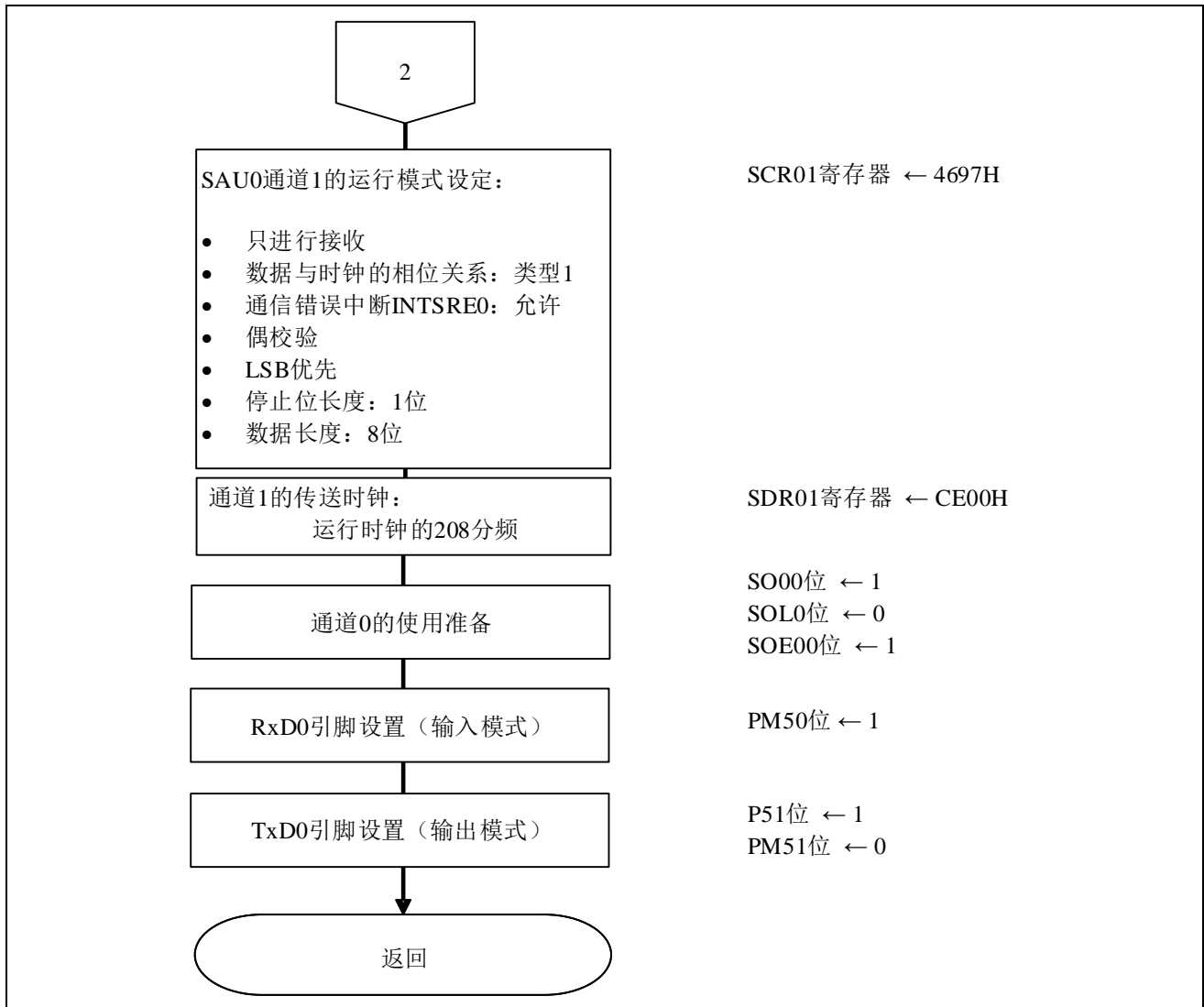
图 5.9 UART0 的设置 (3/3)
