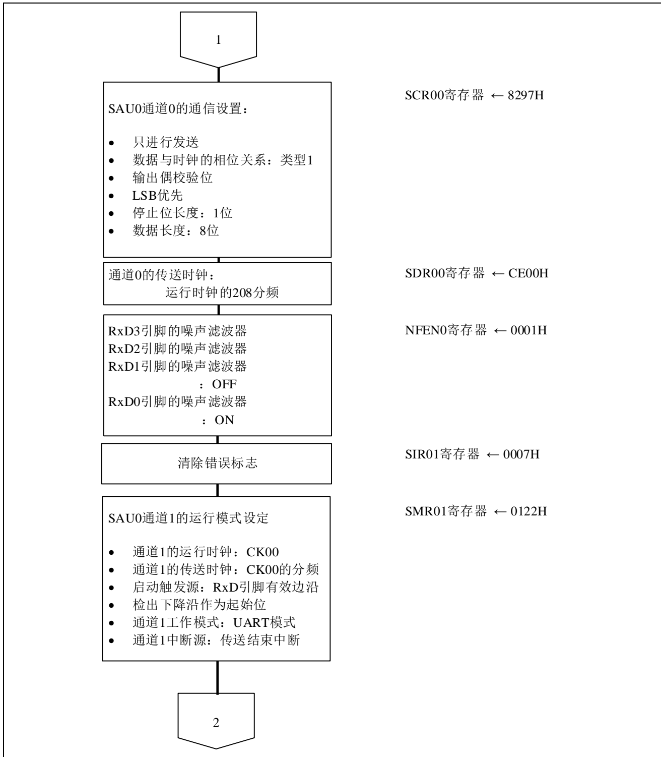
图 5.8 UART0 的设置 (2/3)
