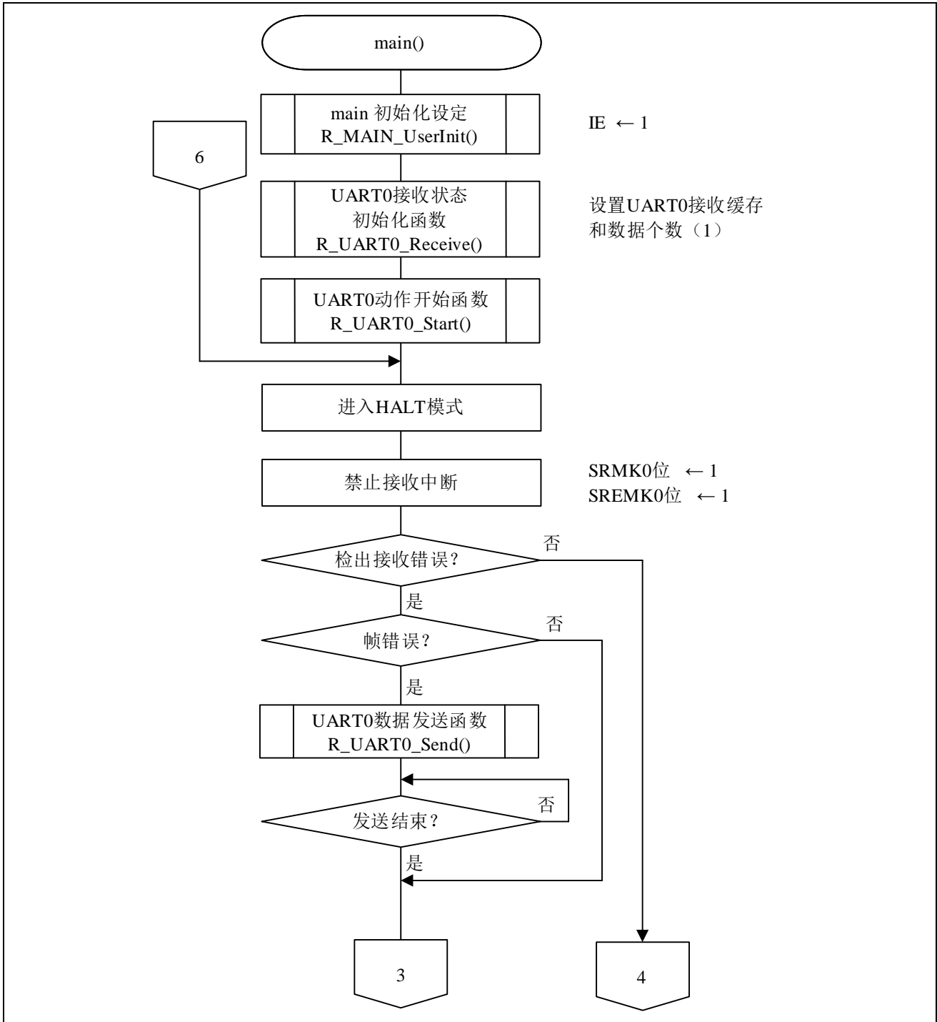
图 5.10 主函数处理 (1/3)
