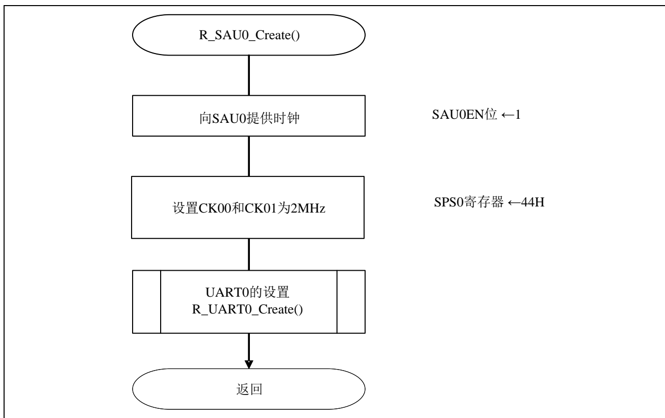
图 5.6 SAU0 的设置
