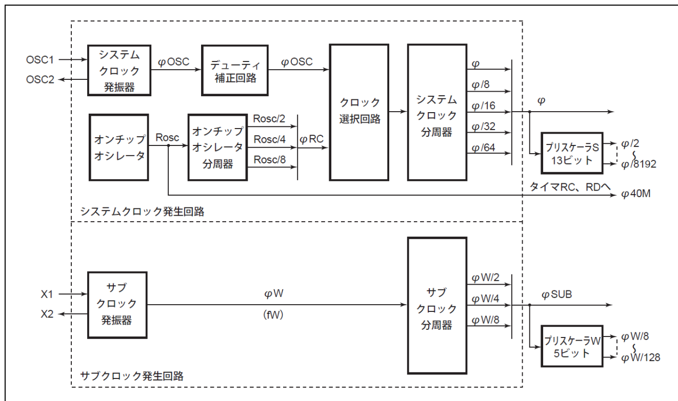
図 1.2 RL78/G14 のクロック発生回路のブロック図
