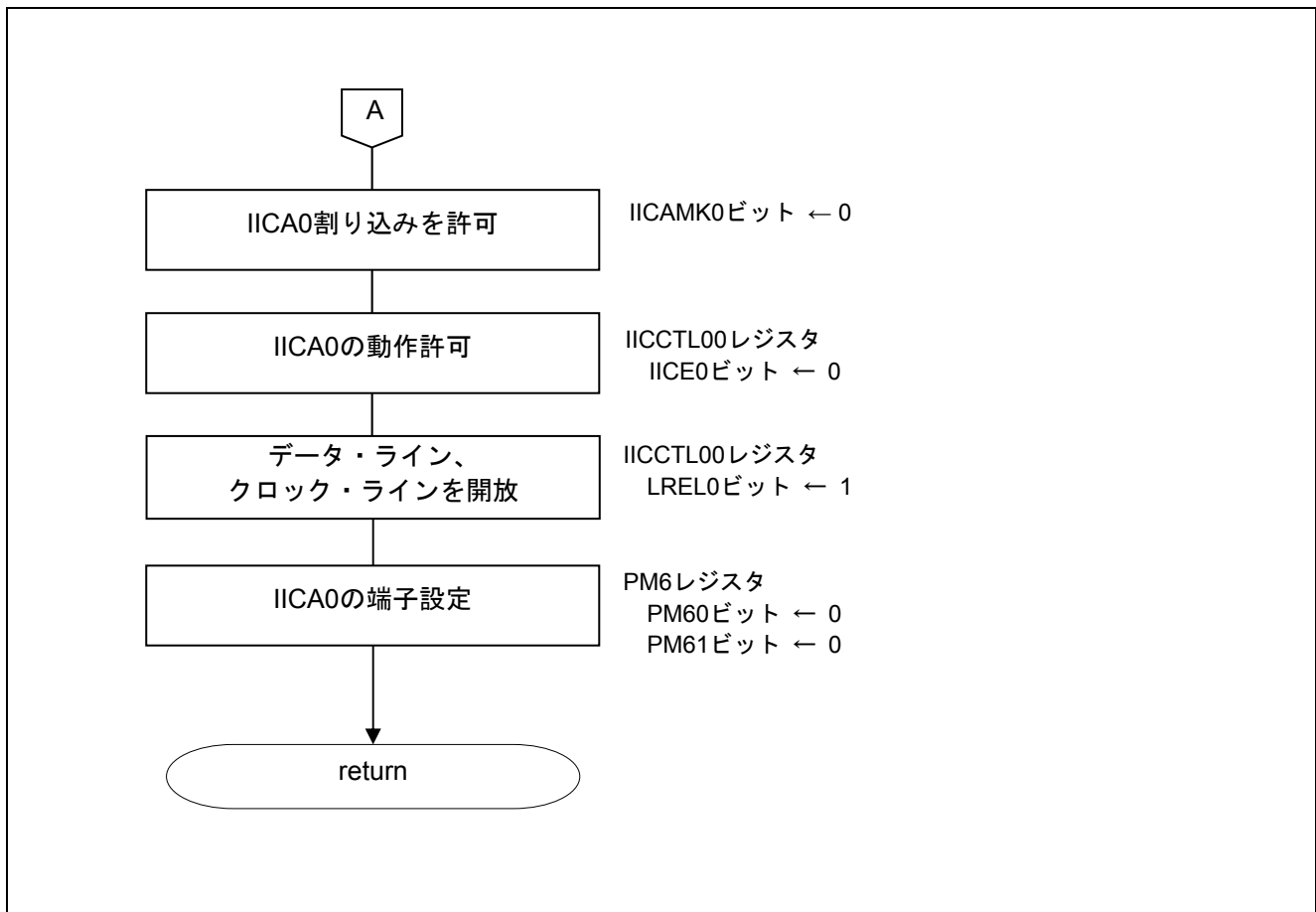
図 5.7 シリアル・インタフェース IICA の設定 (2/2)
