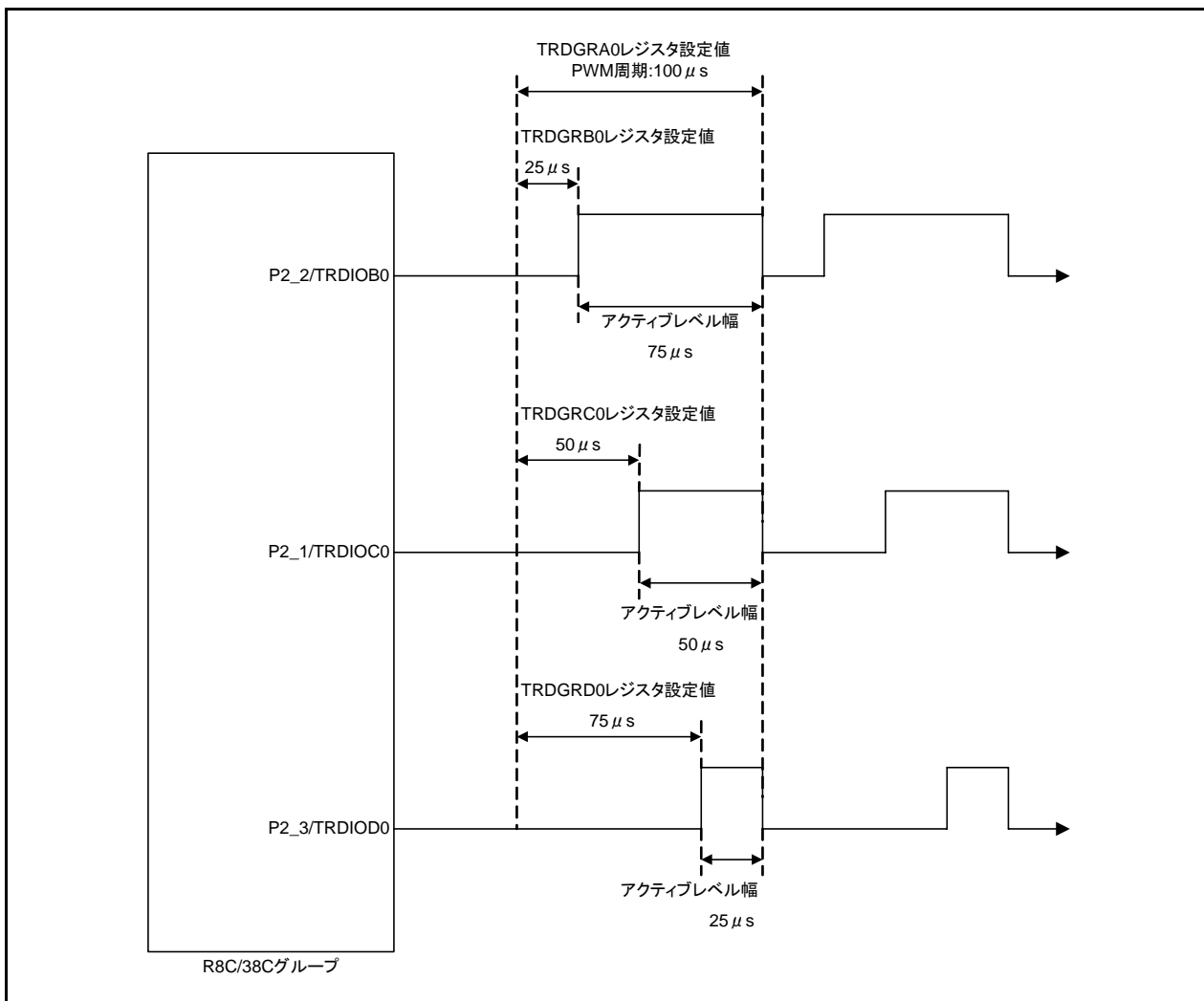
図 3.2 出力タイミング図
