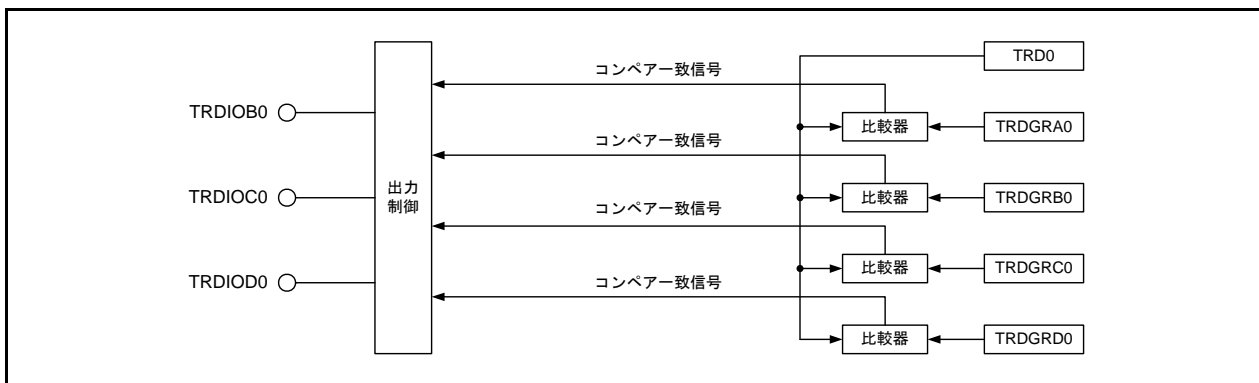
図 3.1 ブロック図
