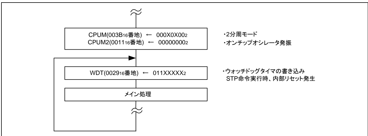
図 3.3 制御手順
