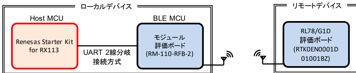
図 2-1 システム構成(1) (RY7011)
